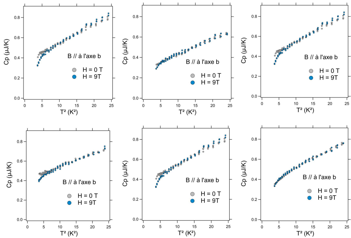
Figure 6.2 Mesures de chaleur spécifique de six échantillons monocristallins bruts de croissance de compositions \text{SrCuO}_2 à 0 T et à 9 T avec le champ appliqué perpendiculairement à l'axe des chaînes de spins (axe b ).
