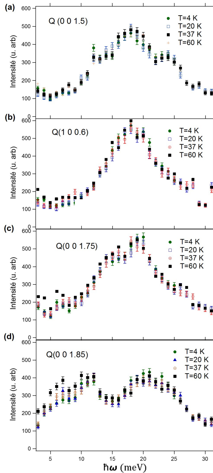
Figure 5.13 Évolution des scans à Q -constant en fonction de la température pour le composé SrCu_{0.99}Mg_{0.01}CuO_2 à T=4, 20, 37 et 60\text{ K} pour (a) Q(0\ 0\ 0.5) (b) Q(0\ 0\ 1.6) (c) (0\ 0\ 1.75) (d) (0\ 0\ 1.85) .
