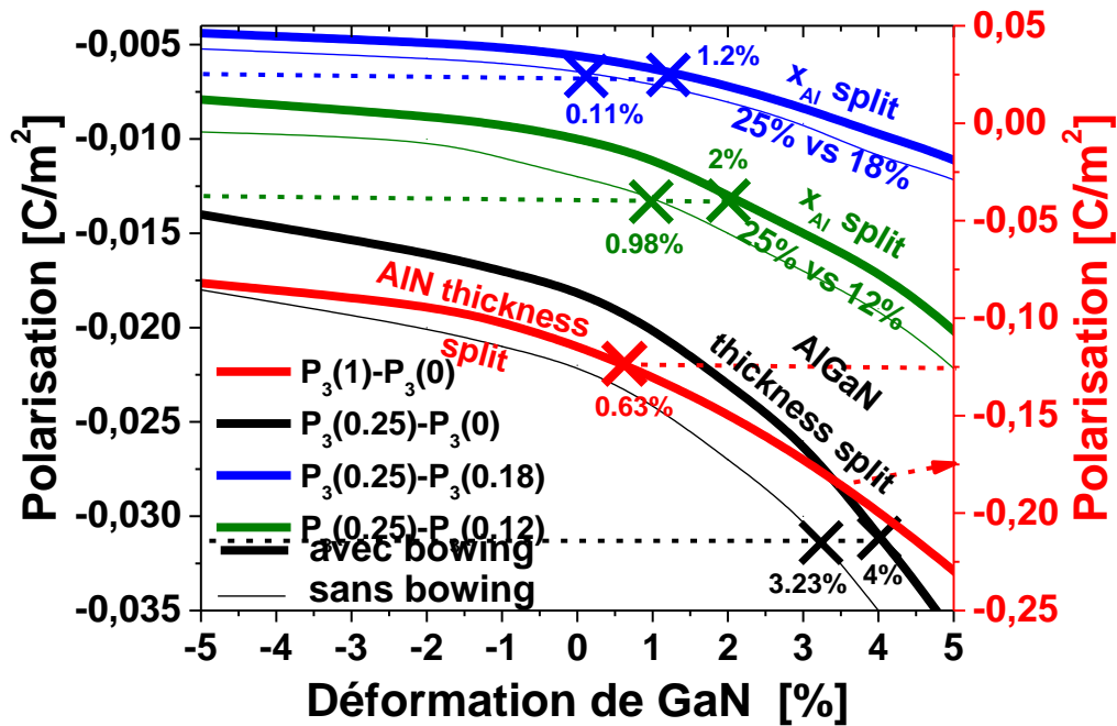
Figure 13 : Différence de polarisation totale calculée (spontanée+piézoélectrique) pour des couches \text{Al}_x\text{Ga}_{1-x}\text{N} déposées sur la couche GaN active et cela, en fonction de la déformation de GaN. Des valeurs expérimentales (crois) obtenues avec la figure 9 sont rapportées.
