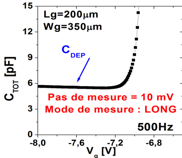
Figure 5 : Zoom sur la figure 4.a autour de la capacité de déplétion, montrant quelques précautions expérimentales nécessaires pour réussir une mesure C_{TOT} .
