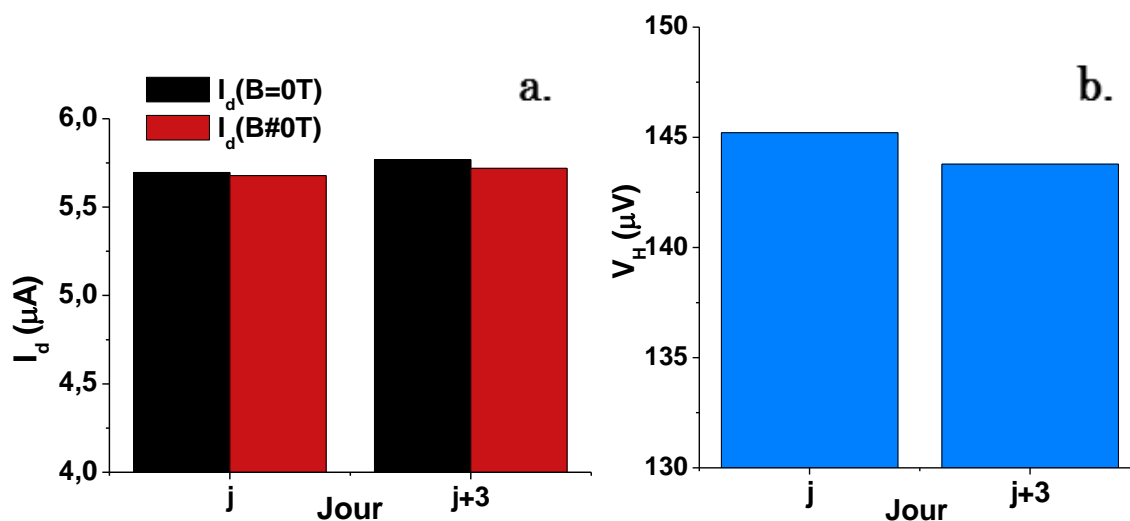
Figure 9 : Valeurs typiques mesurées à deux jours différents et à V_g=0 V sur une barre de Hall de la plaque D du a : courant de drain I_d , b : tension de Hall V_H .
