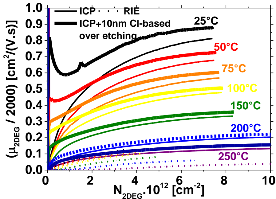
Figure 13 : Caractéristiques \mu_{\text{eff}}(N_{2\text{DEG}}) pour des températures variant de 25 à 250 °C pour le lot d'étude destiné à l'analyse de l'influence du type du procédé de gravure utilisé pour graver la couche de passivation \text{Si}_3\text{N}_4 .
