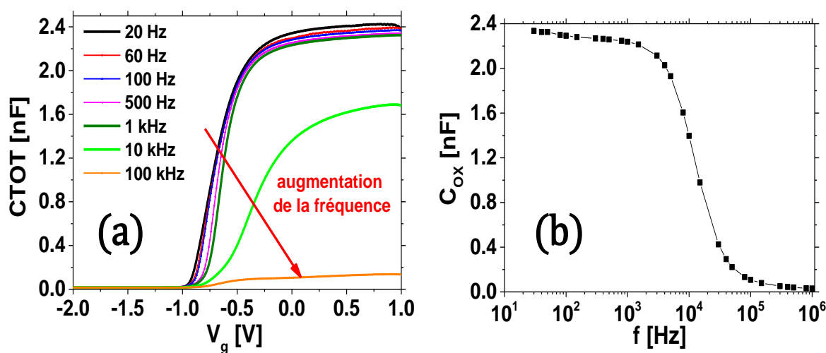
Figure 16 : (a) caractéristiques C_{TOT}(V_g) d'un échantillon brut sans métallisation pour différentes fréquences. (b) C_{Ox} en fonction de la fréquence de la mesure, C_{Ox} diminue avec l'augmentation de la fréquence.
