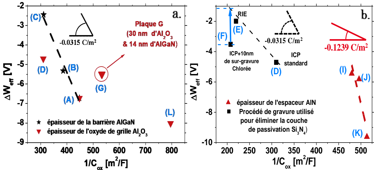
Figure 9 : \Delta W_{\text{eff}} en fonction de 1/C_{\text{ox}} pour les variantes technologiques faisant varier successivement a : l'épaisseur d' \text{AlGaN} et d' \text{Al}_2\text{O}_3 . b : l'épaisseur d' \text{AlN} et du procédé de gravure utilisé pour éliminer la couche de passivation \text{Si}_3\text{N}_4 .
