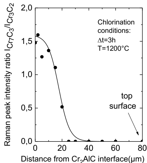
Figure 22. Rapport entre le pic Raman Cr_7C_3 à 275 \text{ cm}^{-1} et le pic Raman Cr_3C_2 à 208 \text{ cm}^{-1} en fonction de la distance de l'interface Cr_2AlC . Température de chloration T = 1200^\circ C et temps \Delta t = 3h . La ligne continue est un guide aux yeux.
