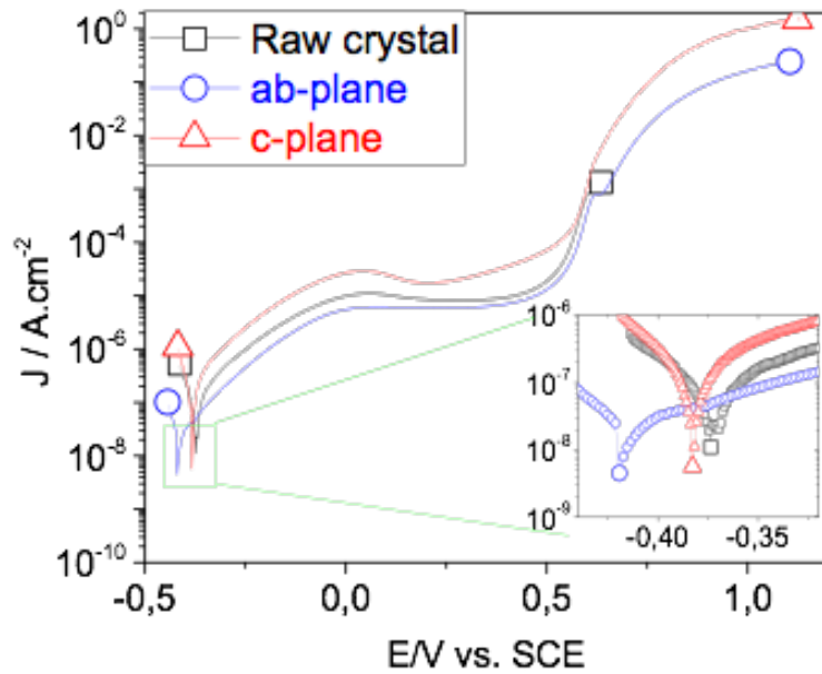
Figure 13. Courbes de polarisation de l'échantillon Cr 2 AlC dans 1M H 2 SO 4 d'OCP à + 1.5V par rapport à l'OCP: plan-c (triangle) plan ab (rond) cristal brut (carré).
