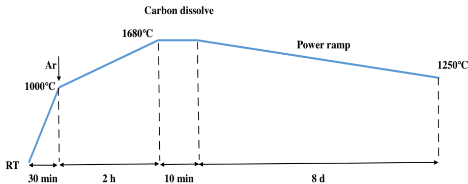
Figure 4. Processus entier de la croissance en solution à haute température.
