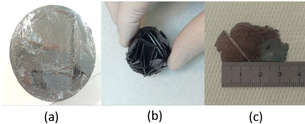
Figure 5. Différentes étapes après le refroidissement ( \text{Cr}_2\text{AlC} ): a) en masse b) après la gravure au HCl c) un échantillon typique après passage aux ultra-sons.
