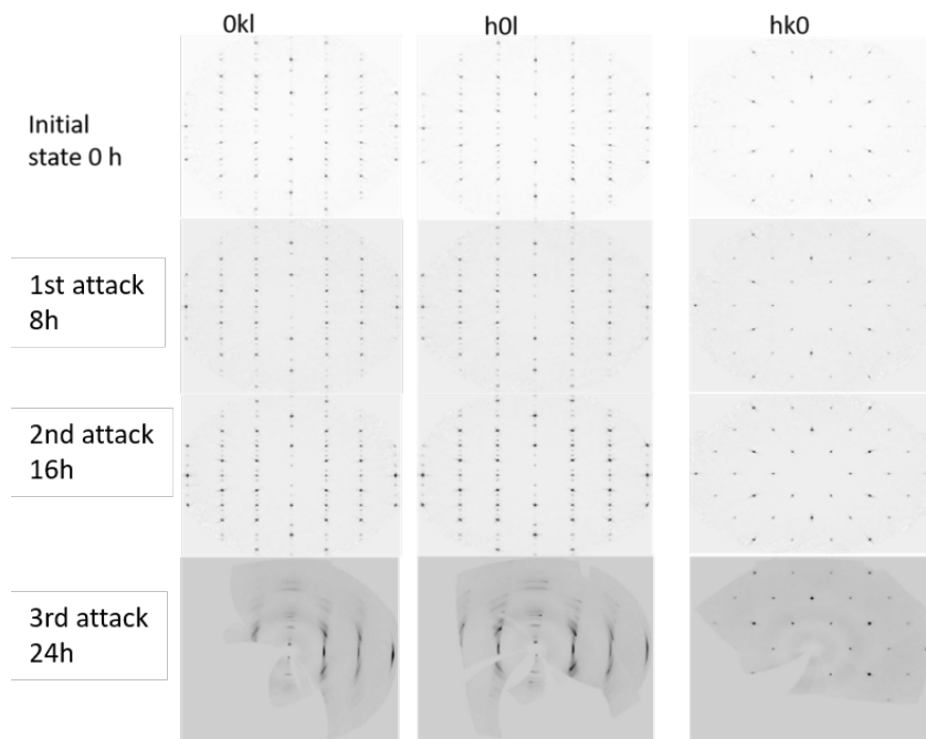
Figure 8. Diagramme XRD de V_2AlC à partir de l'état initial, gravure 8h, gravure 16h et 24h de gravure.
