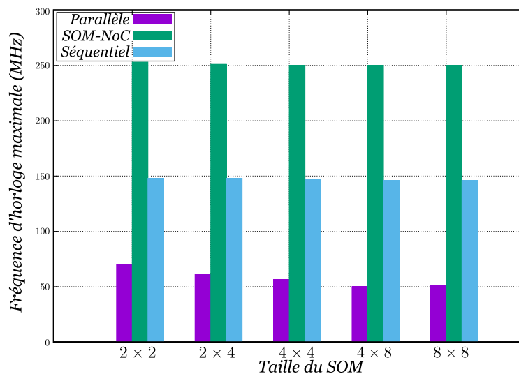
FIGURE 3.22 – Comparaison de la fréquence maximale de l'architecture proposée par rapport aux architectures classiques
