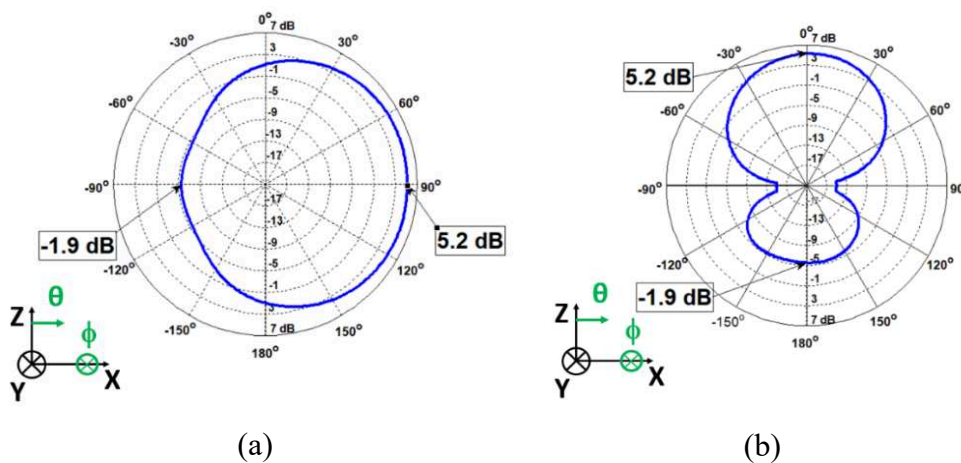
Figure 63: Gain total réalisé à f=2,45 GHz de l'antenne contenant un directeur. (a) Gain réalisé en élévation ( \phi=0^\circ ), (b) gain réalisé en azimut ( \theta=90^\circ )
