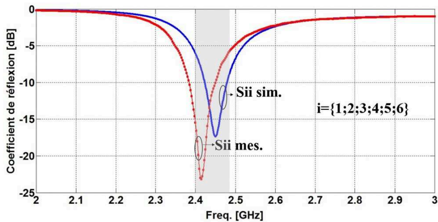
Figure 104: Coefficients de réflexion simulés et mesurés de l'antenne
