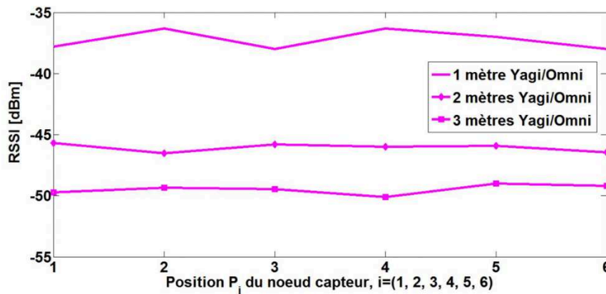
Figure 81: RSSI mesurés en configuration Omni/Omni pour des rayons de 1, 2 et 3m
