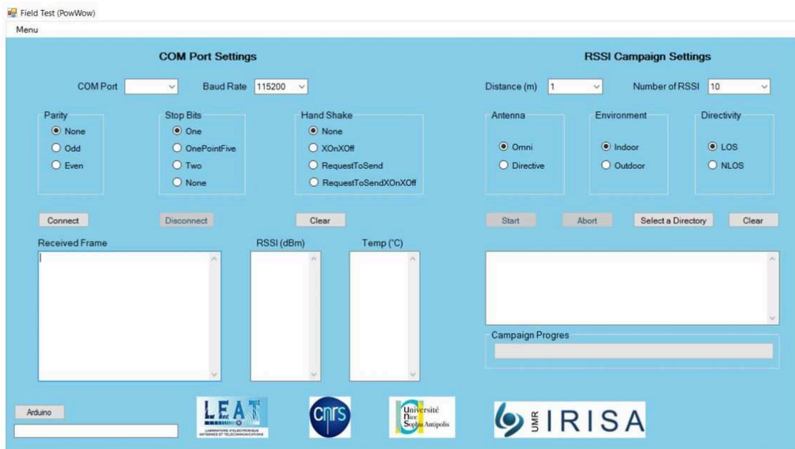
Figure 14: Interface graphique en C#
