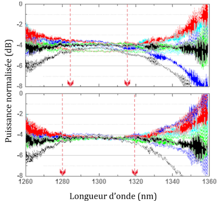
Figure IV-21 : Spectres des transmissions normalisées de chaque sortie du coupleur sur 5 puces différentes. La figure du haut correspond à un coupleur optimisé pour une seule longueur d'onde et celle du bas pour le coupleur robuste en longueur d'onde. Chaque couleur représente une mesure sur une puce différente. [124]
