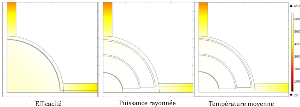
Figure IV-7 : Positions des pistes optimales selon chaque critère avec la cartographie de la température (°C) en fonctionnement.
