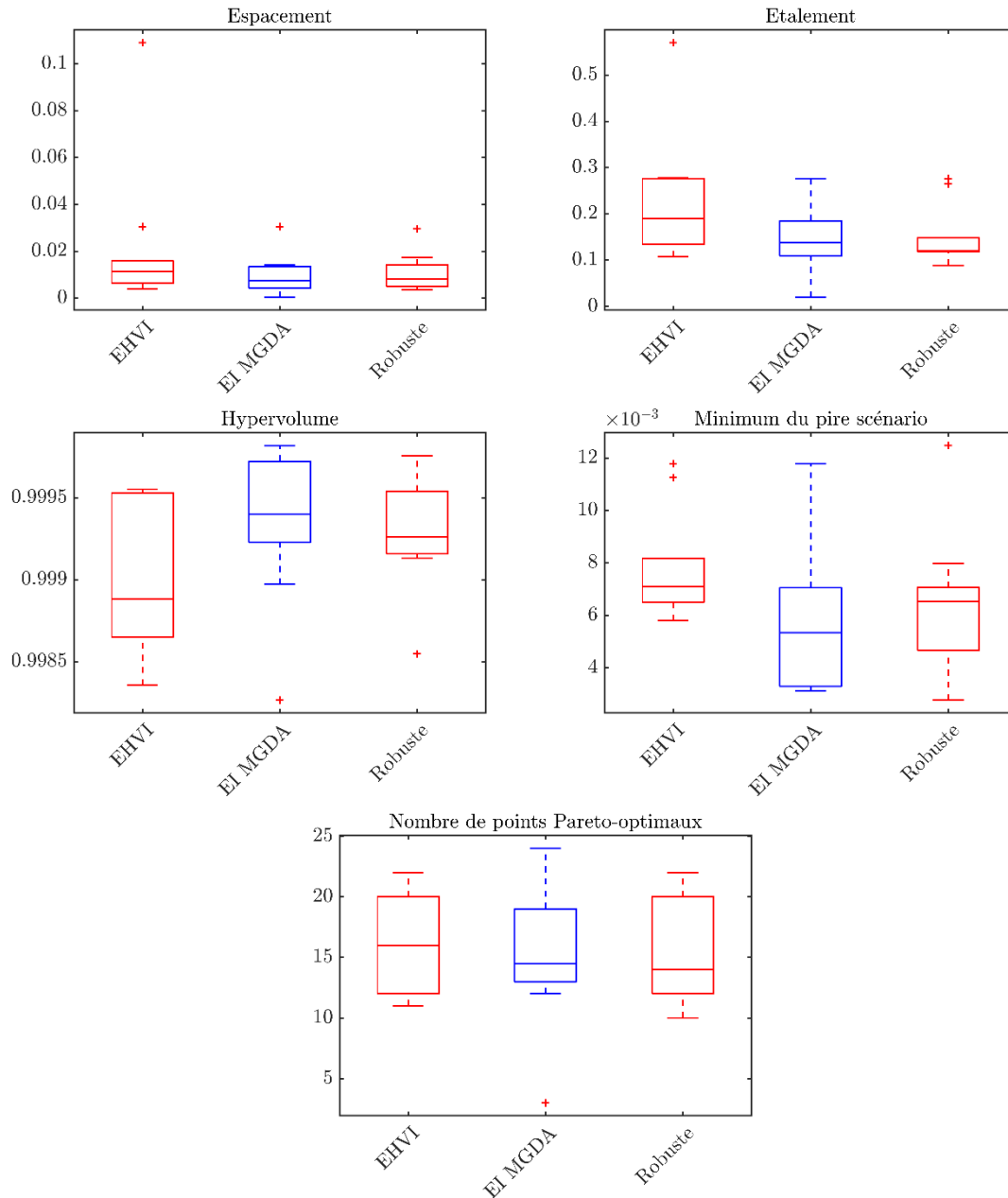
Figure IV-30 : Comparaison des résultats de l'optimisation multi-objectif de l'écart au taux de couplage par critère EHV1, EI MGDA et optimisation robuste classique.
