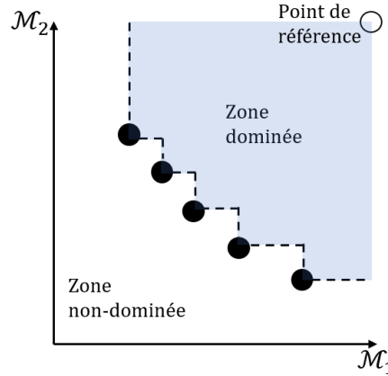
Figure III-14 : Front de Pareto, représentation de l'ensemble Y^{PF} . Le point de référence y_{ref} est défini comme la pire valeur possible des objectifs \mathcal{M}_1 et \mathcal{M}_2 .
