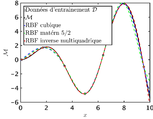
Figure II-22 : RBF avec fonction radiale cubique, matérn 5/2 et inverse multiquadratique. Optimisation des hyperparamètres par leave-one-out sur \mathcal{M}(x) = x \sin(x) avec 7 points d'entraînement.
