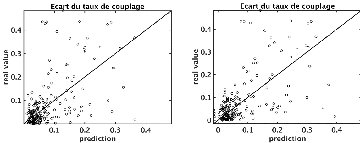
Figure II-39 : Graphique de comparaison entre les valeurs prédites et les valeurs réelles pour le krigeage (à gauche) et pour les RBF (à droite) sur la prédiction de l'écart au taux de couplage.
