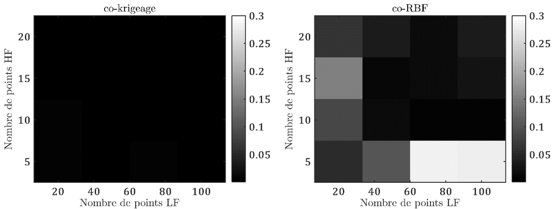
Figure IV-18 : Ecart type de l'erreur de prédiction (RAAE) de la fréquence de résonance sur 5 plans d'expériences différents.
