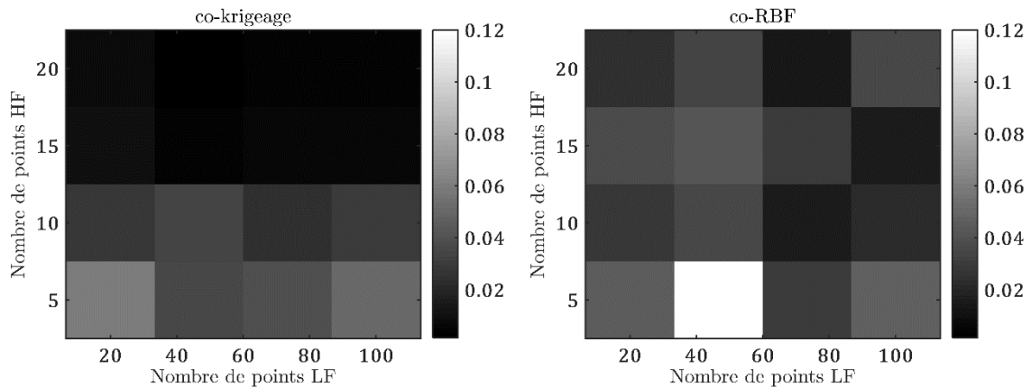
Figure IV-15 : Ecart type de l'erreur de prédiction (RAAE) du signal sur 5 plans d'expérience différents.
