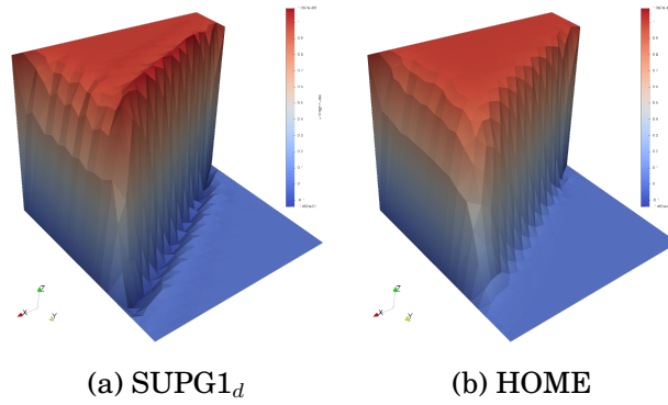
Figure 21 – Intérêt des méthodes de capture de choqe sur un cas-test avec une importante discontinuité. SUPG1 d sans capture de choqe, HOME avec capture de choqe
