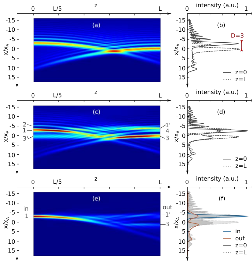
Figure C.13: Guides d'onde photo-induits à l'aide de deux faisceaux d'Airy contrepropageants désalignés dans un cristal photoréfractif ( D = 3 normalisé selon x_A ). (a) (resp. (c)) Distribution d'intensité à l'intérieur du milieu et (b) (resp. (d)) profils d'intensité transverses aux extrémités du cristal dans des conditions linéaires (resp. non linéaires focalisantes). (e)-(f) Propagation linéaire d'un faisceau test dans la structure de guide d'onde (b): (e) distribution d'intensité et (f) profils transverses du faisceau gaussien guidé le long de 1 \rightarrow (1', 3) .
