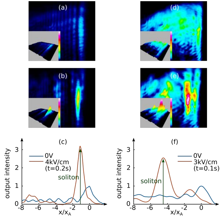
Figure C.5: Soliton expérimental émis d'un faisceau d'Airy auto-focalisant pour un rayon de lobe décroissant [Fig. D.2]: (a)-(c) \chi_A = 14 \mu\text{m} , P_A = 7 \mu\text{W} (d)-(f) \chi_A = 9.5 \mu\text{m} , P_A = 43 \mu\text{W} . Distribution d'intensité du faisceau d'Airy à z = L (a),(d) après propagation linéaire, (b),(e) durant la propagation fortement non linéaire et (c),(f) profils d'intensité transverse des faisceaux de sortie linéaire et solitonique.
