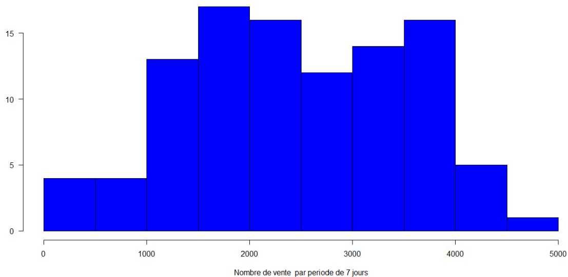
FIGURE 3.5 – NOMBRE DE VENTES PAR PÉRIODE T = 7 JOURS . Cette figure représente le nombre de ventes observées sur la période du 01 Janvier 2010 au 16 mars 2012 pour la Peugeot 207 HDI Berlin par période de 7 jours. Le moyenne est de \mu_{P,207} = 2467 et l'écart-type est \sigma_{P,207} = 1086.72 .
