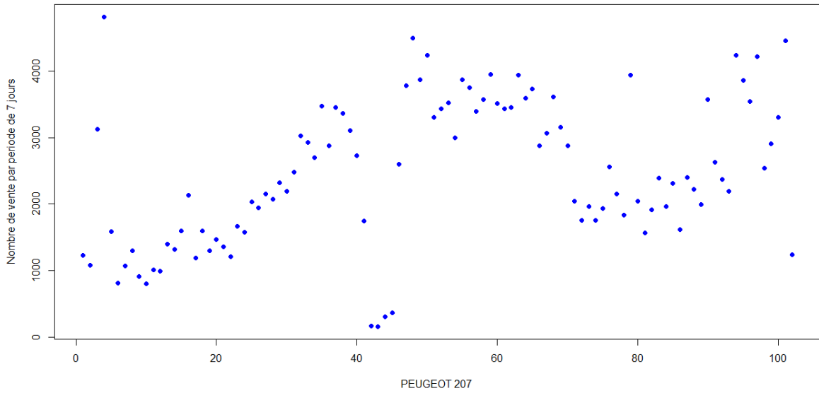
FIGURE 3.1 – NOMBRE DE VO VENDUS PAR PÉRIODE DE 7 JOURS. Cette figure concerne la dispersion des délais de vente associés à la Peugeot 207 HDI Berline pour des annonces observées sur la période de janvier 2010 à février 2011. Nous voyons à travers ces figures qu'il y a des périodes où des observations se démarquent significativement des autres. Nous pouvons supposer que les dates correspondant à ces observations sont pour la plupart des dates de retrait après une longue publication de l'annonce et non des dates de vente. Nous avons supprimé ces observations.
