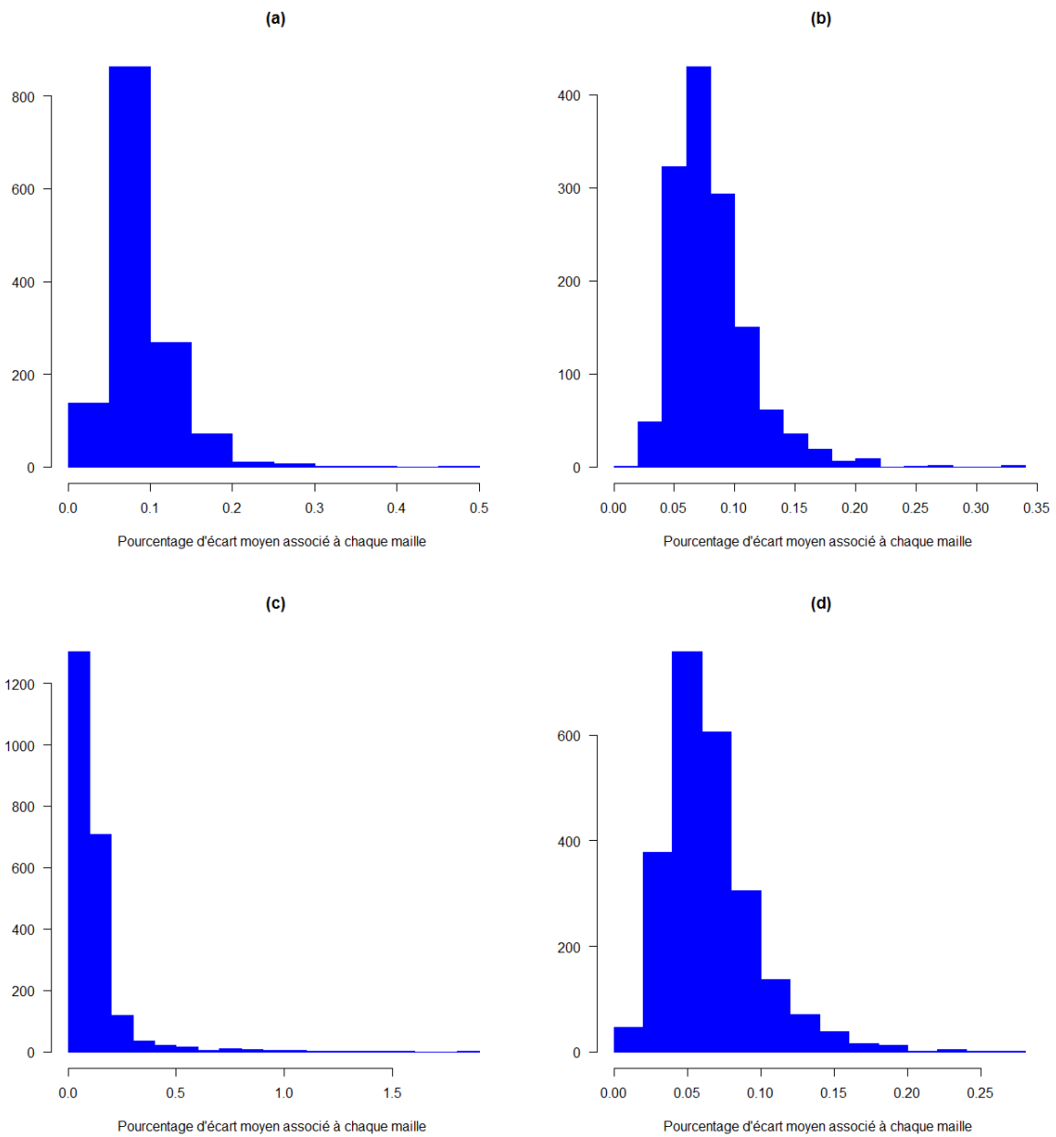
FIGURE 2.11 – APPRÉCIATION DE L'ERREUR RELATIVE À L'ÉCHELLE DE LA MAILLE. Cette figure traduit ce que nous avons présenté en TAB.2.9. (a) correspond au modèle ML, (b) au modèle MLog, (c) au modèle MAdd et (d) au modèle Mqr.
