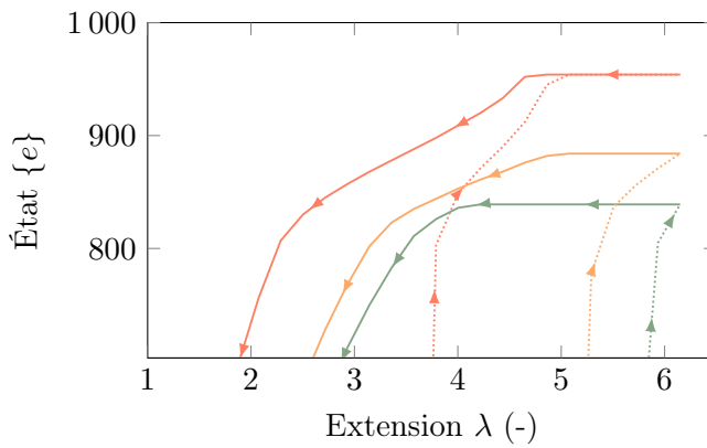
FIGURE VI.9 – États successifs de quelques chaînes représentatives (figure VI.7(b)) pendant la charge (ligne pointillée) et la décharge (ligne pleine) en fonction de l'extension globale appliquée à la sphère du modèle full-network . Paramètres de référence.
