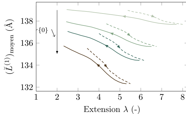
FIGURE VI.30 – Évolution des hauteurs de cristallites moyennes L^{(1)} pour différents degrés de réticulation, qui vont dans l'ordre croissant des courbes du haut (couleur claire) à celles du bas (couleur foncée).
