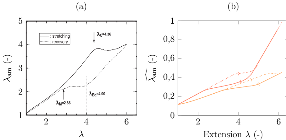
FIGURE VI.16 – (a) \lambda_{am} en fonction de \lambda . D'après [Albouy 12]. (b) \lambda_{am} en fonction de \lambda pour les chaînes polaires et de la couronne.
