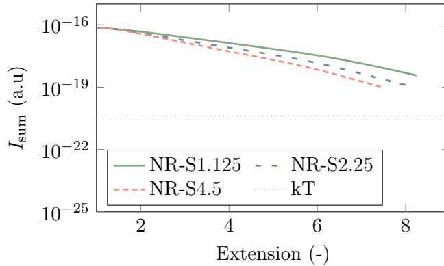
FIGURE IV.10 – Enthalpie libre critique \Delta G^* en fonction de l'extension sur une échelle logarithmique avec les valeurs de la littérature (table IV.9). La ligne horizontale pointillée indique la valeur de kT .
