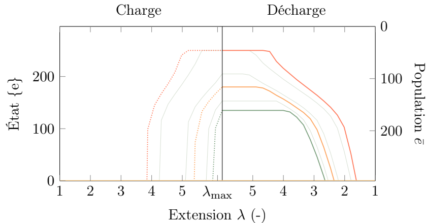
FIGURE VI.8 – États successifs et population \bar{e} subissant la transformation correspondante (resp. axe des ordonnées gauche et droit) de quelques chaînes représentatives (figure VI.7(b)) et quelques autres chaînes intermédiaires) pendant la charge et la décharge en fonction de l'extension globale appliquée à la sphère du modèle full-network . Paramètres de référence.
