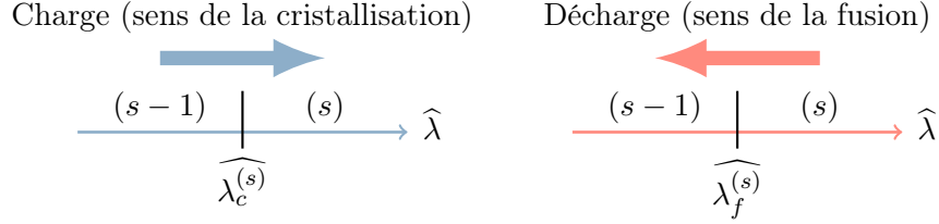
FIGURE V.13 – Transition entre les états à la charge et à la décharge.
