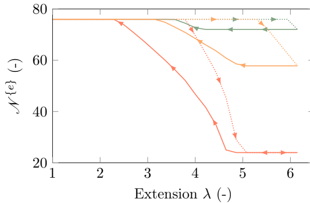
FIGURE VI.14 – Évolution du nombre caractéristique de segments \mathcal{N}^{\{e\}} de la portion amorphe de quelques chaînes représentatives (figure VI.7(b)) pendant la charge (ligne pointillée) et la décharge (ligne pleine) en fonction de l'extension globale appliquée à la sphère du modèle full-network . Paramètres de référence.
