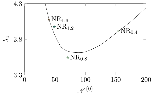
FIGURE VII.4 – Extensions-seuils de cristallisation \lambda_c en fonction de \mathcal{N}^{(0)} . Les valeurs expérimentales données par Candau et al. [Candau 14a, Candau 16] des quatre échantillons étudiés sont reportées.
