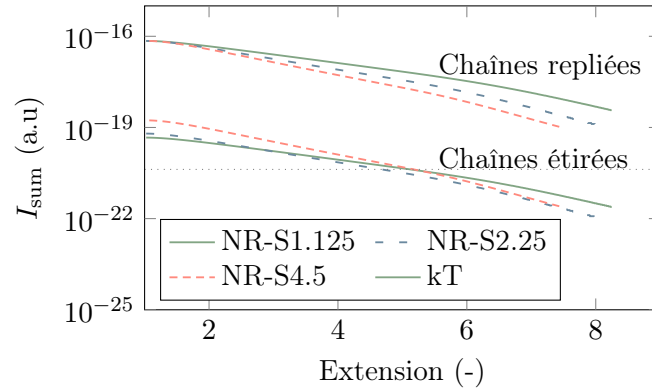
FIGURE IV.13 – \Delta G^* calculées avec les valeurs d'énergies d'interface pour les germes à chaînes repliées (tableau IV.9; tracés identiques à ceux de la figure IV.10) et pour les germes à chaînes étirées (tableau IV.12). La ligne horizontale pointillée indique la valeur de kT .
