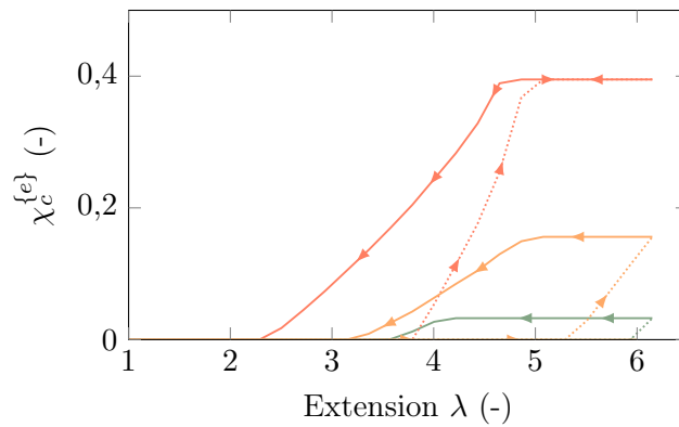
FIGURE VI.11 – Taux de cristallinité de quelques chaînes représentatives (figure VI.7(b)) pendant la charge (ligne pointillée) et la décharge (ligne pleine) en fonction de l'extension globale appliquée à la sphère du modèle full-network . Paramètres de référence.
