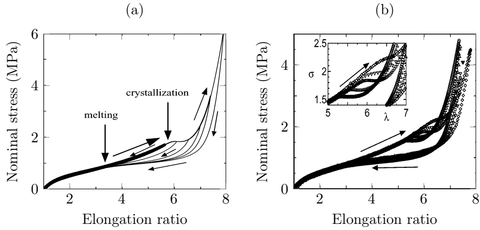
FIGURE I.5 – Influence de l’extensions maximale (a) et de la vitesse de chargement (b) sur la courbe contrainte-déformation pour un cycle de traction uniaxiale. Température : 29 °C; légende : \circ , \triangle , \square , \nabla puis \diamond pour des vitesses variant resp. de 0,0007 à 7 s -1 . D’après [Miyamoto 03].
