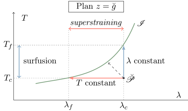
FIGURE IV.20 – Dans le plan z = \check{g} , courbe d'équilibre \mathcal{S} et chemins de fusion y menant depuis le point \mathcal{P} représentant la cristallite stable, par changement de température à \lambda constant (flèche verticale), et par changement d'extension à T constant, induisant les effets de surfusion et de superstraining respectivement. La flèche tiretée est un exemple de chemin quelconque de fusion.
