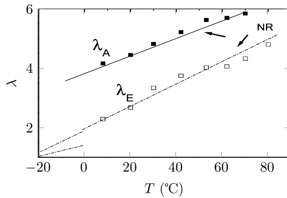
FIGURE I.17 – Extensions-seuils (associées aux courbes de la figure I.15) de cristallisation et de fusion ( \lambda_A et \lambda_E respectivement) pour différentes températures d’essai. \nu = 0,57-0,60 \times 10^{-4} mol/cm 3 . Adaptée d’après [Rault 06b].
