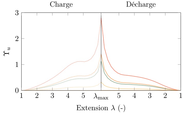
FIGURE VI.17 – Force dans quatre chaînes représentatives (faisant respectivement un angle des 0, 10, 45 et 90 degrés avec la direction de traction) en fonction de l'extension globale appliquée à la sphère du modèle full-network lors de la charge et décharge. Paramètres de référence.
