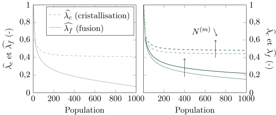
FIGURE VI.22 – (a) Courbe générique de référence. (b) Courbe générique pour des mailles amorphes 1,13 et 1,33 fois plus petites.
