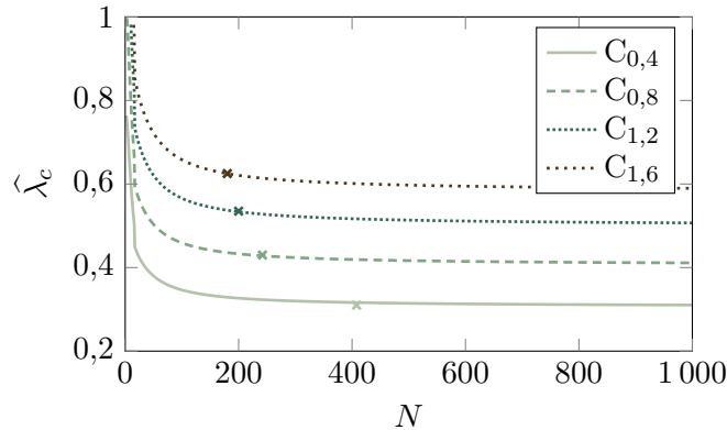
FIGURE VII.2 – Courbes génériques d’extension-seuil normalisée de cristallisation pour les quatre valeurs indiquées sur la figure VII.1 correspondant aux quatre échantillons testés. Les croix indiquent N_{\max} pour chacun d’eux et donc l’extension normalisée à laquelle débute la cristallisation dans le réseau.
