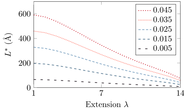
FIGURE IV.7 – Influence de l'extension \lambda et des énergies d'interface \gamma sur les tailles critiques (calculées avec les paramètres N = 200 , T = 20 °C. \gamma varie de 0,005 à 0,035 J/m 3 ).
