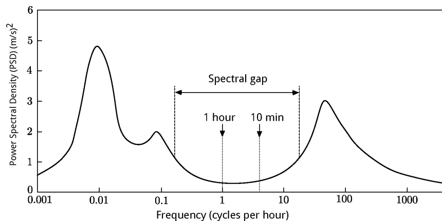
FIGURE 2.4: Van Der Hoven spectrum [13].
