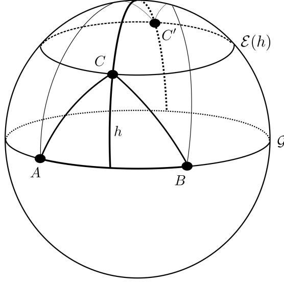
Figure 3: Nous traçons une géodésique \mathcal{G} passant par deux points A et B . Nous traçons une courbe equidistante \mathcal{E}(h) qui est à distance sphérique h de cette géodésique. Les points C et C' sont les lieux où l'aire du triangle ayant pour base AB et un sommet sur \mathcal{E}(h) est minimale et maximale, respectivement. De plus, les sommets de deux triangles appartiennent à la géodésique qui passe par le pôle de \mathcal{G} (et ainsi de \mathcal{E}(h) ) et le milieu de AB .
