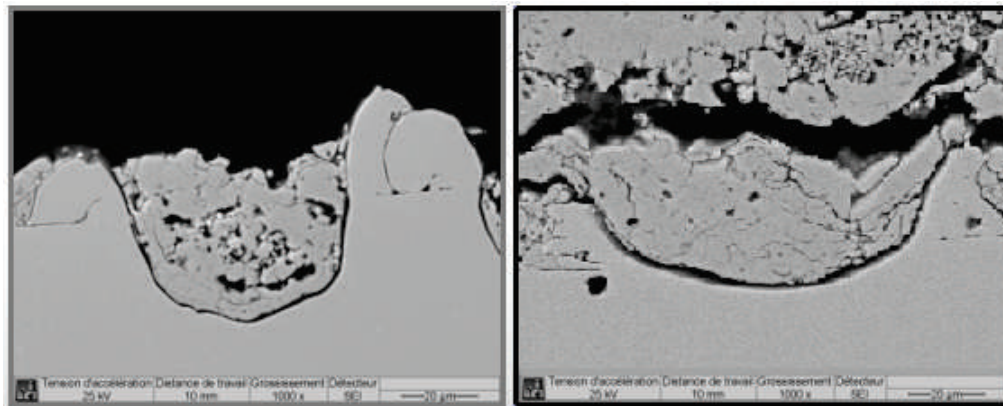
Figure IV.118: Vue en coupe des faciès de rupture pour des motifs S60 et S80 pour le couple YSZ/304L par essai de traction adhésive
