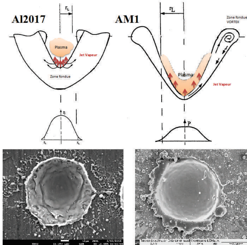
Figure III.94: Vue en surface d'impacts laser réalisés sur l'Al2017 et sur l'AM1 après 10 impacts aux même flux et schémas explicatifs des mécanismes de création d'un motif dans les deux cas
