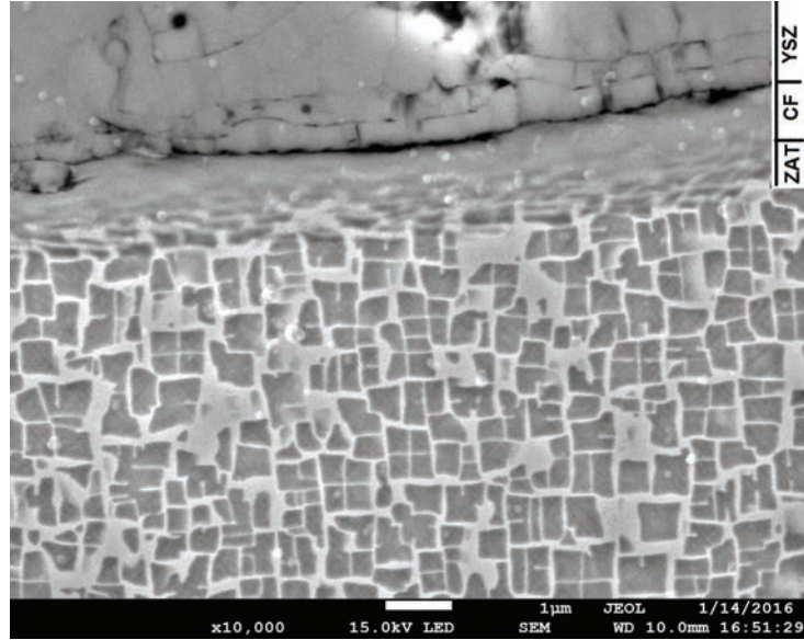
Figure III.86: Microstructure de l'AM1 après texturation laser en fond de trou illustrant la couche fondue (CF) et la zone affectée thermiquement (ZAT)
