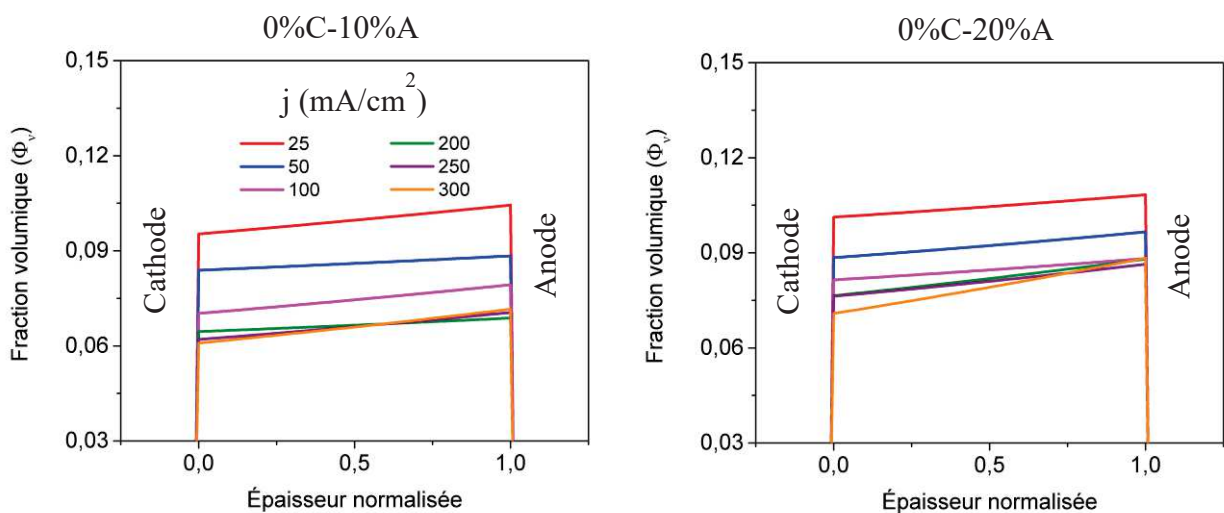
Figure 3-7 : Profils d'eau à travers l'épaisseur de la membrane dans les conditions du groupe III : 0%C-10%A, 0%C-20%A. La position d'enregistrement est dans le canal au centre de la pile.
