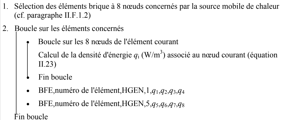
Figure II.24 : Organigramme de la programmation de la source mobile de chaleur dans le modèle éléments finis
