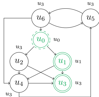
(d) 2 nd iteration: detection & update
