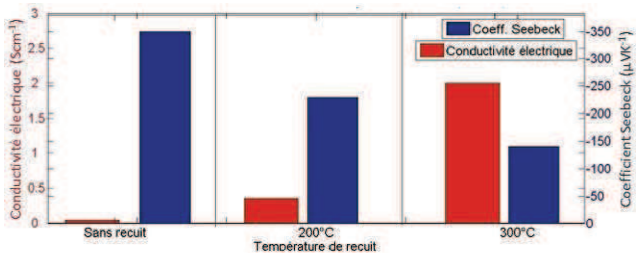
Figure A. 2. 3. Conductivité électrique et Coefficient Seebeck du (\text{GO})_x\text{V}_2\text{O}_5 en fonction de la température de recuit : sans recuit, 200° C, 300° C. Concentration massique de 5%.
