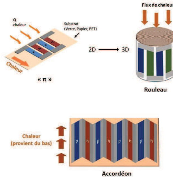
Figure III. 28. Architectures « \pi » et « accordéon ». Le passage 2D-3D est possible avec matériaux et substrats flexibles.
