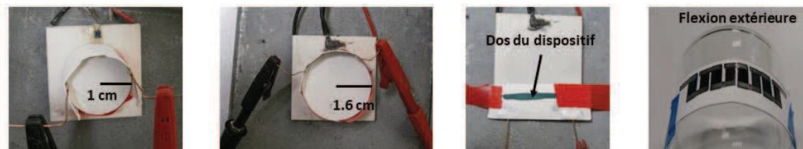
Figure III. 63. Flexions intérieures et extérieures des dispositifs thermoélectriques imprimés sur papier.
