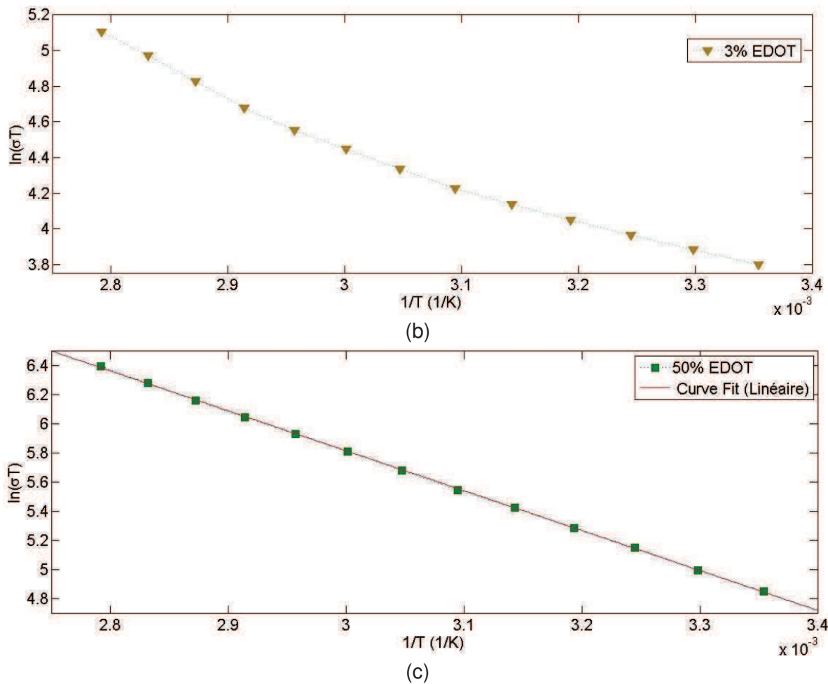
Figure II. 37. Dépendance \ln(\sigma T) de 1/T selon le modèle SPH des échantillons de V_2O_5 contenant (a) 0% d'EDOT ( V_2O_5 pur), (b) 3% (c) 50% d'EDOT.
