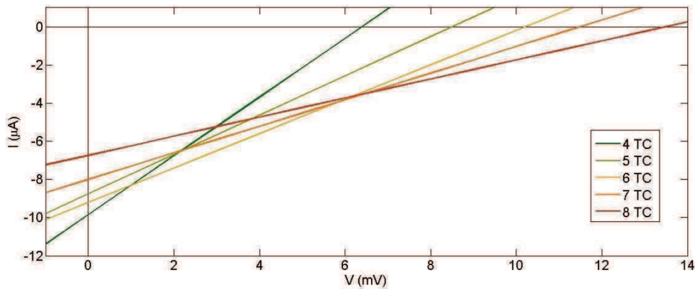
Figure III. 58. Profil I(V) des générateurs à base de PEDOT:PSS et TiS_2(HA)_x asymétriques.
