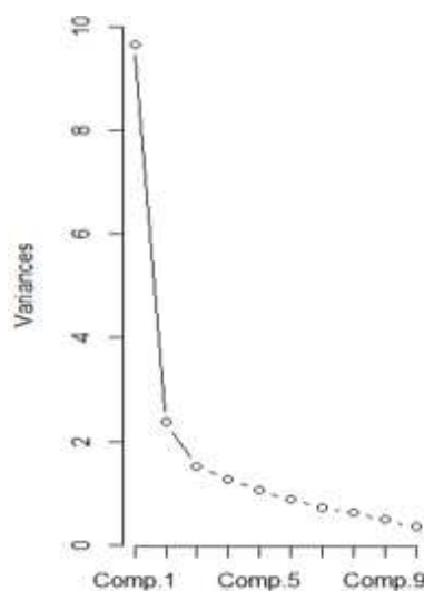
Figure 11 : Variance expliquée de l'ACP
