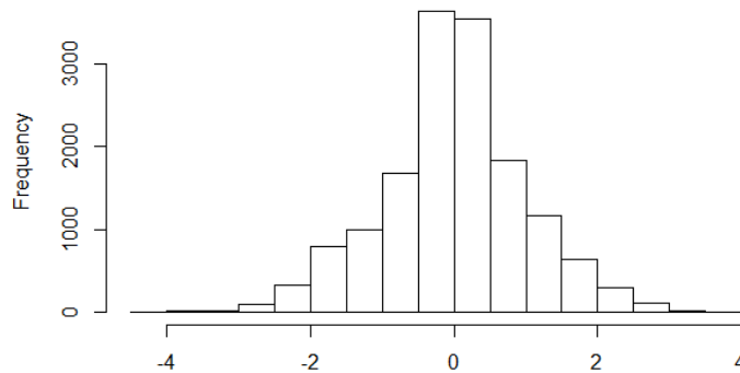
Figure 52 : Graphique des résidus du modèle d'estimation de la distance parcourue en voiture conducteur
