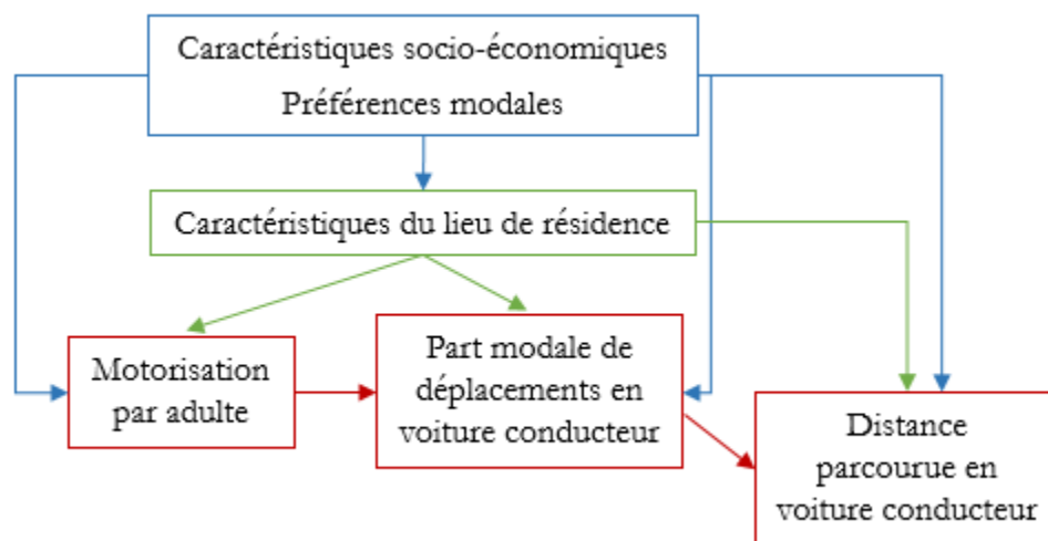
Figure 60 : Schéma théorique du modèle d'équations structurelles – comportements de mobilité
