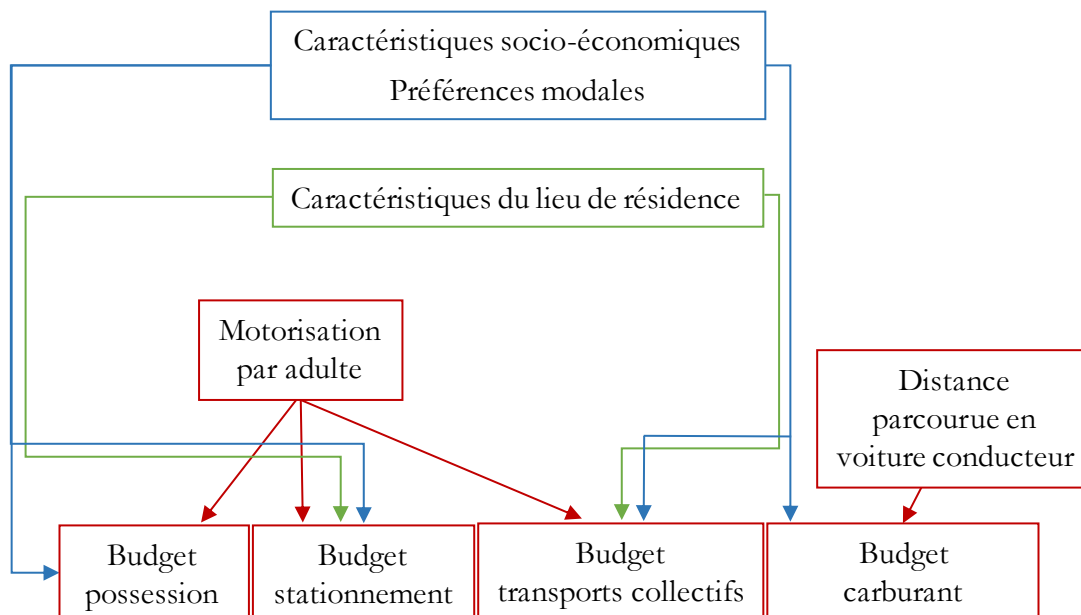
Figure 57 : Construction du modèle théorique générale – étape n°3 – sous-catégories du budget mobilité
