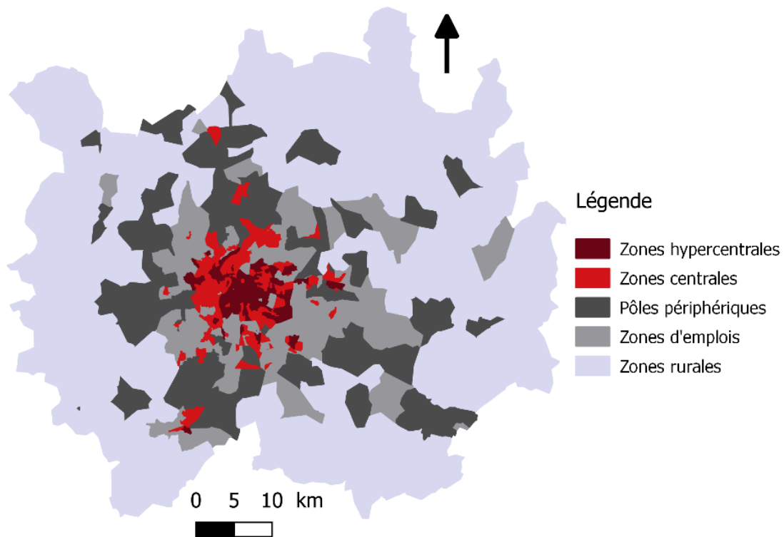
Figure 12 : Clustering de l'aire urbaine lyonnaise
