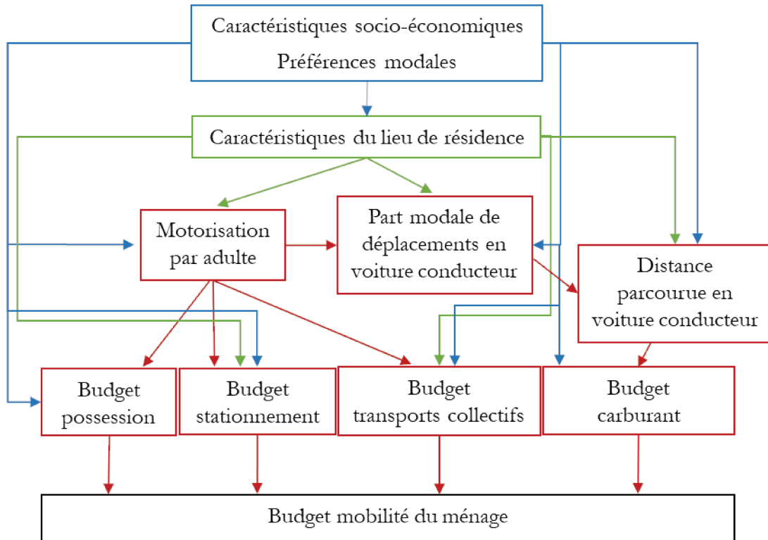
Figure 58 : Schéma théorique du modèle d'équations structurelles
