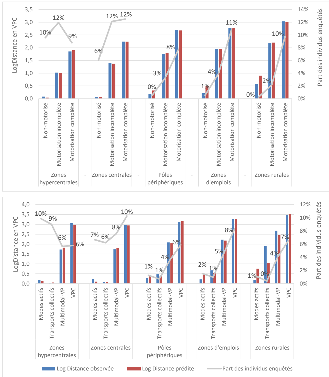
Figure 53 : Comparaison des logDistances parcourues en voiture conducteur observées et prédites par le modèle n°4 en fonction de la localisation, du mode principal et de l'accès à l'automobile
