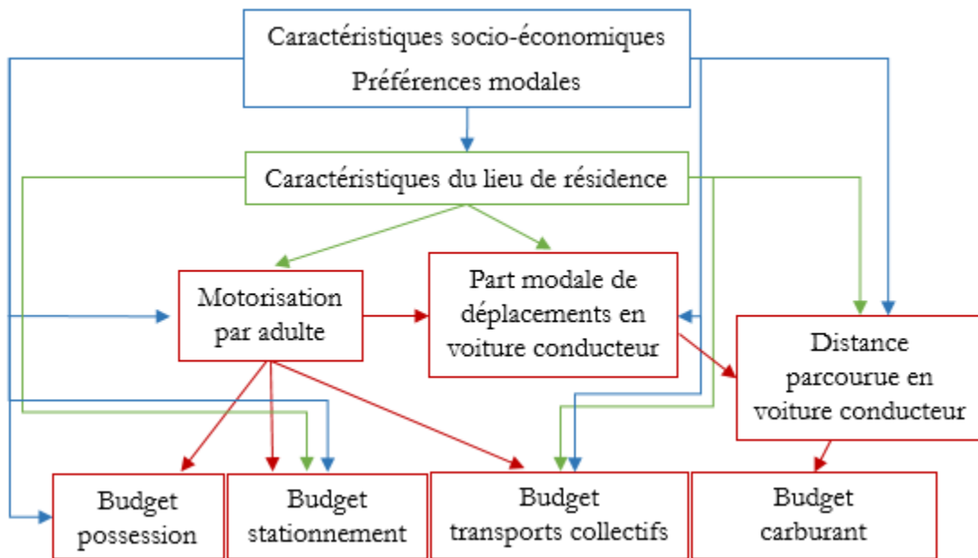
Figure 61 : Schéma théorique du modèle d'équations structurelles – budget mobilité
