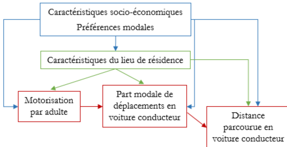
Figure 62 : Schéma théorique du modèle d'équations structurelles – comportements de mobilité
