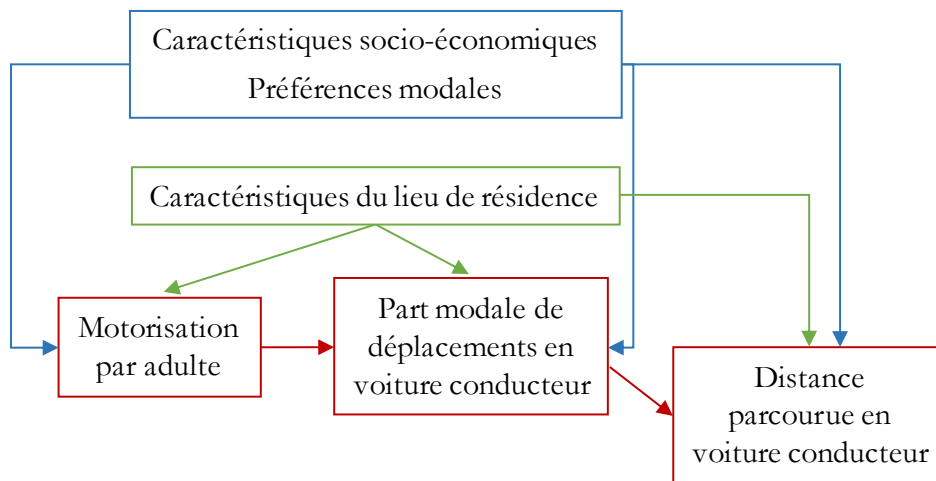
Figure 56 : Construction du modèle théorique générale – étape n°2 – comportements de mobilité
