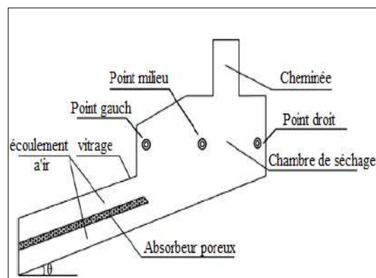
Figure I. 1 : Diagramme schématique du séchoir solaire avec absorbeur poreux [19].
