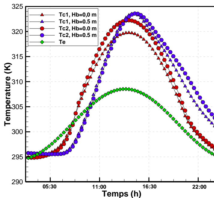
Figure V. 3 : Évolution de la température T_{c1} et T_{c2} avec et sans lit thermique.
