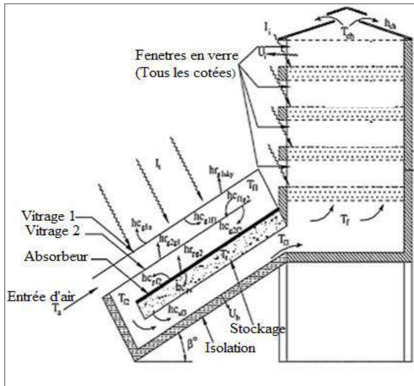
Figure I. 6 : Séchoir multi-claies avec capteur à air incliné multi-passes avec un stockage thermique intégré.
