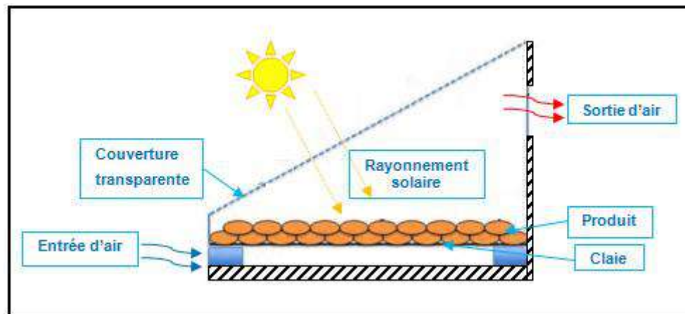
Figure II. 9 : Le principe d'un séchoir solaire direct.
