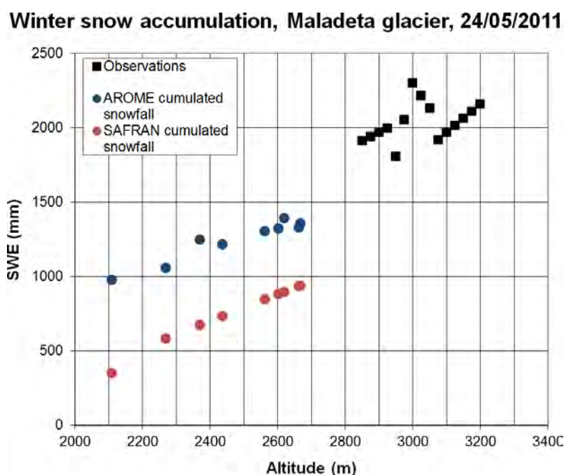
FIGURE 3.17 – Mesures de l'accumulation neigeuse hivernale au 24 mai 2011 en 15 points du glacier de Maladeta (carrés noirs), comparées aux chutes de neige cumulées du 1 octobre 2010 au 24 mai 2011 aux 9 points de grille les plus proches par AROME (ronds bleus) et SAFRAN (ronds rouges).
