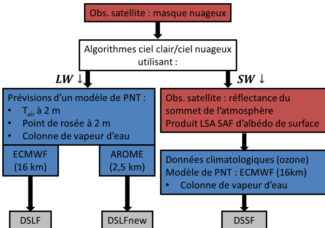
FIGURE 4.1 – Représentation schématisée des observations (en rouge), prévisions et données climatologiques (en bleu) utilisées par les algorithmes calculant DSSF, DSLF et DSLFnew. Les valeurs entre parenthèse indiquent la résolution horizontale des systèmes de PNT.
