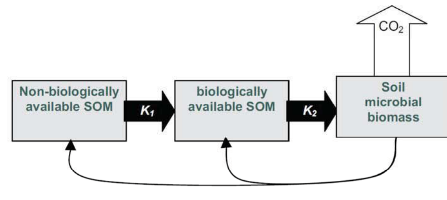
Figure II.18. | Représentation schématique de la 'Regulatory gate hypothesis'. K_1 = transformations abiotiques de la SOM non bio-disponible. K_2 = minéralisation biologique de la SOM bio-disponible. Les flèches indiquent que la biomasse microbienne peut créer de la MO bio-disponible et non bio-disponible mais n'est pas capable d'influencer directement les taux du processus K (Kemmitt et al. , 2008).
