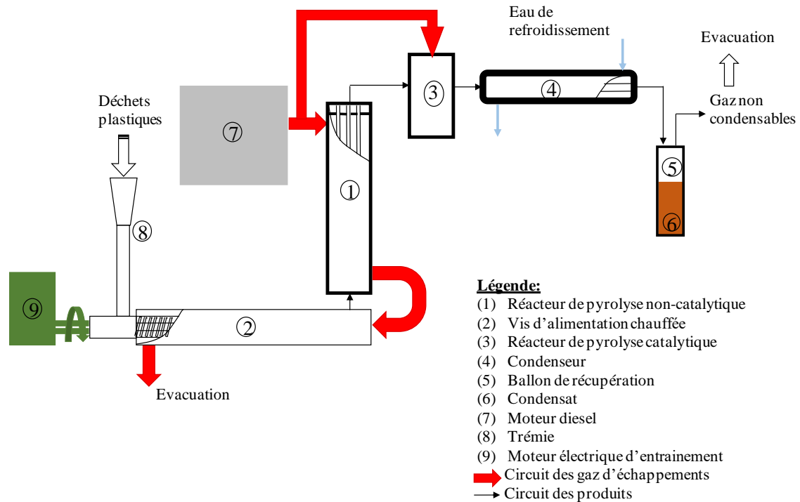
Figure 4. 12 : Schéma de l'installation en continu avec le catalyseur placé en aval du réacteur de pyrolyse non-catalytique
