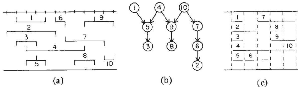
FIGURE 2.28 – (a) exemple de canal de routage, (b) graphe de contraintes verticales, (c) représentation en zone
