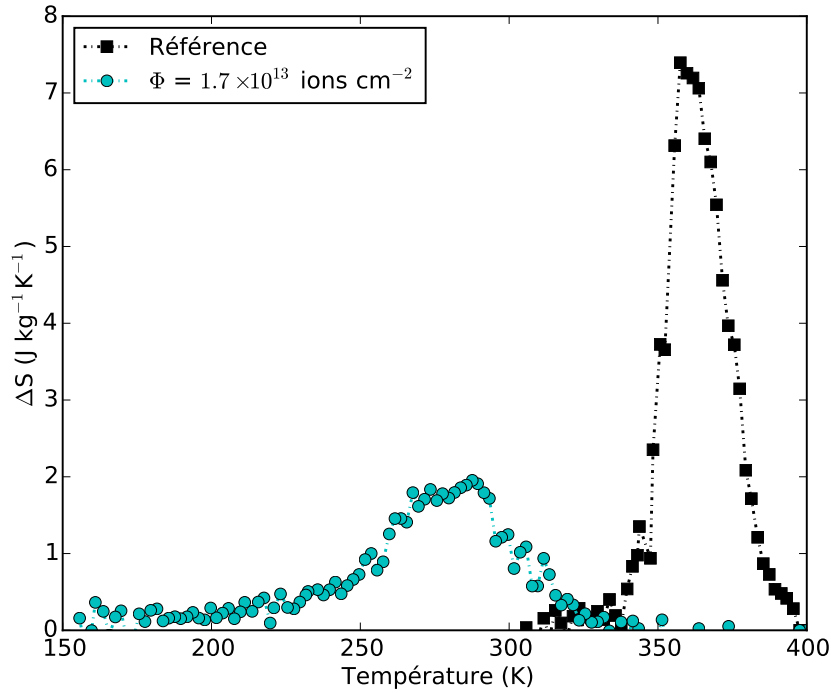
FIGURE 4.9 – Variation d'entropie magnétique de l'échantillon de référence (en noir) et d'un échantillon irradié avec une fluence de 1.7 \times 10^{13} ions cm -2 de Ne 5+ (en cyan) en fonction de la température. \Delta S a été calculée à partir des courbes de l'aimantation en fonction de la température lorsque la température de l'échantillon augmente pour des champs magnétiques variant de 0 à 2 T.
