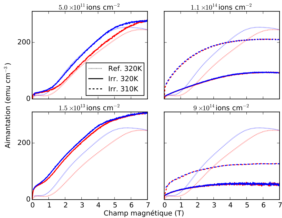
FIGURE 3.23 – Évolutions de l'aimantation en fonction du champ magnétique mesurées sur les échantillons ayant été irradiés avec des ions néon et différentes fluences ( 5.0 \times 10^{11} \text{ ions cm}^{-2} \rightarrow 9 \times 10^{14} \text{ ions cm}^{-2} ). Les courbes en trait plein et en pointillés correspondent respectivement aux mesures de M = f(H) faites à 320 K sur les échantillons irradiés et sur l'échantillon de référence. Les courbes en ligne tiretée ont été obtenues à 310 K. Les couleurs bleu et rouge sont associées respectivement à la diminution et à l'augmentation du champ magnétique appliqué.
