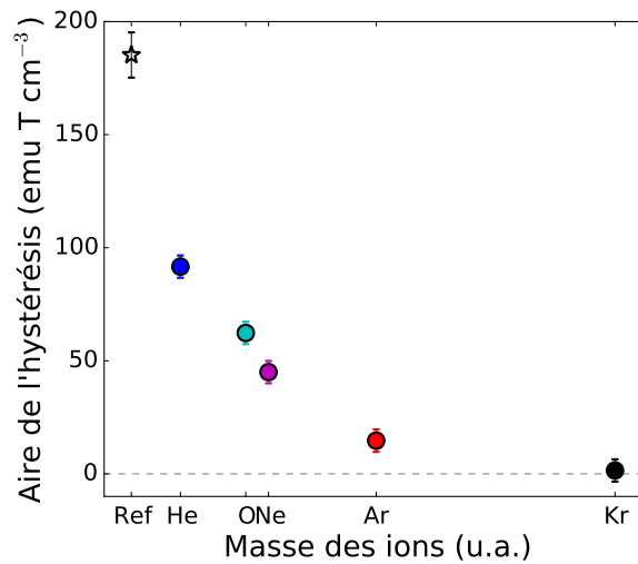
FIGURE 3.16 – Aires des hystérésis thermiques des échantillons irradiés avec une même fluence de l'ordre de 10^{13} ions \text{cm}^{-2} sont tracées en fonction de la masse des ions incidents. Les aires sont calculées à partir des courbes présentées sur la figure 3.15. Les barres d'erreur, explicitées au chapitre 2, sont représentées mais peuvent être de l'ordre de la taille des points.
