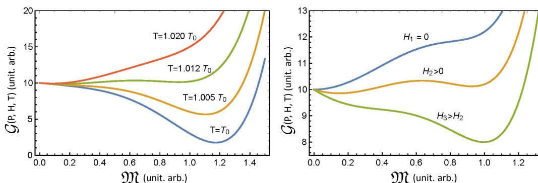
FIGURE 1.4 – Évolution de l'énergie de Gibbs en fonction du moment magnétique pour différentes températures du système à gauche et différents champs magnétiques appliqués, à droite. Dans ces calculs arbitraires les coefficients de Landau a et c sont positifs et b est négatif.
