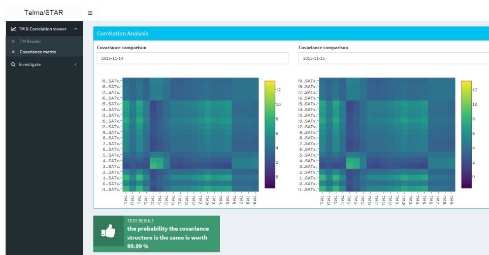
FIGURE 1.27 – Application STAR pour l’analyse des télémessures - onglet pour visualiser et comparer la matrice de covariance de deux jours de télémessures.
