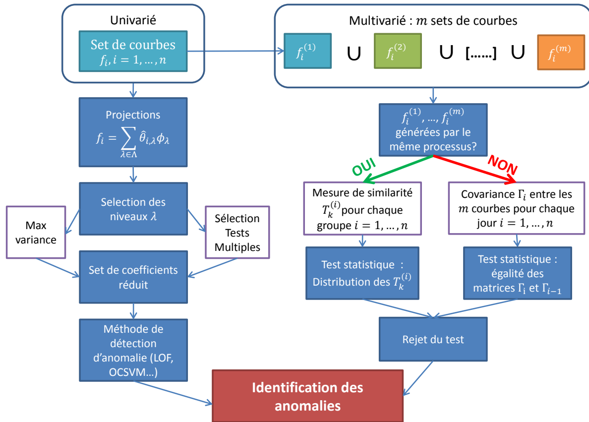
FIGURE 1.17 – Schéma de notre procédure pour détecter des anomalies dans des données fonctionnelles univariées ou multivariées.
