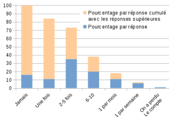
FIGURE 1.5 – Nombre d'attaques par Dénis de Service Distribuées subies sur 12 mois, entre 2016 et 2017. (Source : Neustar)
