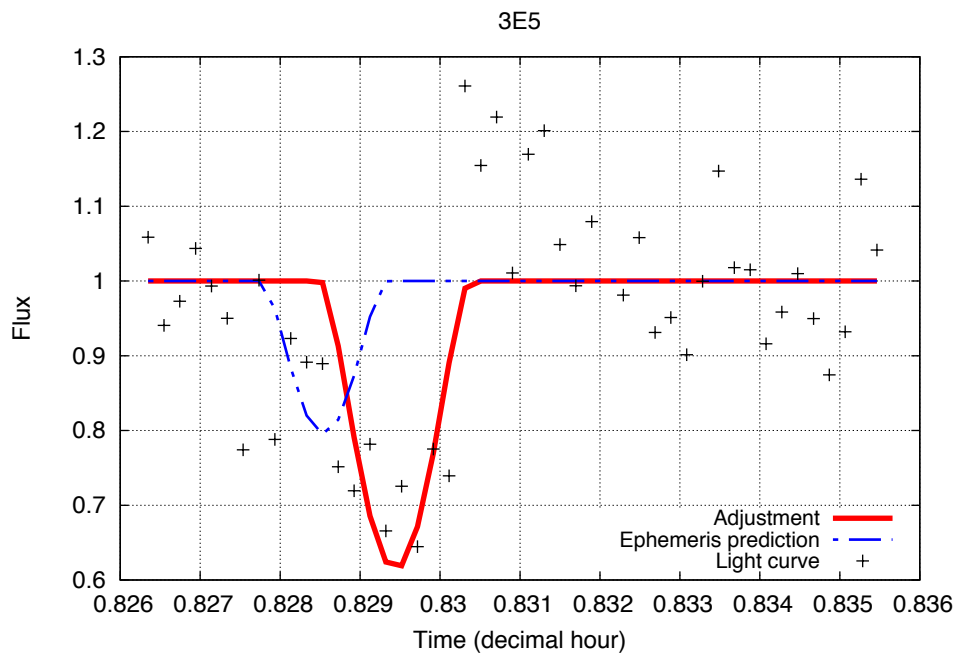
Figure 6.9 – Ajustement de la courbe de lumière de phénomène mutuel 3E5. Ganymède éclipse Amalthée le 07/01/2015. Les pointillés bleus montrent la chute en flux théorique d’après les éphémérides JUP310 [Jacobson, 2013], la ligne rouge montre l’ajustement de la chute en flux du phénomène.
