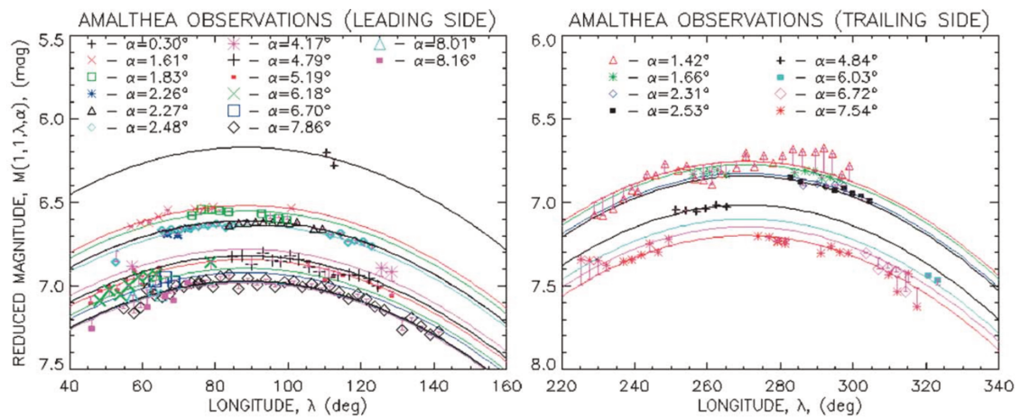
Figure 4.13 – Courbes photométriques d’Amalthee en fonction de l’angle de phase obtenues pour le filtre méthane (CH 4 ) par Kulyk [2008] : la figure située à gauche présente la courbe pour la face avant ( leading side ), la figure à droite présente la courbe pour la face arrière ( trailing side ).
