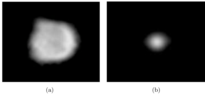
Figure 1.10 – Images de Métis (a) et Adrastée (b) prises par la sonde Galileo . Crédit : NASA.
