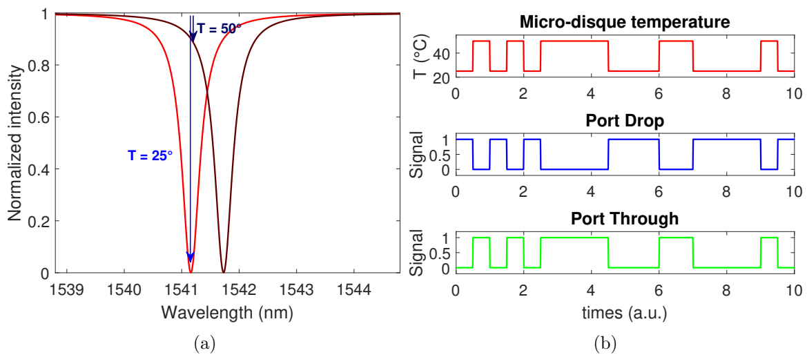
FIGURE 1.24 – (a) Influence d'une augmentation de température de 25°C sur les résonances dans un disque de SiC de 5 \mu\text{m} de rayon. En rouge clair une résonance à 25°C. En rouge foncée la même résonance à 50°C. Les flèches bleues indiquent la possibilité de réaliser un switch thermo-optique avec une telle configuration. Une émission laser continue à 1541.1 nm est transmise à la température de 50°C et pas à celle de 25°C. (b) Principe d'un commutateur thermo-optique. La courbe rouge représente la température du micro-disque. La courbe bleue correspond au signal dans le port Drop et la courbe verte dans le port Through. Le signal est considéré comme binaire : 1 ou 0.
