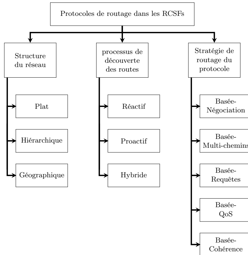
FIGURE 2.1 – Classification des protocoles de routage dans les RCSFs.
