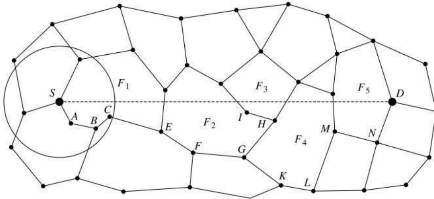
FIGURE 2.4 – Routage en mode périmètre (ou par face) d'un paquet depuis le nœud S vers le nœud D (le chemin emprunté est SABCEFGHIGKLMND ), en utilisant la règle de la main gauche [8].
