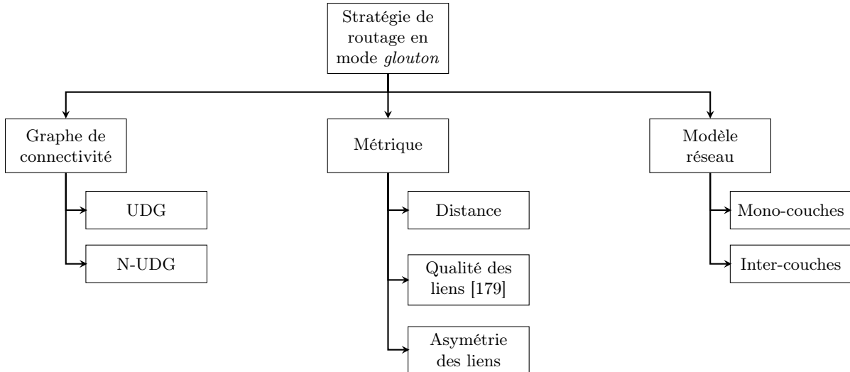
FIGURE 3.1 – Classification des stratégies de routage en mode glouton .
