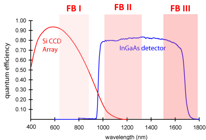
Figure 1.11 : Rendement quantique des détecteurs Si et InGaAs. Superposition des différentes fenêtres de transparences des tissus. Adapté de Smith et al. 41 .
