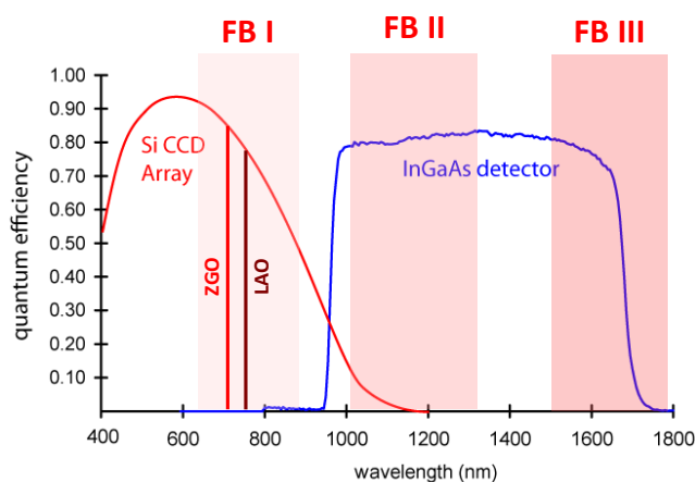
Figure 4.34 : Efficacité des détecteurs CCD et InGaAs en fonction de la longueur d'onde et des différentes fenêtres biologiques. Adapté de Smith et al. 21 .
