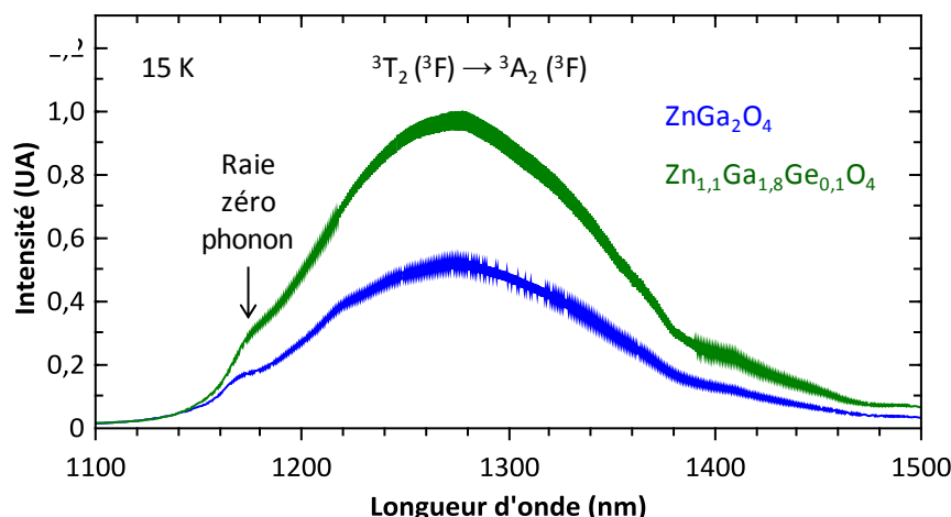
Figure 5.9 : Spectres de photoluminescence ( \lambda_{ex} = 365 \text{ nm} ) à 15 K de nanoparticules de \text{ZnGa}_2\text{O}_4:\text{Ni}^{2+}_{(0,75\%)} calcinées 2 h à 800^\circ\text{C} et de \text{Zn}_{1,1}\text{Ga}_{1,8}\text{Ge}_{0,1}\text{O}_4:\text{Ni}^{2+}_{(0,75\%)} calcinées 2 h à 800^\circ\text{C} .
