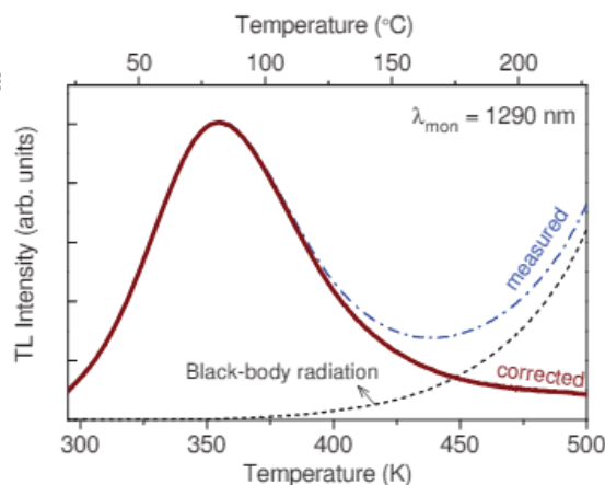
Figure 5.2 : Courbe de thermoluminescence enregistrée après 20 min d'excitation à 300 nm de 295 à 500 K (pointillé bleu). La courbe en pointillé noir correspond à l'irradiation du corps noir. La courbe rouge est la soustraction de la courbe mesurée à celle du corps noir. Adapté de Liu et al. 1 .
