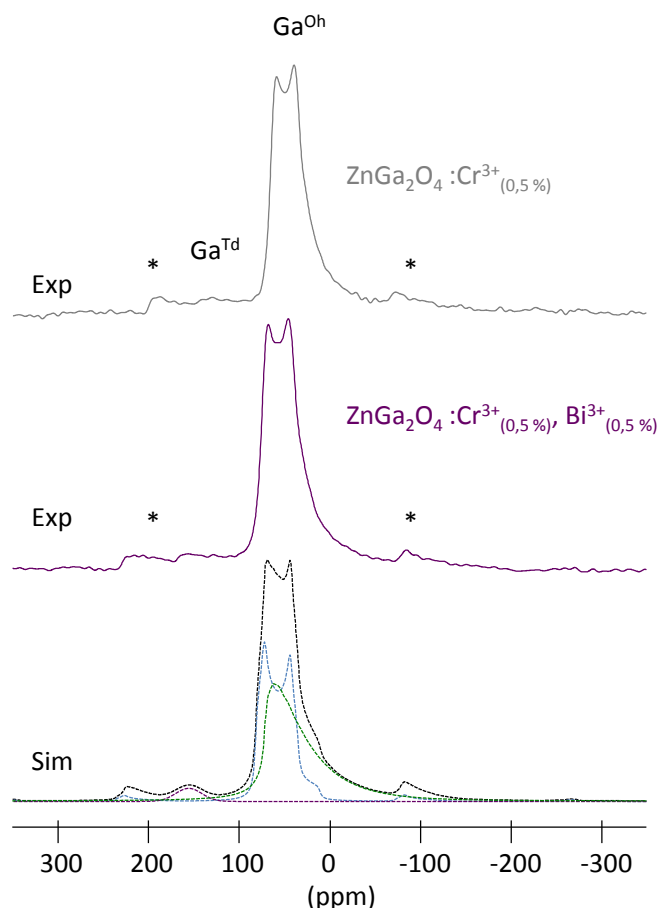
Figure 4.17 : Spectres expérimentaux et simulés de RMN ^{71}\text{Ga} MAS ( 16,5 T , fréquence de rotation = 33 kHz , trait plein) de nanoparticules de \text{ZnGa}_2\text{O}_4:\text{Cr}^{3+}_{(0,5\%)}\text{@SiO}_2 calcinées 1000^\circ\text{C} 2 h et de \text{ZnGa}_2\text{O}_4:\text{Cr}^{3+}_{(0,5\%)}, \text{Bi}^{3+}_{(0,5\%)}\text{@SiO}_2 calcinées 1000^\circ\text{C} 2 h. Les bandes de rotation sont indiquées par un astérisque et les contributions individuelles sont représentées en traits pointillés.
