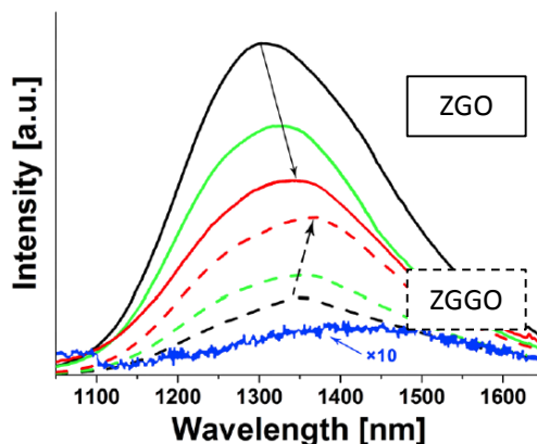
Figure 5.8 : Spectres de photoluminescence de nanocristaux de \text{Zn}_{1+x}\text{Ga}_{2-2x}\text{Ge}_x\text{O}_4:\text{Ni}^{2+} dans une matrice vitrocéramique. Adapté de Gao et al. 9 .
