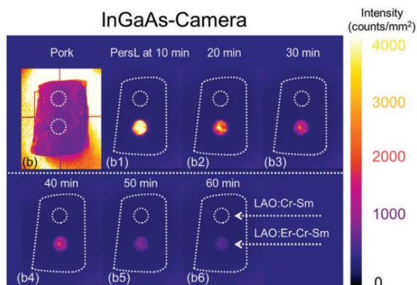
Figure 5.47 : Imagerie in vitro à travers un tissu de porc (épaisseur de 0,5 cm) après 10 min d'excitation à 254 nm (lampe UV 6 W), suivi de l'émission pendant 1 h. Adapté de Xu et al. 26 .
