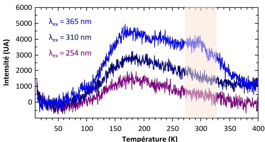
Figure 5.15 : Courbes de thermoluminescence de nanoparticules \text{ZnGa}_2\text{O}_4:\text{Ni}^{2+}_{(0,75\%)} calcinées 2 h à 800°C pour 3 longueurs d'onde d'excitation différentes ( \lambda_{\text{ex}} = 365, 310 et 254 nm).
