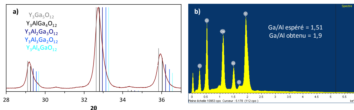
Figure 5.32 : Étude de la stœchiométrie par a) Diffractogramme de RX ; b) MEB-EDX.
