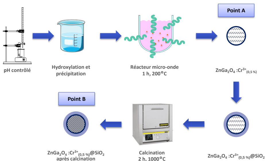
Figure 3.1 : Résumé de la voie de synthèse de nanoparticules de \text{ZnGa}_2\text{O}_4:\text{Cr}^{3+}_{(0,5\%)} retenue pour l'étude.
