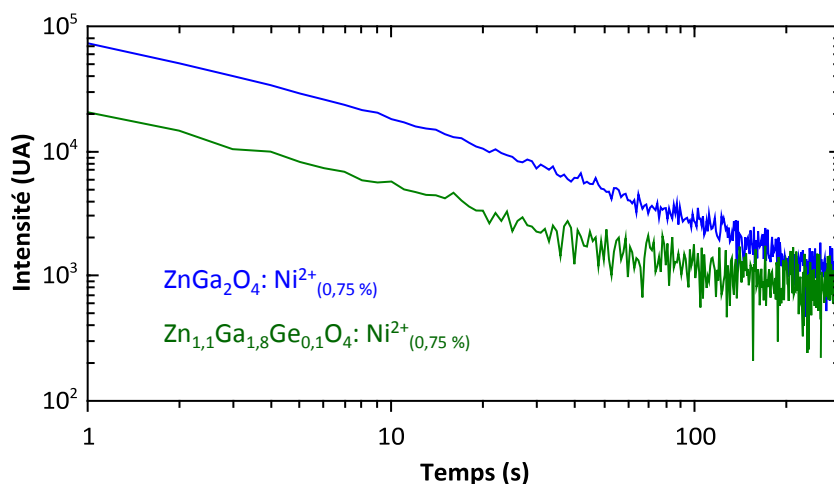
Figure 5.13 : Déclin de la luminescence persistante de nanoparticules de \text{ZnGa}_2\text{O}_4:\text{Ni}^{2+}_{(0,75\%)} calcinées 2 h à 800^\circ\text{C} et de \text{Zn}_{1,1}\text{Ga}_{1,8}\text{Ge}_{0,1}\text{O}_4:\text{Ni}^{2+}_{(0,75\%)} calcinées 2 h à 800^\circ\text{C} enregistré 5 s après 2 min d'excitation UV ( \lambda_{\text{ex}} = 365 \text{ nm} ).
