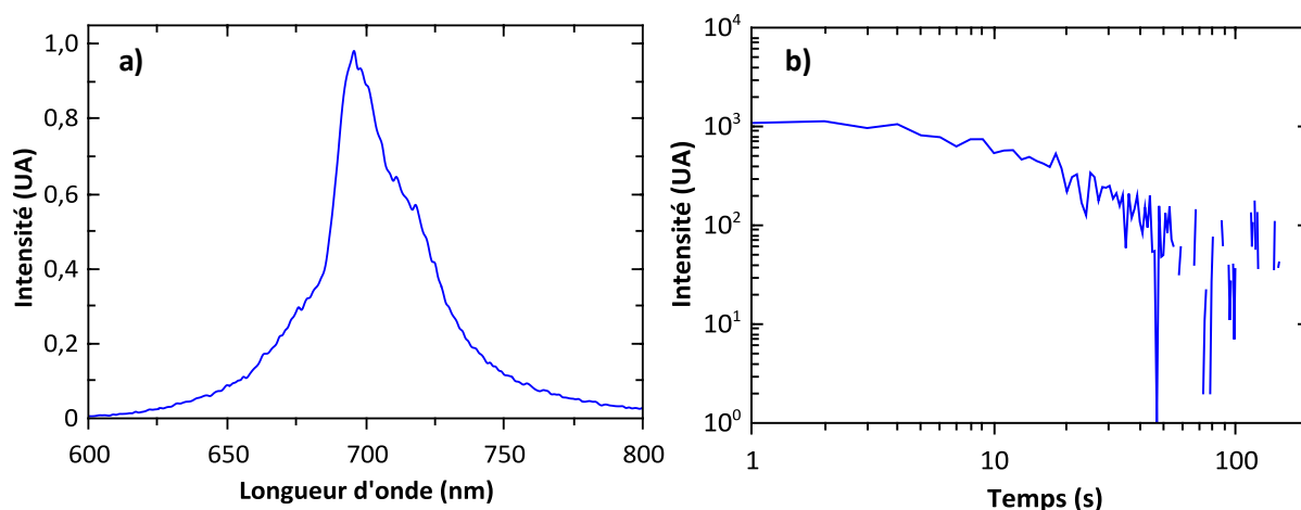
Figure 2.12 : a) Spectre de photoluminescence de nanoparticules de \text{ZnGa}_2\text{O}_4:\text{Cr}^{3+}_{(0.5\%)} ( \lambda_{\text{ex}} = 254 \text{ nm} ) ; b) Déclin de luminescence persistante de nanoparticules de \text{ZnGa}_2\text{O}_4:\text{Cr}^{3+}_{(0.5\%)} enregistré 5 s après 2 min d'irradiation UV ( \lambda_{\text{ex}} = 254 \text{ nm} ).
