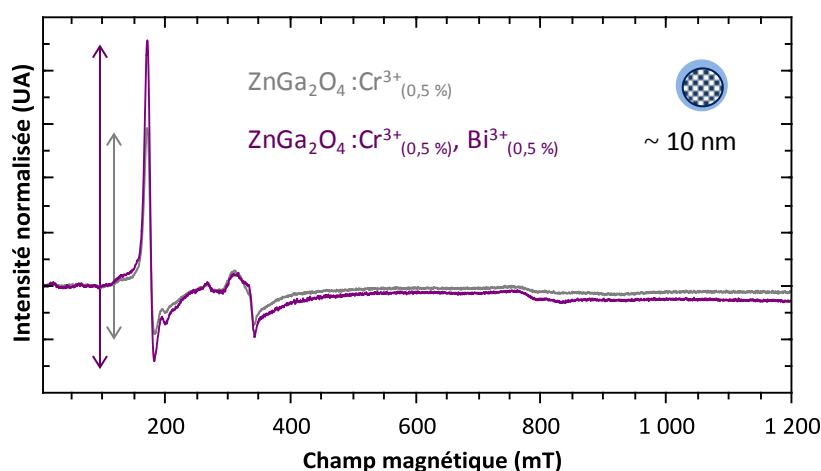
Figure 4.15 : Spectres RPE (bande X) normalisés de nanoparticules de \text{ZnGa}_2\text{O}_4:\text{Cr}^{3+}_{(0,5\%)}@ \text{SiO}_2 calcinées 1000^\circ\text{C} 2 h et de \text{ZnGa}_2\text{O}_4:\text{Cr}^{3+}_{(0,5\%)}, \text{Bi}^{3+}_{(0,5\%)}@ \text{SiO}_2 calcinées 1000^\circ\text{C} 2 h.
