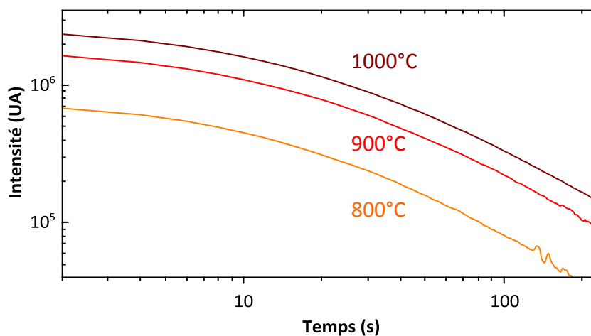
Figure 2.19 : Déclin de la luminescence persistante de nanoparticules de \text{ZnGa}_2\text{O}_4:\text{Cr}^{3+}_{(0.5\%)}@\text{SiO}_2 enregistré 5 s après 2 min d'excitation UV ( \lambda_{\text{ex}} = 254 \text{ nm} ) en fonction de la température de calcination.
