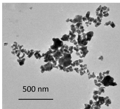
Figure VIII.3 : Image MET des nanoparticules de \text{LaAlO}_3:\text{Cr}^{3+}\text{-Sm}^{3+} obtenues par coprécipitation et traitement thermique à 1000°C pendant 2 h.
