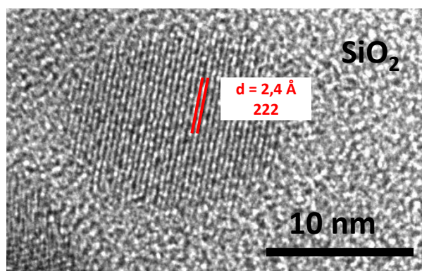
Figure 4.14 : Image HRTEM de nanoparticule de \text{ZnGa}_2\text{O}_4 : \text{Cr}^{3+}_{(0,5\%)}@ \text{SiO}_2 calcinées 1000^\circ\text{C} 2 h.
