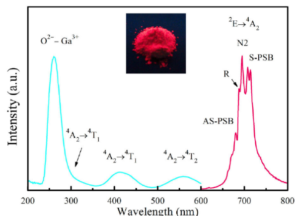
Figure 2.3 : Spectre d'excitation (trait bleu) et spectre d'émission (trait rouge) de nanoparticules de ZnGa_2O_4:Cr^{3+} obtenues par voie hydrothermale, recouvertes de silice et calcinées à 900°C 4h. Adapté de Zou et al. 20 .
