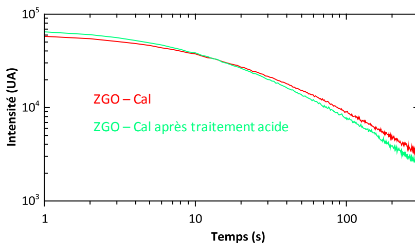
Figure VI.2 : Déclin de la luminescence persistante enregistré 5 s après 2 min d'excitation UV ( \lambda_{\text{ex}} = 254 \text{ nm} ) de nanoparticules ZGO – Cal (en rouge) et ZGO – Cal après traitement avec \text{NH}_5\text{F}_2 0,1 \text{ mol.L}^{-1} pour dissoudre la couche de \text{SiO}_2 (en vert).
