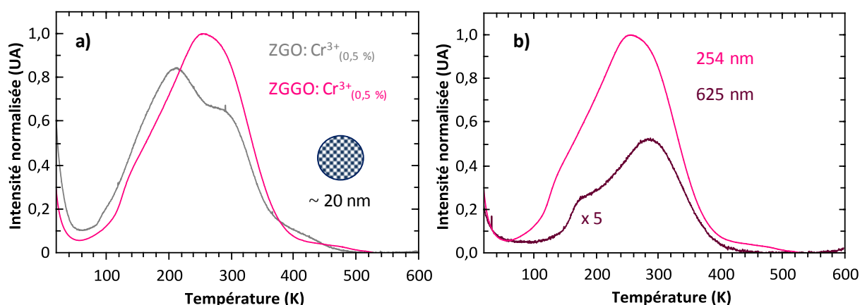
Figure 4.25 : Courbes de thermoluminescence de 10 à 600 K ( 10 \text{ K.min}^{-1} ) après 5 min d'excitation à 10 K. a) Comparaison de la composition chimique de nanoparticules de \text{ZnGa}_2\text{O}_4:\text{Cr}^{3+}_{(0,5\%)} calcinées à 800^\circ\text{C} 2 h et de \text{Zn}_{1,1}\text{Ga}_{1,8}\text{Ge}_{0,1}\text{O}_4:\text{Cr}^{3+}_{(0,5\%)} calcinées à 800^\circ\text{C} 2 h, excitation UV ( \lambda_{\text{ex}} = 254 \text{ nm} ) ; b) Comparaison de la longueur d'onde d'excitation pour les nanoparticules de \text{Zn}_{1,1}\text{Ga}_{1,8}\text{Ge}_{0,1}\text{O}_4:\text{Cr}^{3+}_{(0,5\%)} calcinées à 800^\circ\text{C} 2 h, excitation UV ( \lambda_{\text{ex}} = 254 \text{ nm} ) et rouge ( \lambda_{\text{ex}} = 625 \text{ nm} ).
