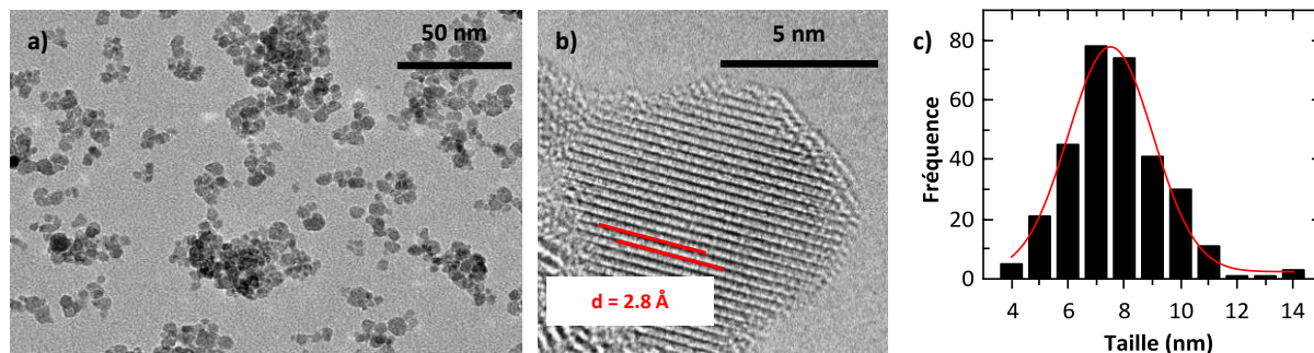
Figure 2.10 : Nanoparticules de \text{ZnGa}_2\text{O}_4:\text{Cr}^{3+}_{(0,5\%)} a) Image MET ; b) Image HRTEM ; c) Distribution en taille.
