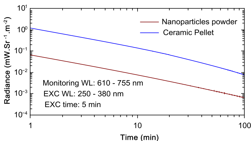
Figure VIII.7 : Déclin de luminescence persistante de nanoparticules de \text{LaAlO}_3:\text{Cr}^{3+}\text{-Sm}^{3+} obtenue par coprécipitation et traitement thermique à 1000°C pendant 2 h et de céramique de \text{LaAlO}_3:\text{Cr}^{3+}\text{-Sm}^{3+} obtenue par voie solide
