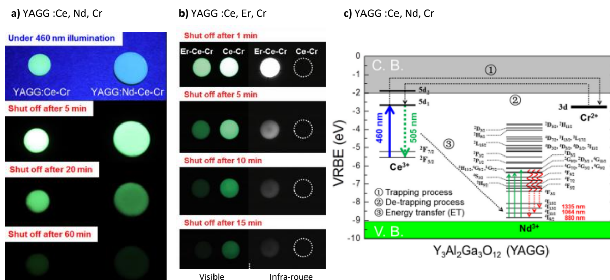
Figure 5.34 : a) Imagerie optique de céramique de \text{Y}_3\text{Al}_2\text{Ga}_3\text{O}_{12} codopée \text{Ce}^{3+} , \text{Nd}^{3+} et \text{Cr}^{3+} sous excitation ( \lambda_{\text{ex}} = 460 \text{ nm} ) puis après avoir coupé la source d'excitation ; b) Céramique de \text{Y}_3\text{Al}_2\text{Ga}_3\text{O}_{12} codopée \text{Ce}^{3+} , \text{Er}^{3+} et \text{Cr}^{3+} après avoir coupé 5 min d'excitation ( \lambda_{\text{ex}} = 455 \text{ nm} ) ; c) Proposition de mécanisme de luminescence persistante. Adapté de Xu et al. 11,12 .
