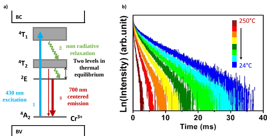
Figure 1 : a) Représentation schématique des niveaux d'énergie de l'ion \text{Cr}^{3+} ; b) Déclin de fluorescence de nanoparticules de \text{ZnGa}_2\text{O}_4:\text{Cr}^{3+}@\text{SiO}_2 calcinée à 1000°C en fonction de la température. D'après les travaux d'Estelle Glais.
