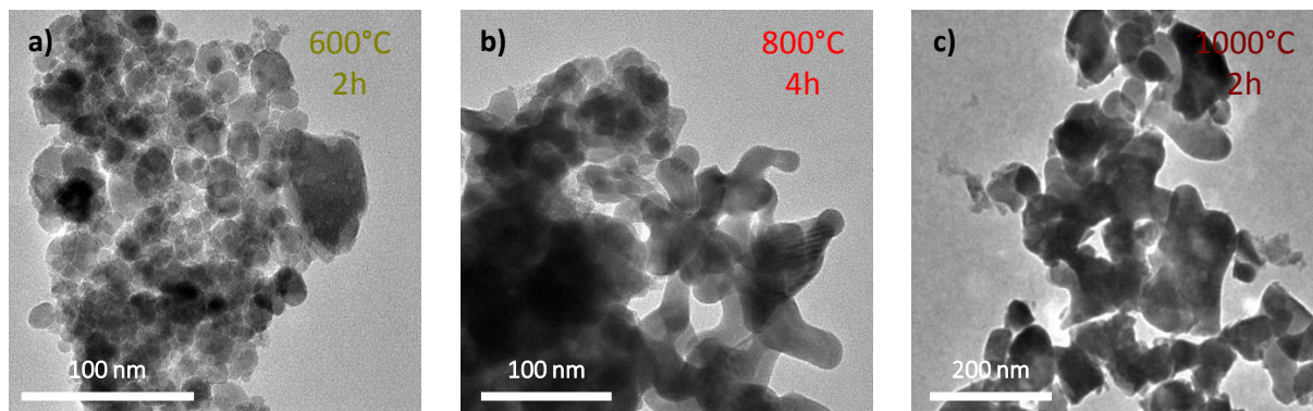
Figure 5.25 : Images MET de Y_3Al_2Ga_3O_{12}:Cr^{3+} en fonction des conditions de calcination : a) 600°C 2h ; b) 800°C 4h ; c) 1000°C 2h.
