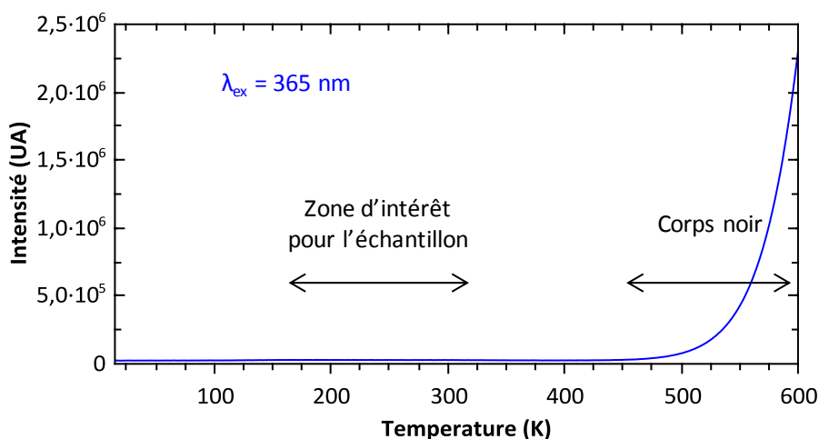
Figure 5.14 : Courbe de thermoluminescence de nanoparticules \text{ZnGa}_2\text{O}_4 : \text{Ni}^{2+}_{(0,75\%)} calcinées 2 h à 800^\circ\text{C} après 2 min d'excitation ( \lambda_{\text{ex}} = 365 \text{ nm} ) à 10 K.
