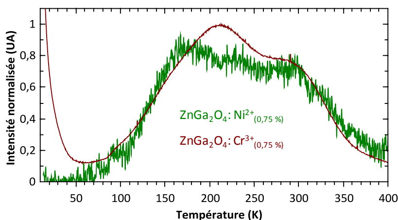
Figure 5.17 : Courbes de thermoluminescence normalisée de nanoparticules de \text{ZnGa}_2\text{O}_4 : \text{Ni}^{2+}_{(0,75\%)} calcinées 2 h à 800^\circ\text{C} après 2 min d'excitation à 10 K ( \lambda_{\text{ex}} = 365 \text{ nm} ) et de \text{ZnGa}_2\text{O}_4 : \text{Cr}^{3+}_{(0,5\%)} calcinées 2 h à 800^\circ\text{C} après 2 min d'excitation à 10 K ( \lambda_{\text{ex}} = 254 \text{ nm} ).
