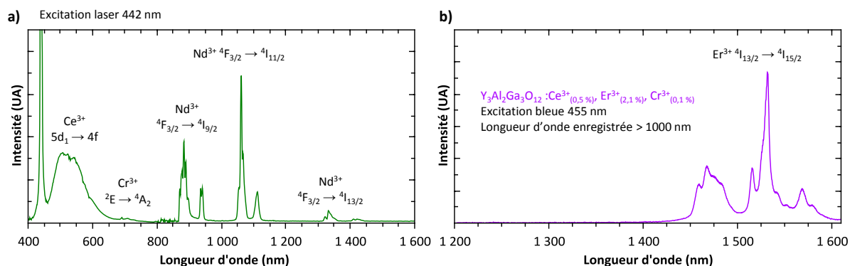
Figure 5.36 : Spectres de photoluminescence de nanoparticules de a) \text{Y}_3\text{Al}_2\text{Ga}_3\text{O}_{12} : \text{Ce}^{3+}_{(0,5\%)}, \text{Nd}^{3+}_{(1\%)}, \text{Cr}^{3+}_{(0,1\%)} sous excitation laser ( \lambda_{\text{ex}} = 442 \text{ nm} ) ; b) \text{Y}_3\text{Al}_2\text{Ga}_3\text{O}_{12} : \text{Ce}^{3+}_{(0,5\%)}, \text{Er}^{3+}_{(2,1\%)}, \text{Cr}^{3+}_{(0,1\%)} sous excitation LED ( \lambda_{\text{ex}} = 455 \text{ nm} ).
