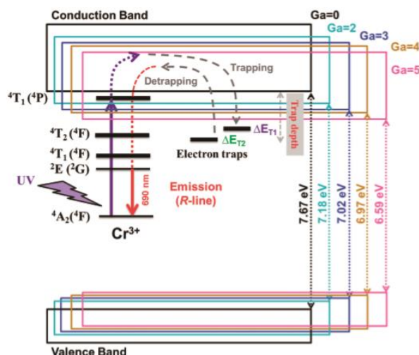
Figure 5.18 : Schéma illustrant les mécanismes de piégeage/dépiégeage dans les grenats du type Y_3Al_{5-x}Ga_xO_{12}:Cr^{3+} . Adapté de Xu et al. 10 .
