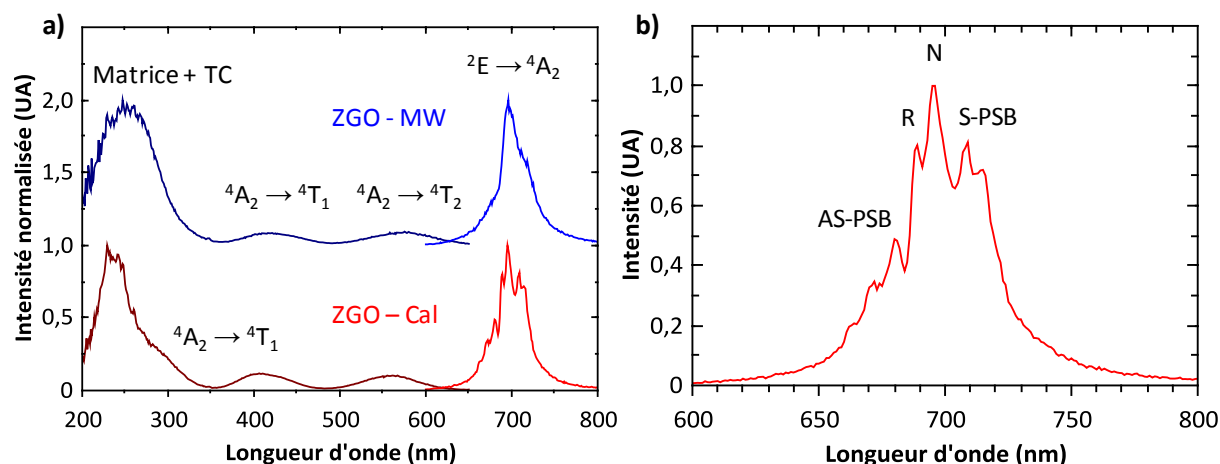
Figure 3.4 : a) Spectres d'excitation de la photoluminescence (traits foncés) ( \lambda_{em} = 695 nm) et spectres de la photoluminescence (traits clairs) ( \lambda_{ex} = 254 nm) de nanoparticules ZGO – MW (en bleu) et ZGO – Cal (en rouge) ; b) Zoom sur le spectre de photoluminescence ( \lambda_{ex} = 254 nm) de nanoparticules ZGO – Cal.
