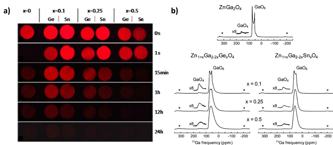
Figure 4.4 : \text{Zn}_{1+x}\text{Ga}_{2-2x}\text{Ge}_x\text{O}_4:\text{Cr}^{3+} ( 0,5\% ) massif, x variant entre 0 et 0,5. a) Déclins de la luminescence persistante sur des pastilles excitées pendant 1 min avec une lampe UV ; b) Spectres RMN ^{71}\text{Ga} MAS. Adapté d'Allix et al. 9 .
