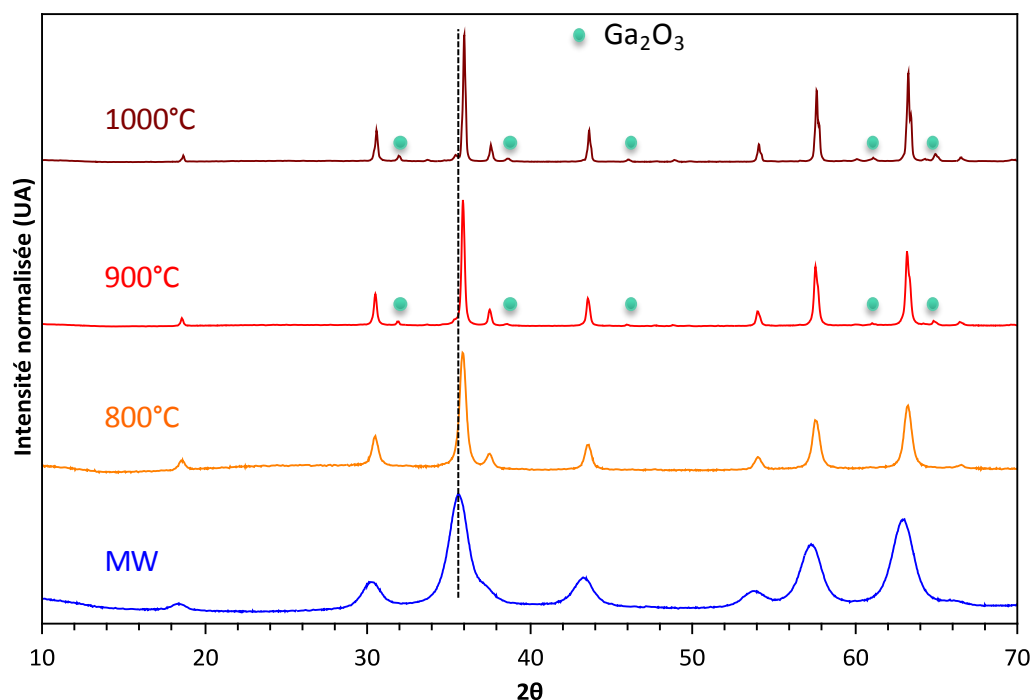
Figure 2.13 : Diffractogrammes de RX correspondant aux différentes températures de calcination de nanoparticules de \text{ZnGa}_2\text{O}_4:\text{Cr}^{3+}_{(0,5\%)} .
