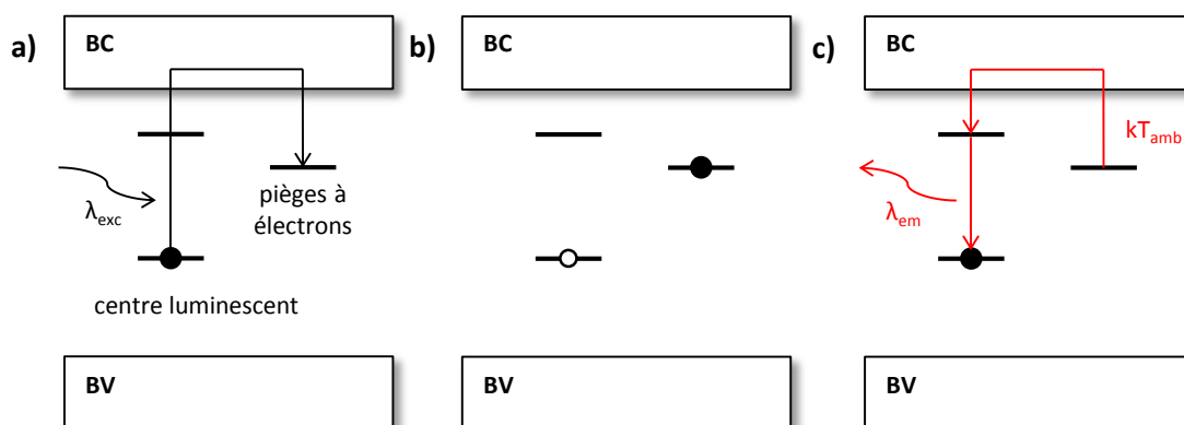
Figure 1.4 : Mécanisme simplifié de la luminescence persistante : a) Excitation du luminophore, création d'un exciton et piégeage de l'électron ; b) État métastable ; c) Dépiégeage progressif des électrons et recombinaison sur le centre luminescent.
