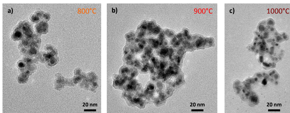
Figure 2.18 : Images MET de nanoparticules de \text{ZnGa}_2\text{O}_4 : \text{Cr}^{3+}_{(0,5\%)} @ \text{SiO}_2 en fonction de la température de calcination : a) 800°C ; b) 900°C ; c) 1000°C.
