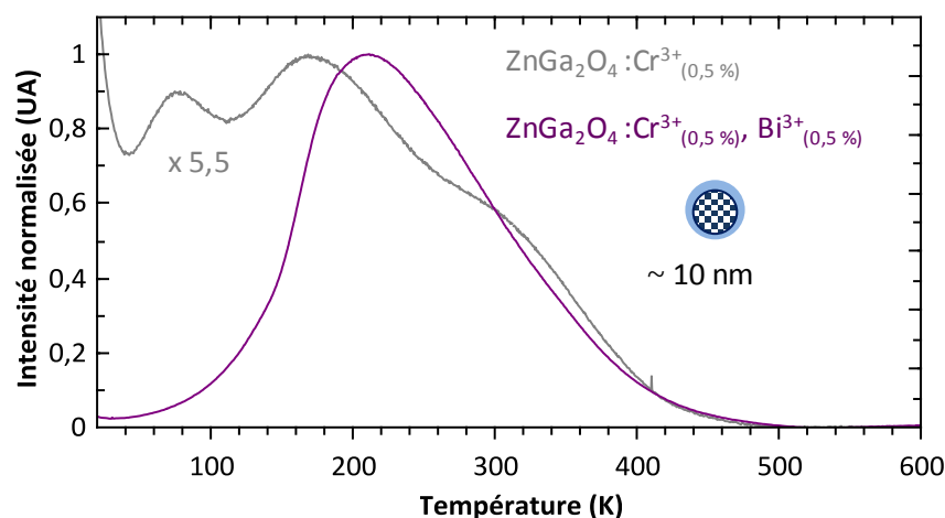
Figure 4.18 : Courbes de thermoluminescence de nanoparticules de \text{ZnGa}_2\text{O}_4:\text{Cr}^{3+}_{(0,5\%)}@ \text{SiO}_2 calcinées 1000^\circ\text{C} 2 h et de \text{ZnGa}_2\text{O}_4:\text{Cr}^{3+}_{(0,5\%)}, \text{Bi}^{3+}_{(0,5\%)}@ \text{SiO}_2 calcinées 1000^\circ\text{C} 2 h de 10 à 600 K ( 10 \text{ K.min}^{-1} ) enregistrées après 5 min d'excitation UV ( \lambda_{\text{ex}} = 254 \text{ nm} ) à 10 K.
