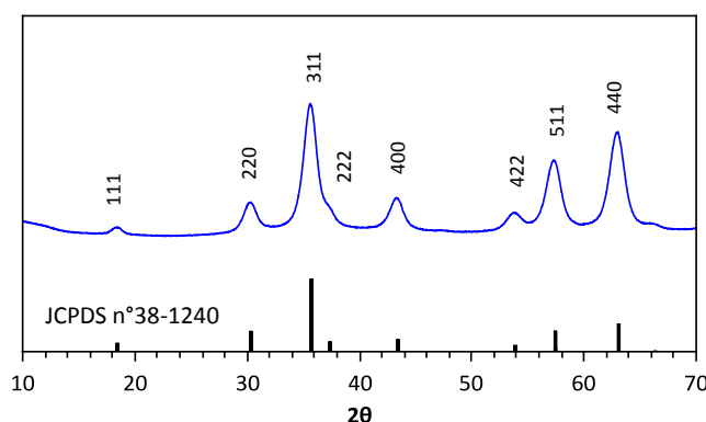
Figure 2.11 : Diffractogramme de RX de nanoparticules de \text{ZnGa}_2\text{O}_4:\text{Cr}^{3+}_{(0,5\%)} après synthèse hydrothermale assistée par chauffage micro-onde.
