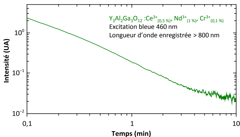
Figure 5.37 : Déclin de la luminescence persistante enregistré après 5 min d'excitation avec une lampe Xe (filtre passe bande 460 nm) de nanoparticules de \text{Y}_3\text{Al}_2\text{Ga}_3\text{O}_{12} : \text{Ce}^{3+}_{(0,5\%)}, \text{Nd}^{3+}_{(1\%)}, \text{Cr}^{3+}_{(0,1\%)} .
