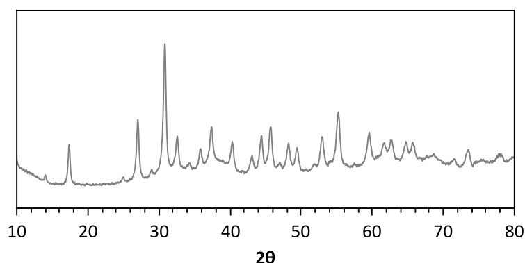
Figure 5.26 : Diffractogramme de RX du précurseur obtenu après synthèse hydrothermale assistée par chauffage micro-onde (200°C, 1 h).
