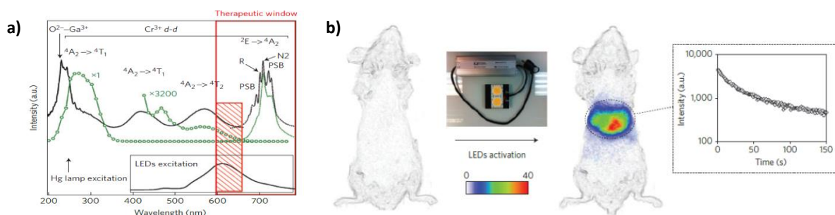
Figure 1.13 : a) Spectre d'excitation de la photoluminescence (trait plein noir), spectre de photoluminescence (trait pointillé noir), et spectre d'excitation de la luminescence persistante (trait et points vert) ; b) Luminescence persistante activée à travers les tissus de l'animal pendant 2 min avec une LED orange/rouge. L'encart présente le déclin de luminescence persistante correspondant au signal provenant du foie. Adapté de Maldiney et al. 44 .
