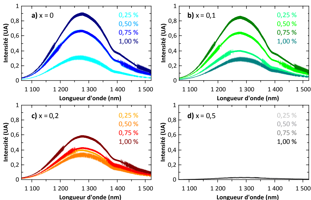
Figure 5.3 : Spectres de photoluminescence ( \lambda_{ex} = 365 nm) de nanoparticules de Zn_{1+x}Ga_{2-2x}Ge_xO_4:Ni^{2+}_{(y\%)} calcinées 2 h à 800°C en fonction de la teneur en nickel et en germanium a) x = 0 ; b) x = 0,1 ; c) x = 0,2 ; d) x = 0,5 .
