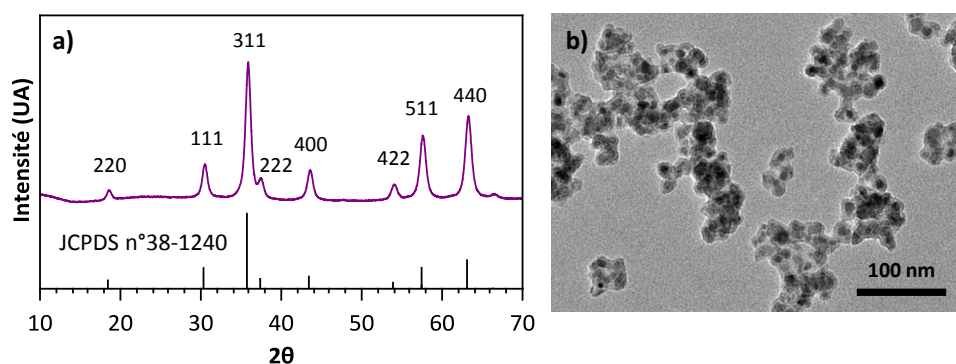
Figure 4.6 : Caractérisation structurale et morphologique de nanoparticules de \text{ZnGa}_2\text{O}_4 : \text{Cr}^{3+}_{(0,5 \%)} \text{Bi}^{3+}_{(0,5 \%)} @ \text{SiO}_2 calcinées 1000°C 2 h. a) Diffractogramme de RX ; b) Image MET.
