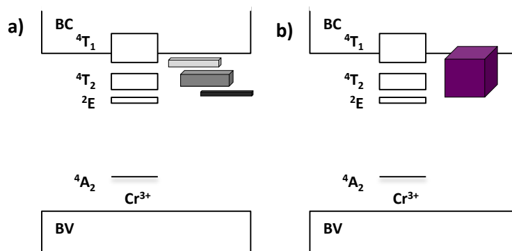
Figure 4.19 : Représentation schématique de la profondeur et de la distribution des pièges dans a) Nanoparticules de \text{ZnGa}_2\text{O}_4:\text{Cr}^{3+}_{(0,5\%)}@ \text{SiO}_2 calcinées 1000^\circ\text{C} 2 h ; b) Nanoparticules de \text{ZnGa}_2\text{O}_4:\text{Cr}^{3+}_{(0,5\%)}, \text{Bi}^{3+}_{(0,5\%)}@ \text{SiO}_2 calcinées 1000^\circ\text{C} 2 h.
