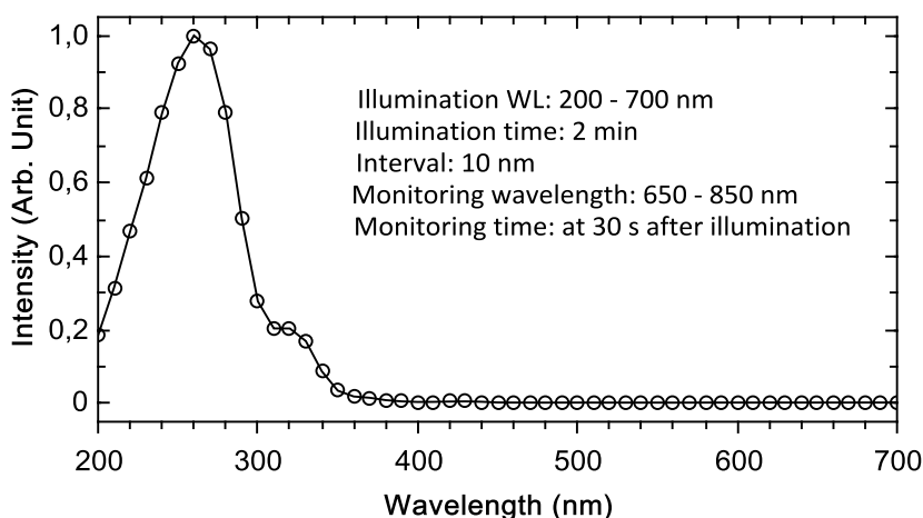
Figure VIII.5 : Spectre d'excitation de la luminescence persistante de nanoparticules de \text{LaAlO}_3:\text{Cr}^{3+}\text{-Sm}^{3+} obtenues par coprécipitation et traitement thermique à 1000^\circ\text{C} pendant 2 h.
