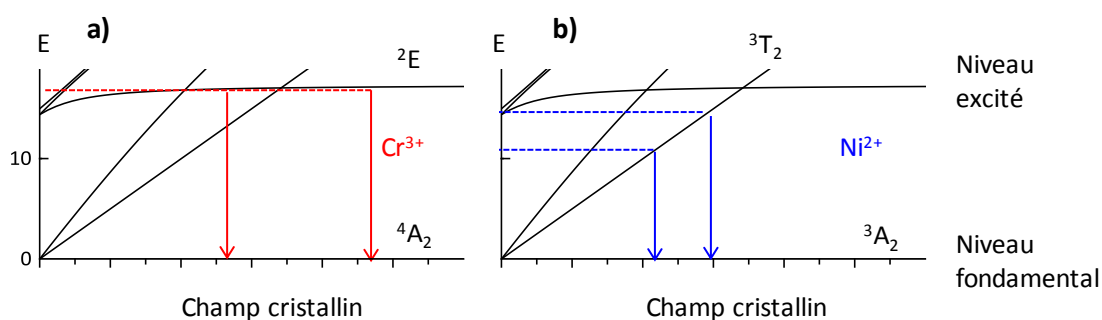
Figure 5.10 : Représentation schématique des niveaux d'énergie impliqués dans l'émission des ions a) \text{Cr}^{3+} ; b) \text{Ni}^{2+} .
