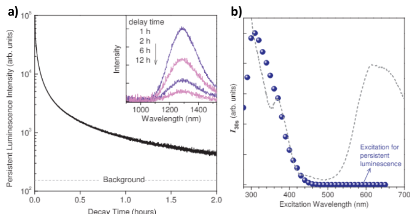
Figure 5.1 : a) Déclin de la luminescence persistante de \text{Zn}_3\text{Ga}_2\text{Ge}_2\text{O}_{10} : \text{Ni}^{2+} après 20 min d'excitation à 300 nm. L'encart présente les spectres d'émission de la luminescence persistante ; b) Spectre d'excitation de la luminescence persistante (points bleus) et spectre d'excitation de la photoluminescence (courbe en pointillés gris). Adapté de Liu et al. 1 .
