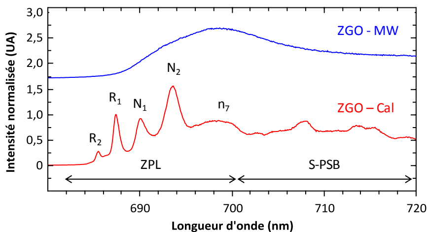
Figure 3.5 : Spectres de photoluminescence sous excitation laser ( \lambda_{ex} = 430 nm) et à 25 K (réseau 1200 traits/mm, haute résolution) de nanoparticules ZGO – MW (en bleu) et ZGO – Ca (en rouge).
