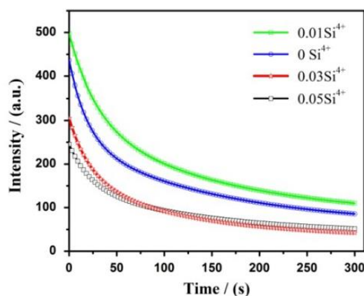
Figure 4.2 : Déclin de la luminescence persistante de \text{ZnGa}_2\text{O}_4:\text{Cr}^{3+}_{(0.5\%)}, \text{Si}^{4+}_{(x\%)} enregistrés après 5 min d'excitation UV ( \lambda_{\text{ex}} = 254 \text{ nm} ). Adapté de Hu et al. 4 .
