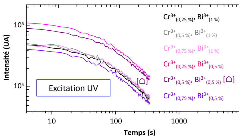
Figure 4.9 : Déclin de la luminescence persistante en fonction de la concentration en dopants des composés de \text{ZnGa}_2\text{O}_4:\text{Cr}^{3+}_{(x\%)}, \text{Bi}^{3+}_{(y\%)}@ \text{SiO}_2 calcinées 1000^\circ\text{C} 2 h enregistrés après 2 min d'excitation UV ( \lambda_{\text{ex}} = 254 \text{ nm} ), 1 min de délai avant le début de l'acquisition. Système de détection Optima, Biospace. La flèche indique l'échantillon sélectionné pour l'étude.
