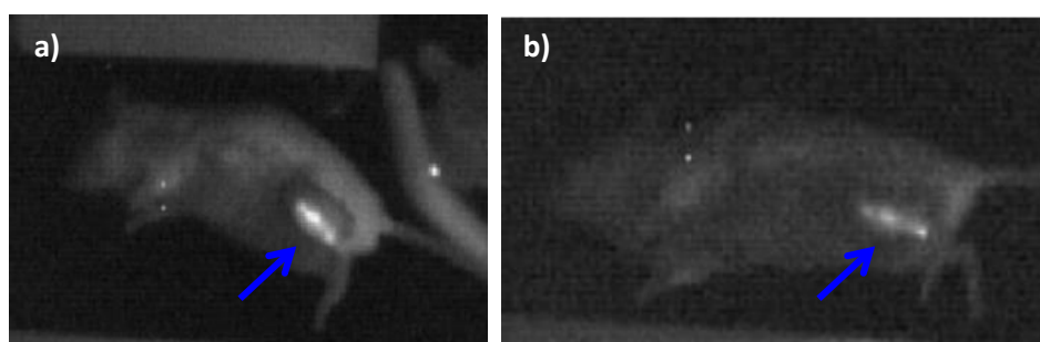
Figure 5.48 : Imagerie in vivo sous excitation à 455 nm réalisée avec des nanoparticules de \text{Y}_3\text{Al}_2\text{Ga}_3\text{O}_{12}:\text{Ce}^{3+}_{(0,5\%)}, \text{Nd}^{3+}_{(1\%)}, \text{Cr}^{3+}_{(0,1\%)} hydroxylées injectées intramusculairement. Caméra Xenics a) immédiatement après l'injection ; b) 24 h après l'injection.
