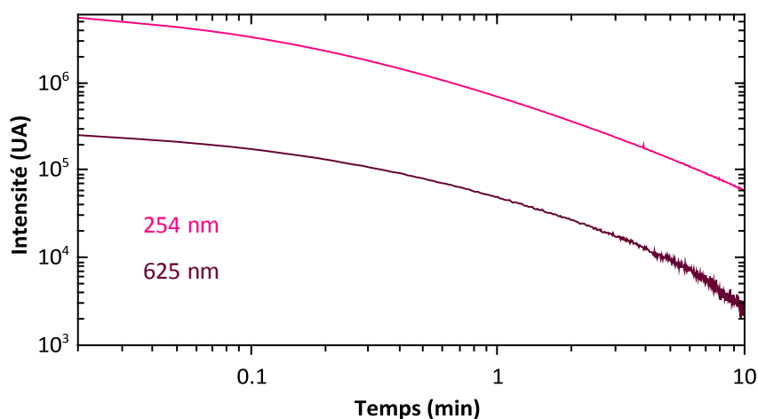
Figure 4.28 : Déclin de la luminescence persistante de nanoparticules de \text{Zn}_{1,1}\text{Ga}_{1,8}\text{Ge}_{0,1}\text{O}_4:\text{Cr}^{3+}_{(0,5 \%)} calcinées 2 h à 800°C enregistré 5 s après 2 min d'excitation UV ( \lambda_{\text{ex}} = 254 \text{ nm} ) ou rouge ( \lambda_{\text{ex}} = 625 \text{ nm} ).
