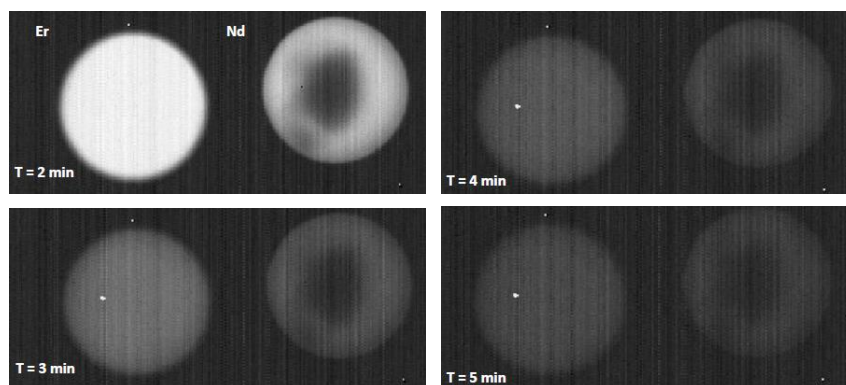
Figure 5.43 : Déclin de la luminescence persistante enregistré après 1 min sous excitation à 455 nm, caméra Princeton. Céramiques ayant pour composition : Y_3Al_2Ga_3O_{12} : Ce^{3+}_{(0,5\%)}, Nd^{3+}_{(1\%)}, Cr^{3+}_{(0,1\%)} et Y_3Al_2Ga_3O_{12} : Ce^{3+}_{(0,5\%)}, Er^{3+}_{(2,1\%)}, Cr^{3+}_{(0,1\%)} .
