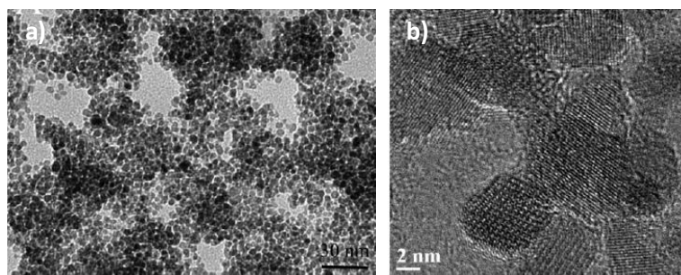
Figure 2.2 : Synthèse solvothermale de nanoparticules de \text{ZnGa}_2\text{O}_4 a) Image MET ; b) Image HRTEM. Adapté de Cao et al. 13 .
