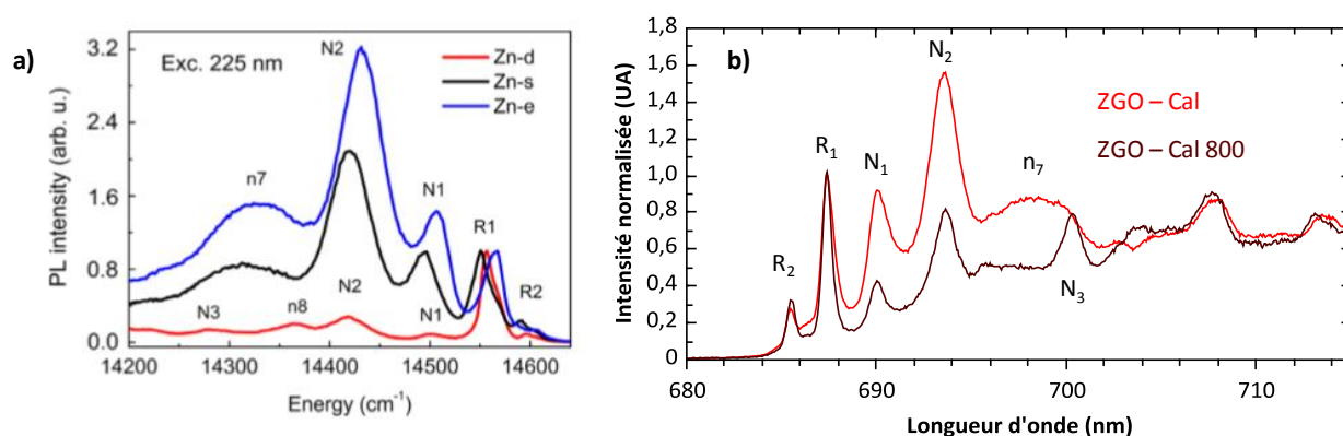
Figure 3.20 : Spectres de photoluminescence a) de ZnGa_2O_4:Cr^{3+} massif sous excitation à 225 nm à 20 K. Adapté de Gourier et al. 4 ; b) de nanoparticules ZGO – Cal et ZGO – Cal 800 sous excitation laser ( \lambda_{ex} = 430 nm) et à 25 K (réseau 1200 traits/mm, haute résolution).
