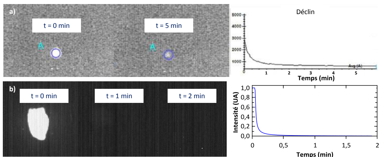
Figure 5.41 : Luminescence persistante de nanoparticules de \text{ZnGa}_2\text{O}_4:\text{Ni}^{2+}_{(0,75\%)} calcinées 800^\circ\text{C} 2 h après 2 min d'excitation à 365 nm enregistré avec a) la caméra Xenics ; b) la caméra Princeton.
