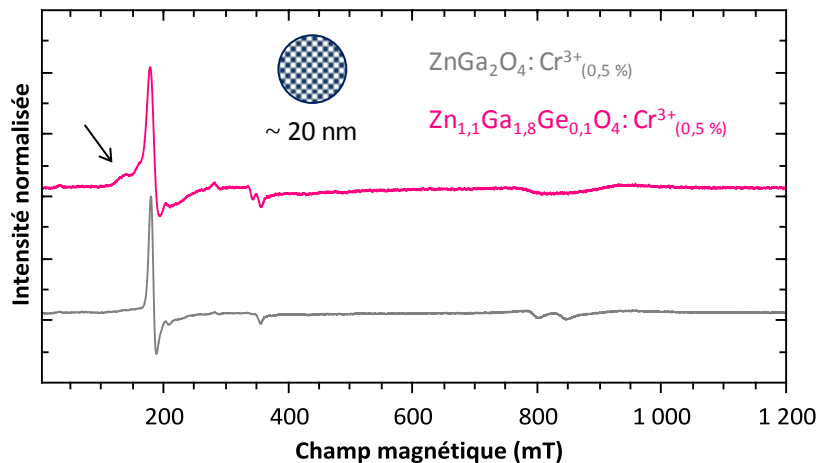
Figure 4.30 : Spectres RPE de nanoparticules de ZnGa_2O_4:Cr^{3+}_{(0,5\%)} calcinées 2 h à 800^\circ C et de Zn_{1,1}Ga_{1,8}Ge_{0,1}O_4:Cr^{3+}_{(0,5\%)} calcinées 2 h à 800^\circ C . La flèche noire indique l'épaulement à 160 mT.
