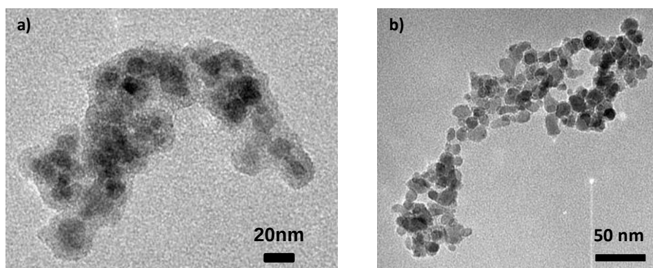
Figure VI.1 : Images MET a) Nanoparticules ZGO – Cal avant la dissolution de la couche de silice ; b) Nanoparticules ZGO – Cal après traitement avec NH 5 F 2 0,1 mol.L -1 pour dissoudre la couche de SiO 2 .
