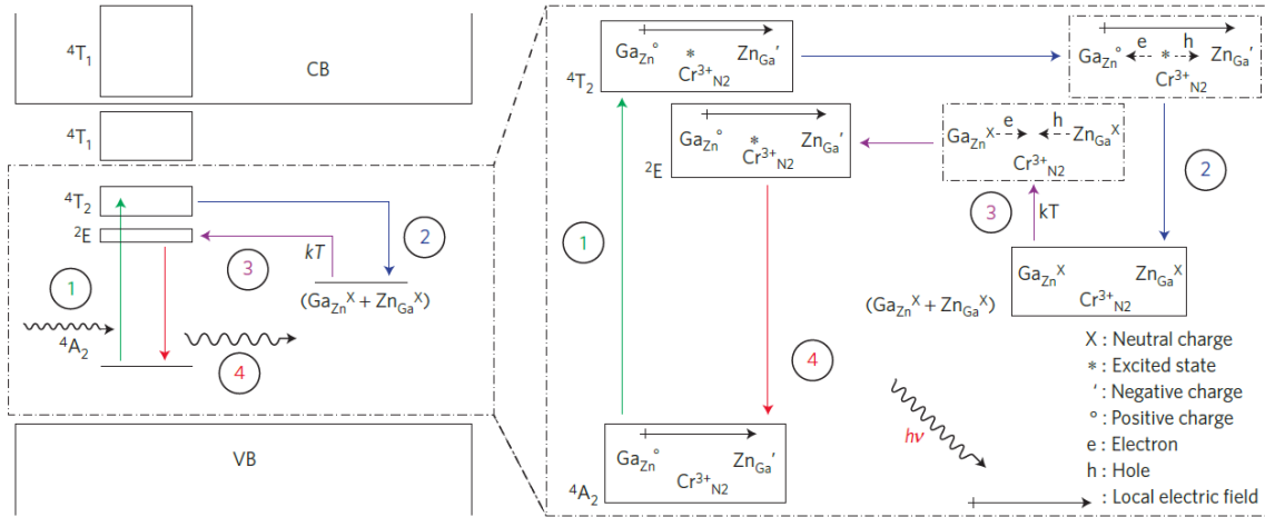
Figure 1.14 : Mécanisme de luminescence persistante après excitation visible de \text{ZnGa}_2\text{O}_4:\text{Cr}^{3+} . Adapté de Maldiney et al. 44 .
