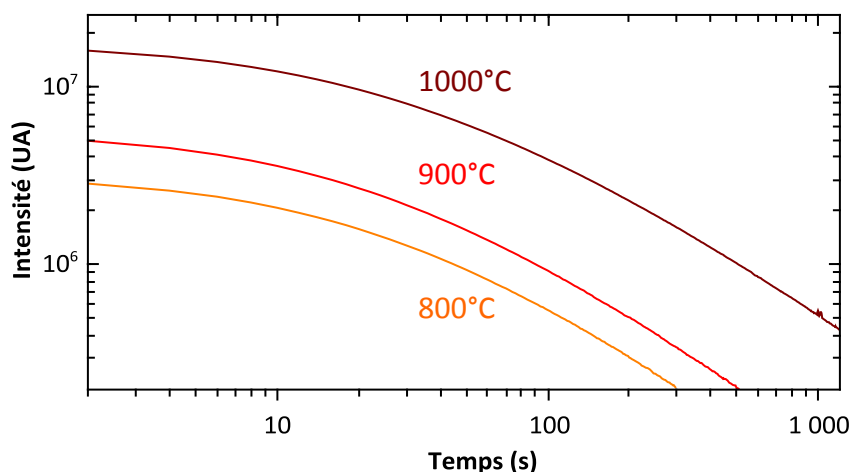
Figure 2.15 : Déclin de la luminescence persistante de nanoparticules de \text{ZnGa}_2\text{O}_4:\text{Cr}^{3+}_{(0,5\%)} enregistré 5 s après 2 min d'excitation UV ( \lambda_{\text{ex}} = 254 \text{ nm} ) en fonction de la température de calcination.
