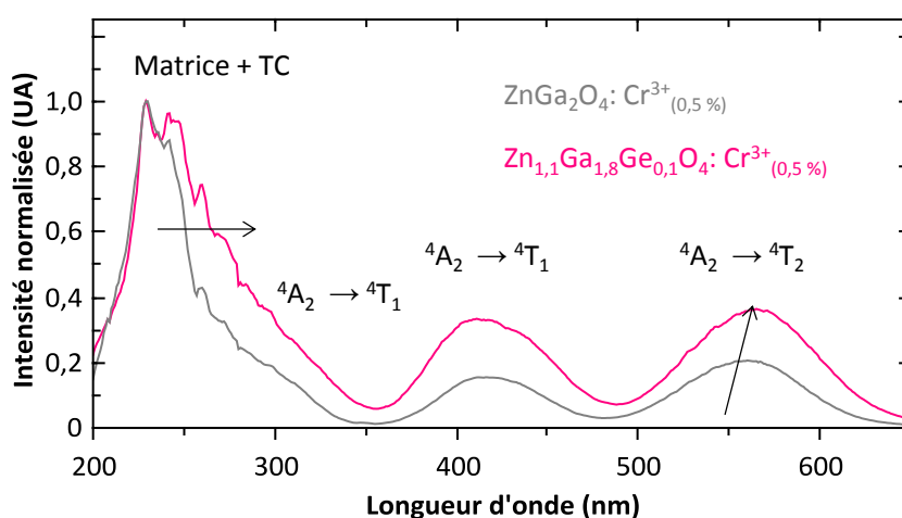
Figure 4.21 : Spectres d'excitation de la photoluminescence ( \lambda_{em} = 695 nm) de nanoparticules de \text{ZnGa}_2\text{O}_4:\text{Cr}^{3+}_{(0,5\%)} calcinées 2 h à 800^\circ\text{C} et de \text{Zn}_{1,1}\text{Ga}_{1,8}\text{Ge}_{0,1}\text{O}_4:\text{Cr}^{3+}_{(0,5\%)} calcinées 2 h à 800^\circ\text{C} .
