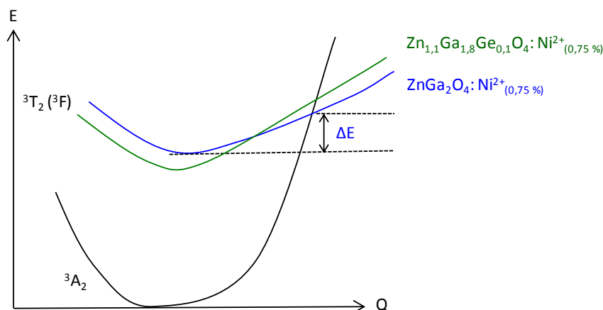
Figure 5.12 : Représentation schématique de l'énergie d'activation de nanoparticules \text{ZnGa}_2\text{O}_4:\text{Ni}^{2+}_{(0,75\%)} calcinées 2 h à 800^\circ\text{C} et de \text{Zn}_{1,1}\text{Ga}_{1,8}\text{Ge}_{0,1}\text{O}_4:\text{Ni}^{2+}_{(0,75\%)} calcinées 2 h à 800^\circ\text{C} .
