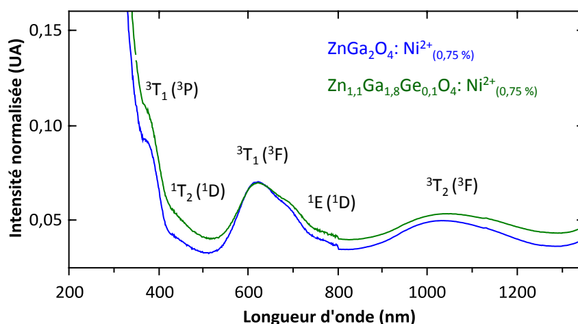
Figure 5.4 : Spectres d'absorption de nanoparticules de \text{ZnGa}_2\text{O}_4:\text{Ni}^{2+}_{(0,75\%)} calcinées 2 h à 800°C et de \text{Zn}_{1,1}\text{Ga}_{1,8}\text{Ge}_{0,1}\text{O}_4:\text{Ni}^{2+}_{(0,75\%)} calcinées 2 h à 800°C.
