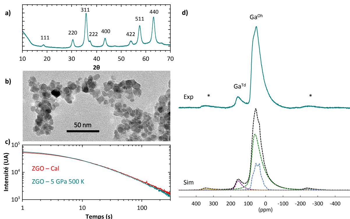
Figure 2 : Cristallisation de nanoparticules de \text{ZnGa}_2\text{O}_4:\text{Cr}^{3+}_{(0,5\%)} sous une pression de 5 GPa à 227°C pendant 10 min. a) Diffractogramme de RX ; b) Images MET ; c) Déclin de la luminescence persistante de nanoparticules de \text{ZnGa}_2\text{O}_4:\text{Cr}^{3+}_{(0,5\%)} enregistré 5 s après 2 min d'excitation UV ( \lambda_{\text{ex}} = 254 \text{ nm} ) ; d) Spectres de RMN ^{71}\text{Ga} MAS (champ magnétique de 16,5 T, fréquence de rotation = 62 kHz, trait plein). Les bandes de rotation sont indiquées par un astérisque et les contributions individuelles sont représentées en traits pointillés.
