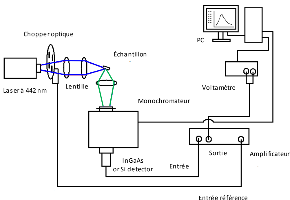
Figure 5.35 : Dispositif optique pour réaliser un spectre de photoluminescence. Adapté de J. Xu.
