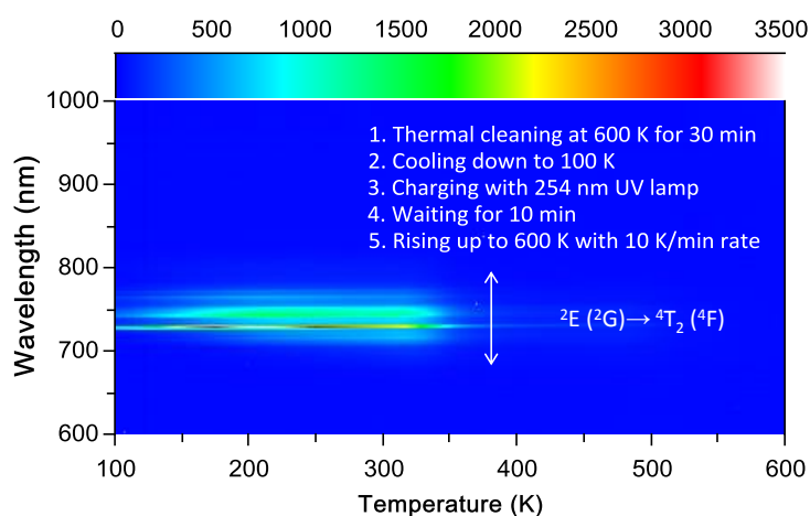
Figure VIII.6 : Spectre 2D de thermoluminescence de nanoparticules de \text{LaAlO}_3:\text{Cr}^{3+}\text{-Sm}^{3+} obtenues par coprécipitation et traitement thermique à 1000^\circ\text{C} pendant 2 h.
