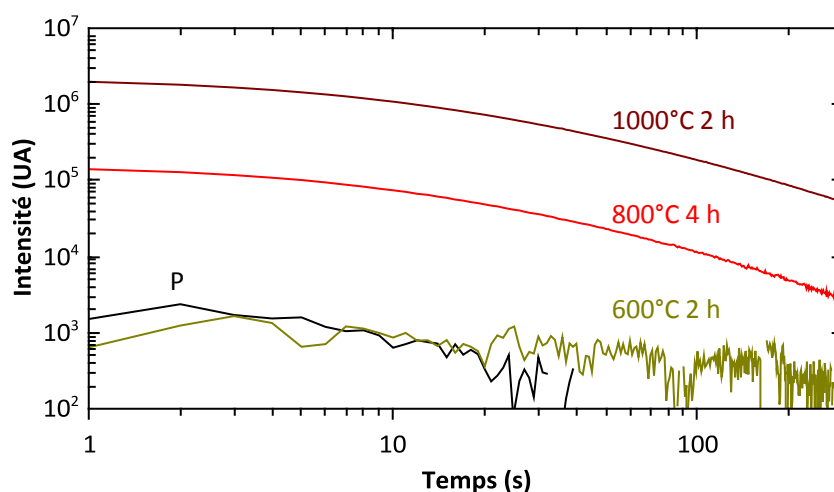
Figure 5.24 : Déclin de la luminescence persistante de Y_3Al_2Ga_3O_{12}:Cr^{3+} enregistré 5 s après 2 min d'excitation UV ( \lambda_{ex} = 254 nm) en fonction des conditions de calcination.
