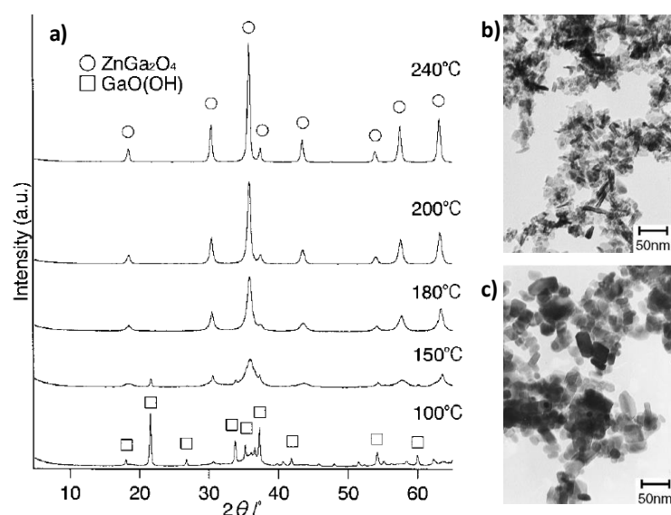
Figure 2.1 : Synthèse de nanoparticules de \text{ZnGa}_2\text{O}_4 par voie hydrothermale a) Diffractogrammes de RX et images MET de NPs synthétisées à b) 180°C et c) 240°C. Adapté d'Hirano et al. 12 .
