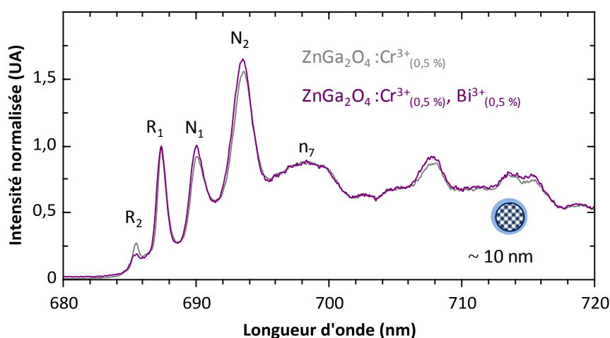
Figure 4.12 : Spectres de photoluminescence sous excitation laser ( \lambda_{\text{ex}} = 430 \text{ nm} ) et à 25 \text{ K} (réseau 1200 traits/mm, haute résolution) de nanoparticules de \text{ZnGa}_2\text{O}_4:\text{Cr}^{3+}_{(0,5\%)}\text{@SiO}_2 calcinées 1000^\circ\text{C} 2 h et de \text{ZnGa}_2\text{O}_4:\text{Cr}^{3+}_{(0,5\%)}, \text{Bi}^{3+}_{(0,5\%)}\text{@SiO}_2 calcinées 1000^\circ\text{C} 2 h. Les spectres sont normalisés à l'aide de la raie R_1 .
