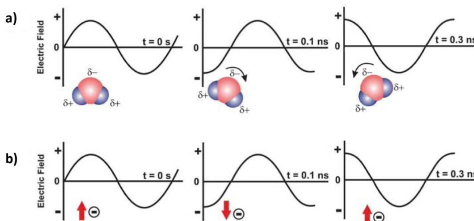
Figure 2.6 : Mécanisme de chauffage sous irradiation micro-onde : a) polarisation dipolaire b) conduction ionique. Adapté de Bilecka et al. 25 .
