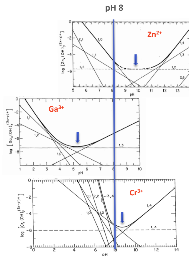
Figure 2.9 : Superposition des diagrammes de solubilité des ions Zn^{2+} , Ga^{3+} et Cr^{3+} . Adapté de Baes et al. 26 .
