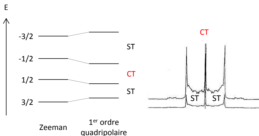
Figure IV.2 : Effet de l'interaction quadripolaire au 1 er ordre en perturbation sur les niveaux d'énergie d'un noyau de spin I = 3/2 ( \gamma > 0 ). Spectre de poudre correspondant, en mode statique.
