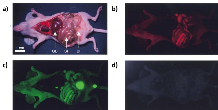
Figure 1.8 : Autofluorescence des tissus selon les longueurs d'onde d'excitation et d'émission utilisées. a) Image en lumière blanche d'une souris après sacrifice, les flèches indiquent la vésicule biliaire (GB), l'intestin grêle (SI) et la vessie (BI). L'autofluorescence des tissus lors de l'utilisation de trois dispositifs de filtres d'émission/excitation différents : b) Filtre vert/rouge (525 – 555 nm/590 – 650 nm) ; Filtre bleu/vert (460 – 500 nm/505 – 560 nm) ; Filtre proche infrarouge (725 – 775 nm/790 – 830 nm). Adapté de Frangioni 39 .
