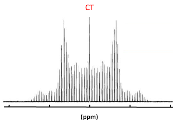
Figure IV.5 : Spectre MAS pour un noyau de spin I = 3/2 (fréquence MAS finie).
