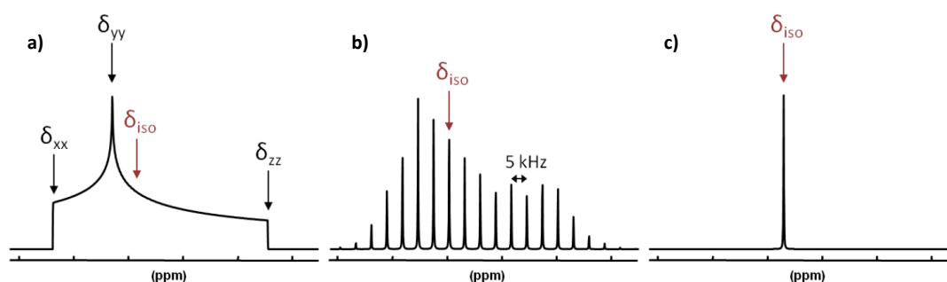
Figure IV.4 : Influence de l'interaction CSA et de la rotation à l'angle magique MAS a) Spectre statique ; b) MAS à fréquence égale à 5 kHz ; c) MAS en fréquence infinie. \delta_{iso} = \delta_{xx} + \delta_{yy} + \delta_{zz} . D'après la thèse de C. Leroy 3 .
