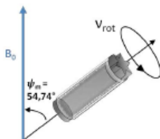
Figure IV.3 : Rotation à l'angle magique. \Psi_m vérifie \frac{1}{2}(3 \cos^2 \Psi - 1) = 0 . D'après la thèse de C. Leroy 3 .
