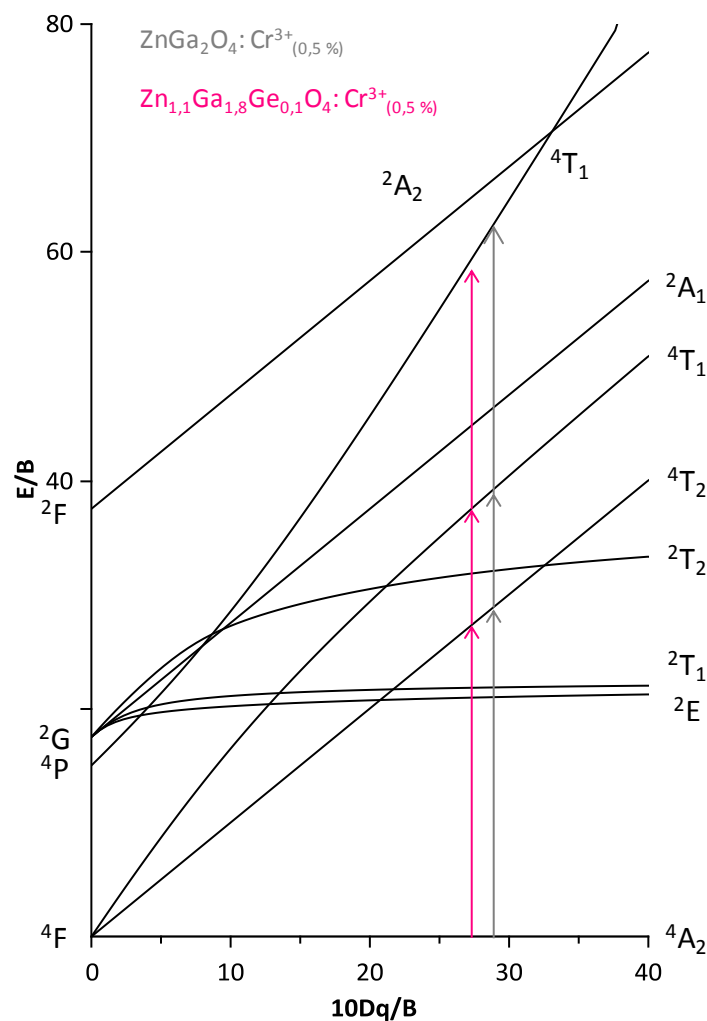
Figure 4.22 : Diagramme de Tanabe-Sugano pour l'ion \text{Cr}^{3+} (environnement octaédrique) d^3 .
