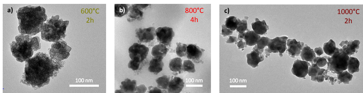
Figure 5.30 : Images MET de grenat \text{Y}_3\text{Al}_2\text{Ga}_3\text{O}_{12}:\text{Cr}^{3+} après calcination à a) 600°C 2 h ; b) 800°C 4 h ; c) 1000°C 2 h.
