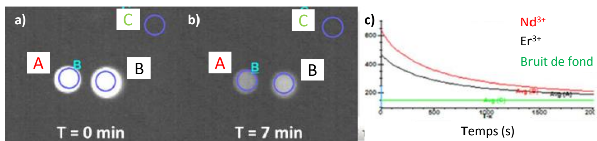
Figure 5.44 : Déclin de la luminescence persistante enregistré 5 s après 2 min d'excitation à 455 nm, caméra Xenics. Céramiques ayant pour composition : \text{Y}_3\text{Al}_2\text{Ga}_3\text{O}_{12} : \text{Ce}^{3+}_{(0,5\%)}, \text{Nd}^{3+}_{(1\%)}, \text{Cr}^{3+}_{(0,1\%)} (A) et \text{Y}_3\text{Al}_2\text{Ga}_3\text{O}_{12} : \text{Ce}^{3+}_{(0,5\%)}, \text{Er}^{3+}_{(2,1\%)}, \text{Cr}^{3+}_{(0,1\%)} (B), bruit de fond (C). a) à t = 0 min ; b) à t = 7 min ; c) Déclin correspondant.
