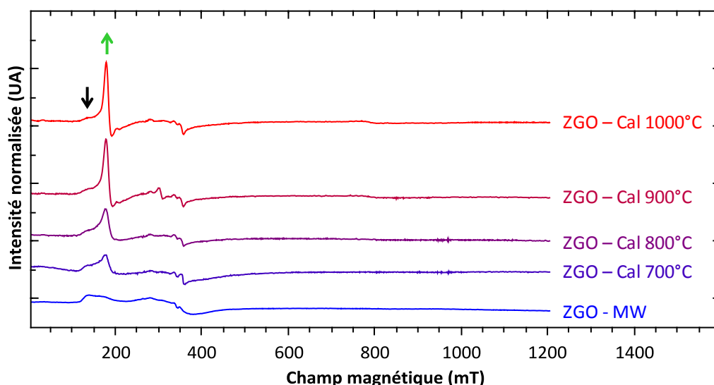
Figure 3.11 : Spectres RPE normalisés en bande X à température ambiante : influence de la température de calcination. La flèche noire montre l'évolution de la raie à 150 mT et la verte celle de la raie à 185 mT.
