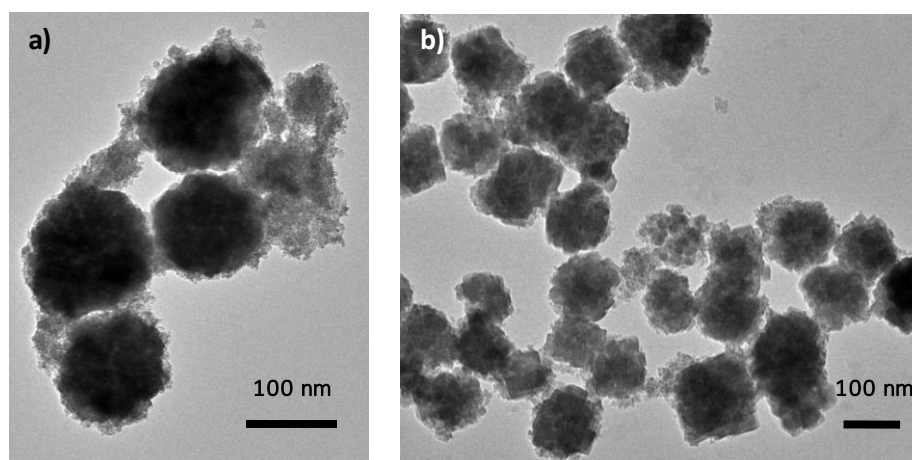
Figure 5.28 : Images MET du précurseur de grenat \text{Y}_3\text{Al}_2\text{Ga}_3\text{O}_{12}:\text{Cr}^{3+} après synthèse micro-onde ( 200^\circ\text{C} , 1 h) a) Lavage à l'eau ; b) Lavage à l'acide chlorhydrique 0,01 M.
