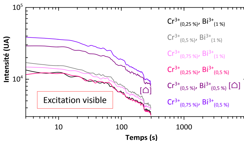
Figure 4.8 : Déclin de la luminescence persistante en fonction de la concentration en dopants des nanoparticules de \text{ZnGa}_2\text{O}_4:\text{Cr}^{3+}_{(x\%)}, \text{Bi}^{3+}_{(y\%)}@ \text{SiO}_2 calcinées 1000^\circ\text{C} 2 h enregistrés après 2 min d'excitation visible (LED orange/rouge), 1 min de délai avant le début de l'acquisition. Système de détection Optima, Biospace. La flèche indique l'échantillon sélectionné pour l'étude.
