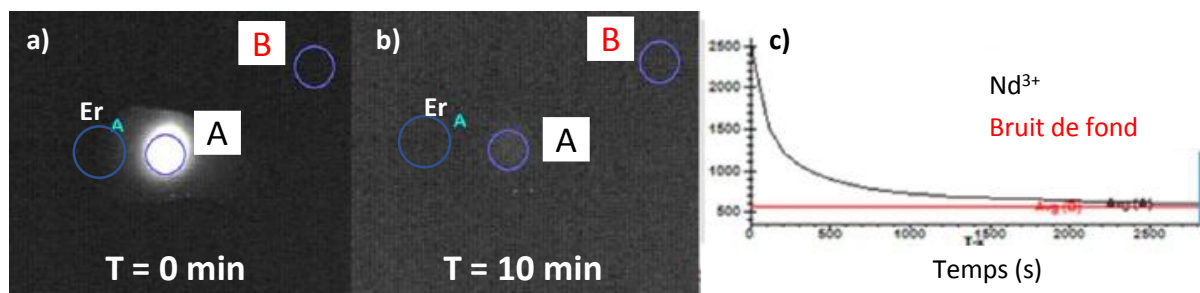
Figure 5.46 : Déclin de la luminescence persistante enregistré 20 s après 5 min d'excitation à 455 nm, caméra Xenics. Céramique ayant pour composition : Y_3Al_2Ga_3O_{12} : Ce^{3+}_{(0,5\%)}, Nd^{3+}_{(1\%)}, Cr^{3+}_{(0,1\%)} (A), Y_3Al_2Ga_3O_{12} : Ce^{3+}_{(0,5\%)}, Er^{3+}_{(2,1\%)}, Cr^{3+}_{(0,1\%)} et bruit de fond (B). a) à t = 0 min ; b) à t = 10 min ; c) Déclin correspondant.
