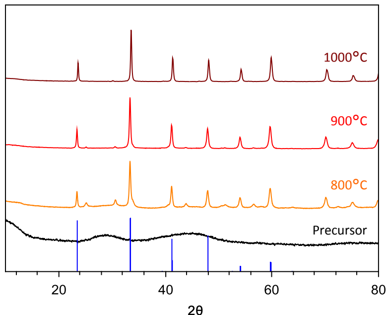
Figure VIII.2 : Diffractogrammes de RX correspondant aux différentes températures de calcination de nanoparticules de \text{LaAlO}_3:\text{Cr}^{3+}\text{-Sm}^{3+} .
