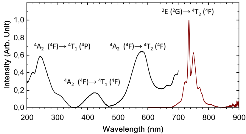
Figure VIII.4 : Spectres d'excitation de la photoluminescence ( \lambda_{em} = 735 nm) et spectre de photoluminescence ( \lambda_{ex} = 579 nm) de nanoparticules de \text{LaAlO}_3:\text{Cr}^{3+}\text{-Sm}^{3+} obtenues par coprécipitation et traitement thermique à 1000^\circ\text{C} pendant 2 h.
