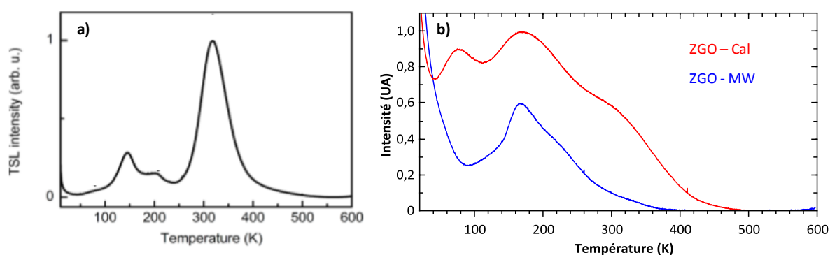
Figure 3.18 : Courbes de thermoluminescence a) \text{ZnGa}_2\text{O}_4:\text{Cr}^{3+} massif, de 10 à 600 K ( 10 \text{ K.min}^{-1} ) après 30 min d'excitation à 10 K. Adapté de Maldiney et al. 25 ; b) ZGO – MW (en bleu) et ZGO – Cal (en rouge) de 10 à 600 K ( 10 \text{ K.min}^{-1} ) après 5 min d'excitation UV ( \lambda_{\text{ex}} = 254 \text{ nm} ) à 10 K.
