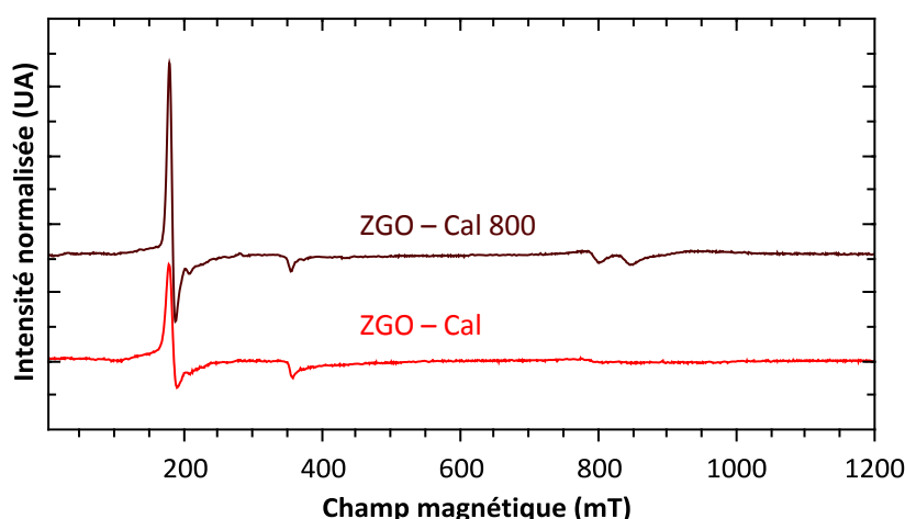
Figure 3.21 : Spectres RPE en bande X à température ambiante de nanoparticules de ZGO – Cal et ZGO – Cal 800.
