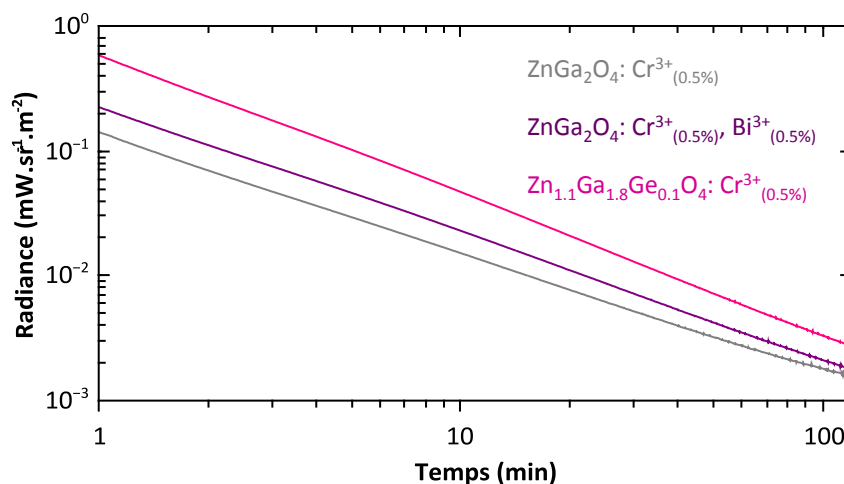
Figure 4.33 : Déclin de la luminescence persistante exprimé en radiance, des différentes nanoparticules de \text{ZnGa}_2\text{O}_4:\text{Cr}^{3+}_{(0,5\%)} calcinées 2 h à 800°C, \text{ZnGa}_2\text{O}_4:\text{Cr}^{3+}_{(0,5\%)}\text{Bi}^{3+}_{(0,5\%)} calcinées 2 h à 800°C et de \text{Zn}_{1,1}\text{Ga}_{1,8}\text{Ge}_{0,1}\text{O}_4:\text{Cr}^{3+}_{(0,5\%)} calcinées 2 h à 800°C. Signal enregistré après 5 min d'excitation UV ( \lambda_{\text{ex}} = 250 - 380 \text{ nm} ).
