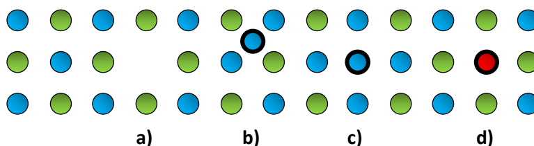
Figure 1.5 : Défauts ponctuels : a) lacune ; b) interstitiel ; c) substitution ; d) dopant en substitution.
