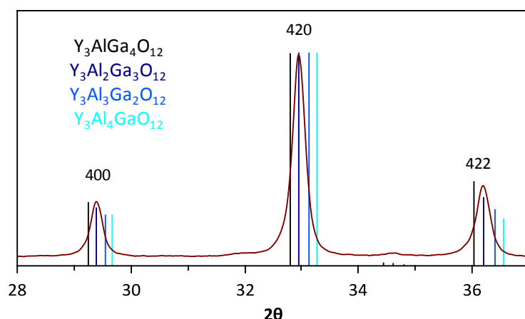
Figure 5.23 : Comparaison du diffractogramme de RX du composé Y_3Al_2Ga_3O_{12} synthétisé par coprécipitation et calciné 2 h à 1000^\circ C par rapport à celui de Y_3AlGa_4O_{12} (Fiche JCPDS n°01-089-6661), de Y_3Al_2Ga_3O_{12} (Fiche JCPDS n°01-089-6660), de Y_3Al_3Ga_2O_{12} (JCPDS n°01-089-6659), et de Y_3Al_4GaO_{12} (JCPDS n°01-089-6658).
