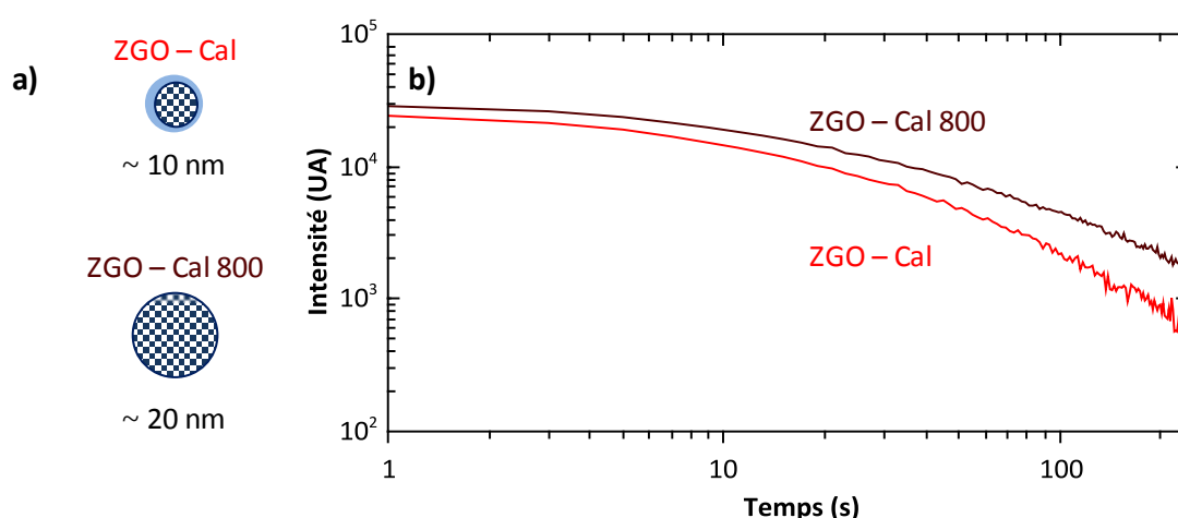
Figure 3.19 : a) Représentation schématique des nanoparticules ZGO – Cal et ZGO – Cal 800 ; b) Déclin de la luminescence persistante enregistrés 5 s après 2 min d'excitation UV ( \lambda_{\text{ex}} = 254 \text{ nm} ) de nanoparticules ZGO – Cal et ZGO – Cal 800.
