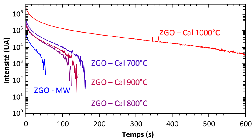
Figure 3.12 : Déclin de la luminescence persistante enregistré 5 s après 2 min d'excitation UV ( \lambda_{ex} = 254 nm) de nanoparticules ZGO calcinées à différentes températures. Les spectres sont réalisés dans les mêmes conditions expérimentales et avec les mêmes quantités de nanoparticules pour pouvoir comparer les échantillons entre eux.
