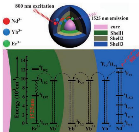
Figure 1.19 : Structure des nanoparticules cœur@coquille pour une émission à 1525 nm après une excitation à 800 nm et proposition de mécanisme de transfert d'énergie à travers les différentes couches de la structure. Adapté de Wang et al. 85 .
