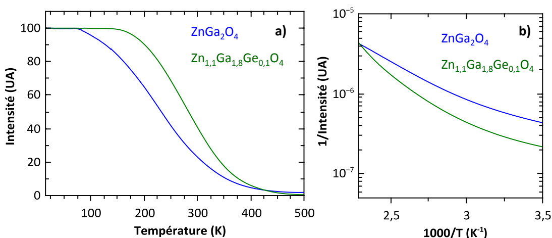
Figure 5.11 : a) Courbes de stabilité thermique ( \lambda_{ex} = 365 nm) de nanoparticules de \text{ZnGa}_2\text{O}_4:\text{Ni}^{2+}_{(0,75\%)} calcinées 2 h à 800°C et de \text{Zn}_{1,1}\text{Ga}_{1,8}\text{Ge}_{0,1}\text{O}_4:\text{Ni}^{2+}_{(0,75\%)} calcinées 2 h à 800°C ; b) Évolution de l'inverse de l'intensité en fonction de l'inverse de la température.
