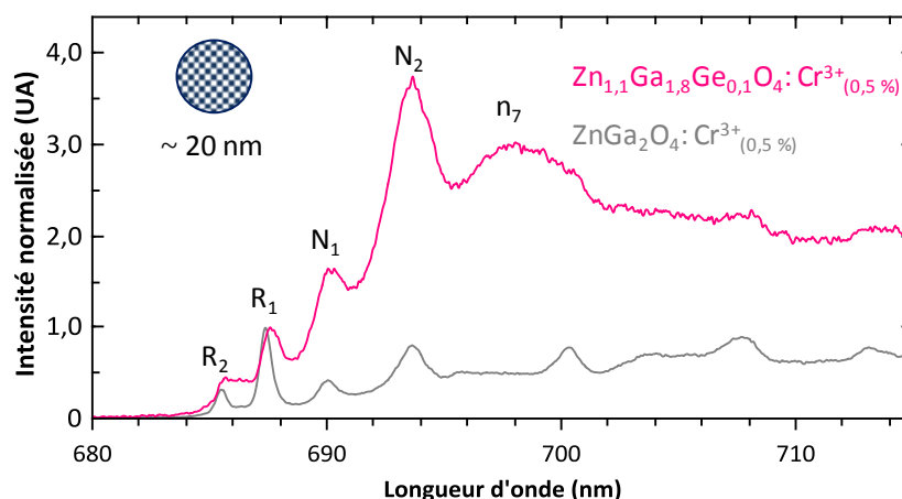
Figure 4.29 : Spectres de photoluminescence sous excitation laser ( \lambda_{ex} = 430 nm) et à 25 K (réseau 1200 traits/mm, haute résolution) de nanoparticules de \text{ZnGa}_2\text{O}_4:\text{Cr}^{3+}_{(0,5\%)} calcinées 2 h à 800°C et de \text{Zn}_{1,1}\text{Ga}_{1,8}\text{Ge}_{0,1}\text{O}_4:\text{Cr}^{3+}_{(0,5\%)} calcinées 2 h à 800°C.
