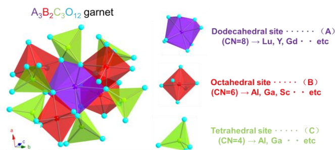
Figure 5.19 : Structure grenat. Adapté de J. Xu.
