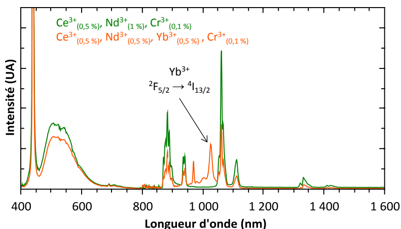
Figure 5.39 : Spectres de photoluminescence de nanoparticules de \text{Y}_3\text{Al}_2\text{Ga}_3\text{O}_{12} en fonction des codopants utilisés.
