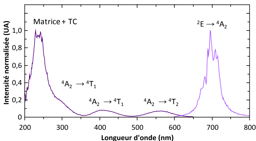
Figure 4.11 : Spectres d'excitation de la photoluminescence en trait foncé ( \lambda_{em} = 695 nm) et de photoluminescence en trait clair ( \lambda_{ex} = 254 nm) de nanoparticules de ZnGa_2O_4 : Cr^{3+}_{(0,5\%)}, Bi^{3+}_{(0,5\%)@SiO_2} calcinées 1000°C 2 h.
