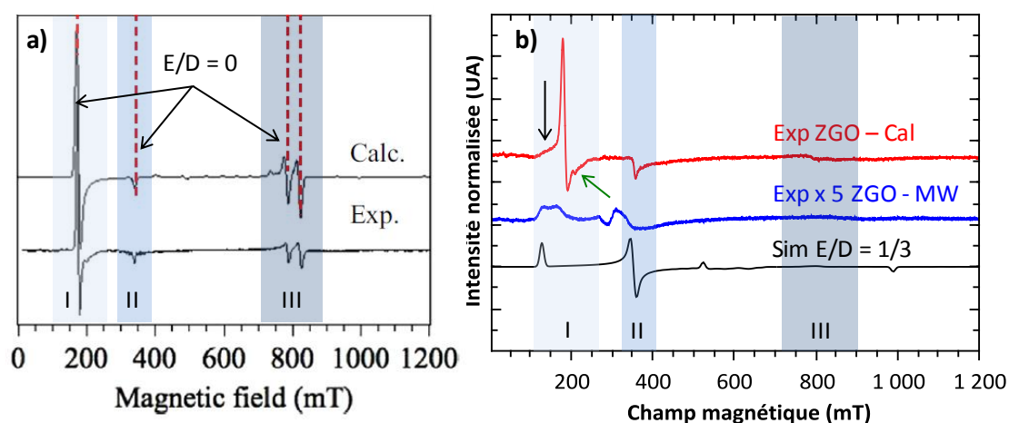
Figure 3.8 : Spectres RPE en bande X à température ambiante a) Spectres expérimental et simulé de \text{ZnGa}_2\text{O}_4:\text{Cr}^{3+} massif correspondant à E/D = 0 . Adapté de Gourier et al. 4 ; b) Spectres RPE expérimentaux de nanoparticules de ZGO – MW (en bleu) et ZGO – Cal (en rouge) et spectre simulé d'un \text{Cr}^{3+} avec E/D = 1/3 (en noir). La flèche noire indique l'épaule à 150 mT et la flèche verte indique les paires \text{Cr}^{3+}\text{-Cr}^{3+} .
