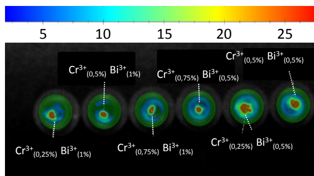
Figure 4.7 : Image de la luminescence persistante de nanoparticules de \text{ZnGa}_2\text{O}_4 : \text{Cr}^{3+}_{(x\%)}, \text{Bi}^{3+}_{(y\%)} @ \text{SiO}_2 calcinées 1000^\circ\text{C} 2 h enregistrée après 2 min d'excitation UV ( \lambda_{\text{ex}} = 254 \text{ nm} ). Acquisition du signal en même temps pour chaque composition.
