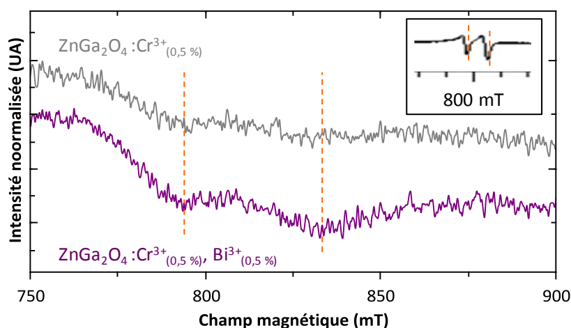
Figure 4.16 : Spectres RPE (bande X) normalisés de nanoparticules de \text{ZnGa}_2\text{O}_4:\text{Cr}^{3+}_{(0,5\%)}@ \text{SiO}_2 calcinées 1000^\circ\text{C} 2 h et de \text{ZnGa}_2\text{O}_4:\text{Cr}^{3+}_{(0,5\%)}, \text{Bi}^{3+}_{(0,5\%)}@ \text{SiO}_2 calcinées 1000^\circ\text{C} 2 h – Zoom de la région des 800 mT. L'encadré présente la même région pour un matériau \text{ZnGa}_2\text{O}_4:\text{Cr}^{3+} synthétisé par voie solide.
