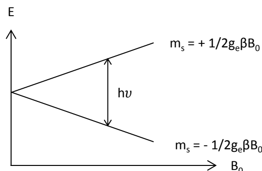
Figure 3.6 : Levée de dégénérescence induite par un champ magnétique B_0 pour un spin électronique, S = 1/2 .
