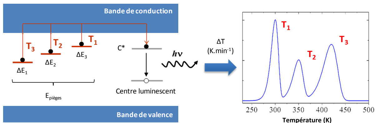
Figure 1.6 : Principe de la thermoluminescence.
