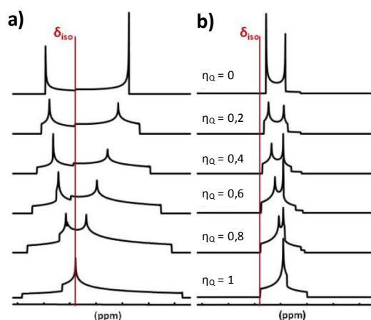
Figure IV.6 : Formes de raies théoriques de la transition centrale a) en mode statique ; b) en MAS à fréquence infinie pour différentes valeurs \eta_Q . D'après la thèse de C. Leroy 3 .
