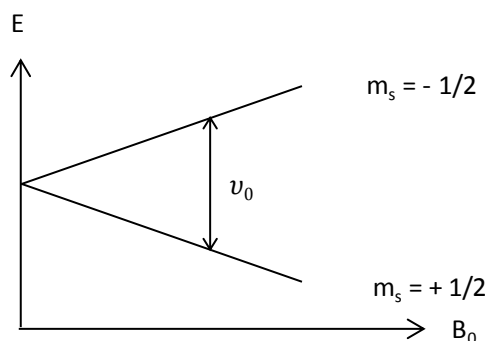
Figure IV.1 : Levée de dégénérescence induite par un champ magnétique B_0 pour un spin I = 1/2 et \gamma > 0 .
