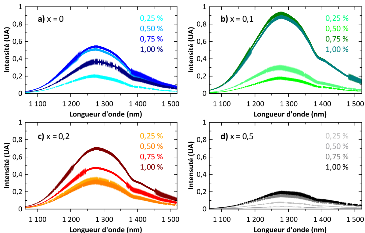
Figure IX.1 : Spectres de photoluminescence ( \lambda_{\text{ex}} = 625 \text{ nm} ) de nanoparticules de \text{Zn}_{1+x}\text{Ga}_{2-2x}\text{Ge}_x\text{O}_4:\text{Ni}^{2+} (y %) calcinées 2 h à 800°C en fonction de la teneur en nickel et en germanium a) x = 0 ; b) x = 0,1 ; c) x = 0,2 ; d) x = 0,5.
