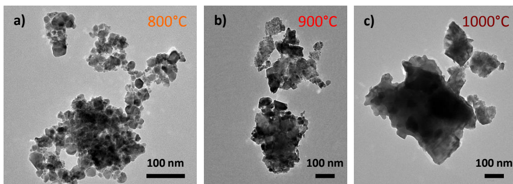
Figure 2.14 : Images MET de nanoparticules de \text{ZnGa}_2\text{O}_4:\text{Cr}^{3+}_{(0,5\%)} en fonction de la température de calcination : a) 800^\circ\text{C} ; b) 900^\circ\text{C} ; c) 1000^\circ\text{C} .
