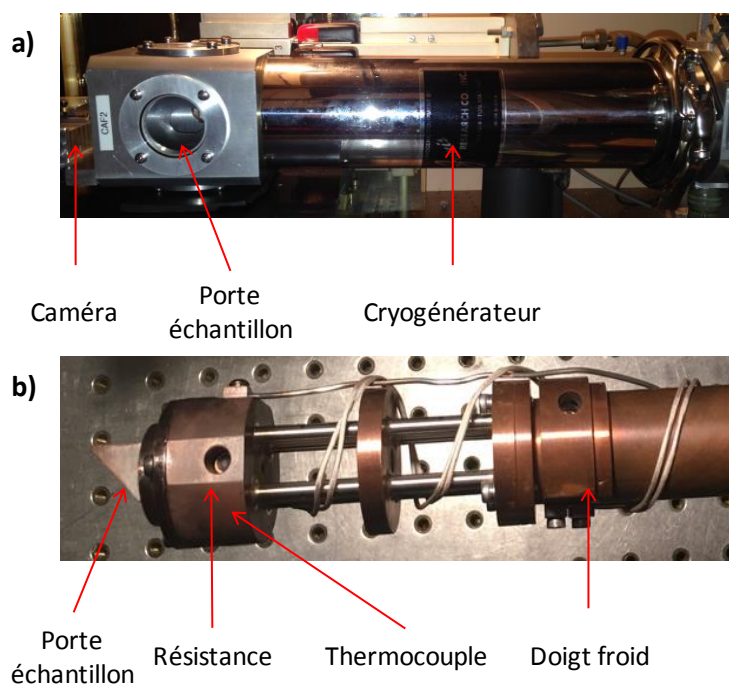
Figure 3.17 : Dispositif expérimental de l'expérience de thermoluminescence a) Vue d'ensemble ; b) Porte échantillon équipé du système de refroidissement et de chauffage.
