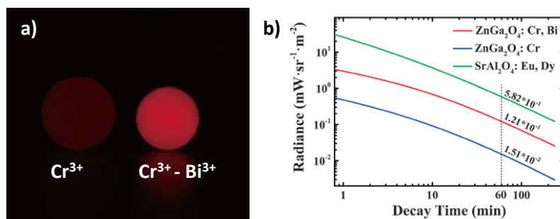
Figure 4.1 : Propriétés de luminescence persistante de \text{ZnGa}_2\text{O}_4:\text{Cr}^{3+} (0,5 %) et \text{ZnGa}_2\text{O}_4:\text{Cr}^{3+} (0,5 %), \text{Bi}^{3+} (1 %) massif. a) Photographie des échantillons 30 s après avoir coupé l'excitation à 330 nm ; b) Déclin de la luminescence persistante (en radiance) enregistrés après 5 min d'excitation UV ( \lambda_{\text{ex}} = 250 - 380 \text{ nm} ). Adapté de Zhuang et al. 3 .
