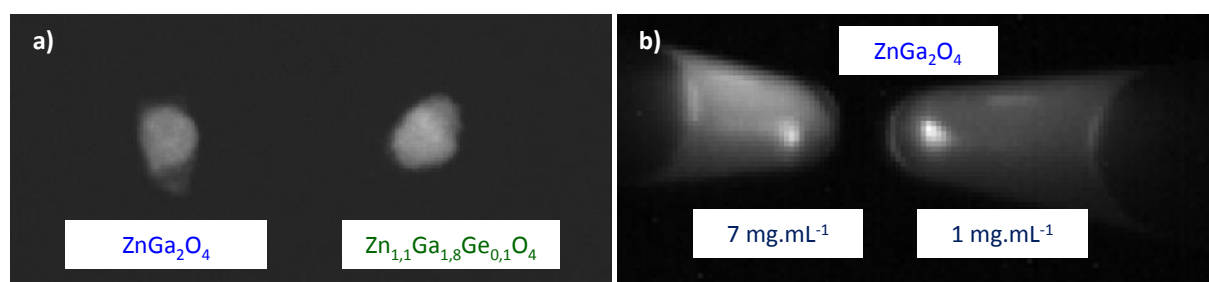
Figure 5.40 : Photoluminescence sous excitation à 365 nm de nanoparticules de \text{ZnGa}_2\text{O}_4:\text{Ni}^{2+}_{(0,75\%)} calcinées 800^\circ\text{C} 2 h : a) Sous forme de poudre, caméra Princeton ; b) En solution à deux concentrations différentes, caméra Hamamatsu.
