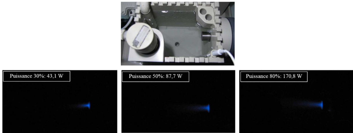
Figure 82 : Mise en évidence des zones chimiquement actives du réacteur par sonochimiluminescence en fonction de la puissance ultrasonore transmise, sans obstacle
