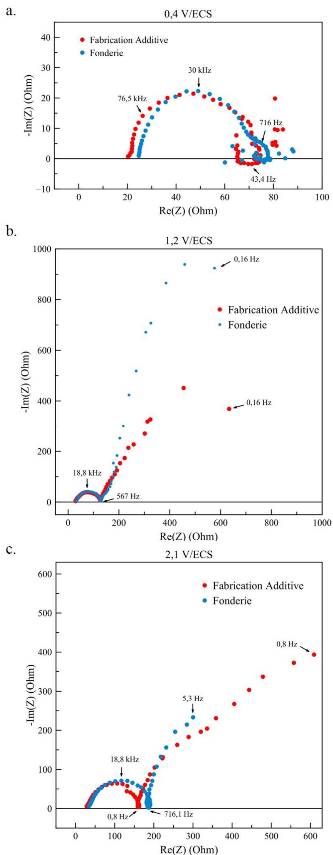
Figure 146 : Évolution en fonction du potentiel des diagrammes d'impédance des aciers inoxydables 316L issus de fonderie (bleu) et de fabrication additive (rouge) tracés en milieu \text{ChCl-EG} à 70^\circ\text{C} et 500 rpm : (a) 0,4 V/ECS, (b) 1,2 V/ECS et (c) 2,1 V/ECS
