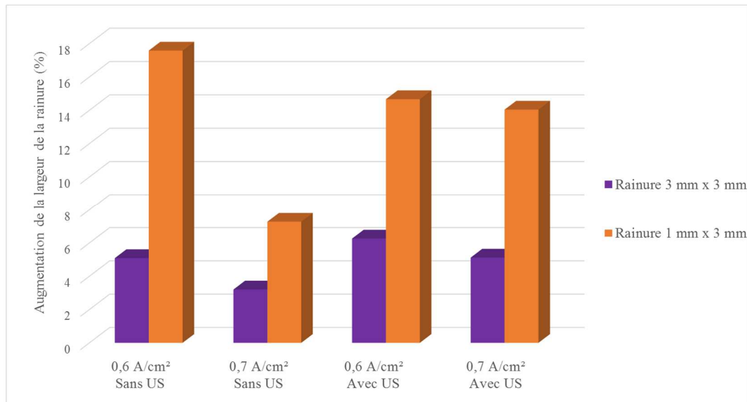
Figure 103 : Évolution des écarts dimensionnels au niveau de la largeur des rainures de 1 x 3 mm et 3 x 3 mm entre la pièce de référence et les pièces électropolies avec et sans agitation ultrasonore pour deux densités de courant
