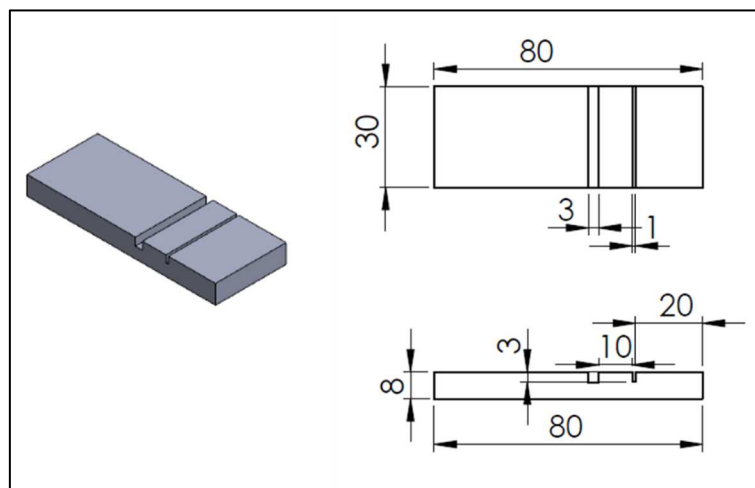
Figure 98 : Plan et cotes des plaques rainurées (en mm)
