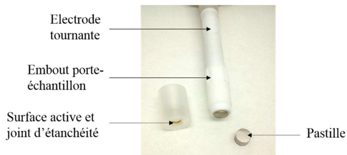
Figure 24 : Porte-échantillon utilisé lors de cette étude
