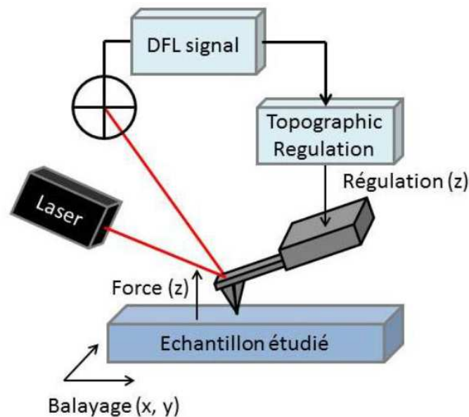
Figure 156 : Principe de fonctionnement d'un AFM. La force appliquée sur le levier est traduite en signal électrique par la mesure de la déflexion sur une photodiode quatre quadrants, cela permet de garder la distance entre la pointe et la surface constante et ainsi obtenir une cartographie de la surface [7]
