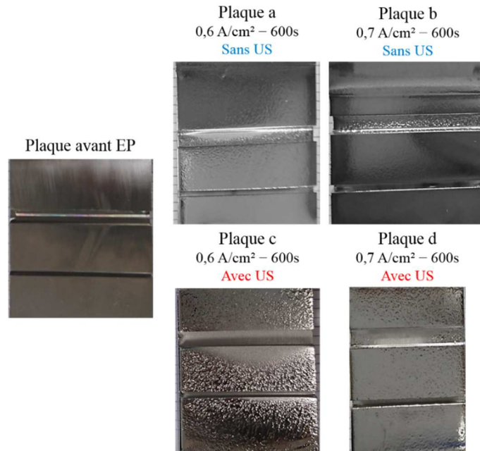
Figure 100 : Plaques rainurées avant et après électropolissage avec et sans ultrasons pour différentes densités de courant
