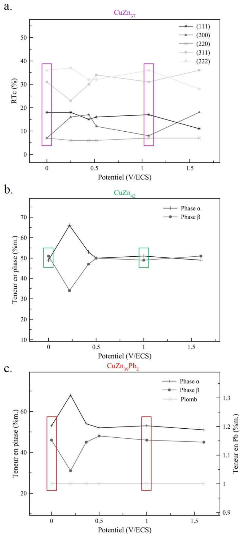
Figure 39 : Évolution des coefficients relatifs de texture pour chacun des plans cristallins pour les échantillons de \text{CuZn}_{37} (a) et évolution de la teneur des phases \alpha , \beta et la teneur en Pb pour les échantillons de \text{CuZn}_{42} (b) et \text{CuZn}_{39}\text{Pb}_2 (c) avant et après électropolissage
