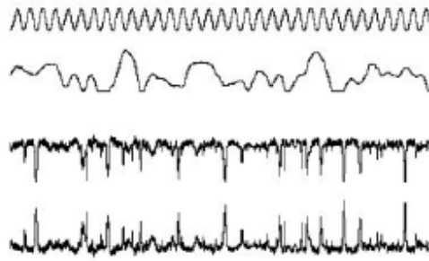
Figure 154 : Schéma de quatre profils possédant la même valeur de Ra [4]
