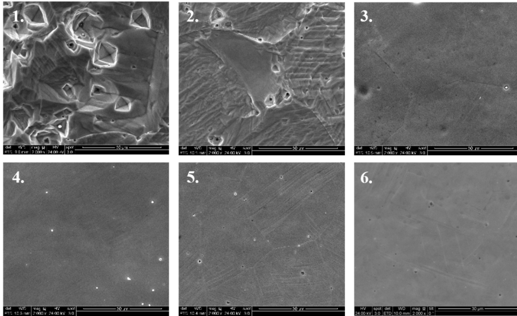
Figure 121 : Évolution de la morphologie de surface pour l'acier inoxydable 316L de fonderie électropoli à différents potentiel en milieu ChCl-EG à 70°C et 500 rpm
