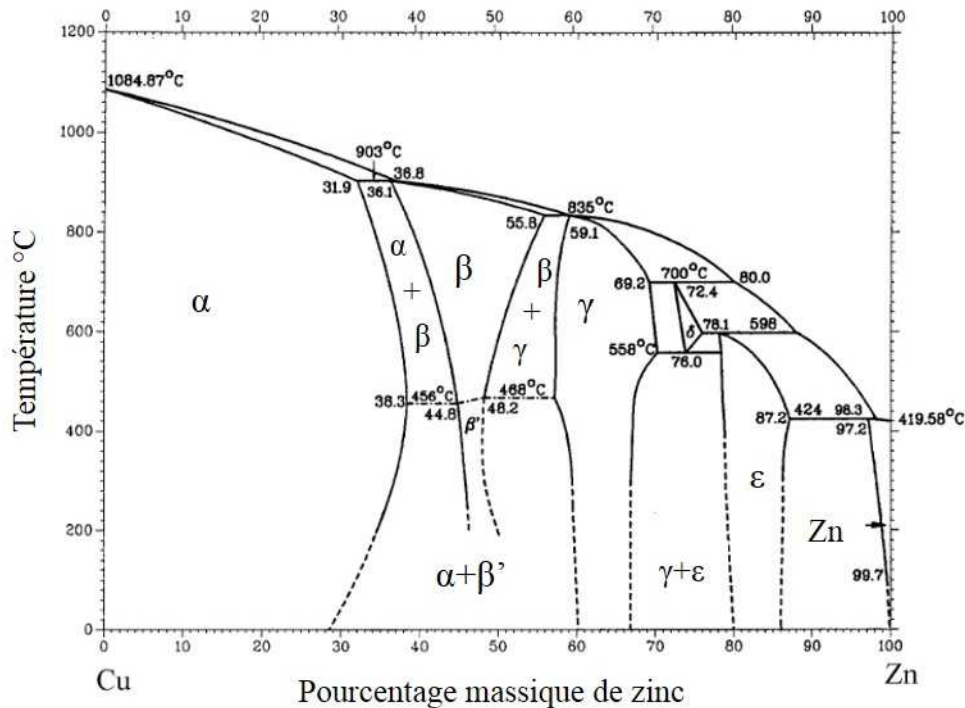
Figure 17 : Diagramme de phase du Cu-Zn
