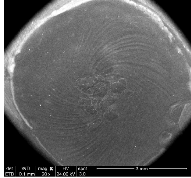
Figure 120 : Image MEB au grossissement x 20 d'un vortex observé après électropolissage en milieu DES à 70°C et 500 rpm
