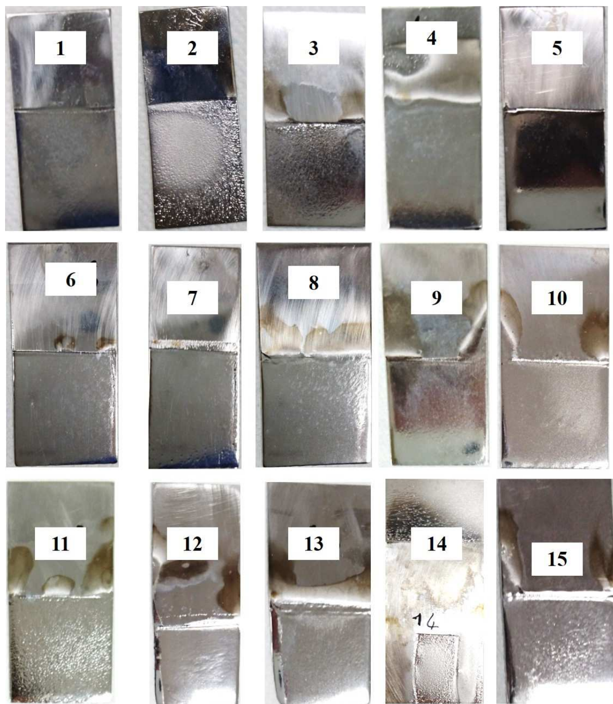
Figure 157 : Aspect visuel des plaques d'acier inoxydable 316L de fonderie après électropolissage dans les conditions présentées dans le Tableau 65, traitées dans le mélange acide phosphorique et acide sulfurique à 70°C sans ultrasons
