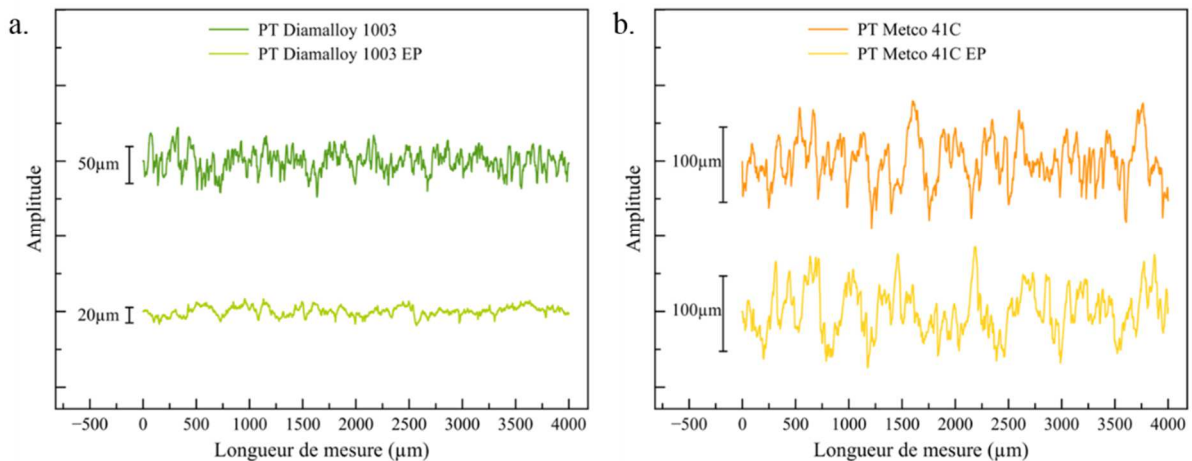
Figure 72 : Profils de la surface des échantillons issus de projection thermique avant et après électropolissage : (a) Diamalloy 1003 et (b) Metco 41C
