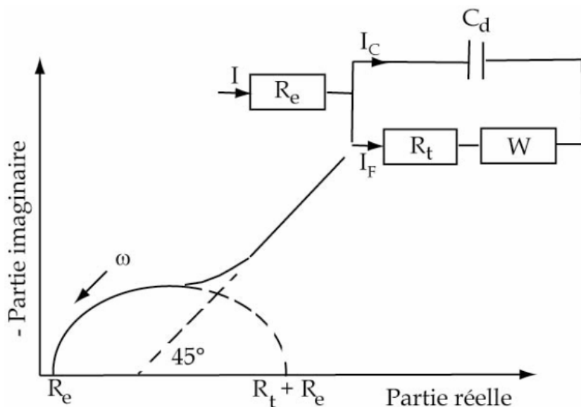
Figure 138 : Diagramme d'impédance électrochimique pour une cinétique mixte d'activation diffusion dans le cas d'une diffusion semi-infinie et circuit électrique équivalent de Randles
