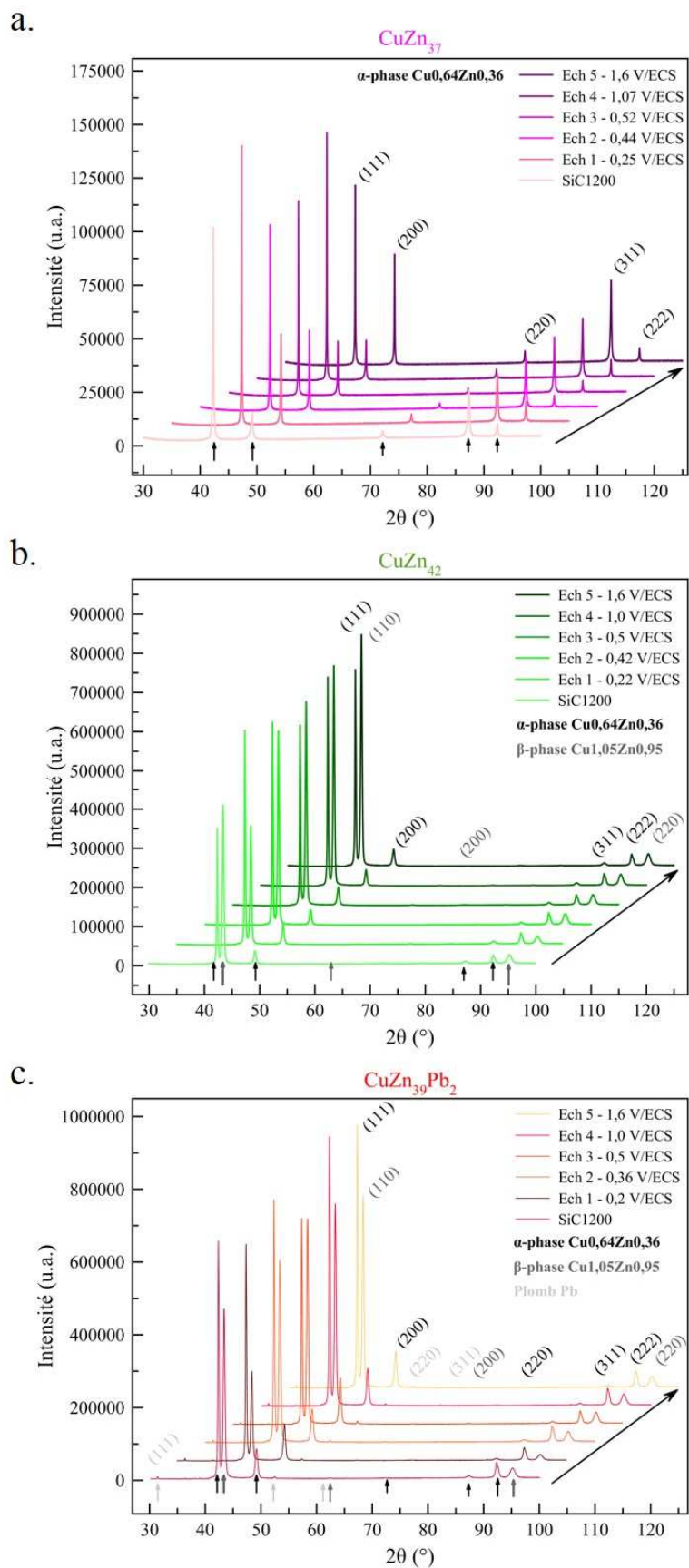
Figure 38 : Diffractogrammes des surfaces de laiton électropolies à 500 rpm et 25°C pour différents potentiels : (a) CuZn 37 , (b) CuZn 42 et (c) CuZn 39 Pb 2
