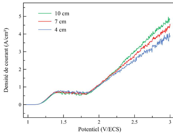
Figure 86 : Comportement anodique de l'acier inoxydable 316L en milieu acide phosphorique/acide sulfurique à 70°C dans la cellule pilote sous conditions silencieuses pour une distance électrode-transducteur entre 4 et 10 cm, pompe seule (2mV/s).
