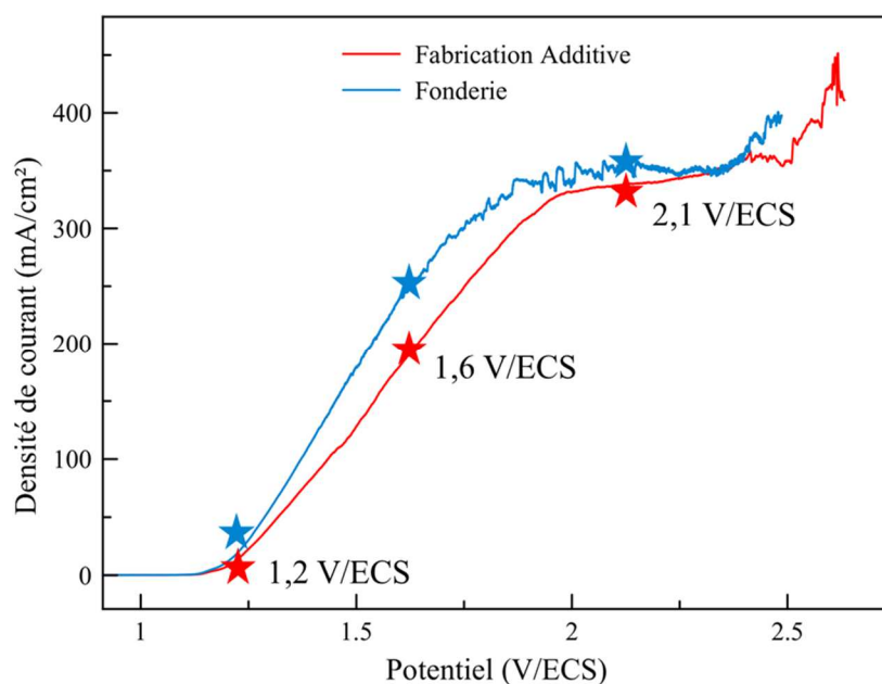
Figure 142 : Potentiels choisis pour les mesures d'impédance électrochimique à partir des courbes intensité-potentiel des aciers inoxydables 316L de fonderie (bleu) et de fabrication additive (rouge) en milieu phospho-sulfurique à 70°C et 500 rpm
