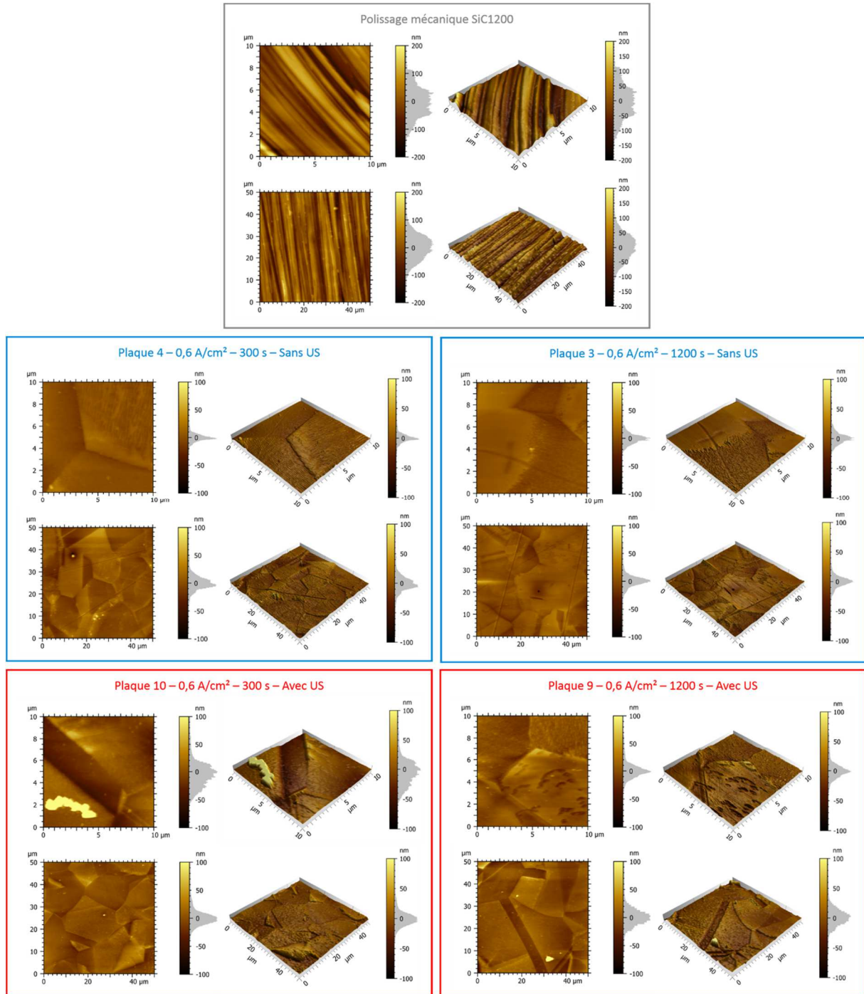
Figure 94 : Images AFM en 2D et 3D pour deux échelles, pour les plaques après polissage mécanique et après électropolissage avec et sans ultrasons (plaques 3, 4, 9 et 10)
