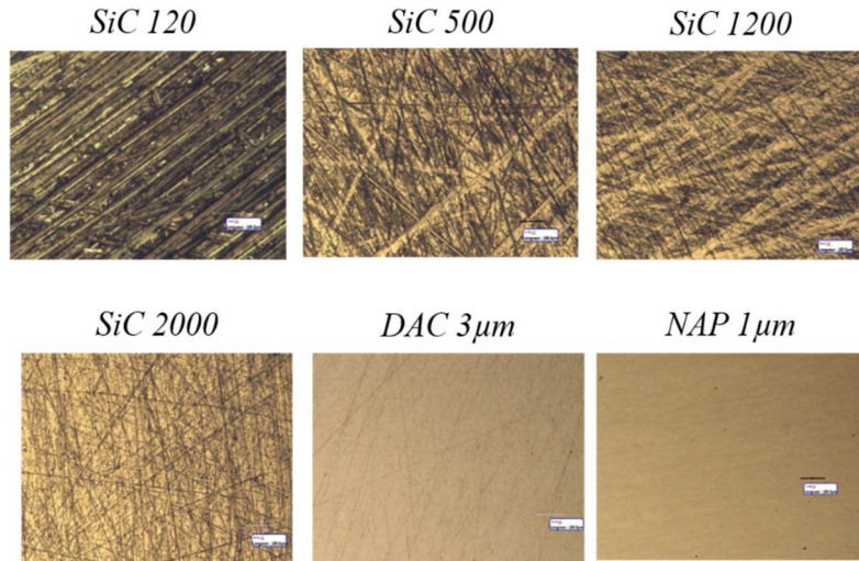
Figure 20 : Images en microscopie optique des échantillons polis mécaniquement avec différents draps de polissage
