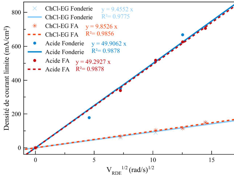
Figure 116 : Droite de Levich pour les aciers inoxydables 316L de fonderie et de fabrication additive en milieu ChCl-EG et en milieu acide à 70°C
