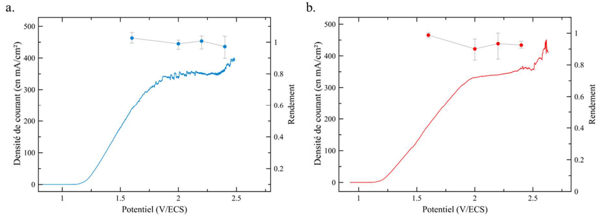
Figure 52 : Évolution du rendement de dissolution en fonction du potentiel pour les aciers inoxydables 316L issus de fonderie (a) et de fabrication additive (b).
