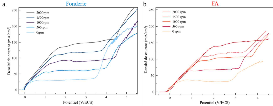
Figure 115 : Courbes de polarisation des aciers inoxydables 316L en milieu ChCl-EG à 70°C pour différentes vitesses de rotation de l'électrode tournante : (a) fonderie et (b) fabrication additive.
