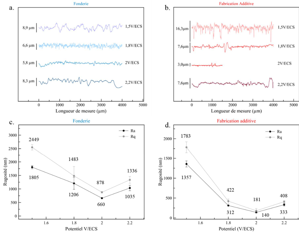
Figure 50 : Évolution de la rugosité de surface après électropolissage des aciers inoxydables 316L en milieu acide à 35°C
