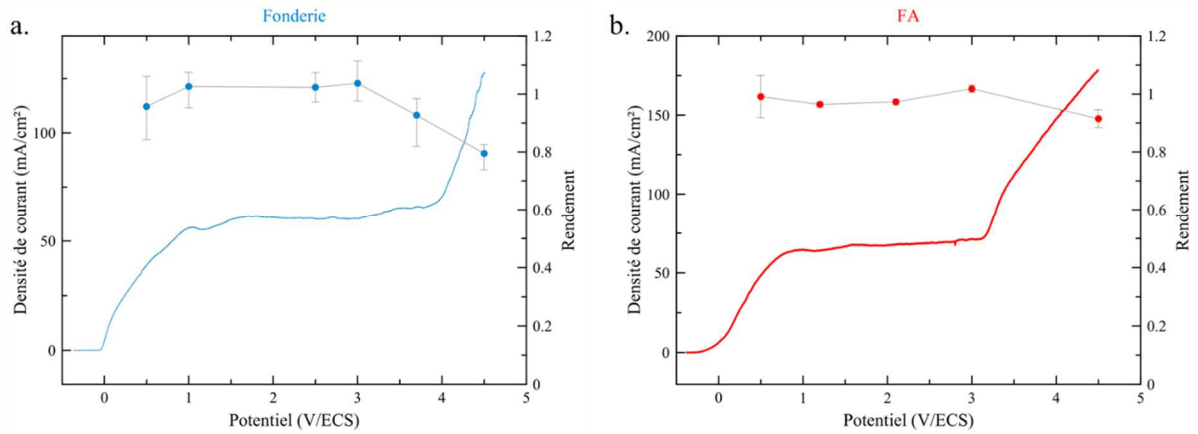
Figure 117 : Évolution du rendement de dissolution en fonction du potentiel lors de l'électropolissage en milieu ChCl-EG à 70°C et 500 rpm : (a) acier inoxydable 316L de fonderie et (b) acier inoxydable 316L de fabrication additive.
