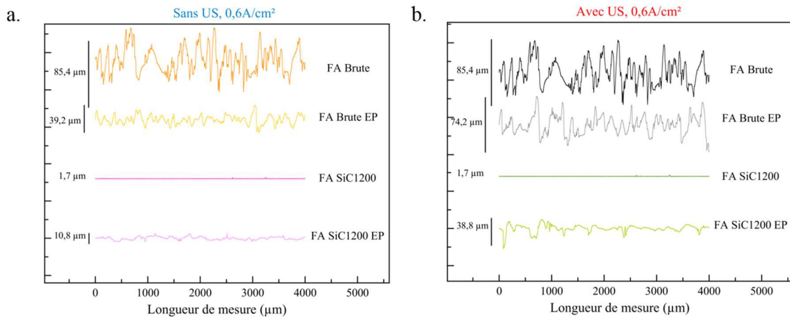
Figure 97 : Évolution des profils de rugosité des plaques de fabrication additive électropolies en milieu acide à 70^{\circ}\text{C} avec et sans ultrasons pour un temps de 10 minutes
