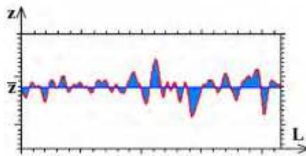
Figure 153 : Représentation schématique du calcul des paramètres conventionnels de rugosité R_a ou R_q d'un profil donné [3]
