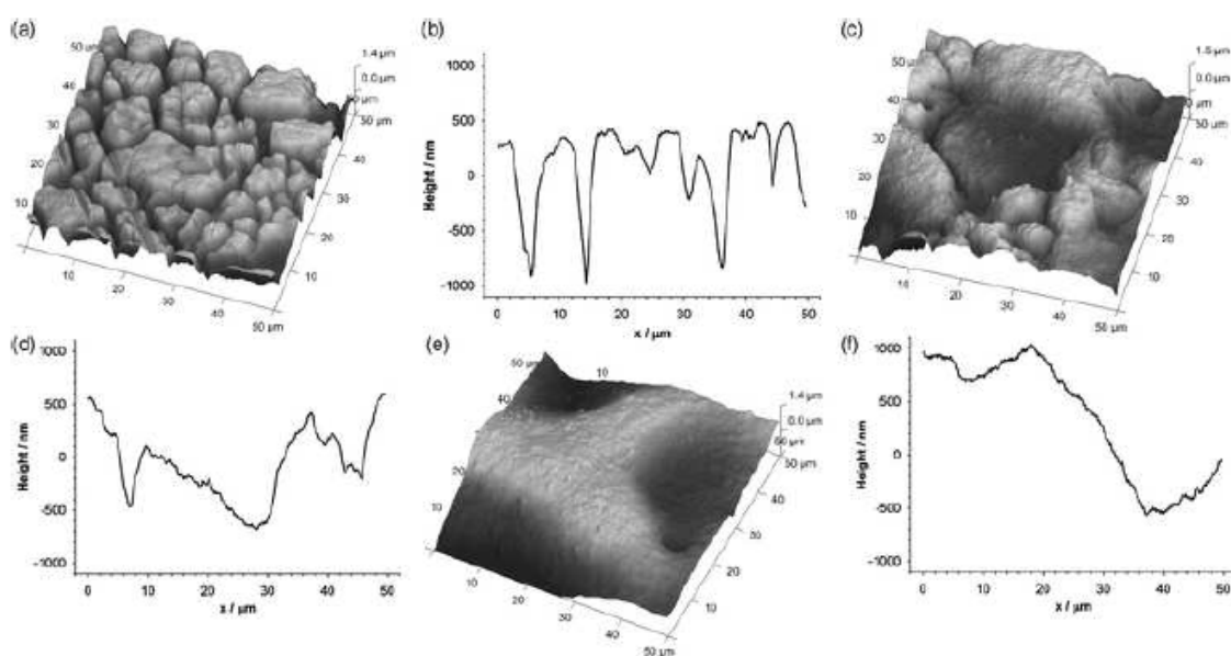
Figure 112 : Images et profils AFM obtenus au cours de l'électropolissage à une densité de courant de 25 mA/cm 2 , (a) (b) surface brute, (c) (d) surface électropolie pendant 10 min et (e) (f) surface électropolie après 25 min [72]
