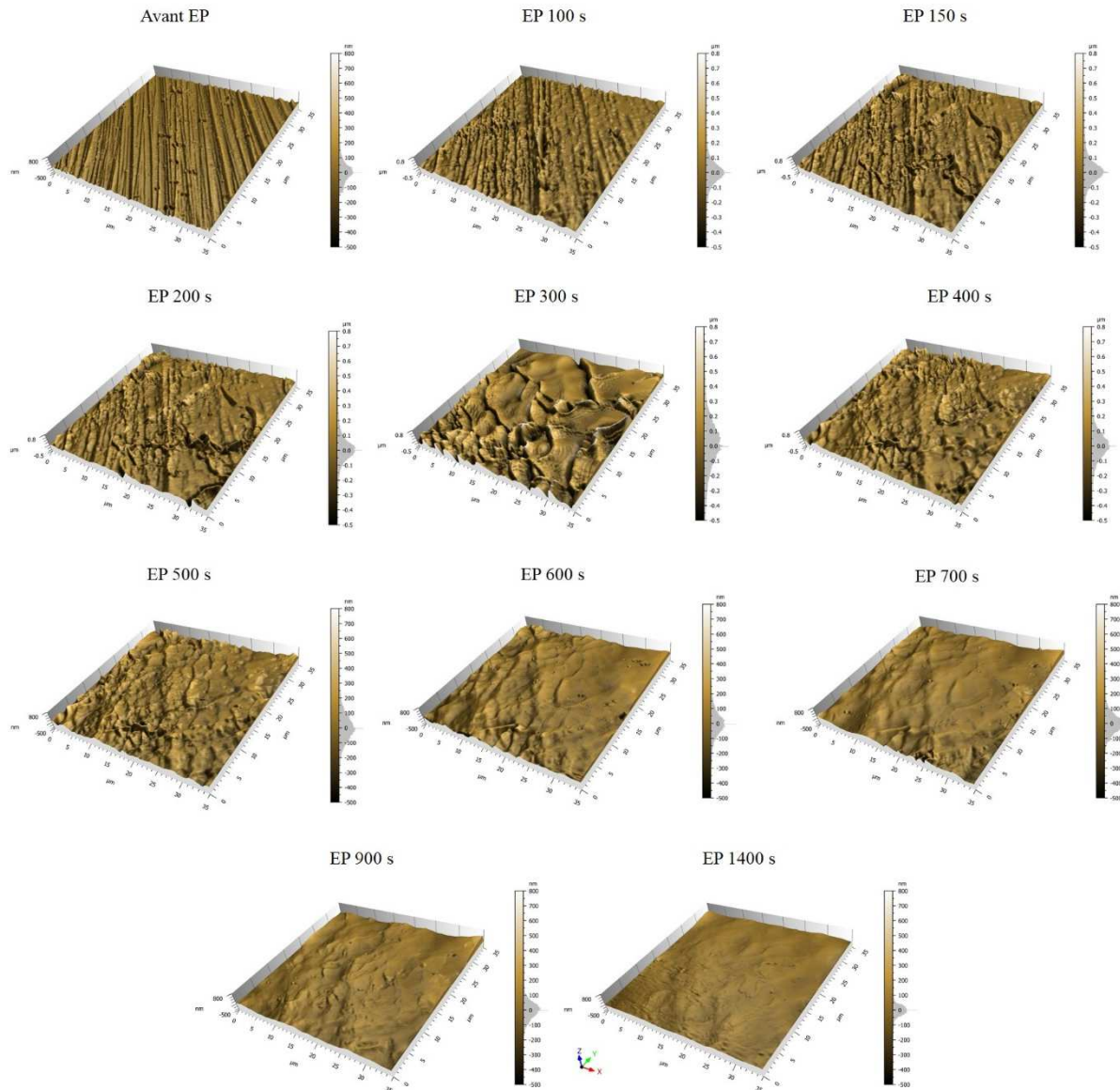
Figure 130 : Images AFM in situ de la surface d'acier inoxydable 316L lors de l'électropolissage
