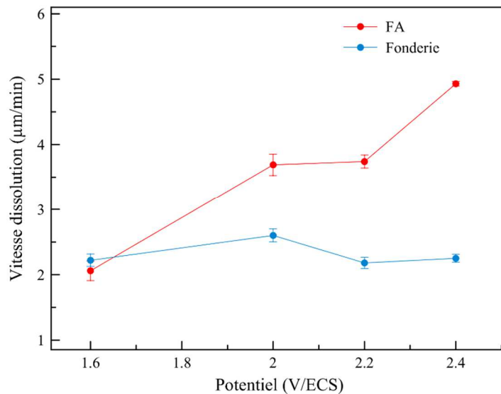
Figure 53 : Évolution des vitesses de dissolution des aciers inoxydables 316L de fonderie et de fabrication additive en milieu acide en fonction du potentiel d'électropolissage
