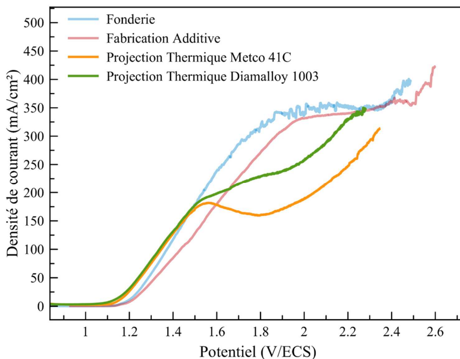
Figure 70 : Courbes de polarisation des échantillons issus de projection thermique en milieu acide à 70°C et 500 rpm ( V_b=2\text{mV/s} )
