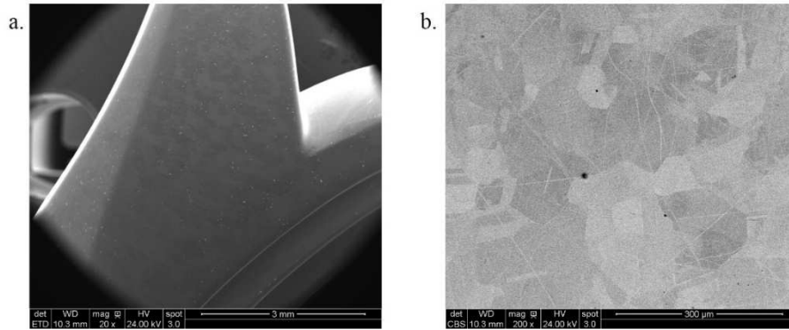
Figure 106 : Images MEB de la carrure électropolie à 0,6 A/cm 2 pendant 2 minutes : (a) grossissement x 20 en électrons secondaires et (b) grossissement x 200 en électrons rétrodiffusés
