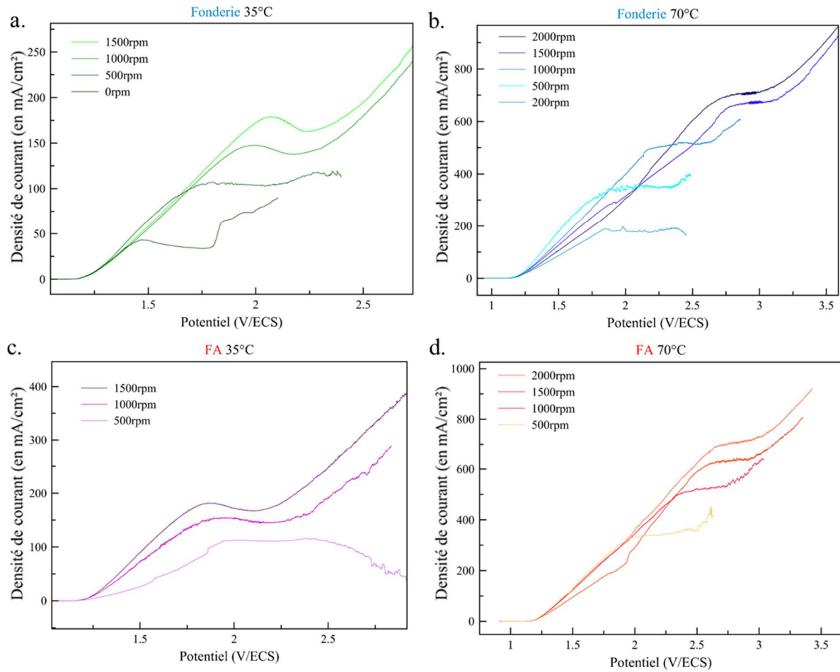
Figure 46 : Courbes de polarisation des échantillons des aciers inoxydables 316L dans un mélange d'acide phosphorique et d'acide sulfurique pour deux températures : fonderie (a) 35°C, (b) 70°C et fabrication additive (c) 35°C, (d) 70°C.
