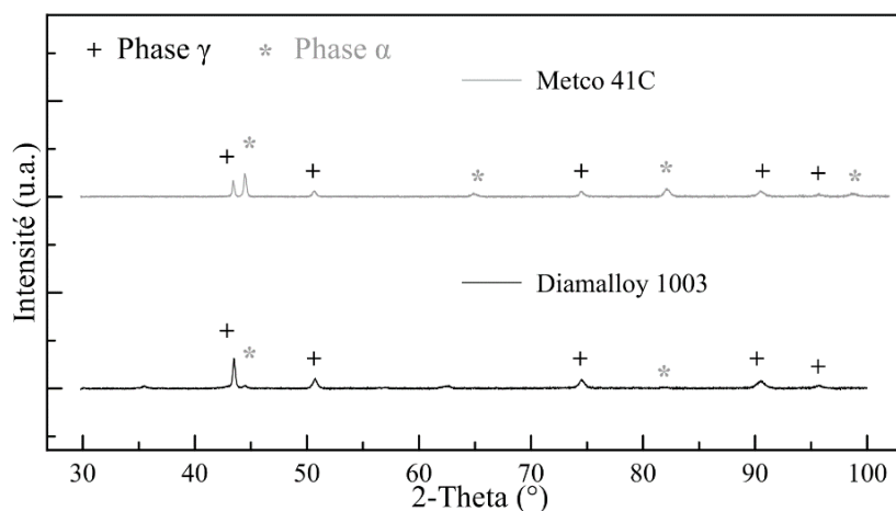
Figure 69 : Diffractogrammes des échantillons issus de projection thermique avant électropolissage
