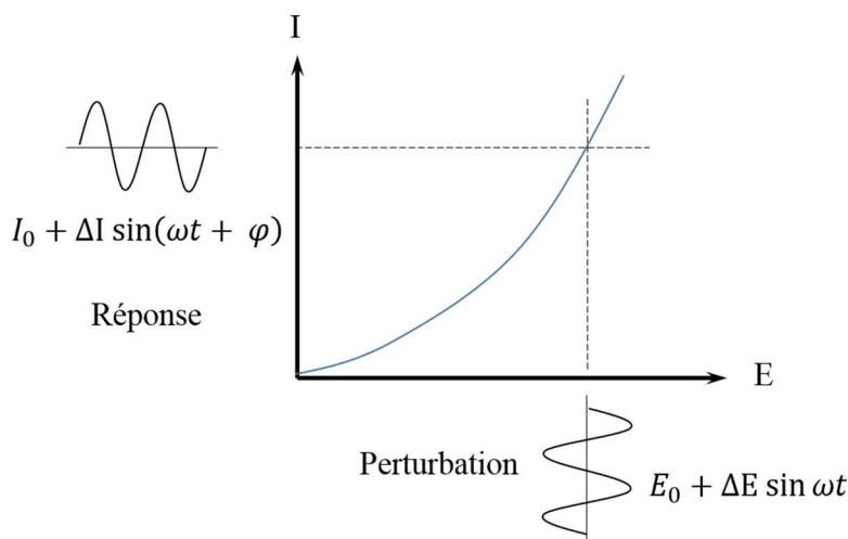
Figure 135 : Principe de la SIE : perturbation en potentiel et réponse en courant
