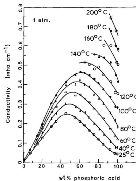
Figure 22 : Évolution de la conductivité en fonction de la concentration en acide phosphorique pour différentes températures [28]
