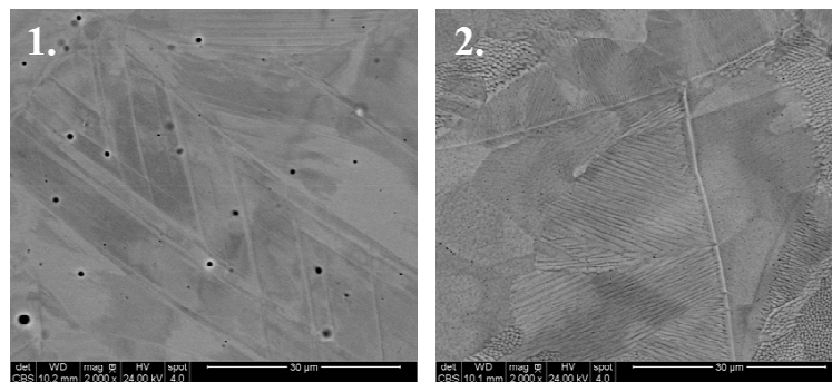
Figure 55 : Images MEB en électrons rétrodiffusés pour les aciers inoxydables 316L électropolis à 2,4 V/ECS pendant 20 minutes : (1) fonderie et (2) fabrication additive
