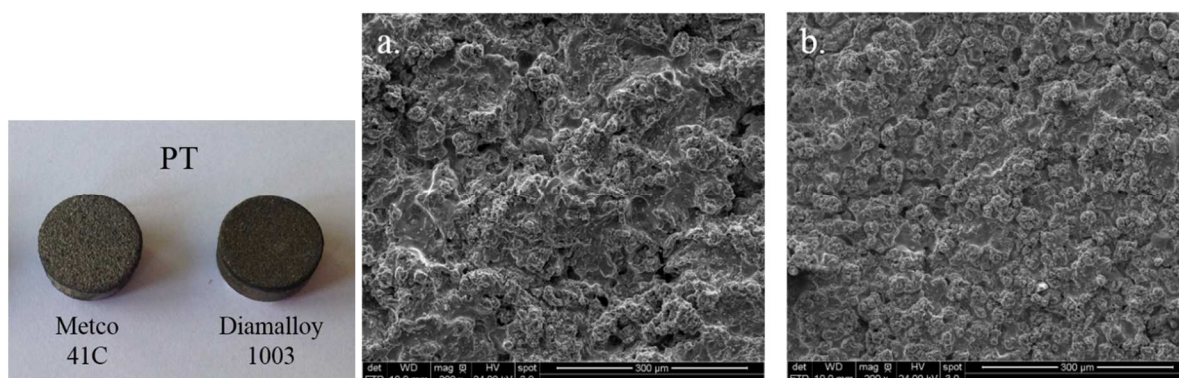
Figure 67 : Échantillons d'aciers inoxydables 316L issus de projection thermique et images MEB de leur surface (a) Metco 41C et (b) Diamalloy 1003
