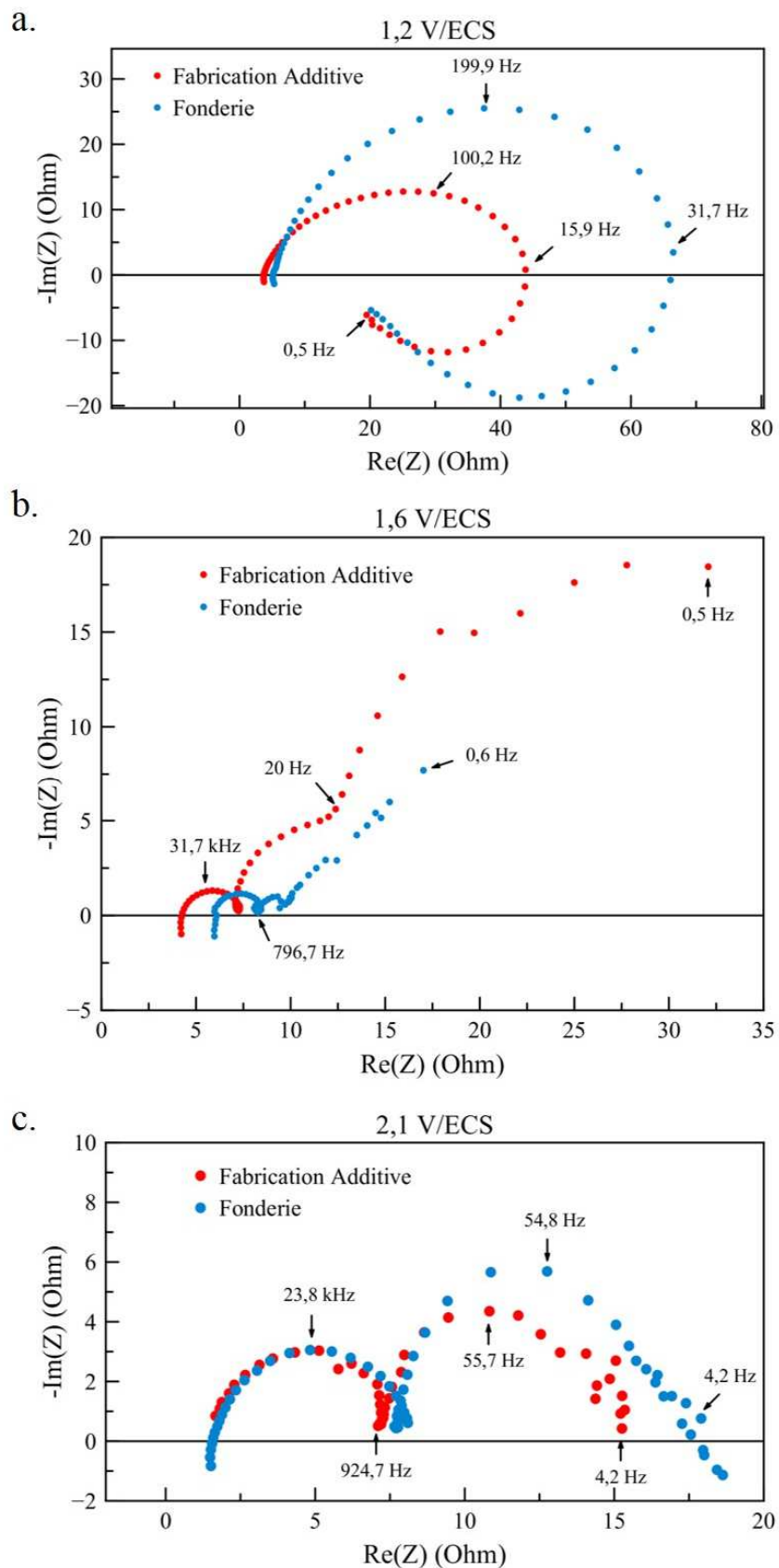
Figure 143 : Représentation de Nyquist des diagrammes d'impédance des aciers inoxydables 316L de fonderie (bleu) et de fabrication additive (rouge) électropolis dans un mélange d'acide phosphorique et sulfurique à 70°C et 500 rpm à différents potentiels : (a) 1,2 V/ECS, (b) 1,6 V/ECS et (c) 2,1 V/ECS
