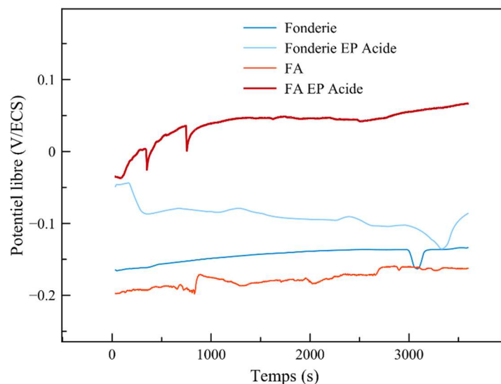
Figure 60 : Évolution du potentiel libre (potentiel de corrosion spontané) en milieu NaCl à 25°C des aciers inoxydables 316L de fonderie et de fabrication additive avant et après électropolissage en milieu acide à 70°C.
