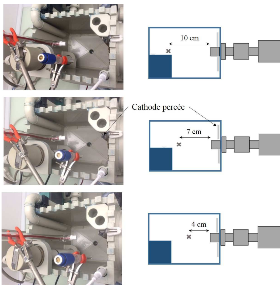
Figure 84 : Les différentes positions de l'électrode de travail pour les mesures de transfert de matière : Position 1 (10 cm), Position 2 (7 cm) et Position 3 (4 cm)
