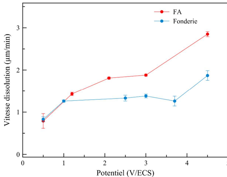
Figure 118 : Évolution de la vitesse de dissolution des aciers inoxydables 316L en milieu DES à 70°C en fonction du potentiel appliqué
