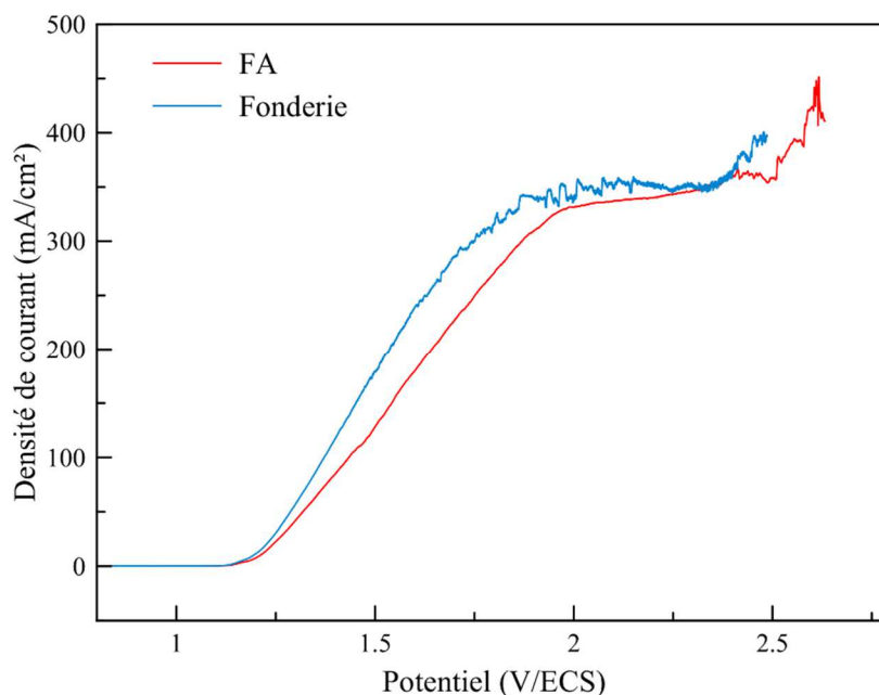
Figure 45 : Courbes intensité-potentiel du phénomène d'électropolissage pour les aciers inoxydables 316L issus de deux procédés de fabrication dans une solution acide à 70°C
