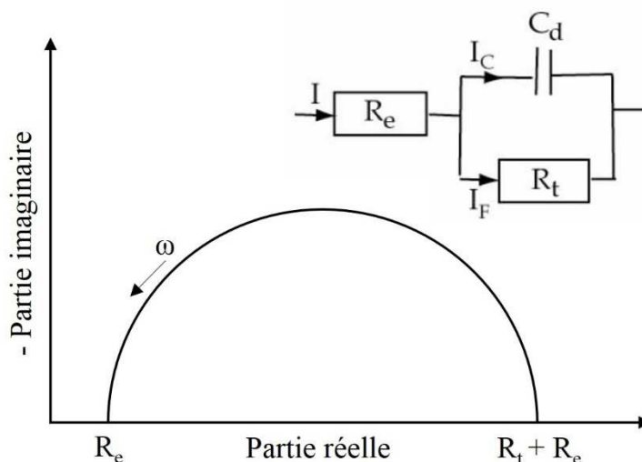
Figure 137 : Représentation de Nyquist de l'impédance électrochimique dans le cas d'un processus de transfert de charge et circuit équivalent
