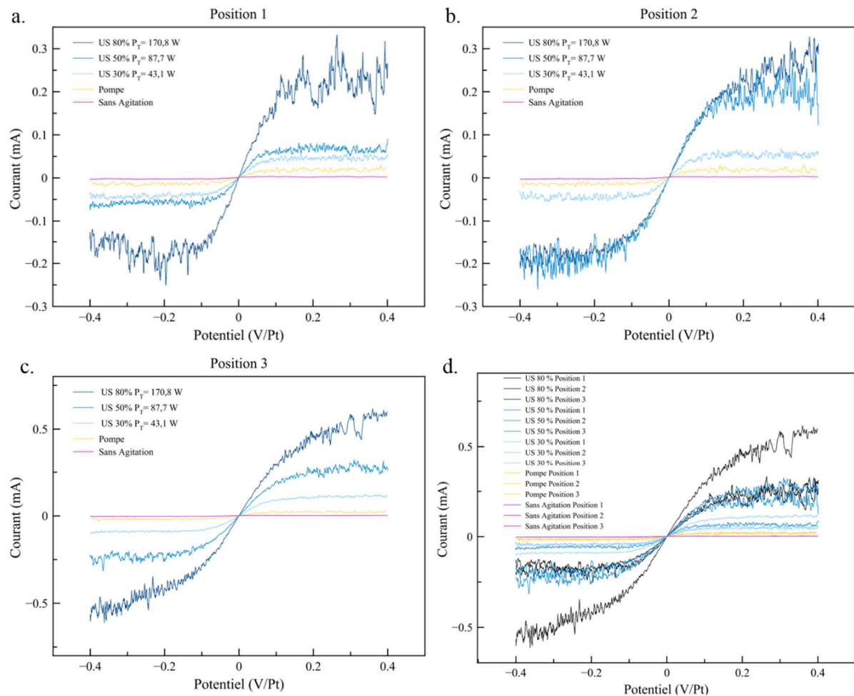
Figure 85 : Transfert de matière dans la cuve pilote pour les différentes conditions hydrodynamiques (a) Position 1 - 10 cm, (b) Position 2 - 7 cm, (c) Position 3 - 4 cm et (d) vue complète des résultats
