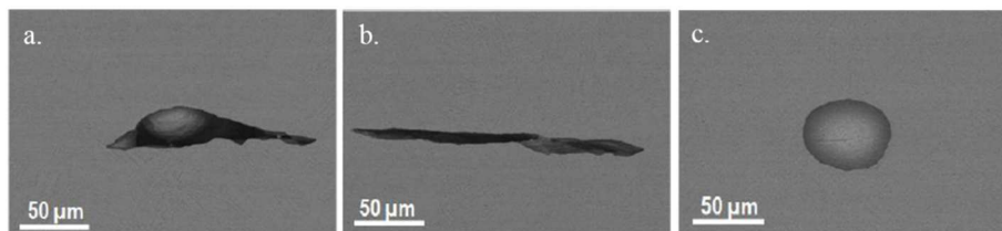
Figure 6 : Exemples de défauts rencontrés sur les pièces issues de Selective Laser Melting : (a) et (b) porosités induites par un manque de fusion entre deux couches de poudre et (c) gaz piégé [22].
