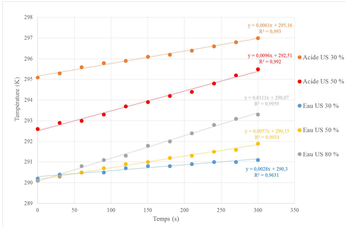
Figure 80 : Courbes de calorimétrie pour différentes amplitudes pour le transducteur à 20 kHz dans l'eau et dans le mélange d'acides
