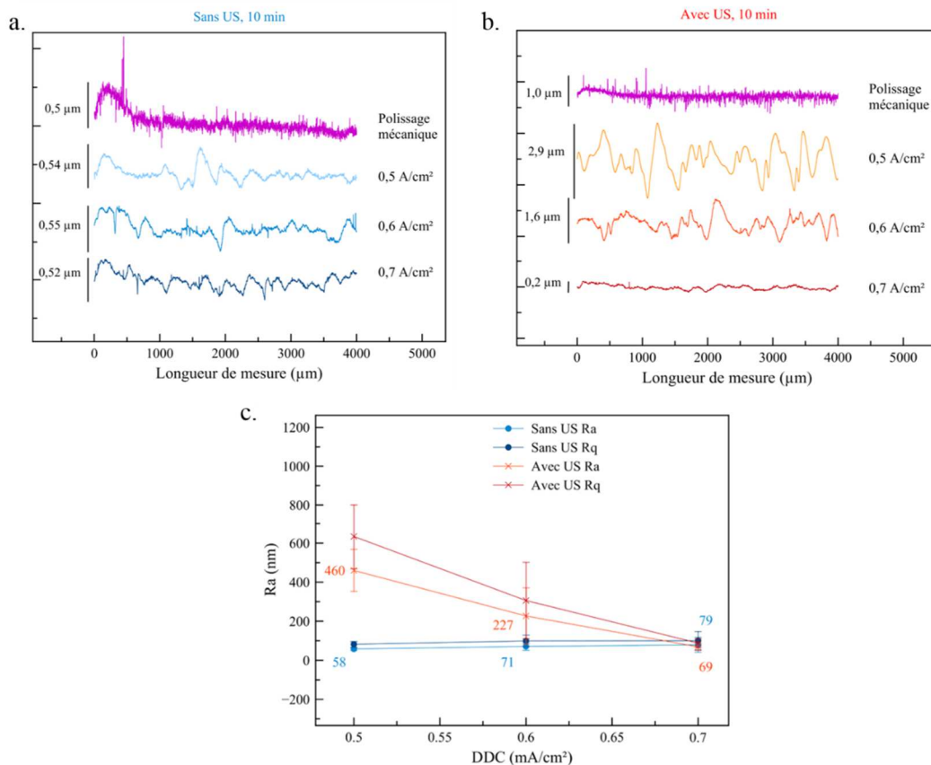
Figure 92 : Évolution de la rugosité de surface obtenue par profilométrie mécanique pour les échantillons d'acier inoxydables électropolés avec et sans ultrasons pendant 10 minutes et pour différentes densités de courant : (a) profils de surface sous conditions silencieuses, (b) profils de surface sous ultrasons et (c) évolution des paramètres de rugosité en fonction de la densité de courant
