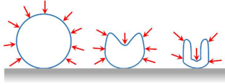
Figure 78 : Schéma de l'implosion d'une bulle de cavitation au voisinage d'une surface
