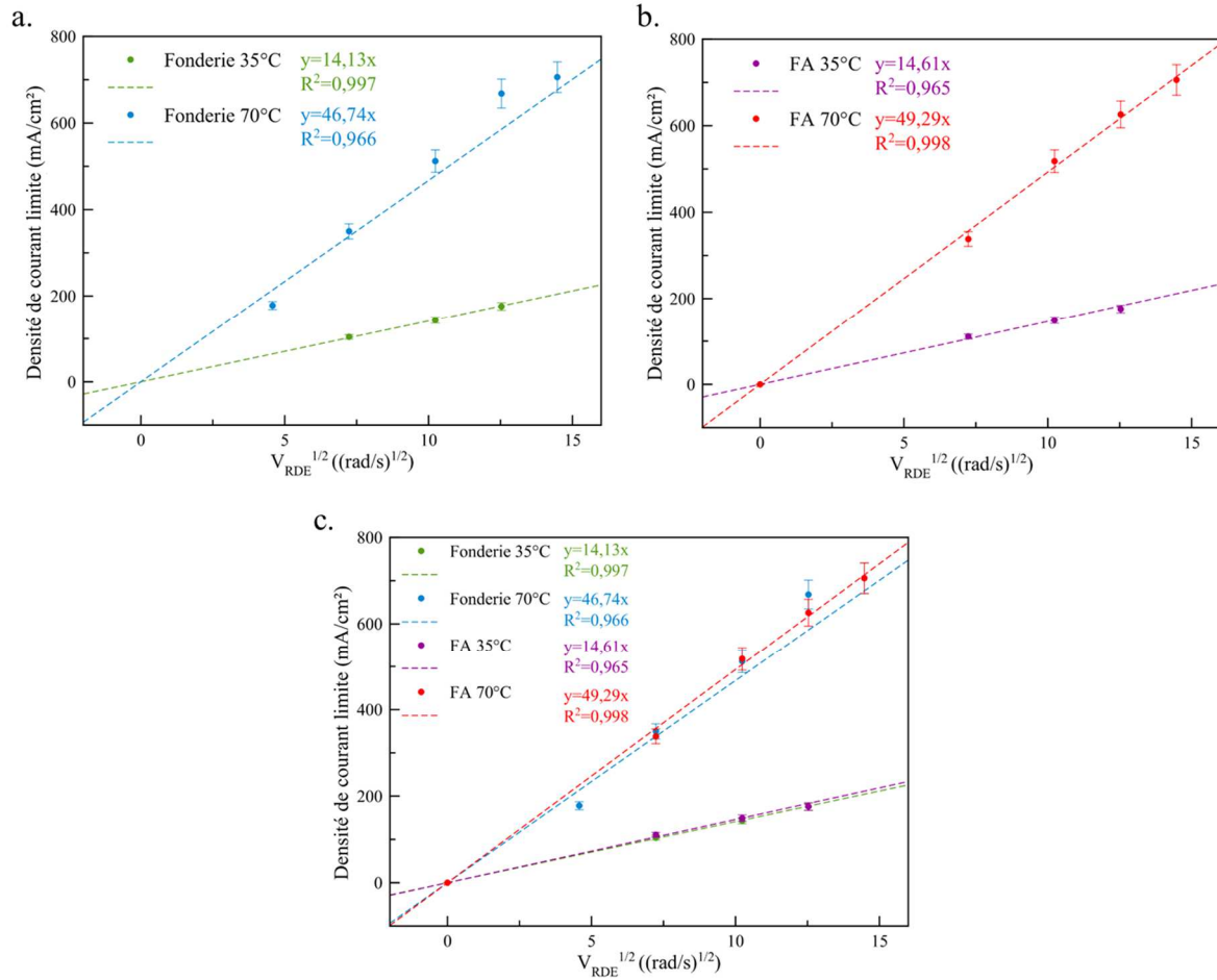
Figure 47 : Évolution des droites de Levich pour les aciers inoxydables à différentes températures : (a) fonderie, (b) fabrication additive et (c) comparaison des deux types de matériaux
