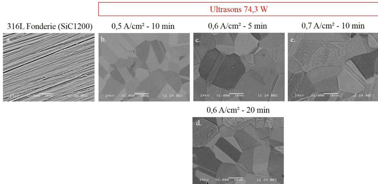
Figure 91 : Morphologie des échantillons électropolis avec ultrasons (20 kHz et 74,3 W) en milieu acide à 70°C pour différentes densités de courant et différents temps : (a) avant électropolissage, (b) plaque 1, (c) plaque 10, (d) plaque 9 et (e) plaque 12.
