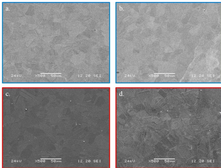
Figure 89 : Images MEB en mode électrons secondaires des plaques électropolies avec (rouge) et sans ultrasons (bleu) : (a) plaque 4, (b) plaque 3, (c) plaque 10 et (d) plaque 9.
