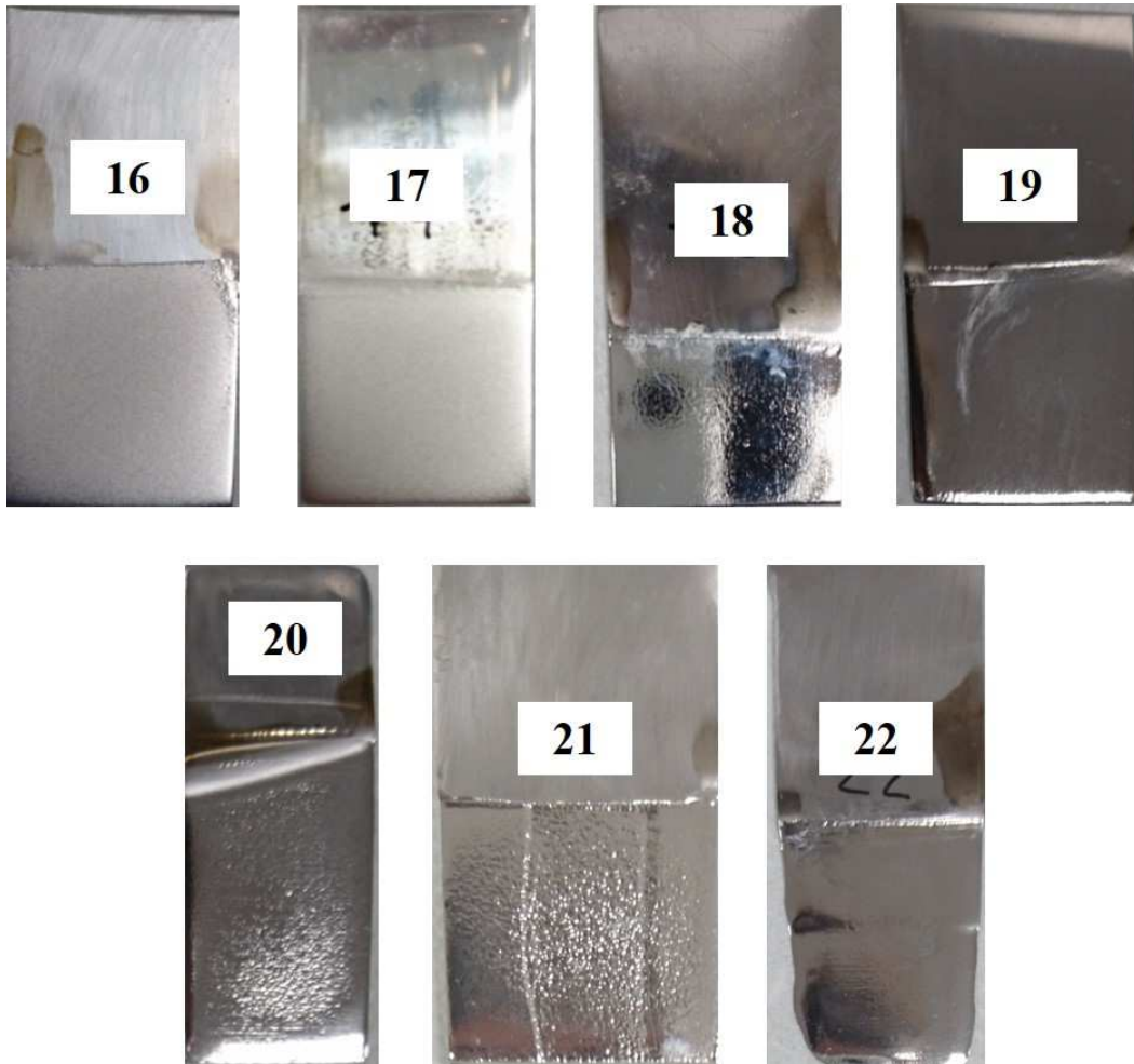
Figure 158 : Aspect visuel des plaques d'acier inoxydable 316L de fonderie après électropolissage dans les conditions présentées dans le Tableau 65, traitées dans le mélange acide phosphorique et acide sulfurique à 70°C avec ultrasons
