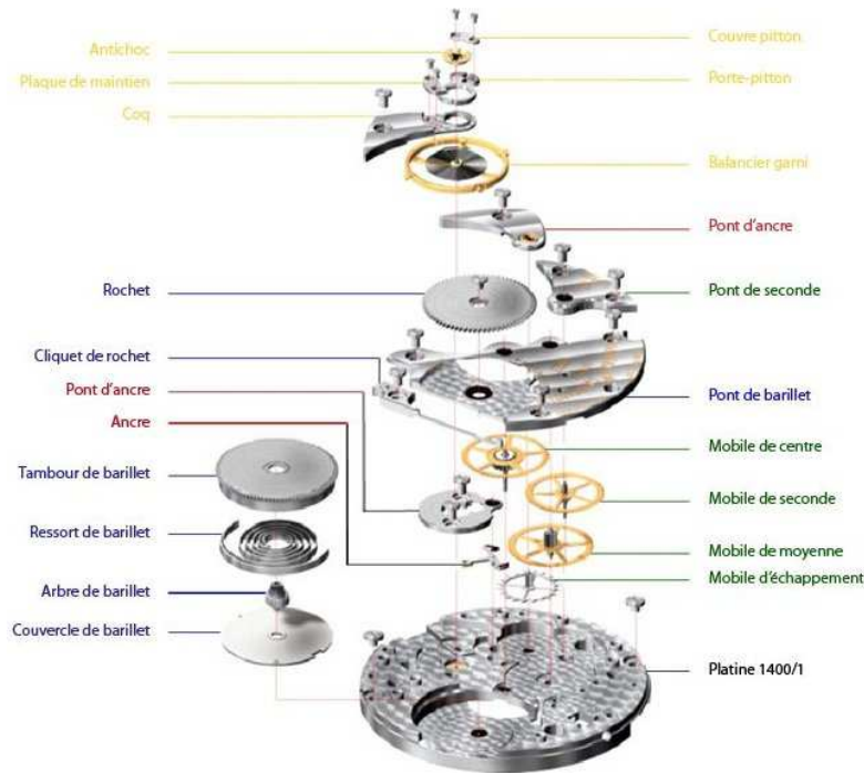
Figure 1 : Schéma d'une montre mécanique (vue éclatée)
