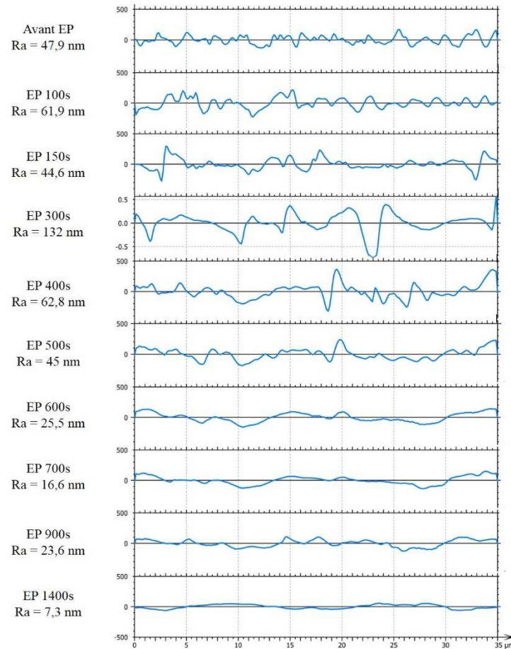
Figure 131 : Profils de rugosité 2D obtenus à partir des images AFM in-situ présentées dans la Figure 130
