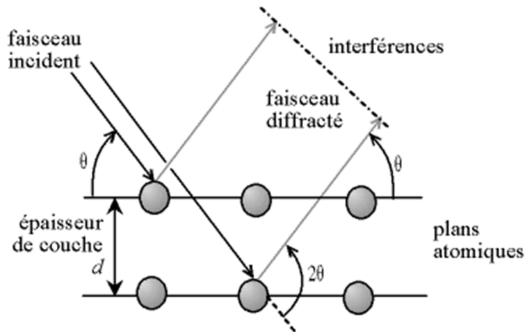
Figure 150 : Schéma du phénomène de diffraction des rayons X, avec \theta l'angle de Bragg
