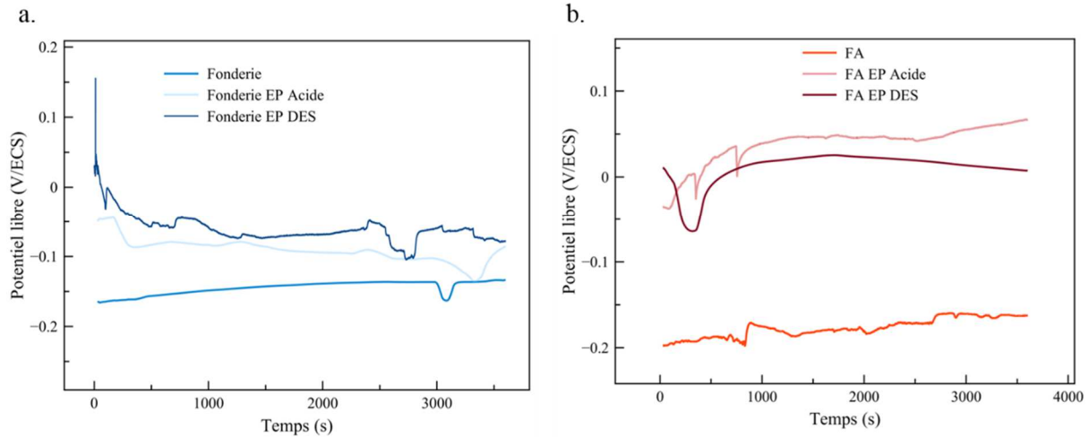
Figure 125 : Suivi du potentiel libre en milieu NaCl à 25°C des aciers inoxydables 316L avant et après électropolissage en milieu DES : (a) fonderie et (b) fabrication additive
