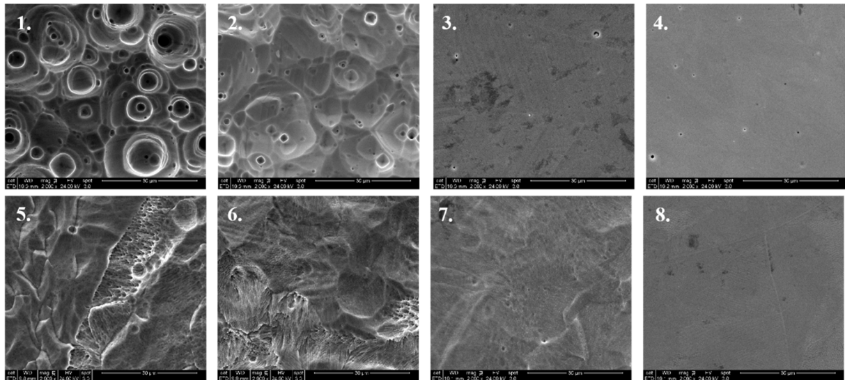
Figure 54 : Images MEB (électrons secondaires) des échantillons d'acier inoxydable électropolis à différents potentiels (1,6 ; 2 ; 2,2 et 2,4 V/ECS) en milieu acide à 70°C et 500 rpm : (1) à (4) fonderie et (5) à (8) fabrication additive
