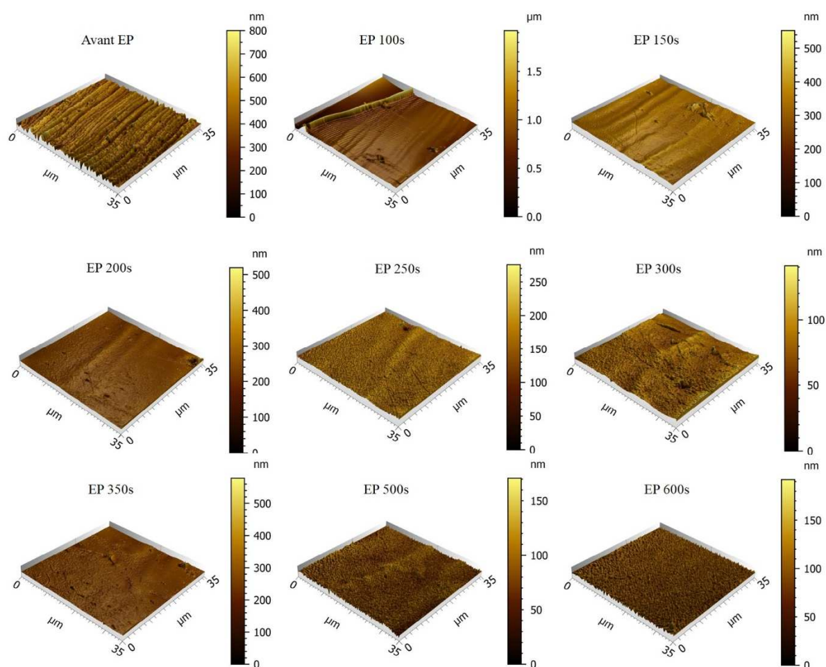
Figure 159 : Évolution au cours du temps des images obtenues par microscopie AFM in situ de la surface d'acier inoxydable 316L de fonderie lors de l'électropolissage en milieu DES ( \text{ChCl-EG} ) à 35^\circ\text{C}
