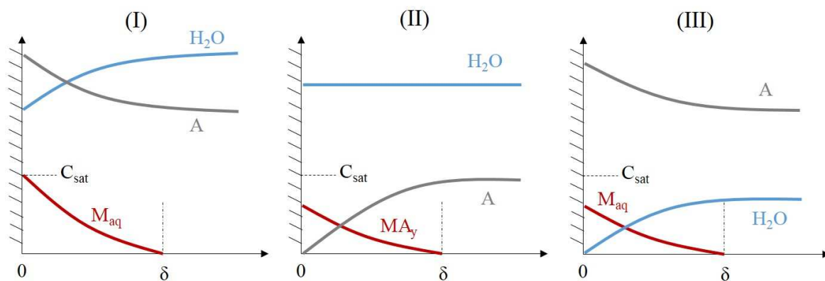
Figure 16 : Représentation schématisée des mécanismes pouvant être impliqués lors de l'électropolissage selon Landolt [92] ou M_{aq} : représente les cations métalliques issus de la dissolution, A est une espèce acceptrice, et MA_y est un complexe contenant le cation métallique.
