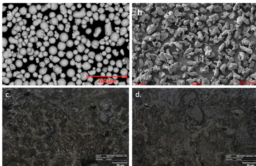
Figure 68 : Images MEB des particules de poudre utilisées en projection thermique (a) Diamalloy 1003 et (b) Metco 41C [84] et microstructure des dépôts après attaque chimique (c) Diamalloy 1003 et (d) Metco 41C
