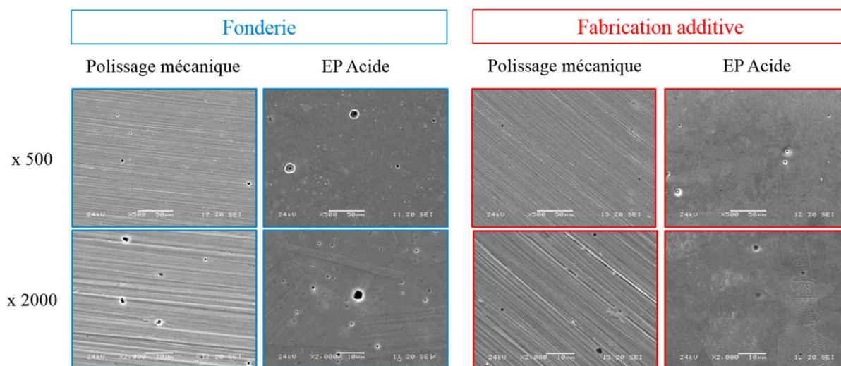
Figure 63 : Pastilles d'aciers inoxydables 316L de fonderie et de fabrication additive avant et après électropolissage, après 1 heure à 100 \mu\text{A}/\text{cm}^2 dans NaCl 3 %
