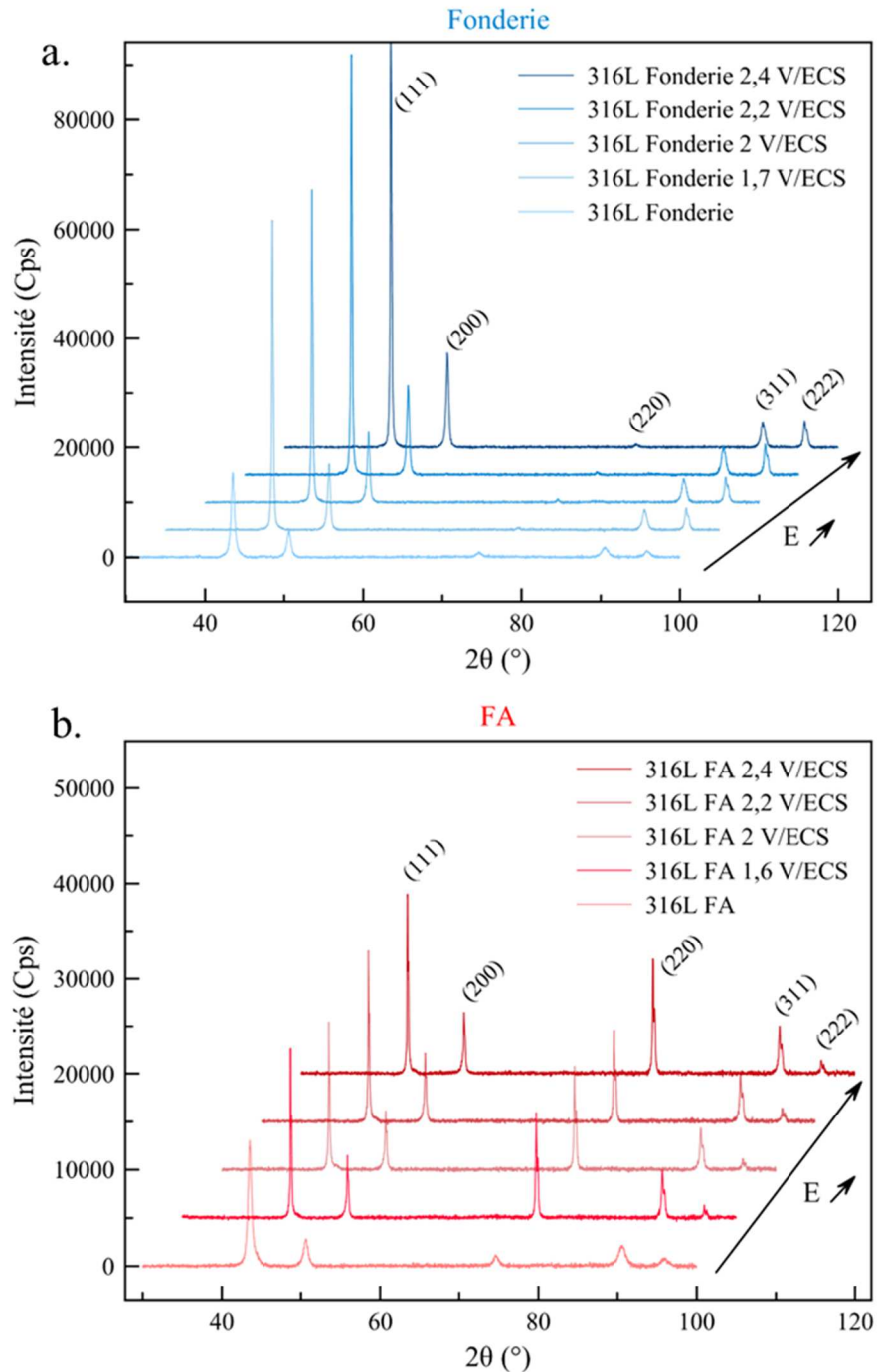
Figure 58 : Évolution des diffractogrammes pour les surfaces d'aciers inoxydables électropolis à différents potentiels en milieu acide à 70°C et 500 rpm : (a), fonderie et (b) fabrication additive
