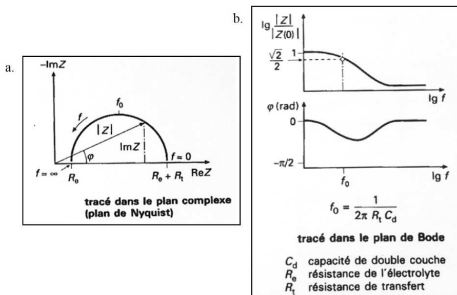
Figure 136 : Représentations graphiques de la fonction de transfert [3]
