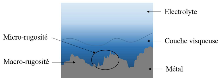
Figure 15 : Représentation schématique des macro et micro-rugosités
