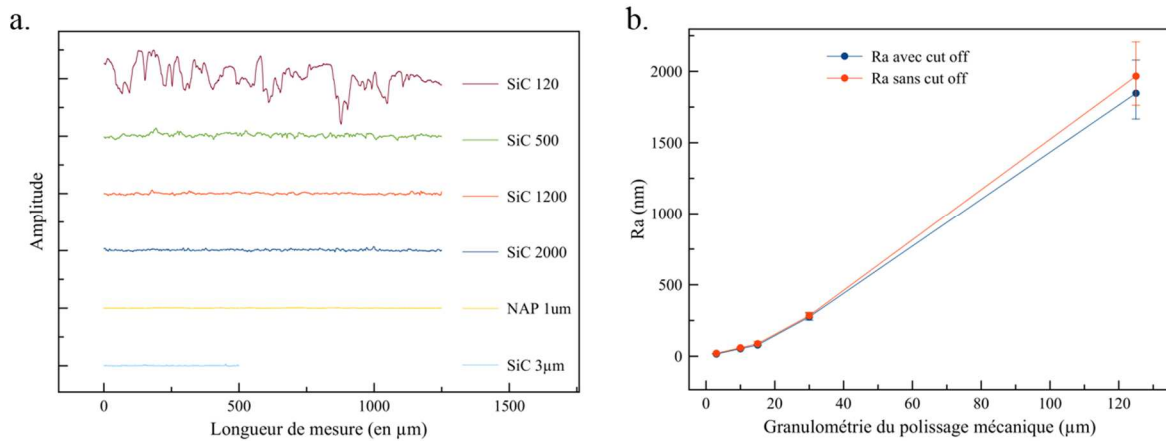
Figure 21 : Profils de rugosité des échantillons polis mécaniquement (a) et évolution du Ra en fonction de la granulométrie utilisée pour le polissage et de l'application d'un "cut off" choisi selon la norme NF EN ISO 4288 :1998 (b)
