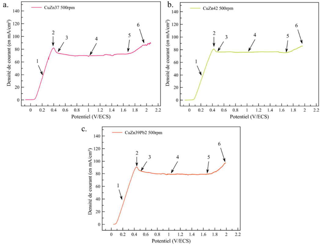
Figure 29 : Voltampérogrammes anodiques des alliages CuZn 37 (a), CuZn 42 (b) et CuZn 39 Pb 2 (c) à 25°C dans l'acide phosphorique 58 %. V_b = 2 \text{ mV/s} , \omega = 500 \text{ rpm}
