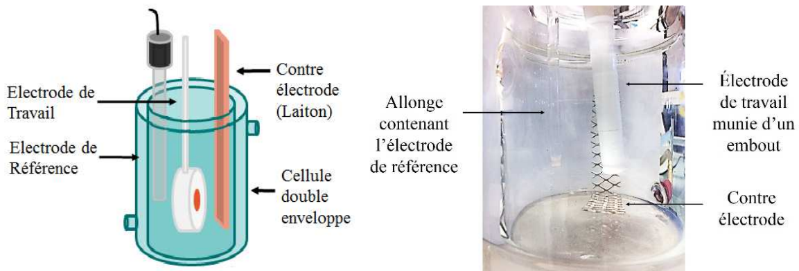
Figure 23 : Schéma et photo de la cellule électrochimique
