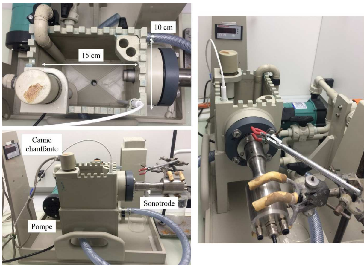
Figure 79 : Cuve pilote avec le transducteur basse fréquence
