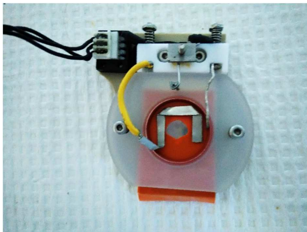
Figure 133 : Nouvelle contre électrode pour la cellule électrochimique d'AFM in situ
