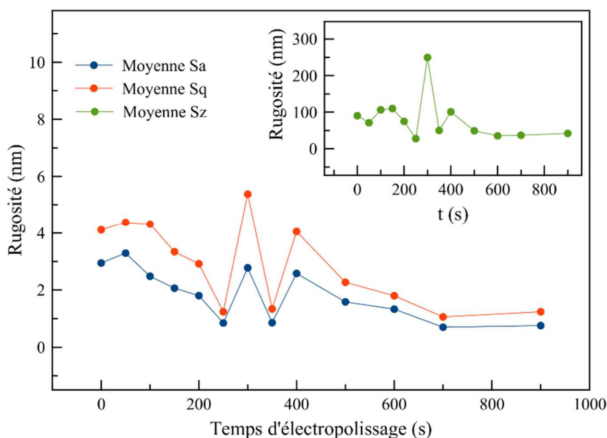
Figure 132 : Évolution de la rugosité (mesures sur la surface en 3D) de surface en fonction du temps d'électropolissage
