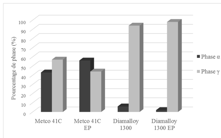
Figure 73 : Évolution du pourcentage de phase des échantillons de projection thermique avant et après électropolissage
