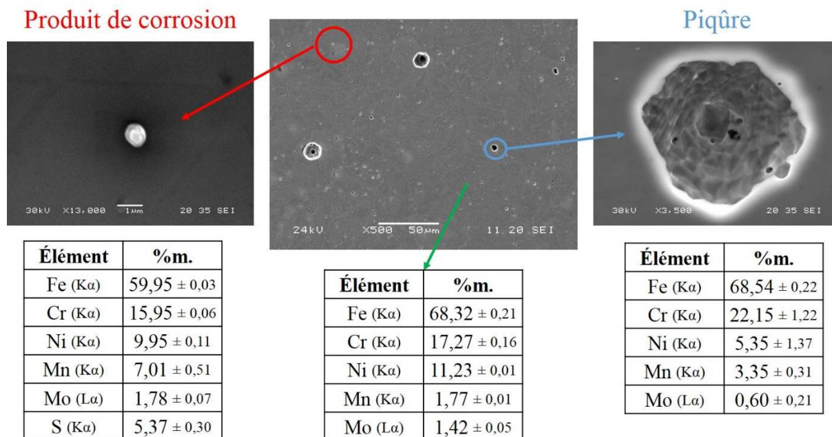
Figure 64 : Analyse quantitative par EDX de différentes zones de l'échantillon de fonderie électropoli ayant subi un test de corrosion (précisions données par l'appareil de mesure)
