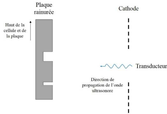
Figure 99 : Schéma représentant le positionnement des plaques rainurées lors de l'électropolissage avec et sans ultrasons
