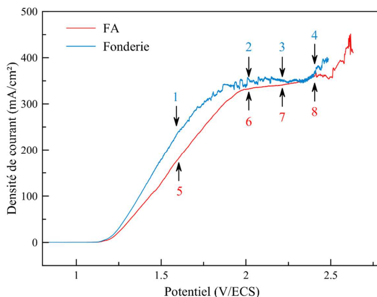
Figure 51 : Voltammétries linéaires anodiques des aciers inoxydables 316L en milieu acide à 70°C et 500 rpm, dans un mélange acide phosphorique et acide sulfurique ( V_b = 2 \text{ mV/s} ). Les potentiels choisis pour l'électropolissage sont marqués de 1 à 8.
