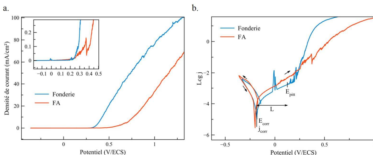
Figure 61 : Courbes de polarisation des aciers inoxydables 316L de fonderie et de fabrication additive avant électropolissage en milieu NaCl 3 % (a). Détermination du potentiel de corrosion ( E_{corr} ), du potentiel de piqûre ( E_{pitt} ), du courant résiduel ( I_{res} ) et de la longueur du plateau de passivation (b).
