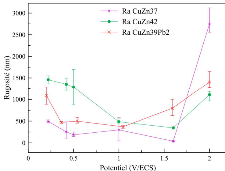
Figure 37 : Comparatif de l'évolution de la moyenne arithmétique de la rugosité (Ra) mesurée par profilométrie mécanique en fonction du potentiel pour les 3 nuances de laiton
