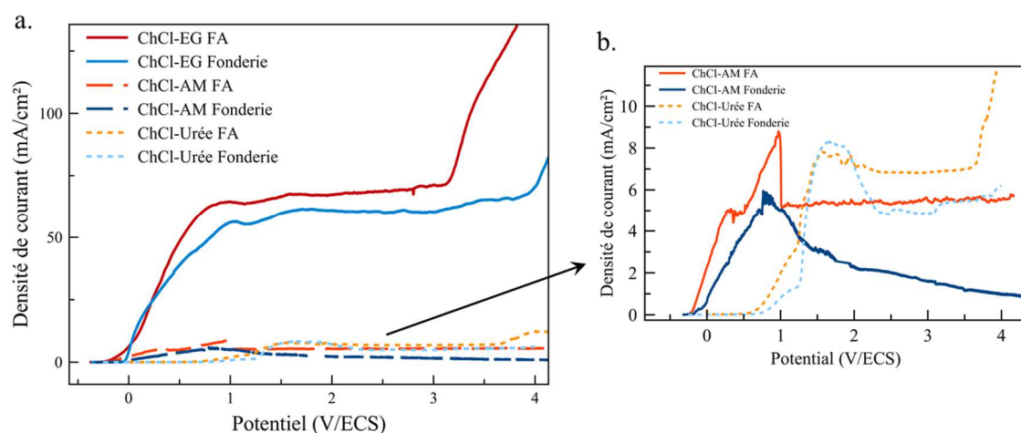
Figure 114 : Courbes de polarisation anodique pour les échantillons de fonderie (bleu) et de fabrication additive (rouge) dans les mélanges ChCl-EG, ChCl-Urée, ChCl-AM à 70°C et 500 rpm : (a) ensemble des solvants et (b) ChCl-Urée et ChCl-AM.
