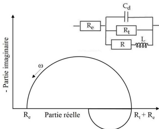
Figure 140 : Représentation du diagramme d'impédance lorsque qu'une espèce est adsorbée à la surface d'une électrode et circuit électrique équivalent [7,8]
