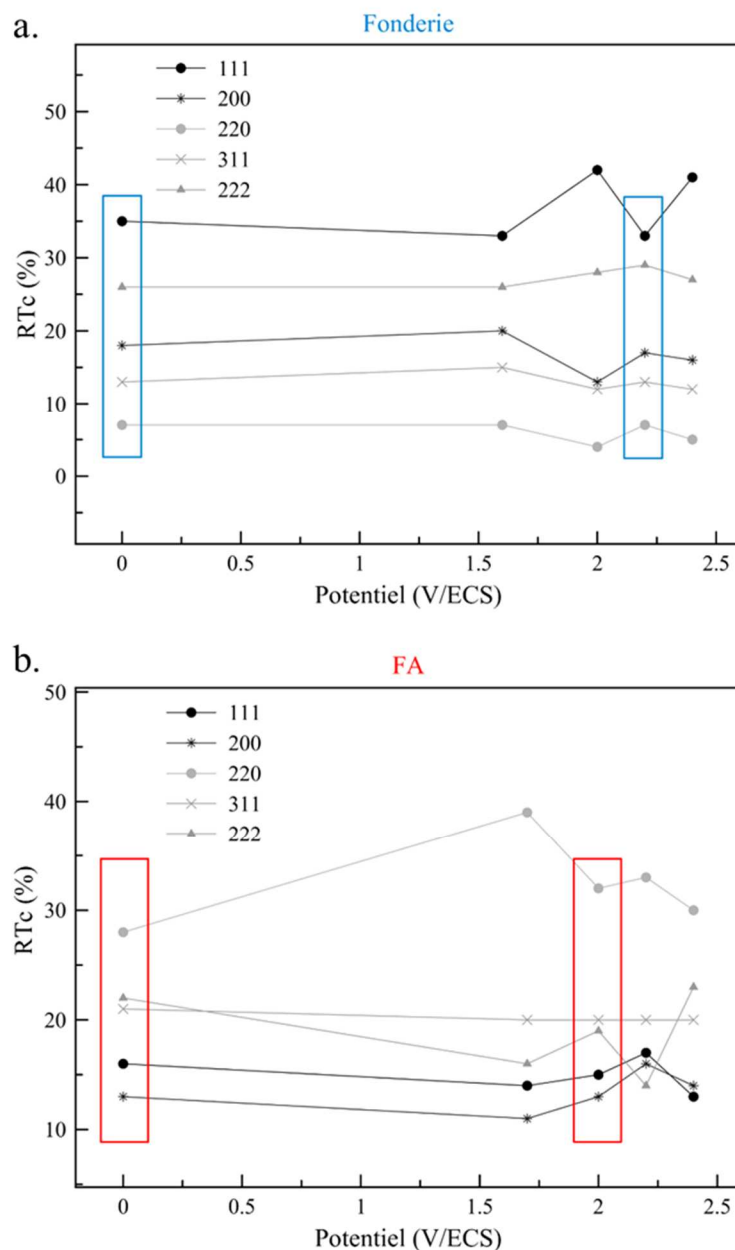
Figure 59 : Évolution des coefficients relatifs de texture pour les surfaces d'aciers inoxydables électropolies à différents potentiels en milieu acide à 70°C et 500 rpm : (a), fonderie et (b) fabrication additive
