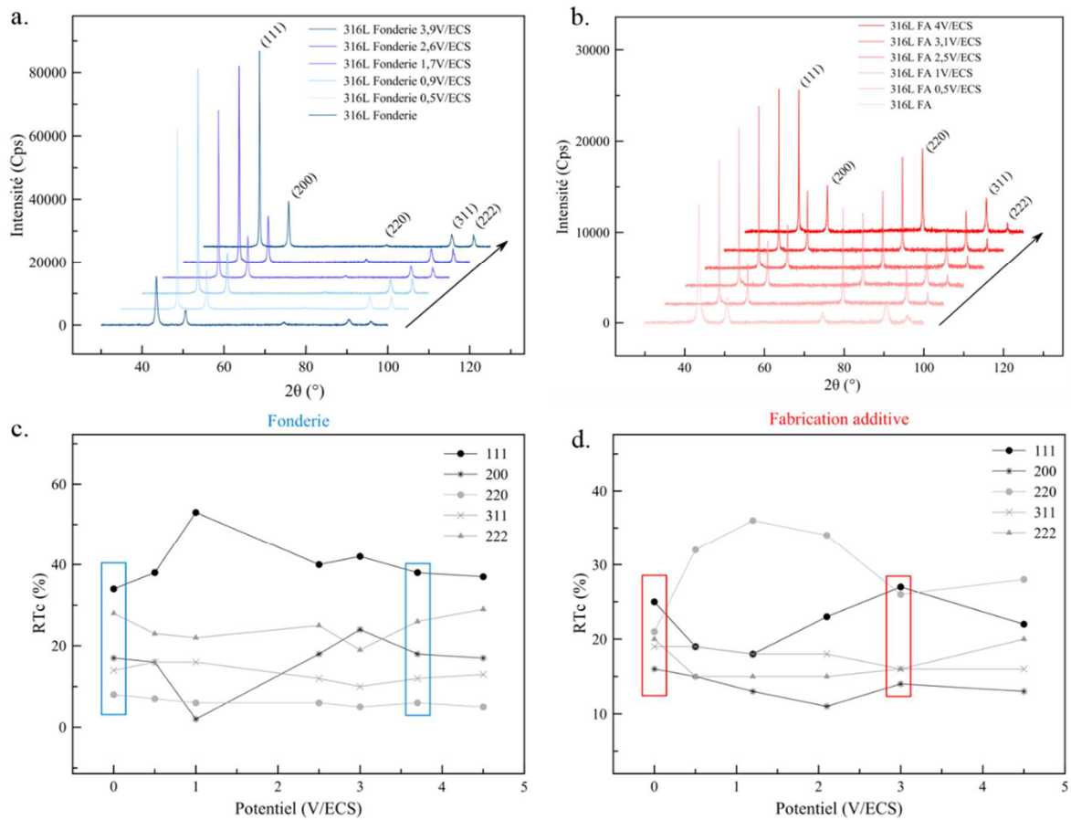
Figure 124 : Évolution des diffractogrammes et des coefficients relatifs de texture pour différents potentiels d'électropolissage en milieu DES : (a), (c) fonderie et (b), (d) fabrication additive
