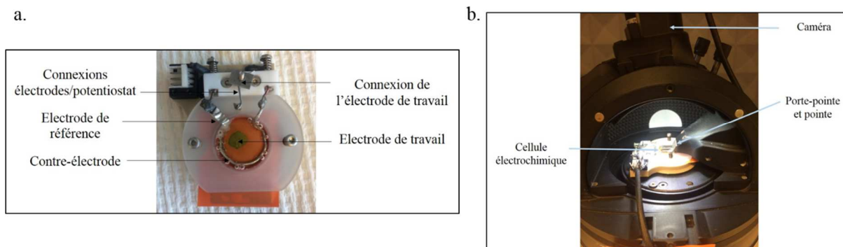
Figure 129 : Montage utilisé pour les expériences d'AFM in-situ : cellule électrochimique utilisée (a.), emplacement de la cellule dans l'AFM (b.).
