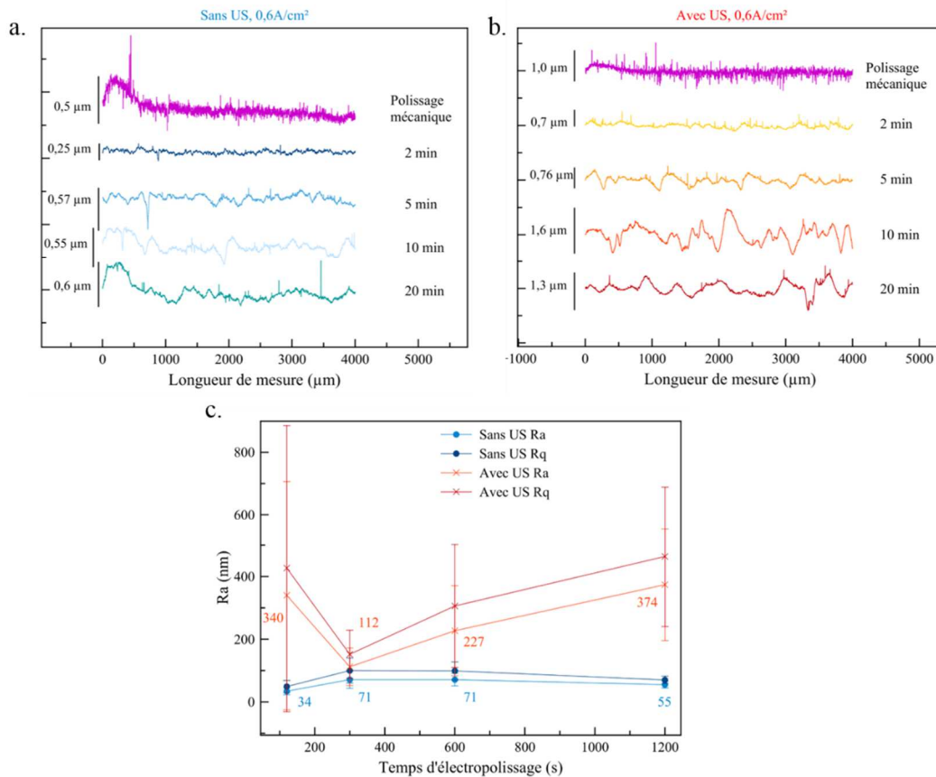
Figure 93 : Évolution de la rugosité de surface obtenue par profilométrie mécanique pour les échantillons d'acier inoxydables électropolisés avec et sans ultrasons pour différents temps à 0,6 \text{ A/cm}^2 : (a) profils de surface sous conditions silencieuses, (b) profils de surface sous ultrasons et (c) évolution des paramètres de rugosité en fonction du temps
