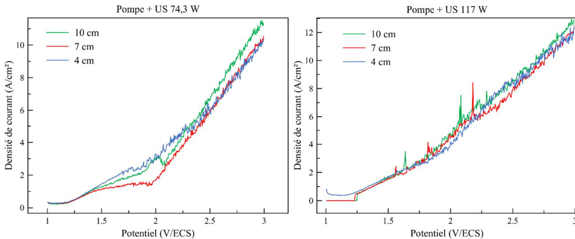
Figure 88 : Comportement anodique de l'acier inoxydable 316L en milieu acide phosphorique/acide sulfurique à 70°C dans la cuve avec la pompe et les ultrasons
