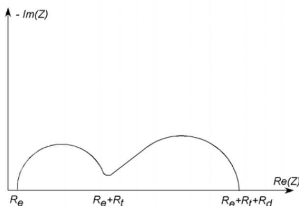
Figure 139 : Diagramme de l'impédance électrochimique d'une cinétique d'activation-diffusion dans une couche de diffusion d'épaisseur finie (dans l'hypothèse de Nernst) [5]
