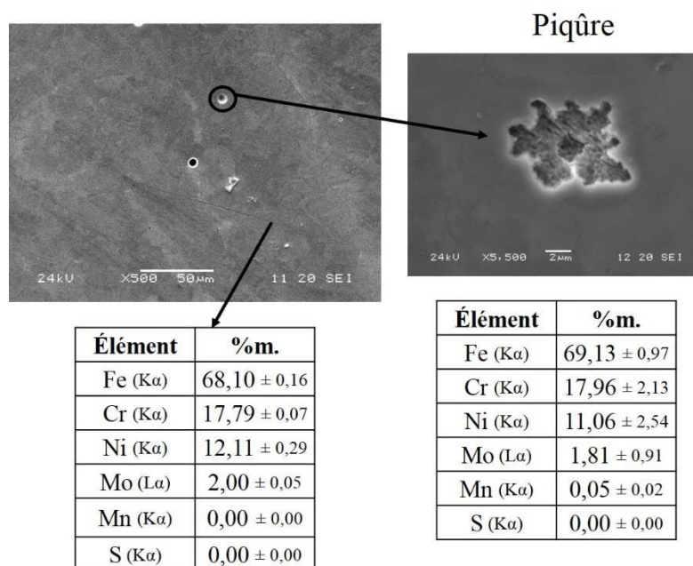
Figure 65 : Analyse quantitative par EDX de différentes zones de l'échantillon de fabrication additive électropoli ayant subi un test de corrosion (précisions données par l'appareil de mesure)
