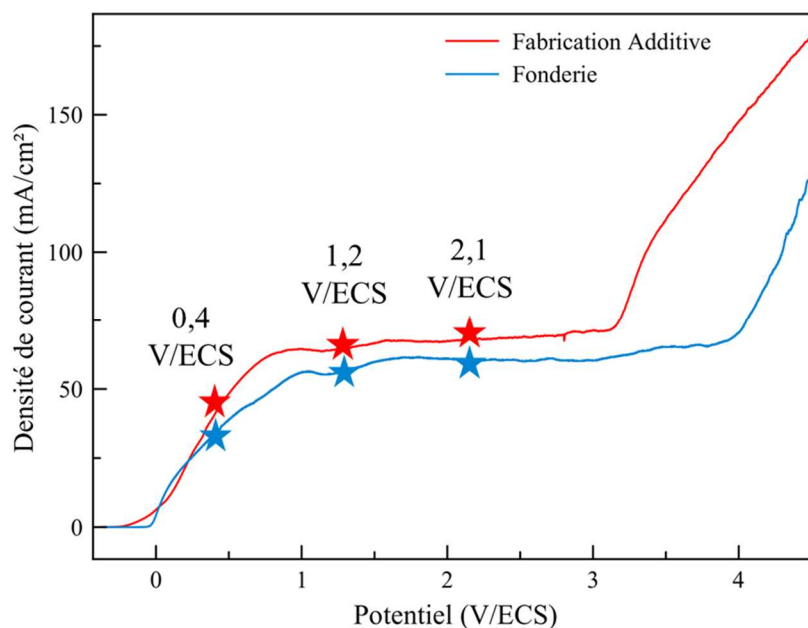
Figure 145 : Potentiels sélectionnés pour les mesures d'impédance électrochimique à partir des courbes intensité-potential des aciers inoxydables 316L de fonderie (bleu) et de fabrication additive (rouge) en milieu \text{ChCl-EG} à 70^\circ\text{C} et 500 rpm
