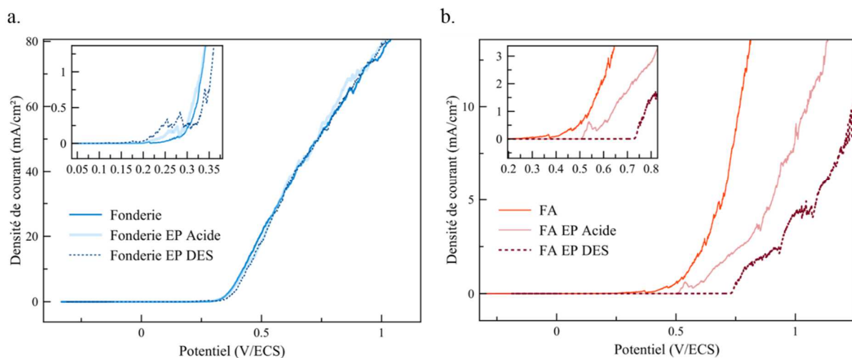
Figure 126 : Courbes de polarisation en milieu NaCl à 25°C des échantillons avant et après électropolissage en milieu acide et milieu DES : (a) acier inoxydable 316L de fonderie et (b) de fabrication additive
