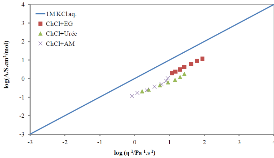
Figure 110 : Diagrammes de Walden pour les DES testés lors de cette étude extraits de [36]
