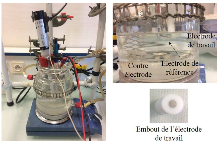
Figure 141 : Cellule électrochimique utilisée pour les mesures par SIE
