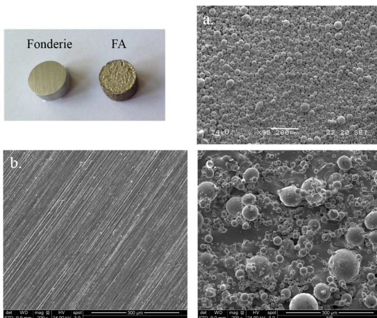
Figure 42 : Echantillons d'aciers inoxydables 316L issus de fonderie et de fabrication additive utilisés lors de cette étude et images MEB de (a) la poudre utilisée pour la fabrication additive et de leurs surfaces (b) fonderie et (c) fabrication additive
