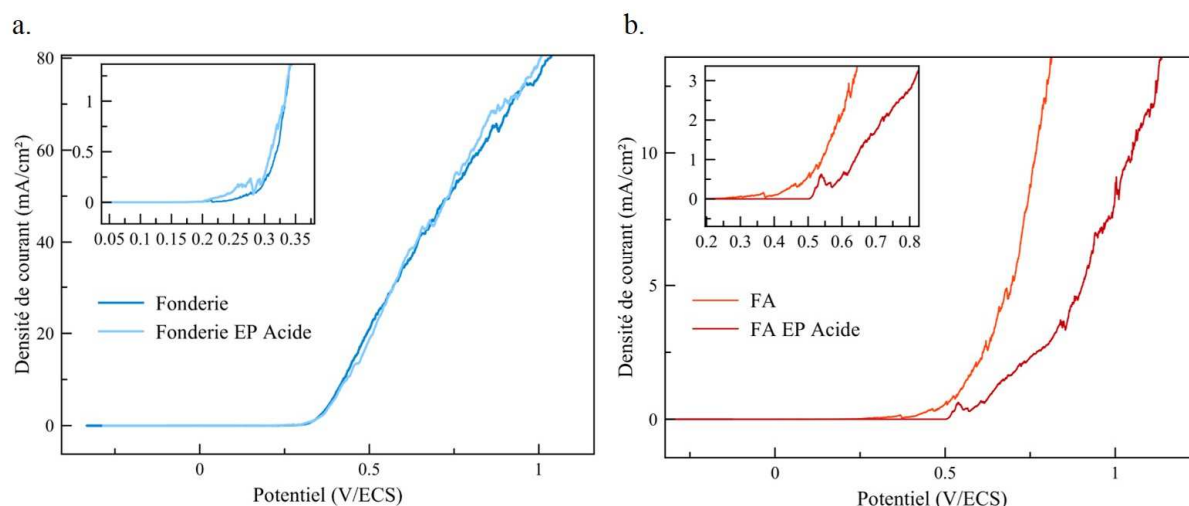
Figure 62 : Courbes de polarisation des aciers inoxydables 316L de fonderie et de fabrication additive avant et après électropolissage en milieu NaCl 3 %
