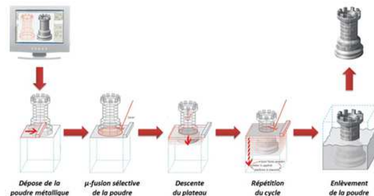
Figure 4 : Procédé de fabrication par fusion laser sur lit de poudre (source BV Proto)
