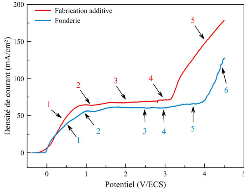
Figure 119 : Potentiels d'électropolissage choisis à partir des courbes intensité-potentiel des deux matériaux en milieu DES à 70°C et 500 rpm
