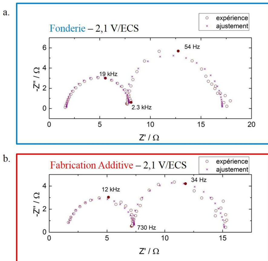
Figure 147 : Comparaison entre les diagrammes d'impédance simulés et expérimentaux pour l'électropolissage des deux aciers inoxydables 316L en milieu acide pour un potentiel de 2,1 V/ECS : (a) fonderie et (b) fabrication additive
