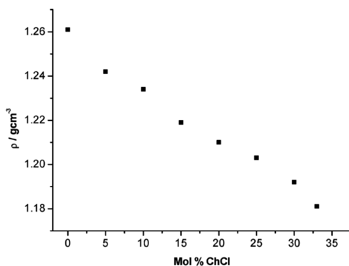
Figure 109 : Densité du DES ChCl-glycérol en fonction de la composition en ChCl d'après [32]
