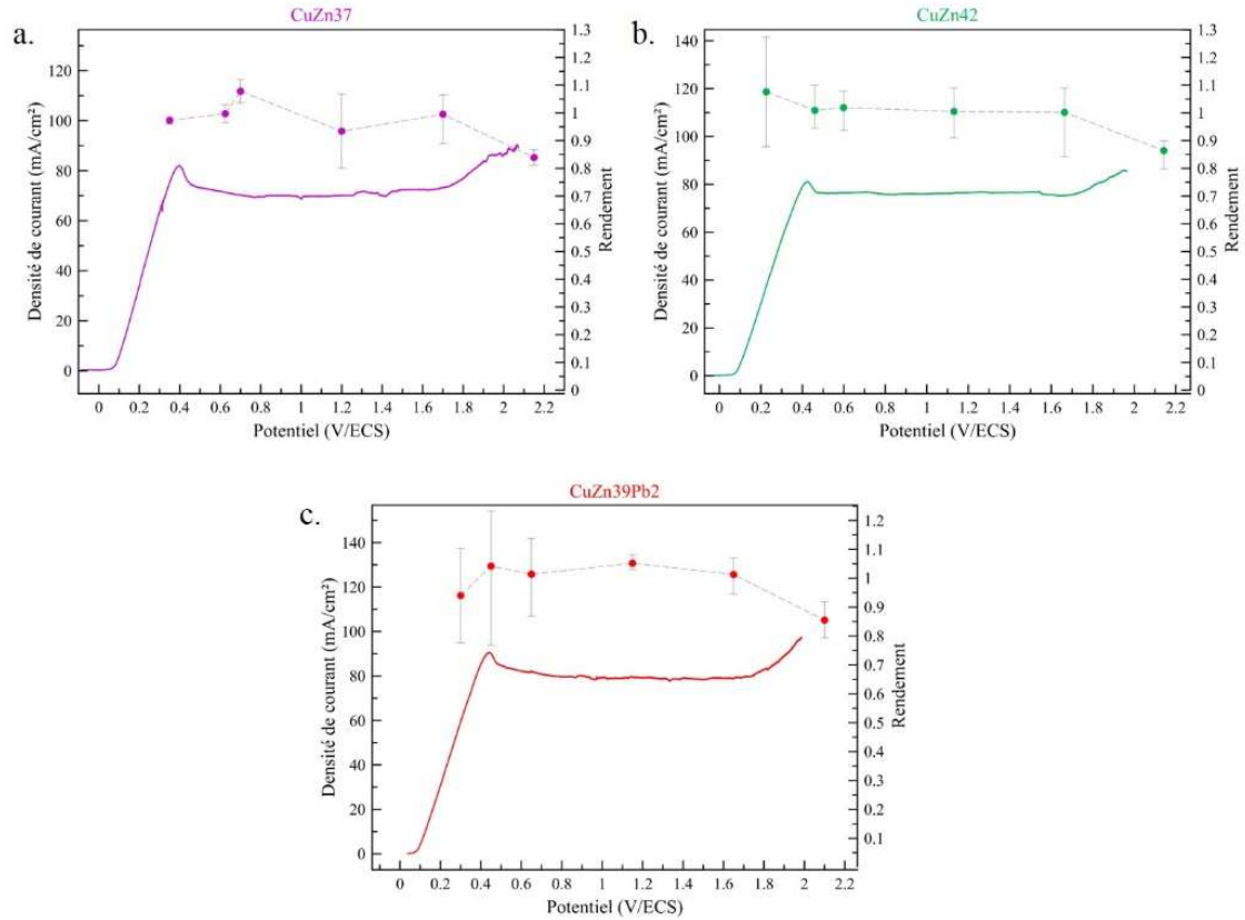
Figure 30 : Évolution du rendement de dissolution des différentes nuances de laiton en fonction du potentiel : (a) CuZn 37 , (b) CuZn 42 et (c) CuZn 39 Pb 2 avec une vitesse de rotation de 500 rpm dans l'électrolyte d'acide phosphorique à 25°C
