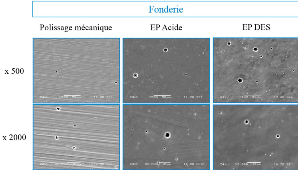
Figure 127 : Images MEB des échantillons de fonderie après croissance des piqûres pendant 1 heure à 100 \mu\text{A}/\text{cm}^2 dans \text{NaCl} 3 %
