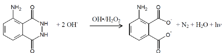
Figure 81 : Réaction d'oxydation du luminol
