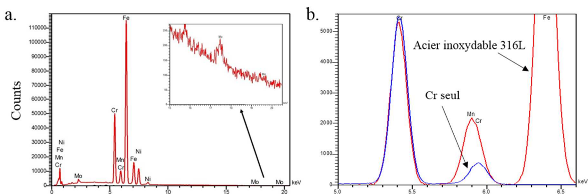
Figure 66 : Spectres EDX obtenus pour la vérification de la présence de molybdène et de chrome dans l'échantillon
