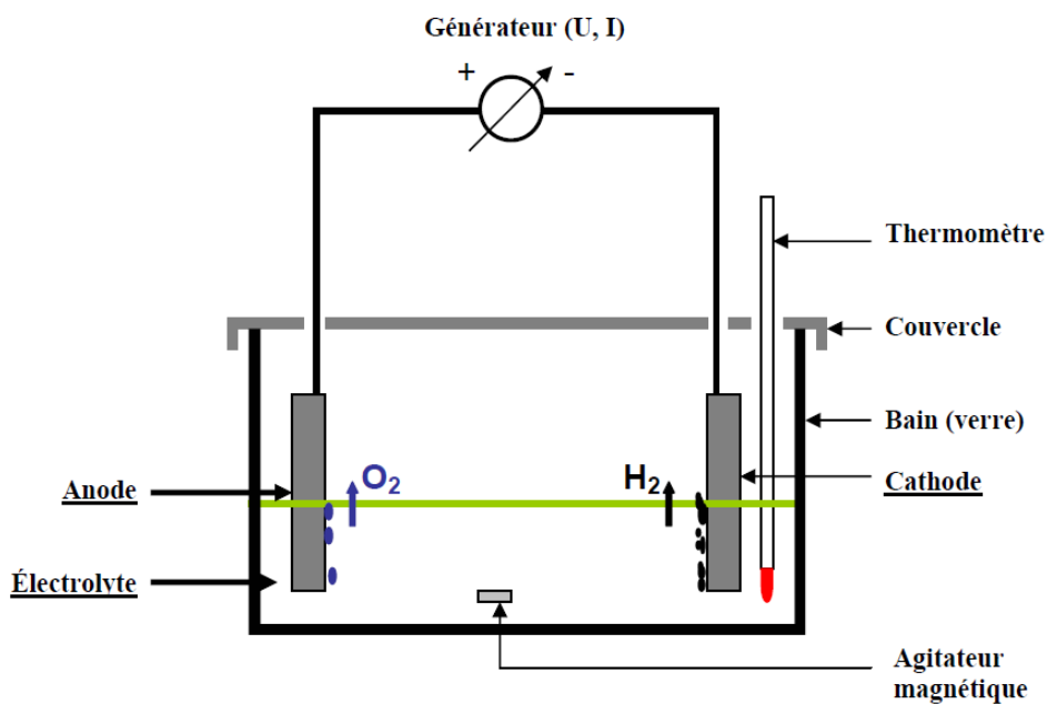
Figure 13 : Schéma d'une cellule d'électropolissage extraite de [36]
