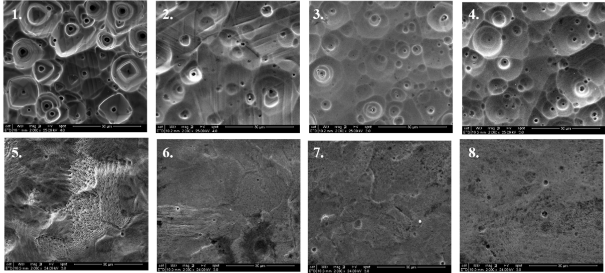
Figure 49 : Images MEB (électrons secondaires) des échantillons d'acier inoxydable électropolis pendant 20 minutes à différents potentiels en milieu acide à 35°C: (1) à (4) fonderie et (5) à (8) fabrication additive
