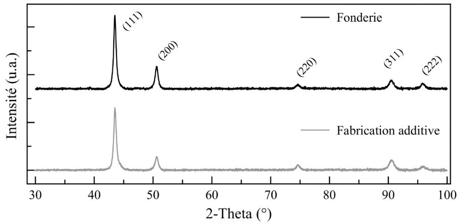
Figure 44 : Diffractogrammes des matériaux avant électropolissage
