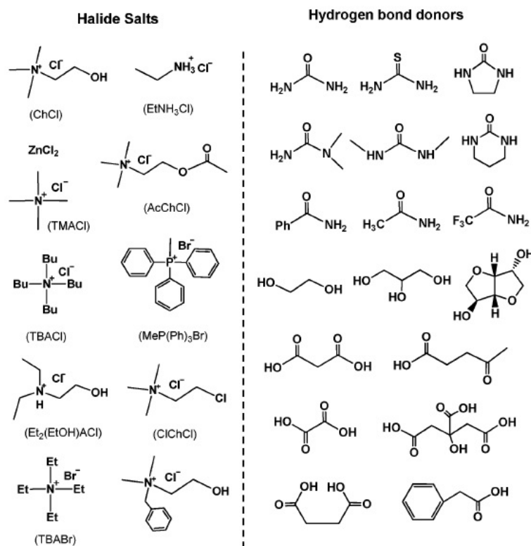
Figure 108 : Principaux sels ioniques et donneurs d'hydrogène utilisés pour la synthèse de DESs [23]
