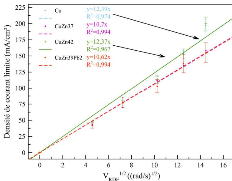
Figure 27 : Évolution des courbes de Levich pour le cuivre et les laiton étudiés dans H 3 PO 4 66 % à 25°C
