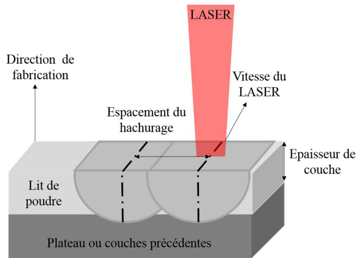
Figure 5 : Schéma illustrant les paramètres du procédé de fabrication additive utilisé lors de cette étude
