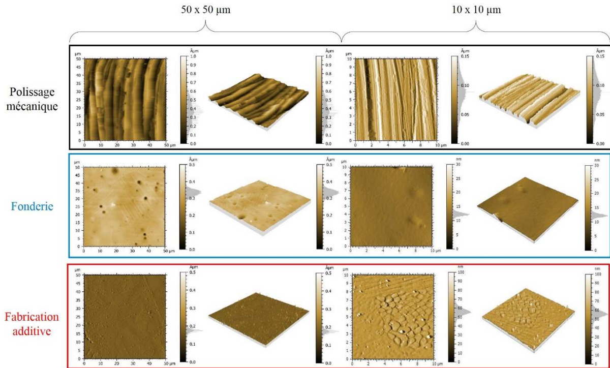
Figure 57 : Images AFM en 2D et 3D des surfaces avant et après électropolissage en milieu acide pendant 20 minutes à 2,4 V/ECS (50 x 50 \mu\text{m} ou 10 x 10 \mu\text{m} )
