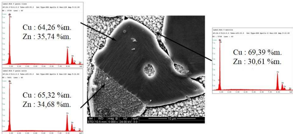
Figure 35 : Image MEB et analyse EDX de l'échantillon 1 de \text{CuZn}_{39}\text{Pb}_2 électropoli à 0,2 V/ECS pendant 10 minutes à 500 rpm
