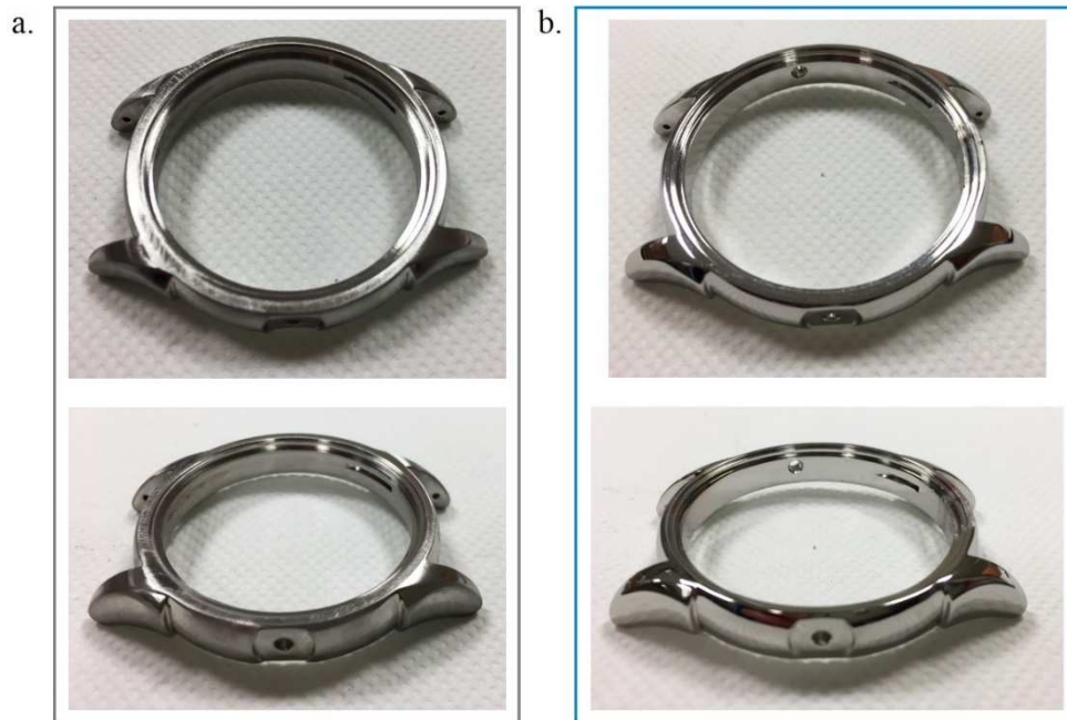
Figure 105 : Carrures avant (a) et après (b) électropolissage en milieu acide phospho-sulfurique à 70°C pendant 2 minutes à 0,6 A/cm 2
