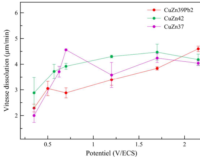
Figure 31 : Évolution des vitesses de dissolution des différents laiton en fonction du potentiel d'électropolissage en milieu acide à 25°C et 500 rpm
