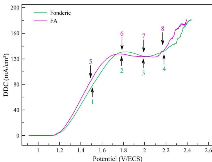
Figure 48 : Courbes de polarisation des aciers inoxydables 316L en milieu acide à 35°C et 500rpm, dans un mélange acide phosphorique et acide sulfurique ( V_b = 2 \text{ mV/s} ). Les potentiels choisis pour l'électropolissage sont marqués de 1 à 8.
