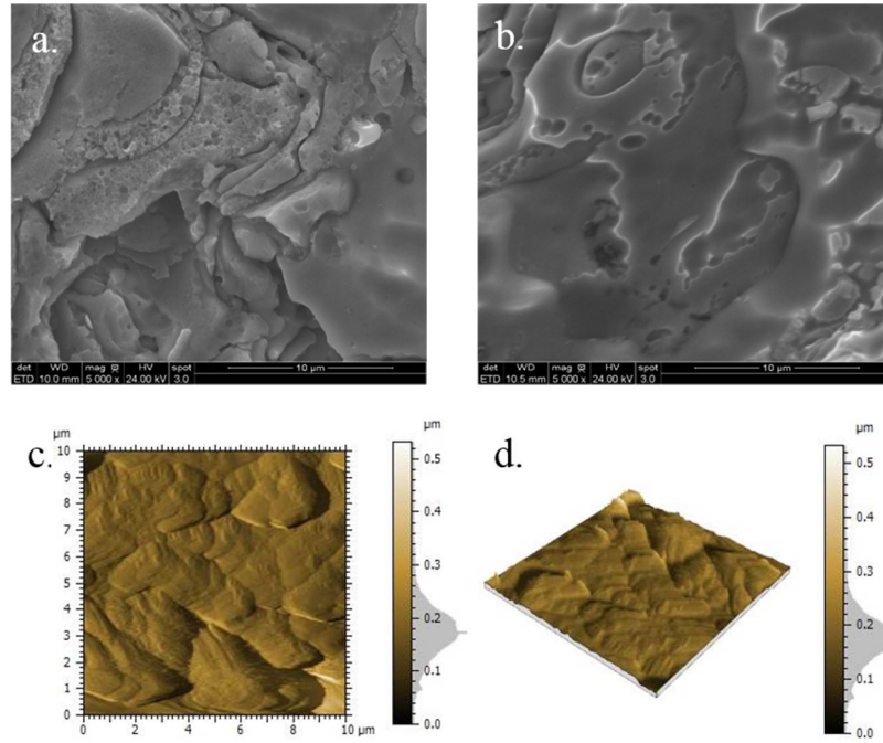
Figure 71 : Images MEB et AFM des échantillons après électropolissage en milieu acide (a)(c)(d) Diamalloy 1003 et (b) Metco 41C
