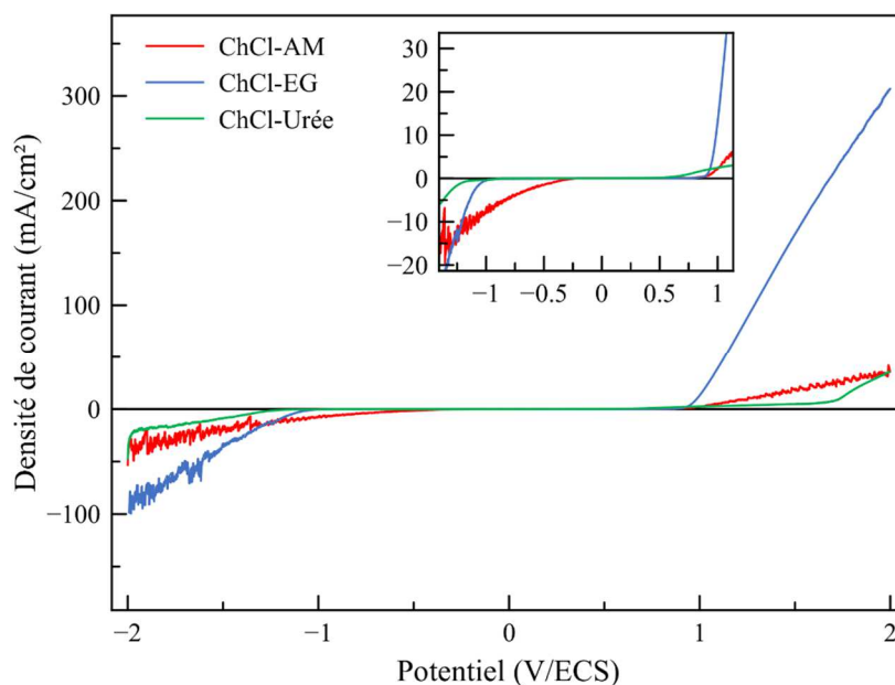
Figure 113 : Courbes de polarisation obtenues dans chacun des DESs à 70°C, 500 rpm
