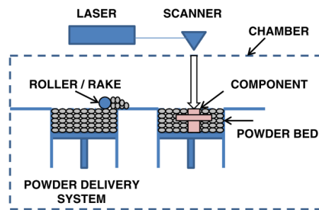
Figure 3 : Représentation schématique du procédé de fabrication additive par fusion laser sur lit de poudre [13]
