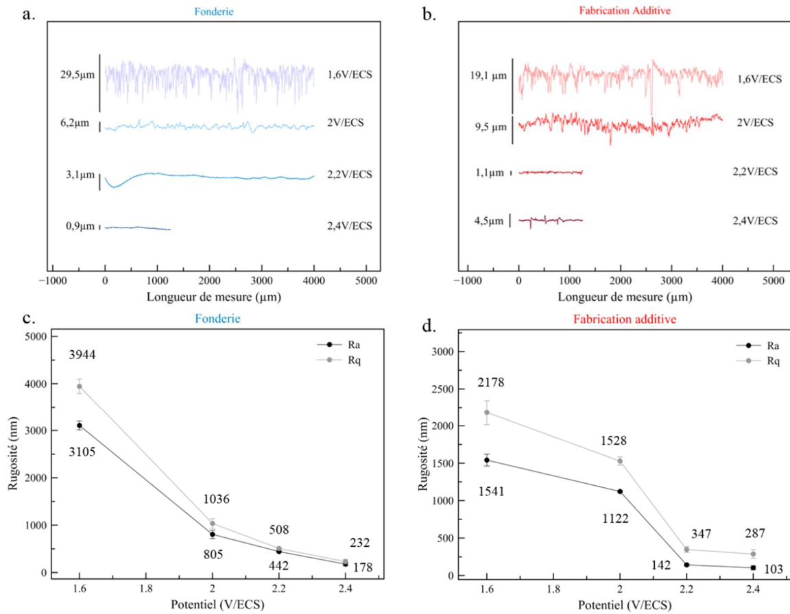
Figure 56 : Évolution des paramètres de rugosité mesurés par profilométrie mécanique pour les échantillons d'acier inoxydable 316L électropolis en milieu acide
