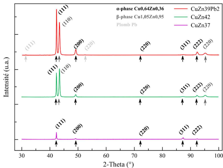
Figure 19 : Diffractogrammes obtenus sur les pastilles de laiton avant électropolissage
