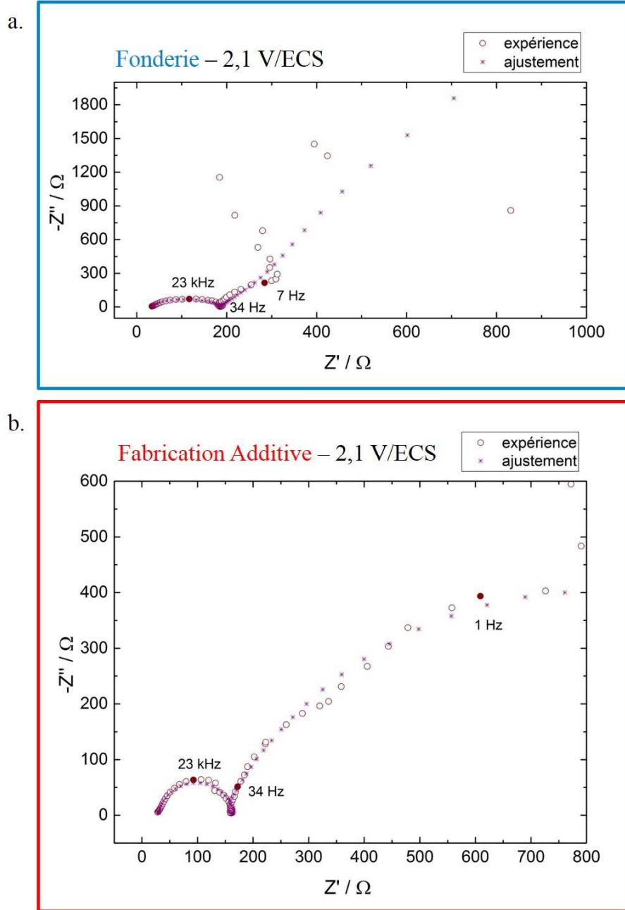
Figure 148 : Comparaison entre les diagrammes d'impédance simulés et expérimentaux pour l'électropolissage des deux aciers inoxydables 316L en milieu \text{ChCl-EG} pour un potentiel de 2,1 V/ECS : (a) fonderie et (b) fabrication additive
