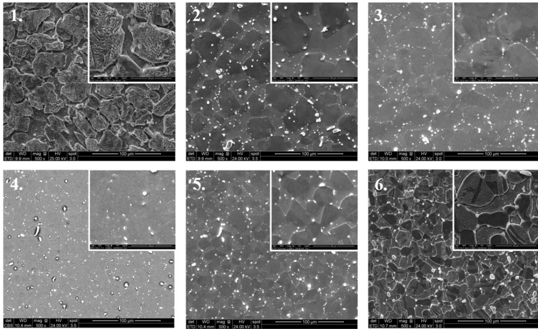
Figure 34 : Image MEB (x 500 et x 2000) des échantillons de \text{CuZn}_{39}\text{Pb}_2 obtenus après électropolissage à différents potentiels (1) 0,2, (2) 0,364, (3) 0,5, (4), 1,0, (5) 1,6, (6) 2,0 V/ECS à 500 rpm.
