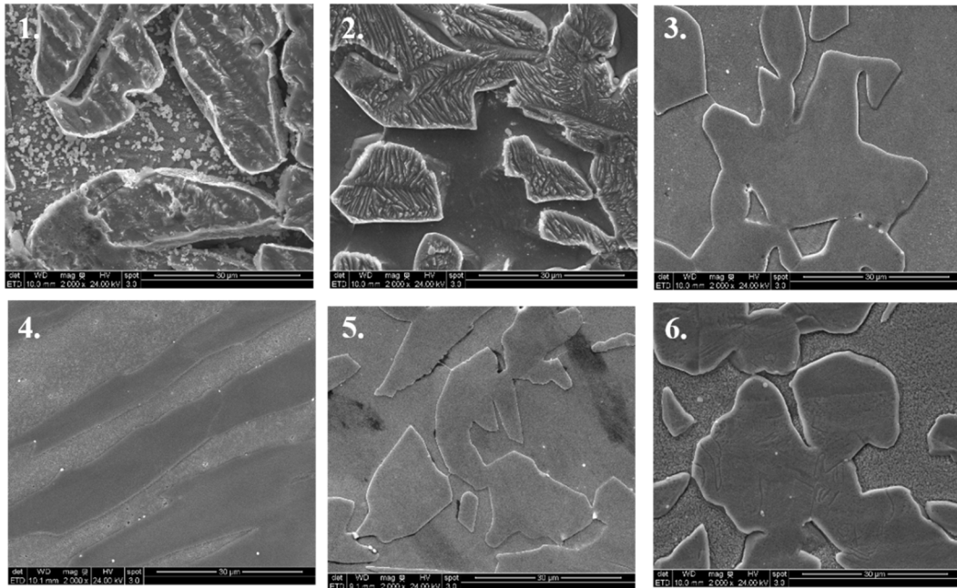
Figure 33 : Images MEB (x 2000) des échantillons de CuZn 42 obtenus après électropolissage à différents potentiels (1) 0,22, (2) 0,42, (3) 0,5, (4) 1,0, (5) 1,6, (6) 2,0 V/ECS à 500 rpm
