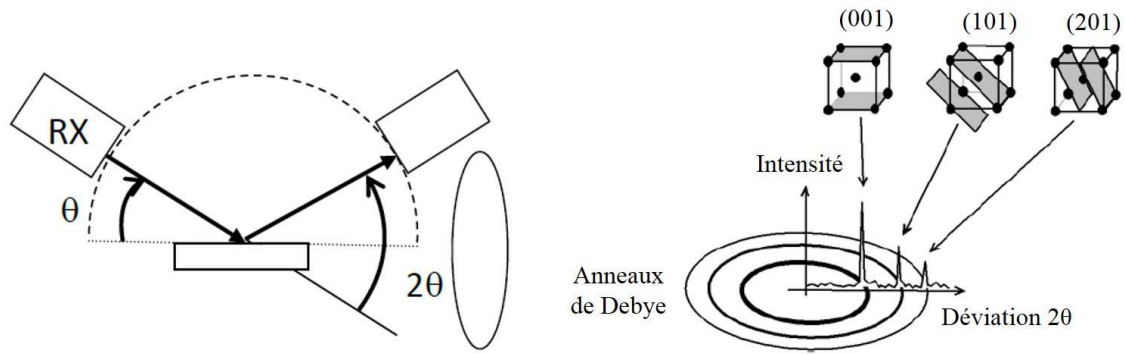
Figure 151 : Principe général de la DRX avec l'utilisation de la loi de Bragg
