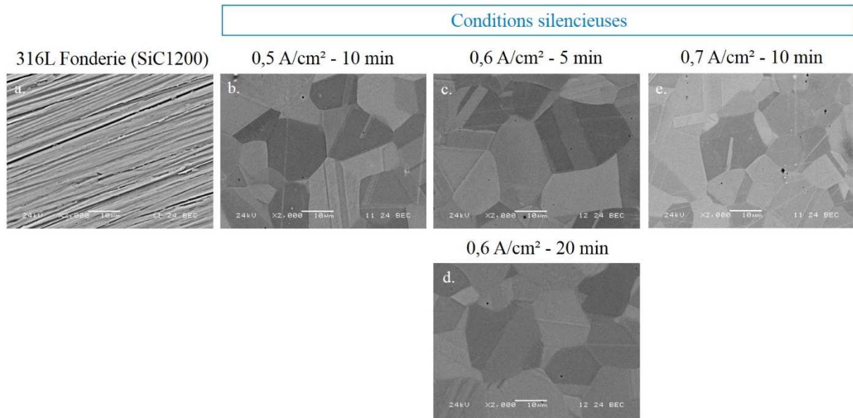
Figure 90 : Morphologie des échantillons électropolis en milieu acide à 70°C pour différentes densités de courant et différents temps : (a) avant électropolissage, (b) plaque 7, (c) plaque 4, (d) plaque 3 et (e) plaque 6.
