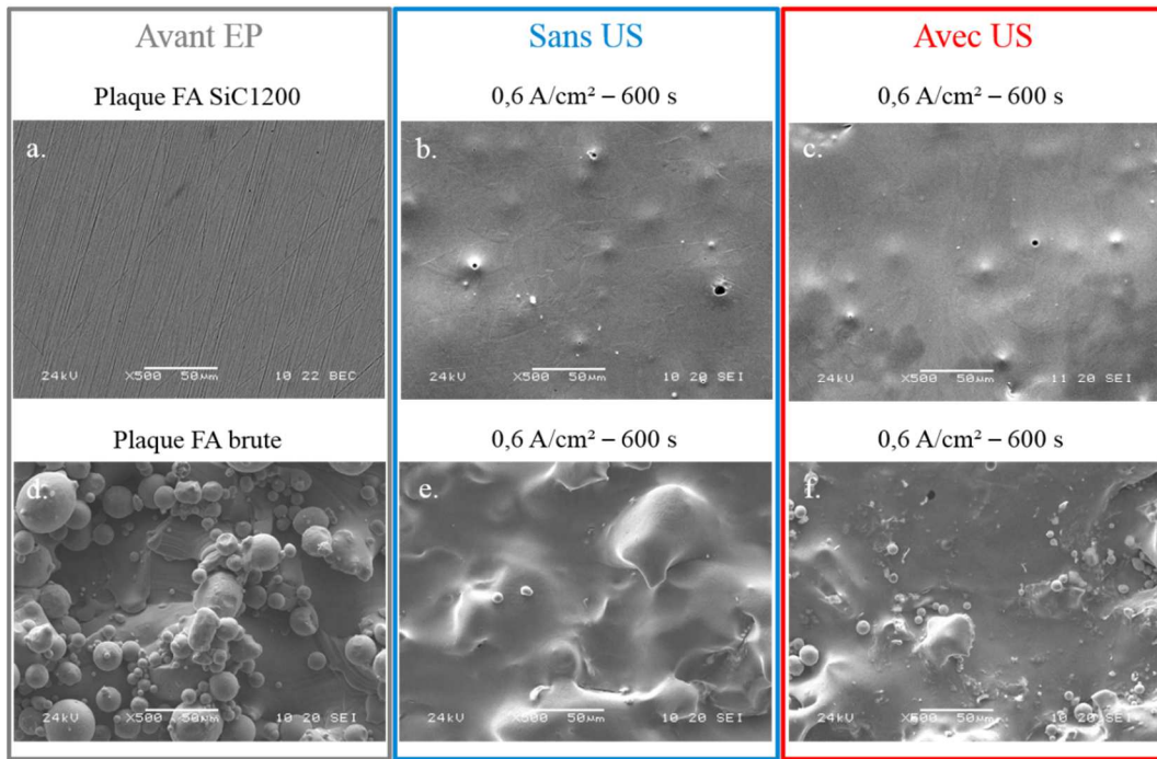
Figure 96 : Images MEB des plaques de fabrication additive avant et après électropolissage en milieu acide avec et sans ultrasons : (a) plaque après pré-polissage mécanique, (b) plaque pré-polie mécaniquement puis électropolie sous conditions silencieuses, (c) plaque pré-polie mécaniquement électropolie avec ultrasons, (d) plaque brute de fabrication additive, (e) plaque brute électropolie sous conditions silencieuses et (f) plaque brute de fabrication électropolie avec ultrasons.
