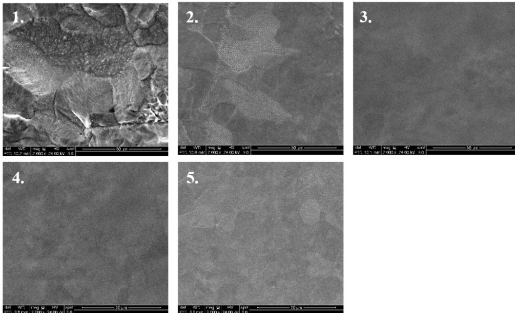
Figure 122 : Analyse morphologique des échantillons d'acier inoxydable 316L de fabrication additive électropolis à différents potentiel en milieu ChCl-EG à 70°C et 500 rpm.
