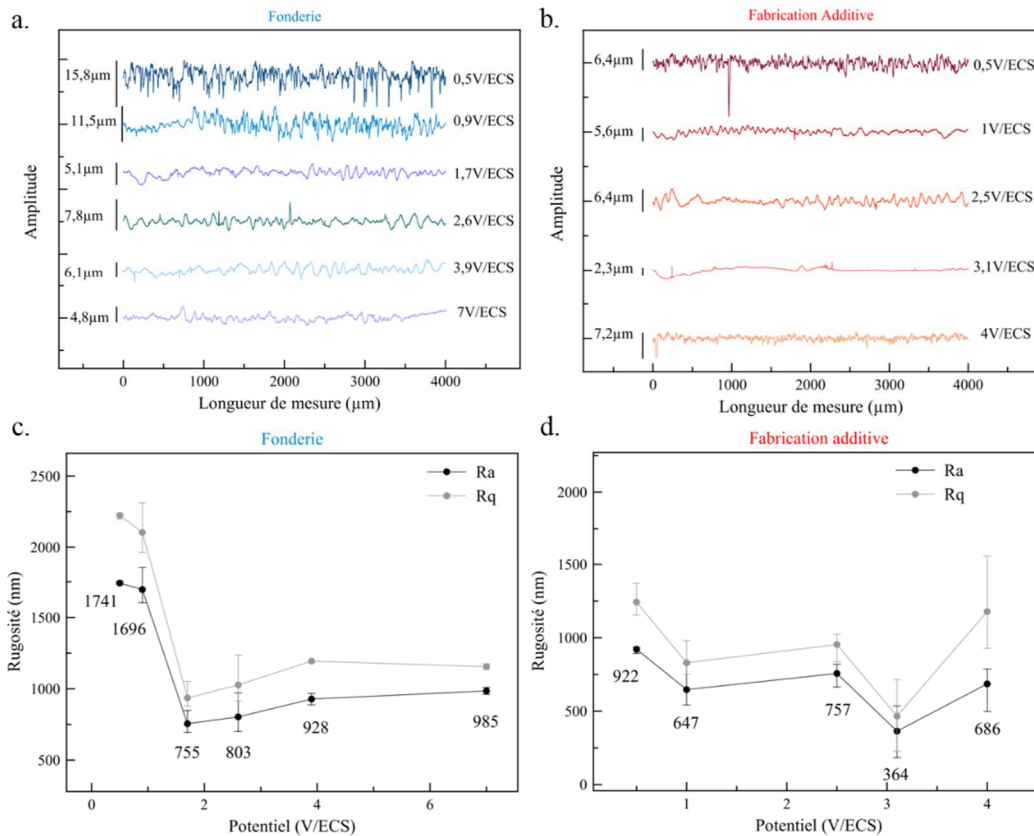
Figure 123 : Évolution des profils de rugosité ainsi que des paramètres Ra et Rq en fonction du potentiel d'électropolissage en milieu DES à 70°C et 500 rpm : (a), (c) acier inoxydable 316L de fonderie et (b), (d) de fabrication additive
