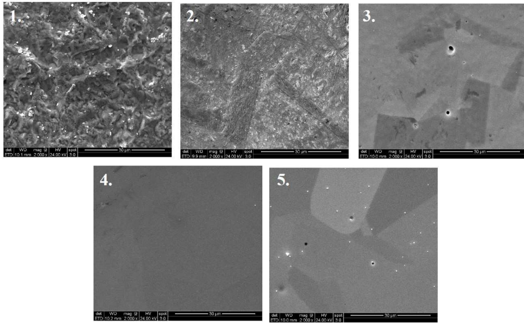
Figure 32 : Images MEB ( \times 2000 ) des échantillons de \text{CuZn}_{37} obtenus après électropolissage à différents potentiels (1) 0,25, (2) 0,44, (3) 0,52, (4), 1,07, (5) 1,6 V/ECS à 500 rpm
