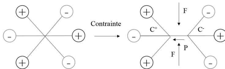
Figure 74 : Matériaux piézoélectriques sous contrainte [1]
