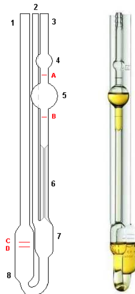
Figure 152 : Schéma et photographie d'un viscosimètre capillaire (viscosimètre de Ubbelohde)
