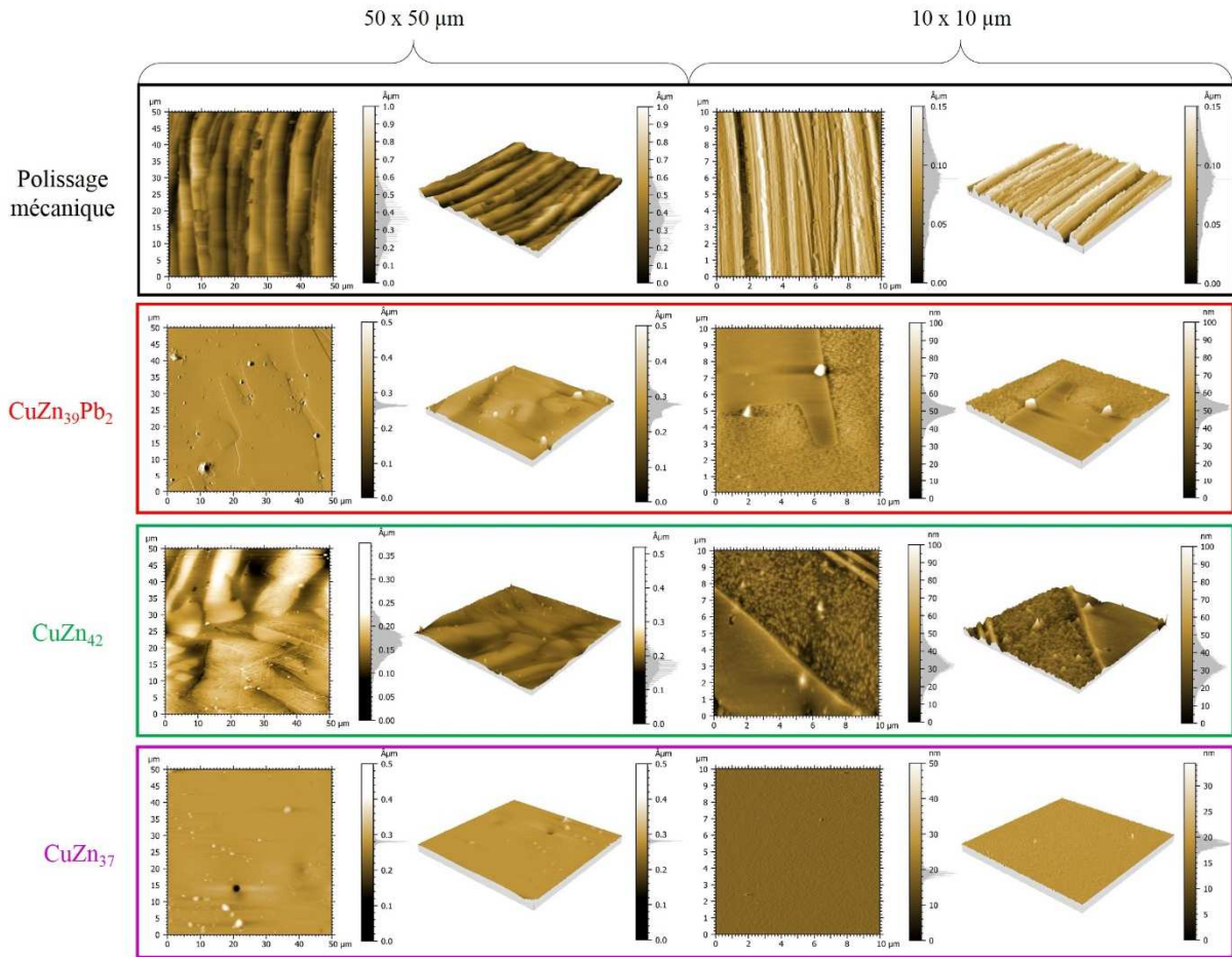
Figure 40 : Images AFM des échantillons électropolis au potentiel du milieu de plateau : avant électropolissage, \text{CuZn}_{39}\text{Pb}_2 , \text{CuZn}_{42} et \text{CuZn}_{37}
