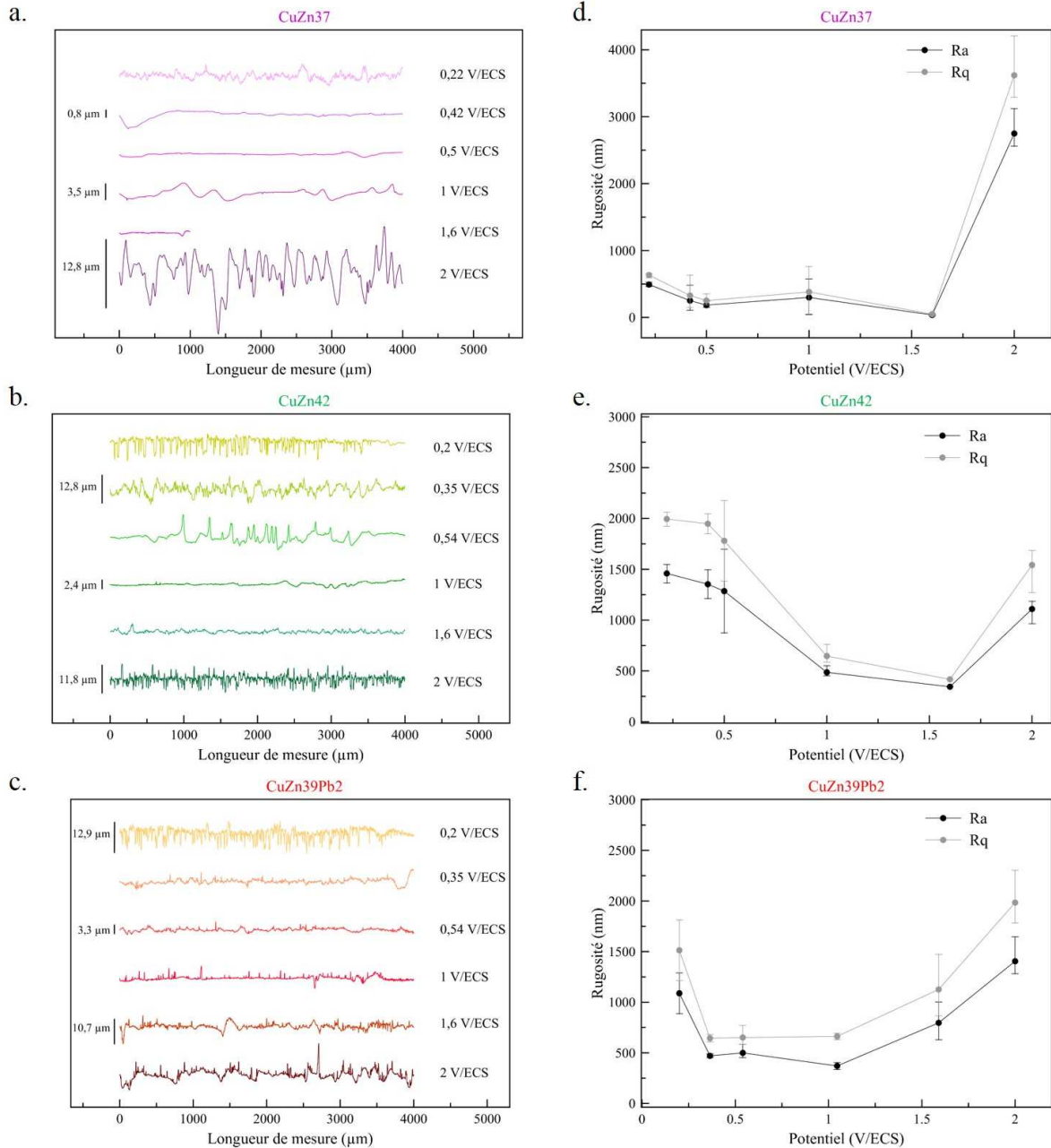
Figure 36 : Évolution des profils de rugosité et des valeurs de rugosité (Ra et Rq) des échantillons de laiton électropolis à différents potentiels : (a), (d) CuZn 37 , (b), (e) CuZn 42 et (c), (f) CuZn 39 Pb 2
