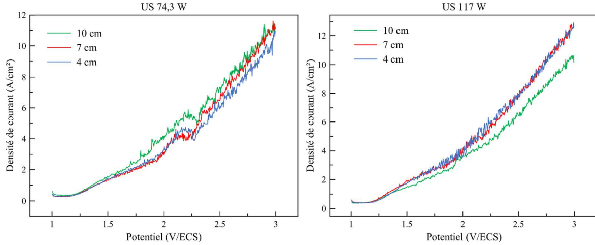
Figure 87 : Comportement anodique de l'acier inoxydable 316L en milieu acide phosphorique/acide sulfurique à 70°C dans la cuve sous ultrasons pour des distances électrode-transducteur entre 4 et 10 cm
