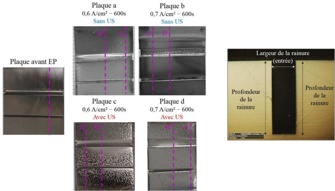
Figure 101 : Emplacement des zones analysées par microscopie optique pour les plaques rainurées électroplées avec et sans ultrasons et description des paramètres mesurés dans les rainures
