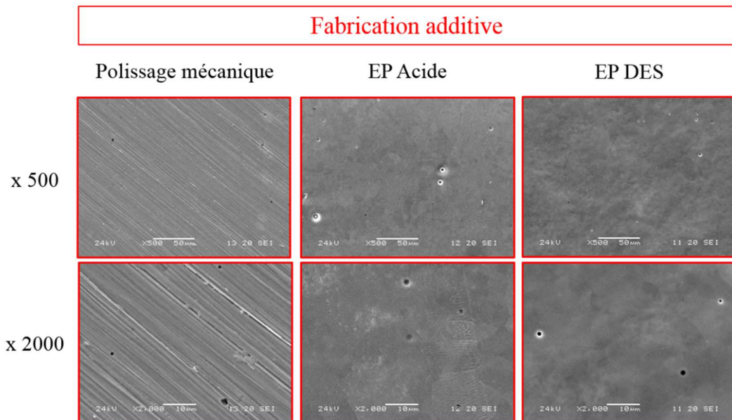
Figure 128 : Images MEB des échantillons de fabrication additive après croissance des piqûres pendant 1 heure à 100 \mu\text{A}/\text{cm}^2 dans \text{NaCl} 3 %
