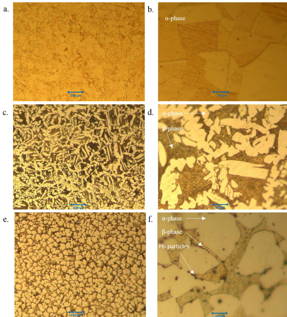
Figure 18 : Images en microscopie optique de microstructures de nuances de laiton après révélation dans une solution de chlorure ferrique : \text{CuZn}_{37} grossissements \times 50 et \times 500 (a, b), \text{CuZn}_{42} grossissements \times 50 et \times 500 (c, d) et \text{CuZn}_{39}\text{Pb}_2 grossissements \times 50 et \times 500 (e, f).
