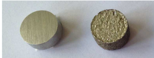
Figure 7 : Echantillons sorti d'usinage (gauche) et issu de fabrication additive (droite)
