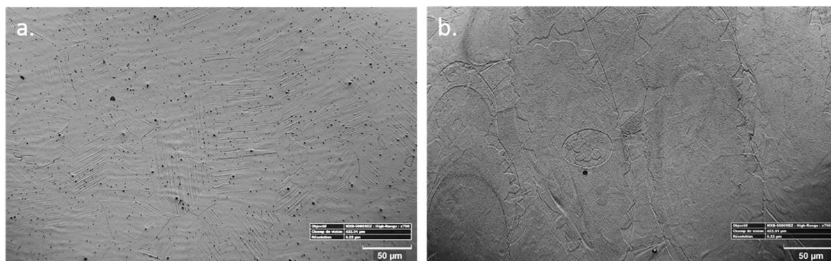
Figure 43 : Micrographies des échantillons après attaque chimique au chlorure ferrique (a) acier inoxydable 316L de fonderie, (b) acier inoxydable 316L issu de fabrication additive.
