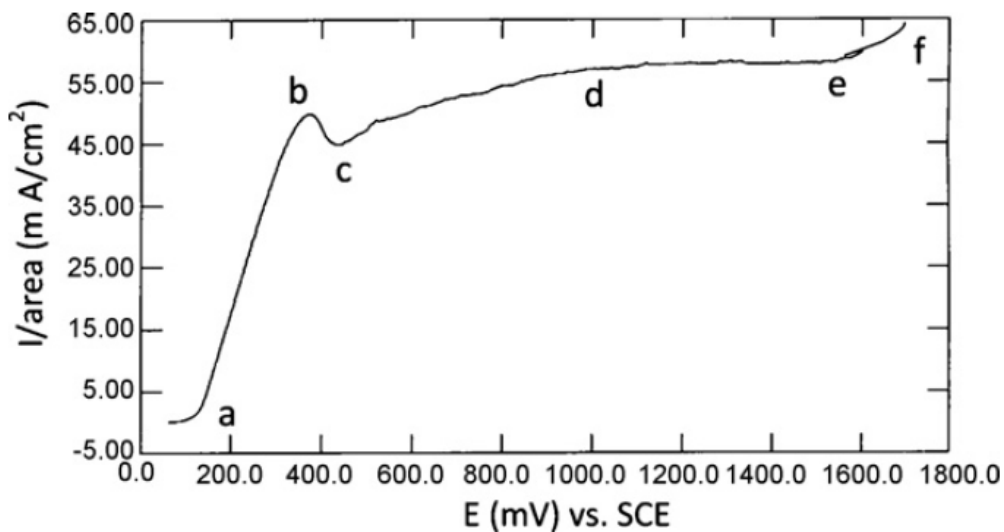
Figure 14 : Courbe de polarisation typique de l'électropolissage du cuivre en milieu phosphorique (extraite de [37])
