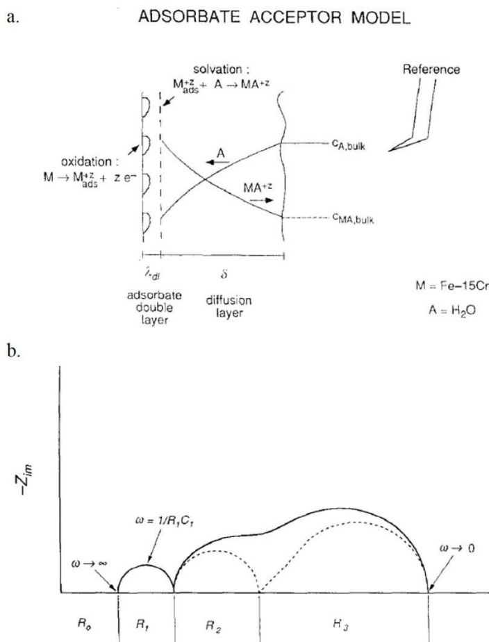
Figure 144 : Modèle de « l'accepteur » dans lequel la réaction d'électropolissage est limitée par la diffusion d'espèces acceptrices : (a) schéma illustrant le principe du modèle et (b) diagramme d'impédance associé au mécanisme réactionnel [2]
