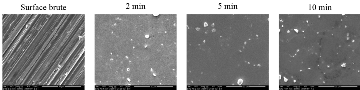
Figure 28 : Etat de surface d'échantillon de \text{CuZn}_{39}\text{Pb}_2 électropolé à 1046 mV/ECS dans l'acide phosphorique à 500 rpm et pour différents temps de traitement
