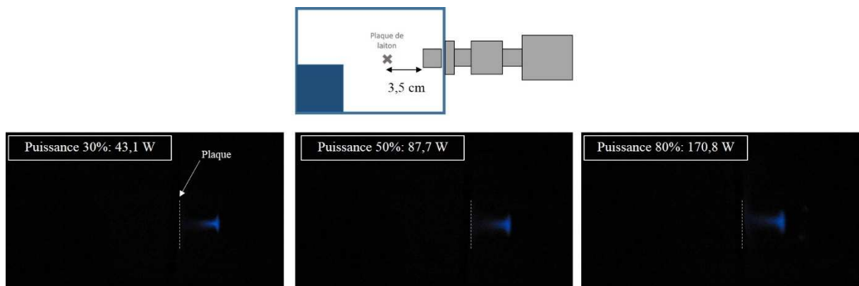
Figure 83 : Mise en évidence des zones chimiquement actives du réacteur par sonochimiluminescence en fonction de la puissance ultrasonore transmise en présence d'un obstacle placé à 3,5 cm du transducteur
