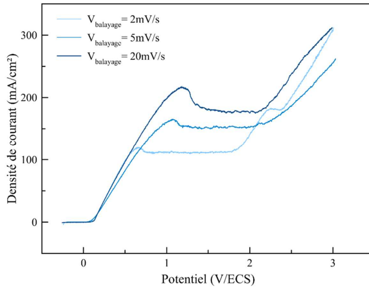
Figure 25 : Courbe de polarisation de \text{CuZn}_{39}\text{Pb}_2 en milieu acide phosphorique à 360 rpm pour différentes vitesses de balayage
