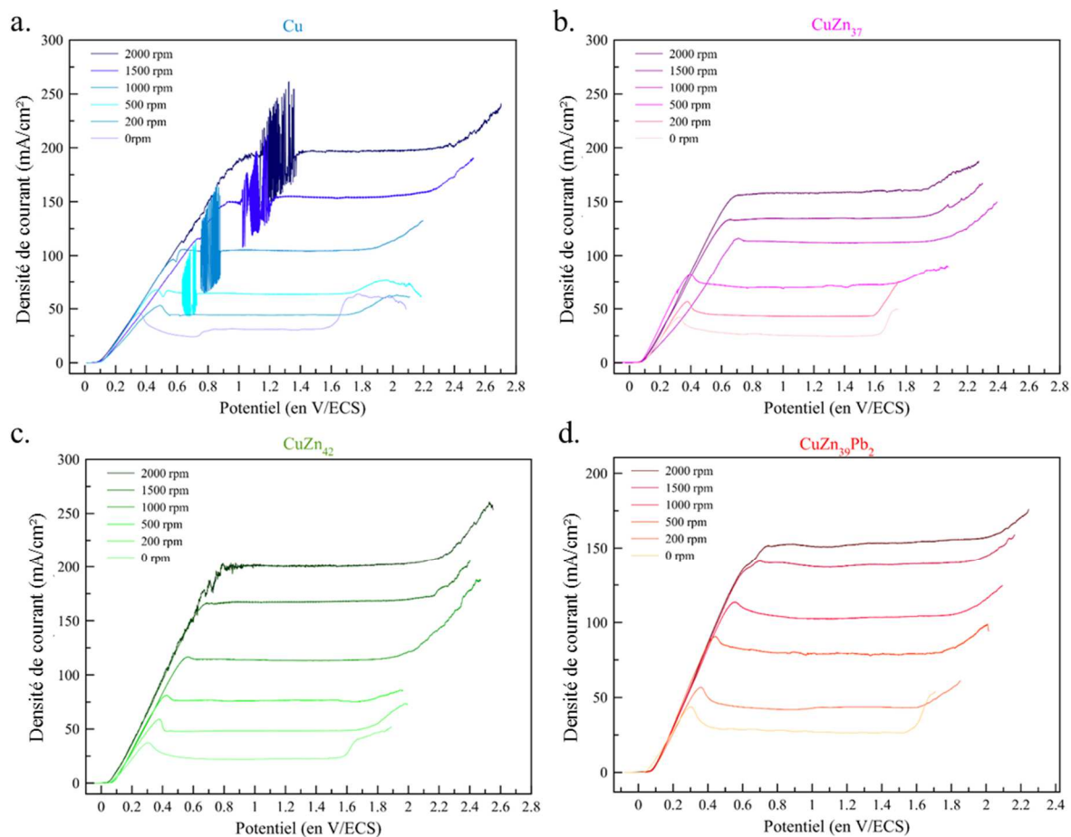
Figure 26 : Courbes de polarisation des alliages : (a) Cu, (b) CuZn_{37} , (c) CuZn_{42} et (d) CuZn_{39}Pb_2 dans H_3PO_4 10 M à 25 °C pour différentes vitesses de rotation d'électrode V_b = 2 mV/s
