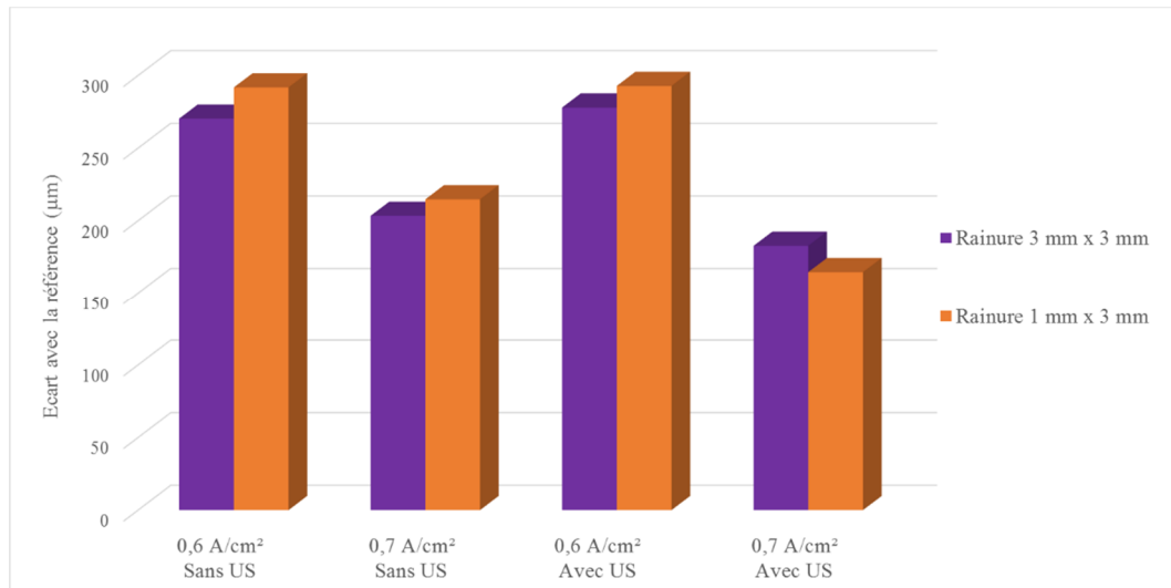
Figure 104 : Évolution des écarts dimensionnels au niveau de la profondeur des rainures de 1 x 3 mm et 3 x 3 mm entre la pièce de référence et les pièces électropolies avec et sans agitation ultrasonore pour deux densités de courant
