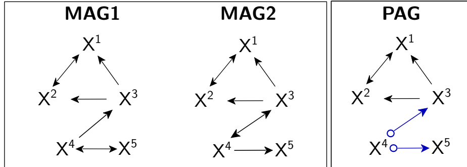
FIGURE 2.8 – Représentation de deux MAG équivalents au sens de Markov (MAG1 et MAG2) et du PAG de la classe d'équivalence.
