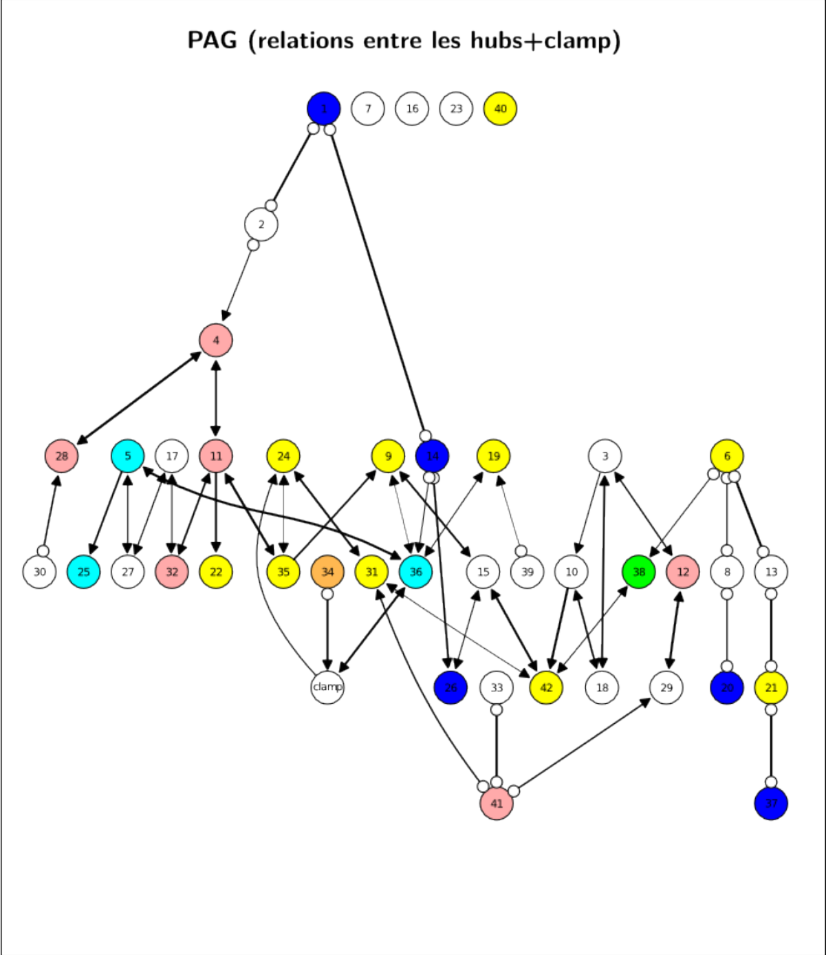
FIGURE 3.6 – Représentation du graphe partiellement ancestral (PAG) estimé par l’algorithme FCI (risque d’erreur \alpha = 0.05 ) sur les hubs des communautés et de la variable clamp. L’épaisseur d’un lien est proportionnelle à sa fréquence d’apparition (sans son orientation) sur les PAGs estimés à partir de 1000 échantillons bootstrap.
