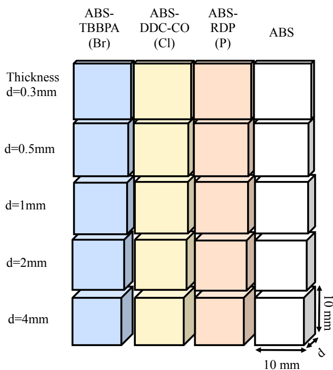
Figure 10: Illustration du fantôme ABS-RF utilisé pour l'imagerie CR spectrale.
