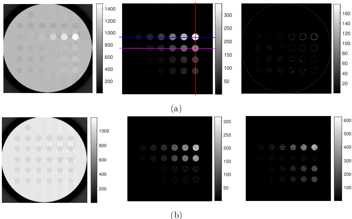
Figure 20: Densité décomposée en unité de mg / cc de base d'eau (colonne de gauche), base de fer (colonne du milieu) et base de potassium (colonne de droite) avec la méthode ima-PR-LS. Paramètres d'acquisition des données: 6 bandes d'énergie, 1 mA·s par projection (a), et 60 bandes d'énergie, 10 mA·s par projection (b).
