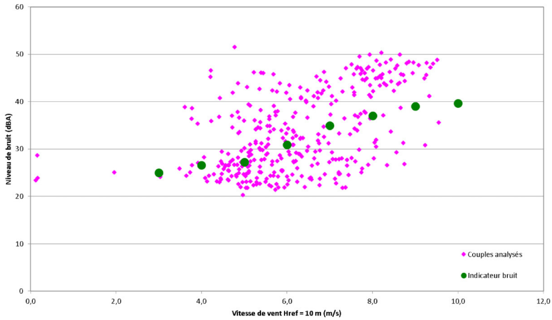
FIGURE 7.1 – Niveaux résiduels observés lors d’une étude acoustique en fonction de la vitesse du vent (losanges roses). Les indicateurs retenus lors de l’étude (ronds verts) ne permettent pas un contrôle optimal du parc éolien.
