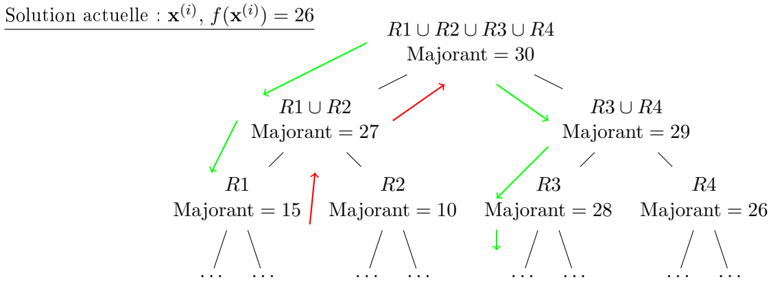
FIGURE 2.4 – Représentation graphique du parcours d'un algorithme branch and bound . En début de parcours, on suppose qu'on connaît une solution non-optimale du problème qui donne une valeur de 26 pour la fonction objectif. Tant que le majorant est plus grand que cette valeur, on continue de s'enfoncer dans l'arborescence de l'arbre (flèches vertes). Lorsque le majorant est inférieur, on supprime le nœud courant et on remonte au nœud père (flèches rouges). Lorsqu'on atteindra une feuille de l'arbre (solution admissible), la valeur de la fonction f sera ainsi nécessairement supérieure.
