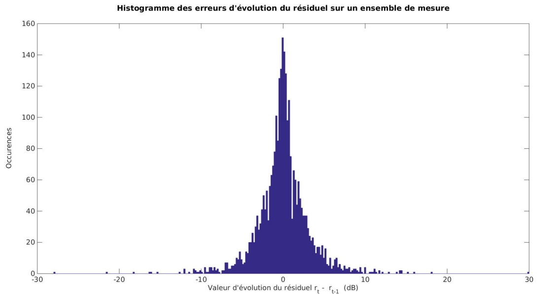
FIGURE 7.4 – Histogramme des évolutions du résiduel sur des données mesurées. Notons que cette distribution est centrée (moyenne de 0 dB) et symétrique (asymétrie statistique \frac{\mu_3}{\mu_2^{3/2}} = -0,14 , où \mu_i est le moment centré d'ordre i ).
