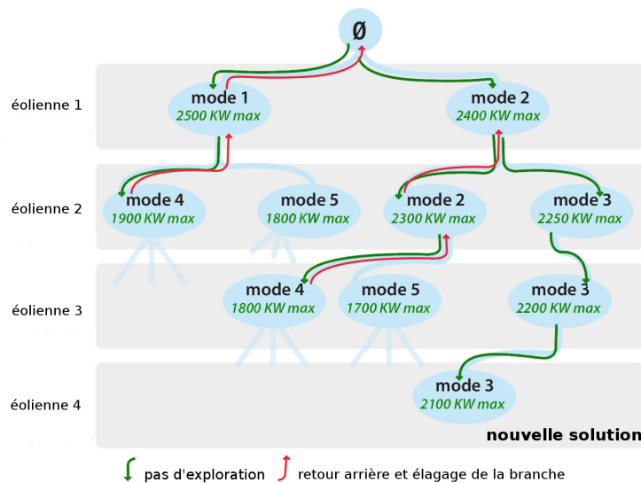
FIGURE 4.2 – Exemple de parcours sur un arbre pour 4 éoliennes et 5 modes de bridage, en partant d'une solution initiale de 2000 kW.
