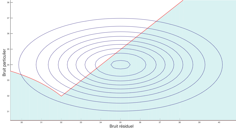
FIGURE 8.1 – Représentation de la loi jointe de [l_t^T \ r_t^T]^T (courbes bleues foncées), de q (courbe rouge) et des solutions admissibles (aire bleue sous la courbe).
