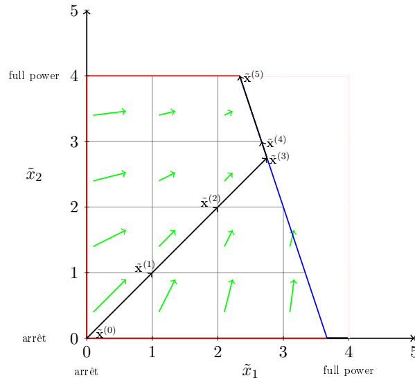
FIGURE 4.7 – Représentation graphique des itérations de l'algorithme de gradient sur l'exemple.
