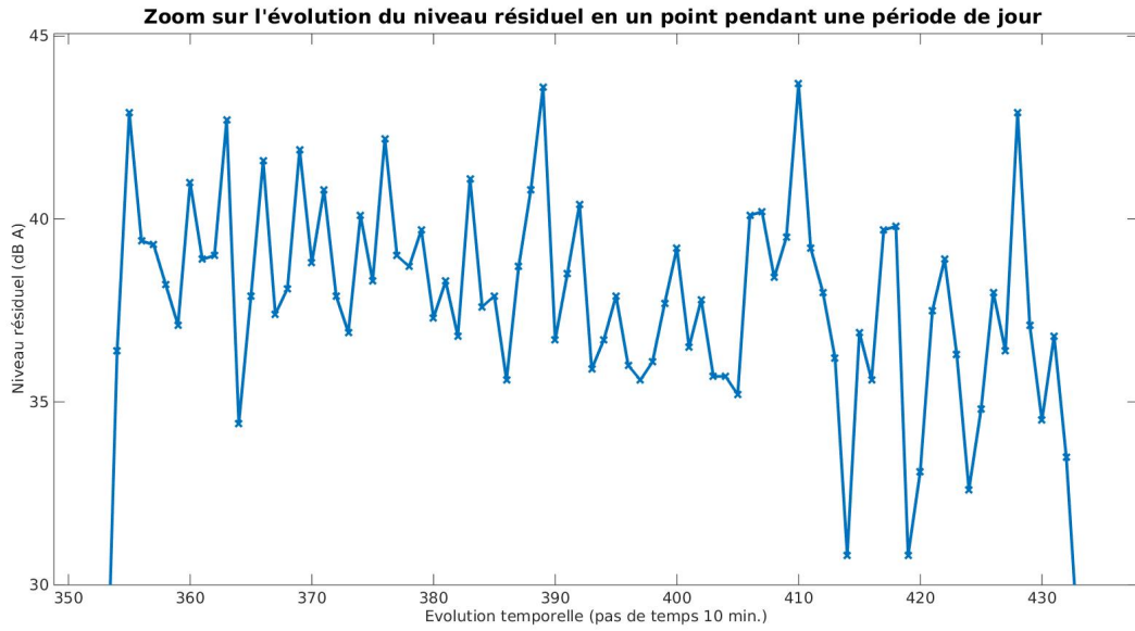
FIGURE 7.3 – Exemple de l'évolution temporelle du niveau résiduel en un point. Zoom sur une période de jour.
