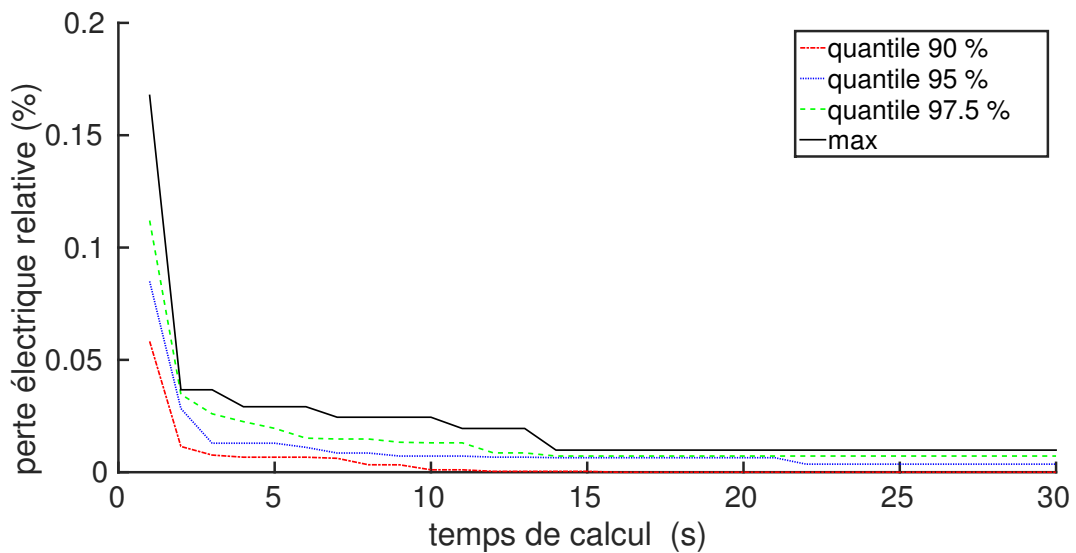
FIGURE 4.12 – Évolution temporelle des erreurs relatives pour l’algorithme branch and bound (variante retenue) pour les échantillons ayant un temps de calcul supérieur à 5 s.
