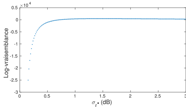
(a) Log-vraisemblance en fonction de l'écart-type sur la séparation.
