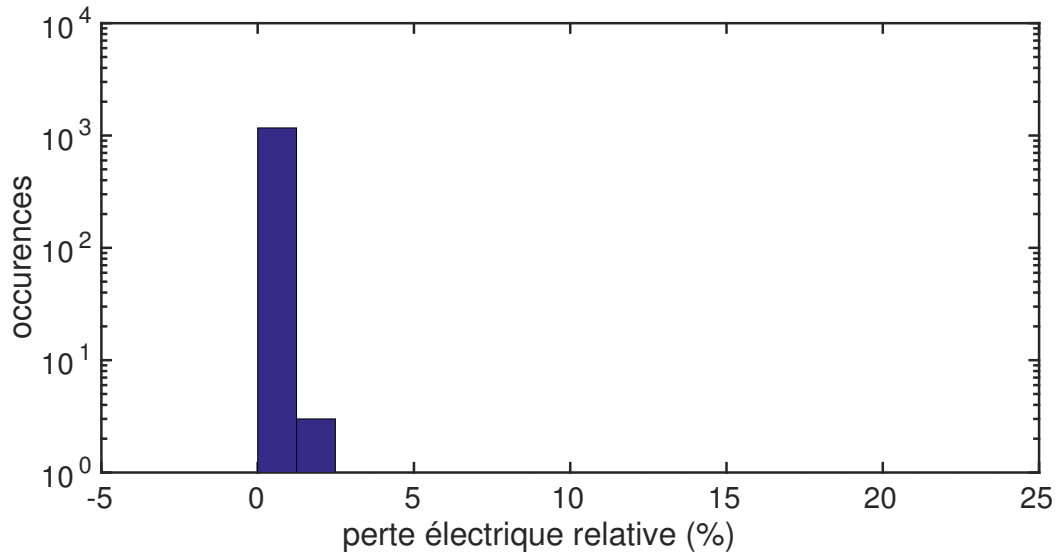
FIGURE 4.11 – Distribution des erreurs relatives pour l’algorithme branch and bound (variante retenue).
