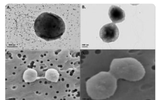
Figure 2: Photos d'un Thermococcus . A,B microscopie à transmission; C,D microscopie à balayage. Les Thermococcus sont des coques d'environ 1 µm de diamètre, ils ne supportent pas l'oxygène (anaérobie), et se nourrissent de sucres, protéines et lipides. Ils sont également capables de se déplacer grâce à leurs flagelles (A,B). (d'après Dalmasso et al., 2016)
