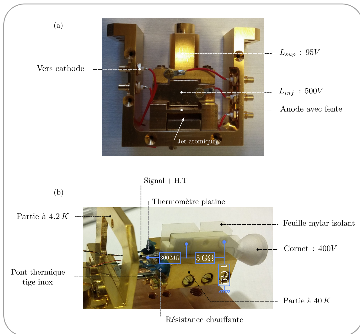
FIGURE II.30 – (a) Photographie de l'intérieur du détecteur. Le jet d'atomes lents est représenté par la flèche blanche. De bas en haut, nous avons la cathode et l'anode permettant l'ionisation puis les lentilles inférieures et supérieures dirigeant les électrons vers le channeltron. L'ensemble des électrodes sont électriquement isolées les unes des autres par l'intermédiaire d'une feuille de mylar. Les divers potentiels sont appliqués soit directement à l'aide d'une cosse vissée sur l'électrode soit par l'intermédiaire d'une vis traversante acheminant le potentiel jusqu'à l'électrode en profondeur, l'isolation par rapport aux autres électrodes est garantie par l'absence de filetage aux travers de ces électrodes et en ajoutant de la gaine thermorétractable sur la partie concernée du corps de la vis. (b) Photographie du channeltron en l'absence d'écran thermique à la température de 4.2 K. Nous avons, en particulier, représenté le pont diviseur de tension, formé des résistances de 1 GΩ, 5 GΩ et 300 MΩ, permettant de répartir la haute tension entre le cornet, la sortie du canal continue formant la dynode et la sortie du channeltron.
