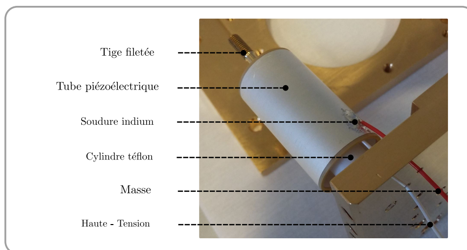
FIGURE II.28 – Assemblage des éléments piézoélectriques. Les tubes piézoélectriques en PIC 151 viennent se glisser sur une pièce en téflon vissée sur la tige filetée. Le fil rouge permet de porter la face externe à la masse tandis que le fil blanc permet d'appliquer une haute tension commune aux quatre tubes, régissant ainsi leur longueur.
