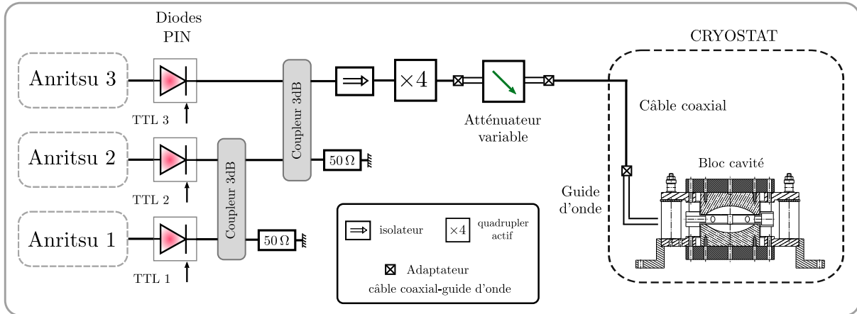
FIGURE II.34 – Ligne de génération du champ micro-onde à l'intérieur du cœur du dispositif expérimental. Les synthétiseurs produisent un signal micro-onde aux alentours de 12.8 GHz. Le signal est ensuite ramené dans la gamme des fréquences d'intérêt via un quadrupleur qui génère l'harmonique de rang 4 aux alentours de 50 GHz. Le signal traverse ensuite un atténuateur variable - dont l'amplitude d'atténuation est ajustée manuellement - puis est envoyé à l'intérieur du cryostat. La durée d'injection est régie par la fermeture du circuit grâce à une diode PIN contrôlée par l'intermédiaire d'un signal TTL.
