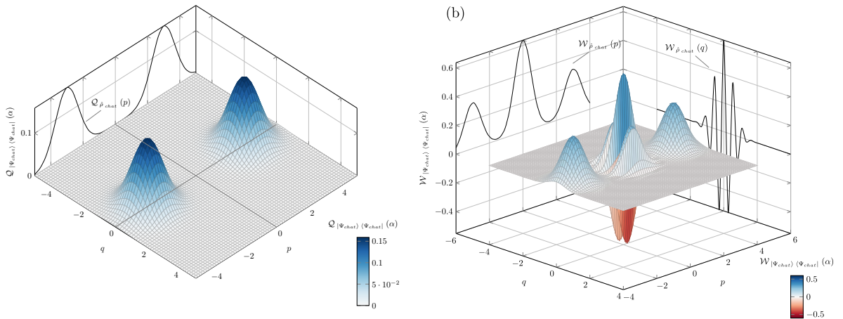
FIGURE I.17 – (a) Représentation dans l'espace des phases de la fonction de Husimi \mathcal{Q}_{chat} , associée à l'état chat de Schrödinger |\Psi_{chat}\rangle = (|3i\rangle + |-3i\rangle)/\sqrt{\mathcal{N}_{chat}} . Nous avons représentés les coupes suivant les axes p et q dans les encarts (b) Représentation dans l'espace des phases de la fonction de Wigner \mathcal{W}_{chat} associée à l'état |\Psi_{chat}\rangle = (|3i\rangle + |-3i\rangle)/\sqrt{\mathcal{N}_{chat}} affichant clairement des valeurs négatives. Nous représentons également les coupes suivant les axes p et q sur le fond des graphiques.
