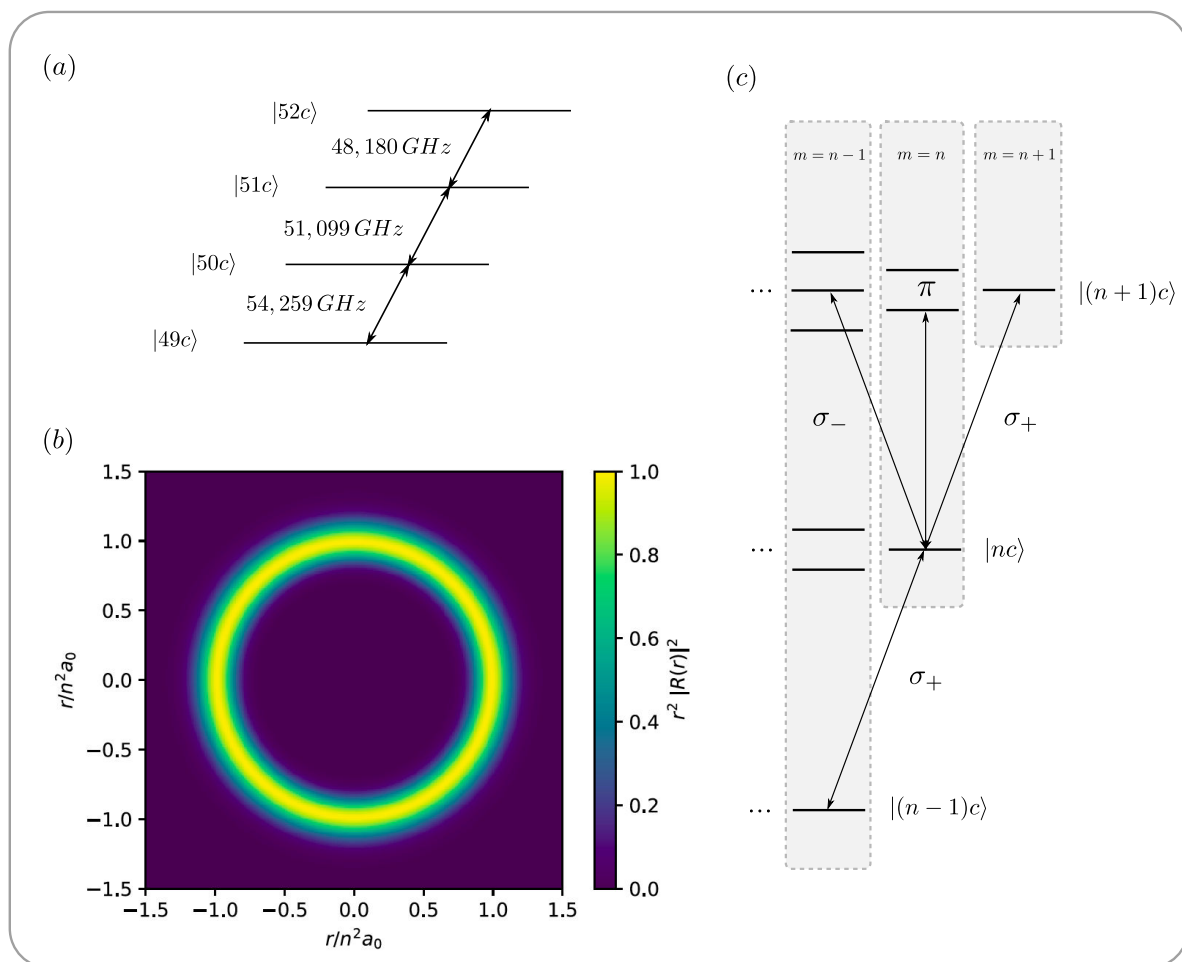
FIGURE I.2 – (a) Diagramme énergétiques des états de Rydberg circulaires |49c\rangle , |50c\rangle , |51c\rangle et |52c\rangle . Les fréquences des transitions entre deux états adjacents sont données au MHz près. (b) Représentation de la densité de probabilité électronique normalisée, suivant le plan ( Oxy ), pour l'état de Rydberg circulaire |n = 51, l = 50, m = 50\rangle . (c) Illustration des transitions énergétiques permises en partant d'un état de Rydberg circulaire quelconque |nc\rangle . En vertu des règles de sélection, ce dernier peut induire des transitions \pi et \sigma_{\pm} vers la multiplicité supérieure mais également se désexciter vers la multiplicité inférieure via une transition de polarisation \sigma_+ .
