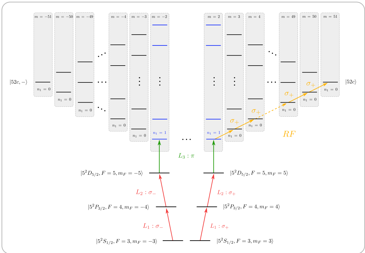
FIGURE II.45 – Diagramme énergétique complet du processus de circularisation permettant d'aboutir à l'état de Rydberg circulaire |52c, +\rangle en partant de l'état de faible moment cinétique orbital |52f, |m| = 2\rangle . La dégénérescence de la polarisation des lasers L_{2,3} fait que nous préparons, à l'issue de l'impulsion laser, les états |52f, m = \pm 2\rangle . Lors du passage adiabatique, le couplage de l'atome avec un champ radiofréquence purement polarisé \sigma_+ permet de briser la symétrie de préparation, seuls les atomes se trouvant dans l'état |52f, m = 2\rangle se voient porter dans l'état de Rydberg circulaire |52c, +\rangle .
