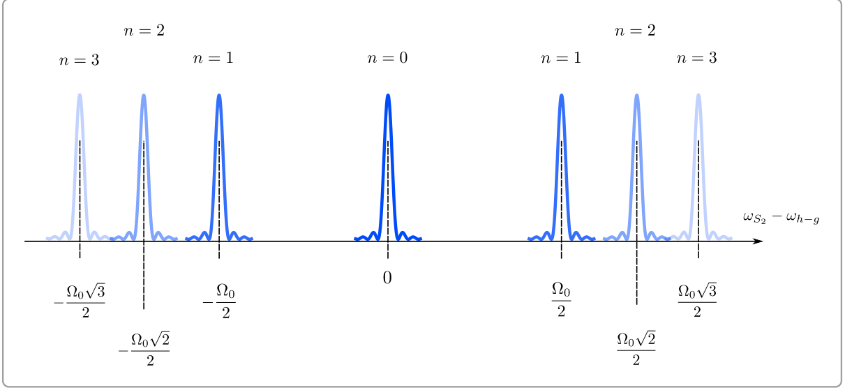
FIGURE I.26 – Illustration schématique du spectre aux alentours de la transition atomique \Delta_0 : |h, 0\rangle \rightarrow |g, 0\rangle . Nous observons deux ensembles de raies. L'un vers les hautes fréquences par rapport à la transition \Delta_0 , correspondant à l'ensemble des transitions \Delta_{+,n} . L'autre vers les basses fréquences par rapport à la transition \Delta_0 , correspondant à l'ensemble des transitions \Delta_{-,n} . Chacun de ces ensembles exhibe des transitions dont les fréquences réalisent une bijection avec l'ensemble des entiers correspondant aux nombres de photons dans la cavité.
