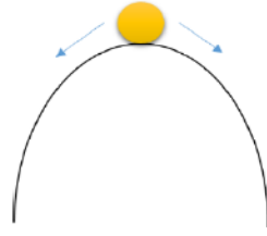
Figure 48 : Situation d'équilibre instable : des perturbations appliquées sur la balle jaune la conduiront à quitter définitivement sa position d'origine
