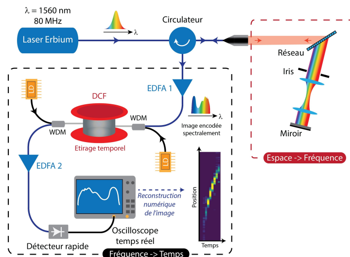
FIGURE 4.7 – Schéma du montage d'imagerie par étirage temporel
