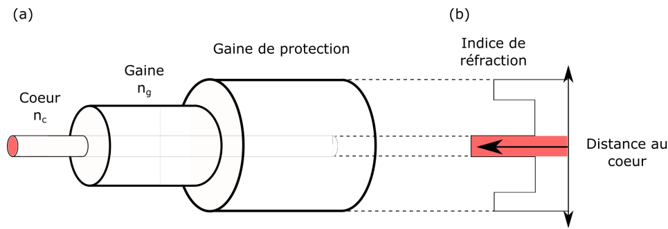
FIGURE 2.1 – Représentation d’une fibre optique à saut d’indice de réfraction. (a) La fibre est composée du cœur et de la gaine, d’indices de réfraction différents. (b) Le guidage de la lumière est imposé par la différence d’indice entre cœur et gaine.
