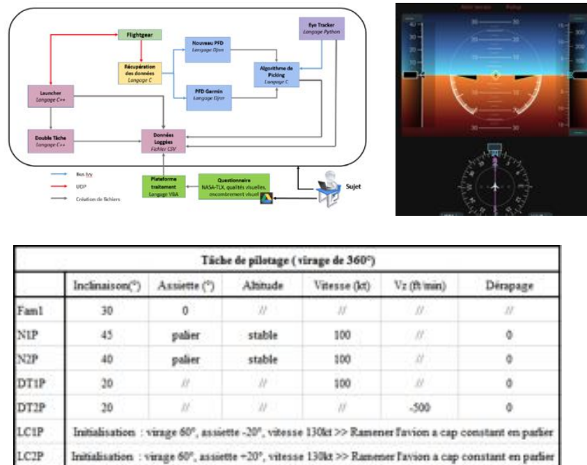
Figure 153: intégration des prototypes avec un simulateur de vol, conception graphique et protocole expérimental pour évaluer le nouvel instrument de pilotage
