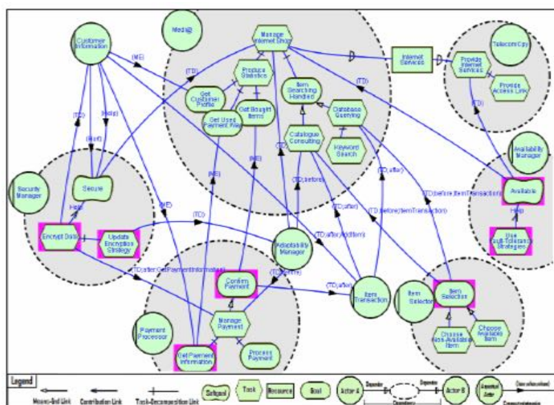
Figure 33: un modèle de buts utilisant la notation i^* issu de (Castro et al. 2009)
