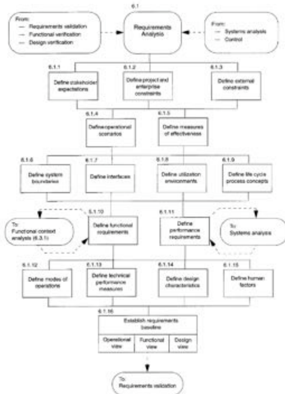
Figure 10: les activités prescrites par IEEE 1220 sur l'ingénierie des exigences
