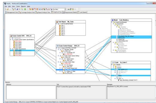
Figure 44: visualisation des traces sur Reqify
