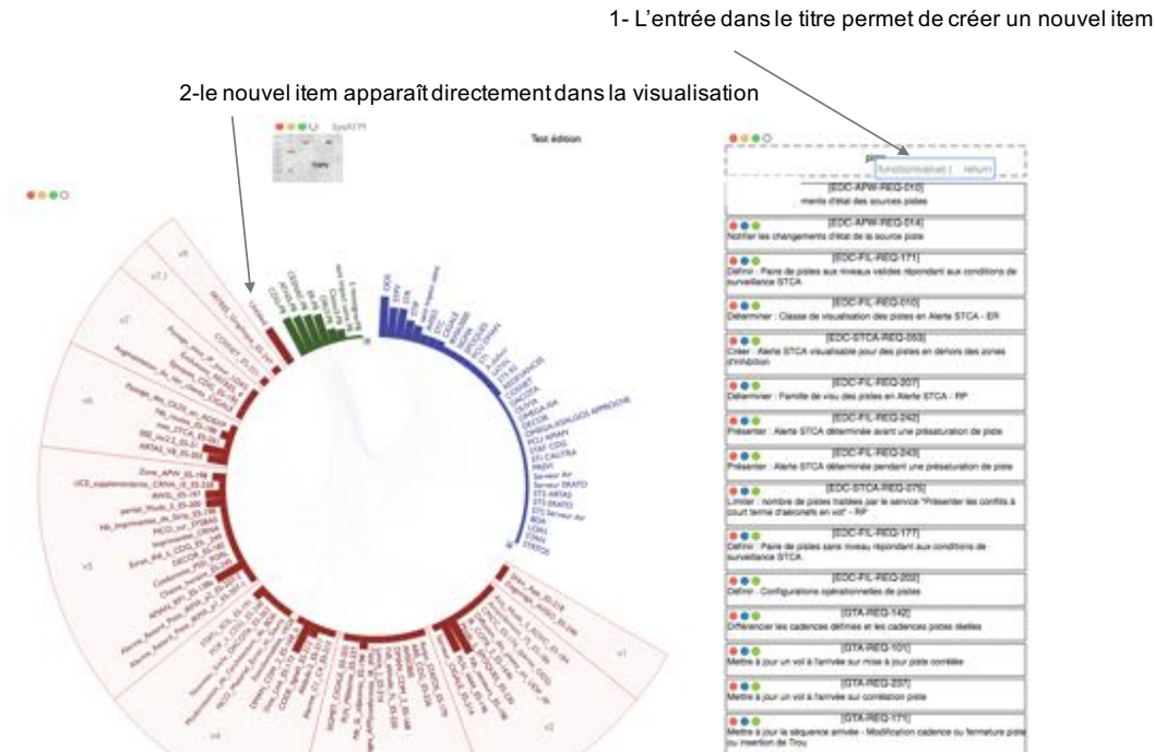
Figure 116: synchronisation des visualisations à la création d'un item
