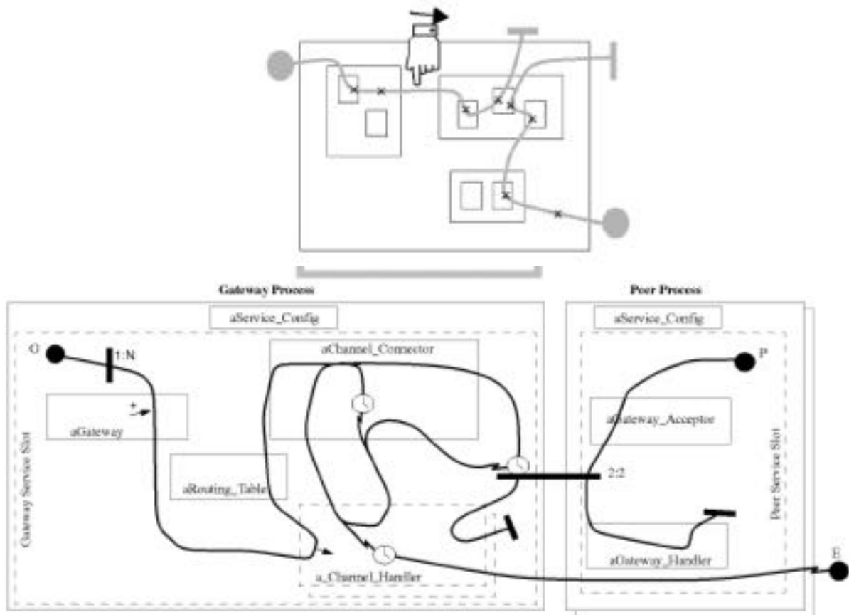
Figure 30: principe de la notation de Use Case Map et exemple (Buhr 1998)
