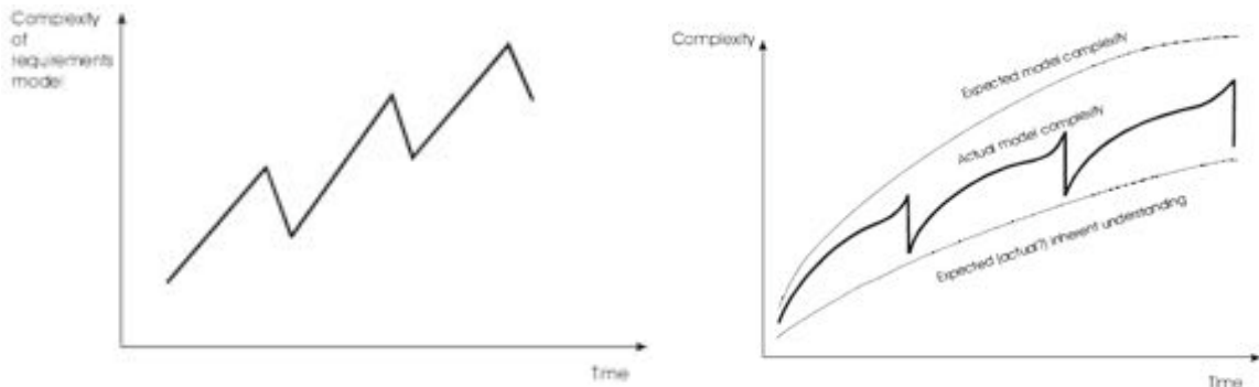
Figure 36: l'évolution de la complexité des modèles, observée par (Nguyen et Swatman 2000)
