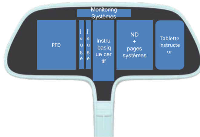
Figure 141: proposition de cockpit, avec les instruments basiques pour la certification, les jauges et la tablette instructeur
