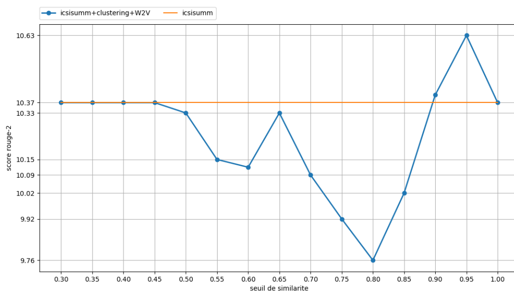
FIGURE 4.4 – Influence du seuil de similarité sur TAC 2009 en utilisant les vecteurs Word2Vec
