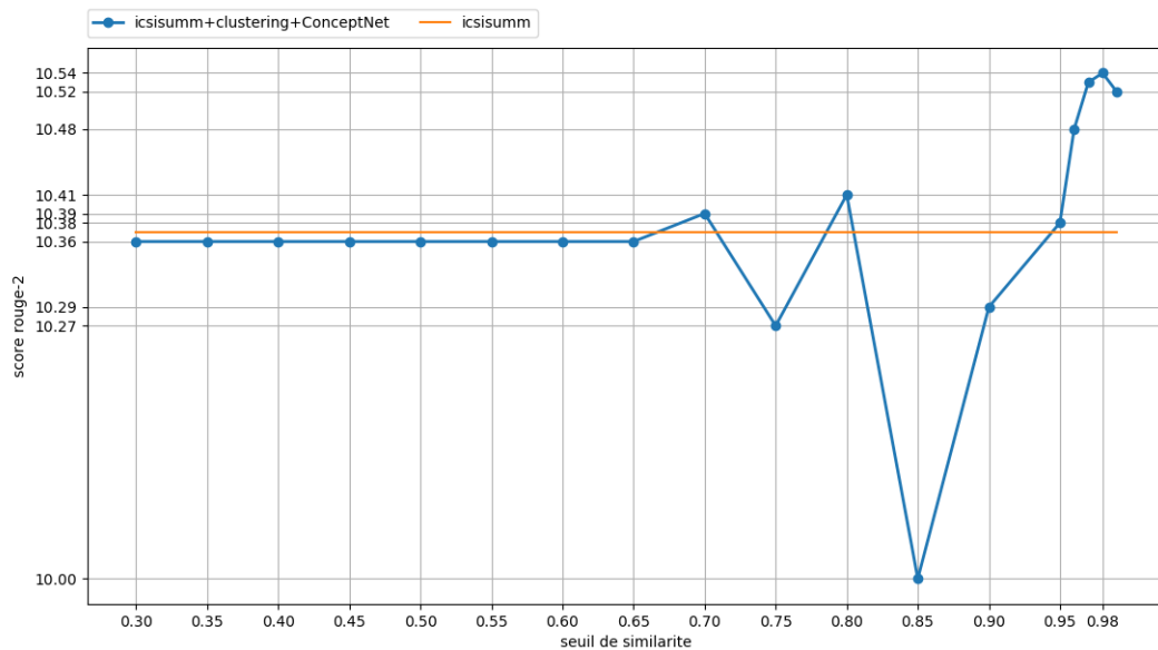
FIGURE 4.6 – Influence du seuil de similarité sur TAC 2009 en utilisant les vecteurs ConceptNet
