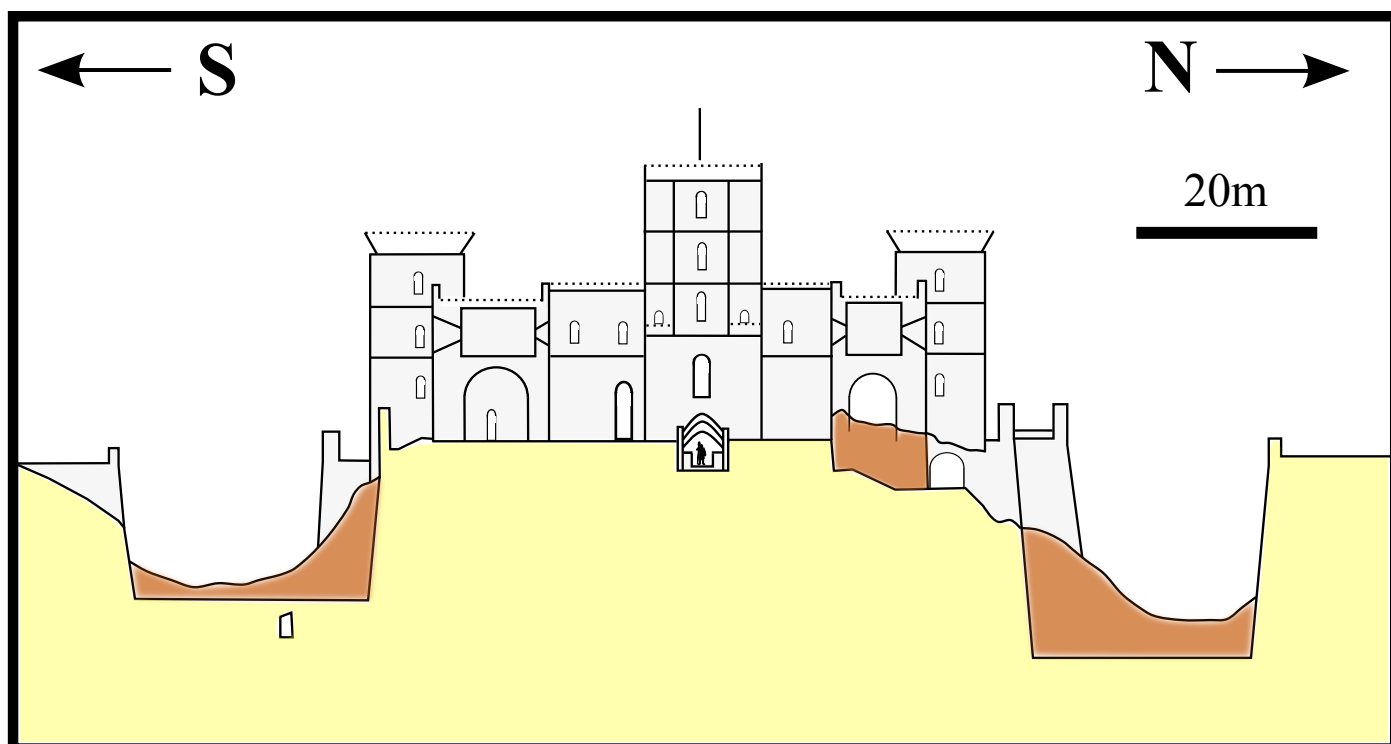
Plan 2 - Le Château d'Arsur (milieu XIIIe siècle) Haut : vue en coupe Bas : vue de front
