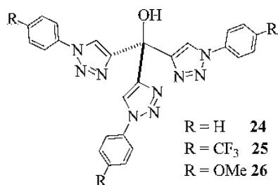
Fig. 31. Tris(aryltriazolyl)methanol ligands.
