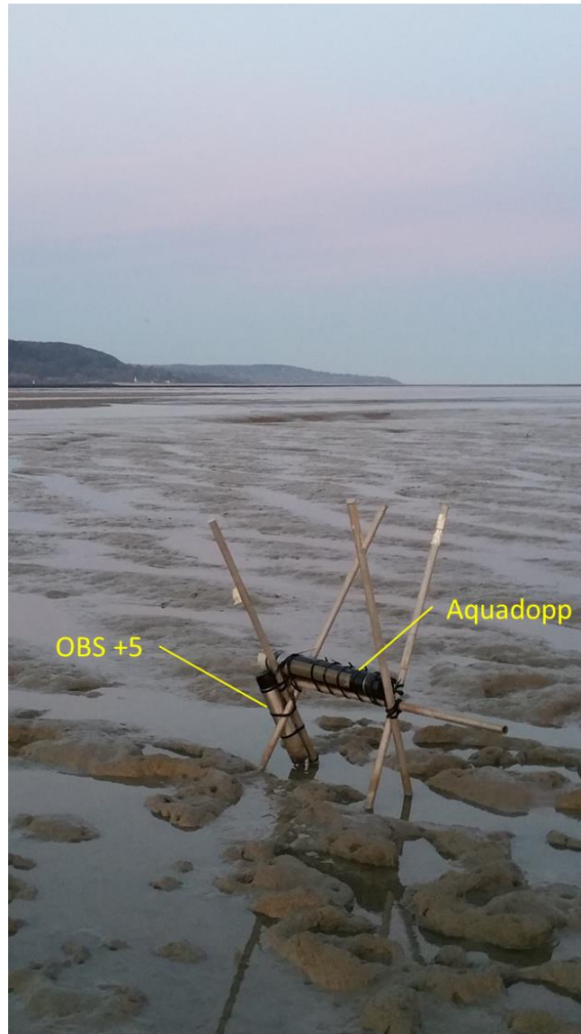
Figure 29 Photographie de l'Aquadopp (implanté de façon horizontale dirigé vers le chenal) et l'OBS-5+ (fixé sur un des mats avec les capteurs regardant vers le haut) (Photo : Vennin, 2017)
