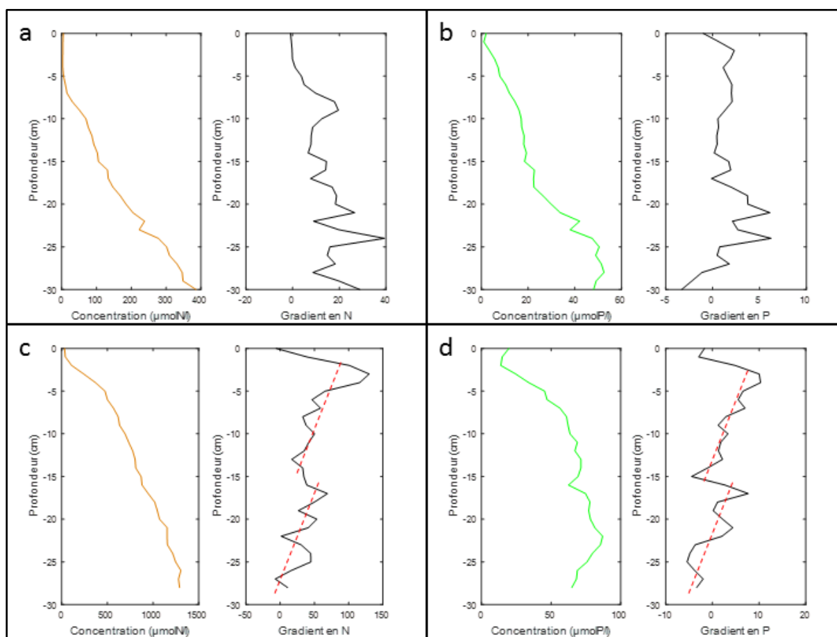
Figure 51 Comparaison entre les valeurs de concentration mesurées dans le sédiment (en orange et vert) et le gradient de concentration associé (en noir) pour la vasière d'embouchure (a et b) et la vasière fluviale intertidale (c et d).
