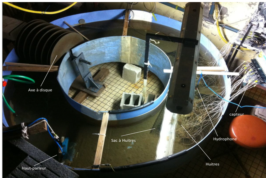
FIGURE 3.2 – Illustration du dispositif expérimental pour la caractérisation du sens de l'audition chez l'huître Magallana gigas . Volume : 350 L, diamètre extérieur : 2 m, diamètre intérieur : 1 m.
