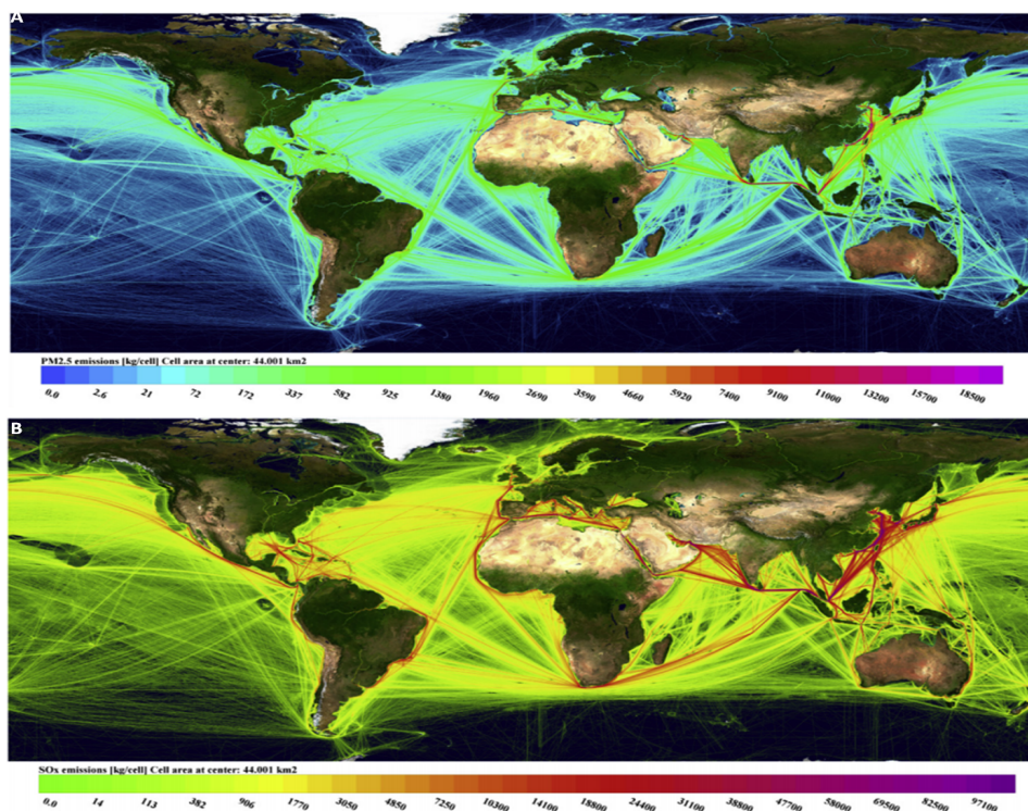
FIGURE 2.11 – Modélisation de la répartition géographique des émissions de particules fines ( PM_{2,5} , A) et de dioxyde de soufre ( SO_x , B) provenant du trafic maritime en 2015. (JOHANSSON et al., 2017).
