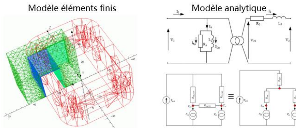
Fig. 7. Les modèles éléments finis et analytique du transformateur
