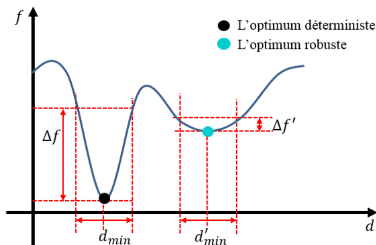
Fig. 2. L'optimum déterministe et l'optimum robuste
