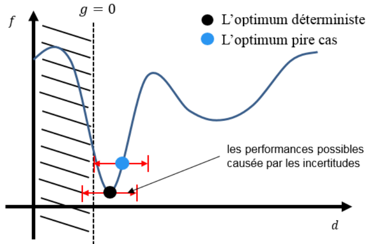
Fig. 1. L'optimum déterministe, l'optimum du pire cas et l'ensemble d'incertitude
