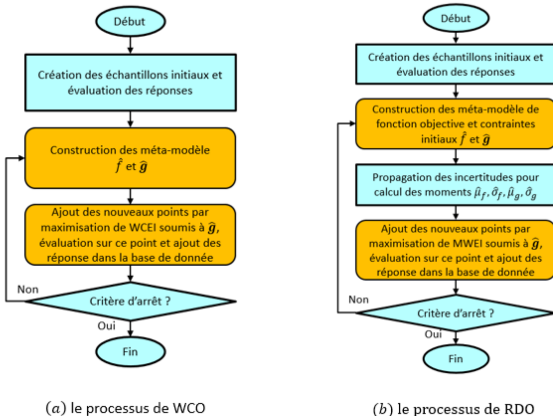
Fig. 5. Les processus de WCO et RDO avec méta-modèle
