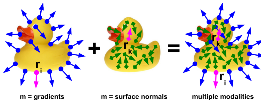
FIGURE 3.8 – RECONNAISSANCE VISUELLE — Illustration de l'algorithme Linemod effectuant l'identification d'objets visuels. Un objet est défini selon plusieurs modalités. ( gauche ) les gradients de l'image sont principalement déterminés à partir des contours de l'objet, ( Milieu ) Normales de surface déterminés par le corps de l'objet, ( Droite ) l'approche Linemod combine ces deux informations afin d'émettre une hypothèse sur la présence d'un objet (figure d'après [257]).
