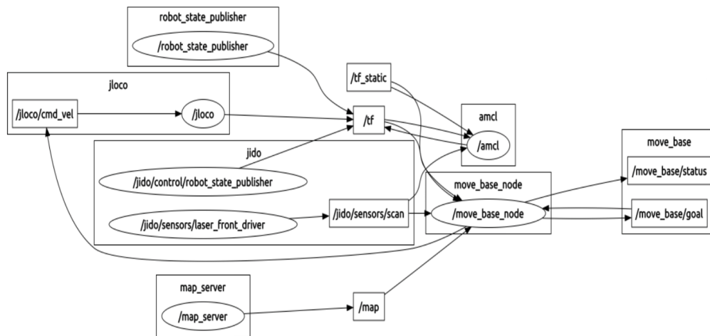
FIGURE 3.15 – Interaction entre les composants requis pour la navigation du robot. (ellipses) nœuds ROS; (boîtes) topique ROS; (boîtes incluant) namespaces regroupant les ressources similaires.
