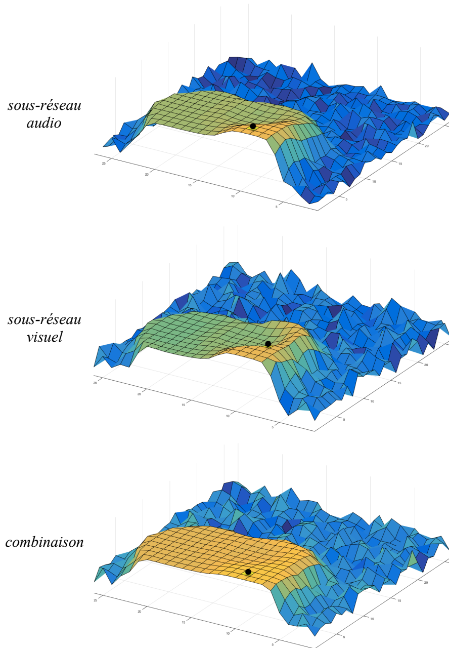
FIGURE 6.7 – MSOM EXEMPLE — Distances euclidiennes normalisées entre un vecteur appartenant à la catégorie male speech et ( haut ) les nœuds du sous-réseau audio, ( centre ) les nœuds du sous-réseau visuel. ( bas ) Combinaison des deux matrices de distances obtenues. ( cercle noir ) nœud gagnant, c'est-à-dire celui dont le vecteur de poids associé à la distance au vecteur d'entrée la plus faible. A des fins de clarté, l'opposé des distances a été représenté : les zones les plus élevées de la carte correspondent aux nœuds ayant la distance la plus faible.
