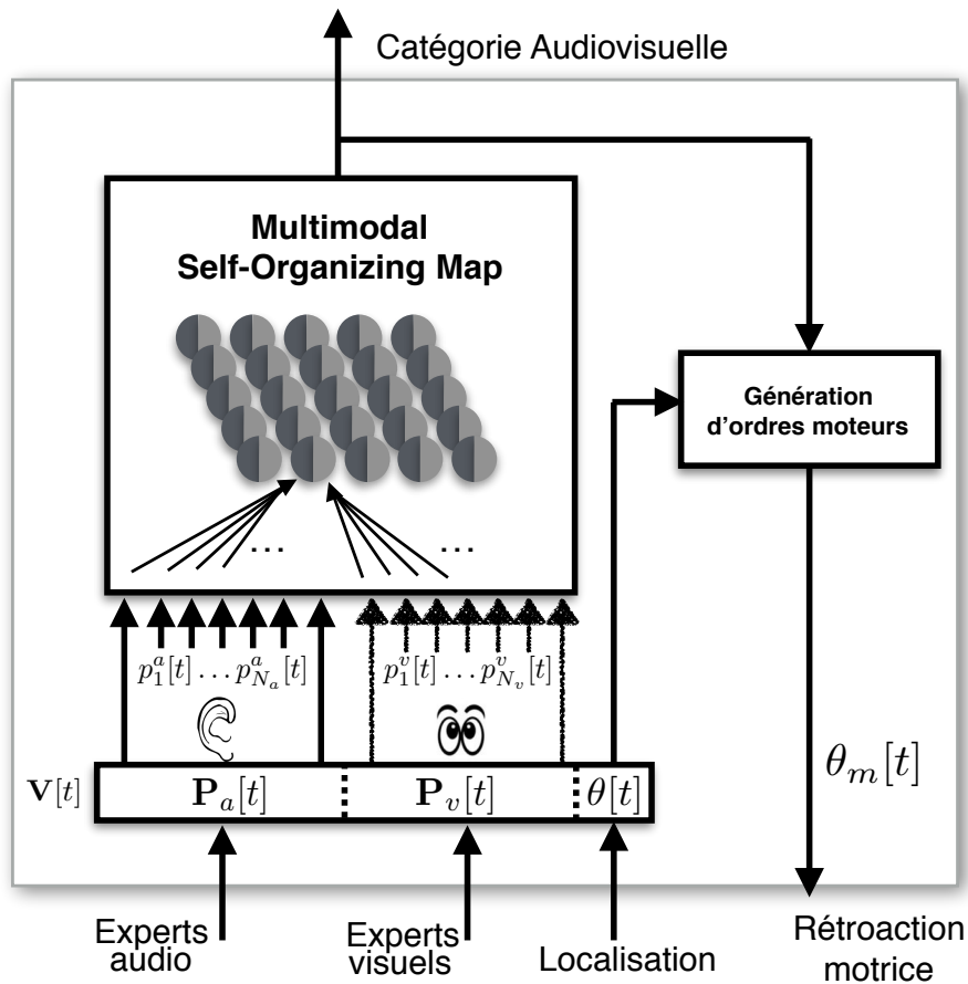
FIGURE 6.1 – Architecture globale du module MFI. Les données issues des experts d'identification sont envoyées au Multimodal Self-Organizing Map (Sec. 6.2) pour l'apprentissage du lien entre la modalité audio et la modalité visuelle. Le module MFI est également responsable de la génération de mouvements de tête, sur la base de la sortie de l'expert de localisation. Le module MFI a pour but d'estimer la catégorie audiovisuelle de l'objet perçu au temps t .
