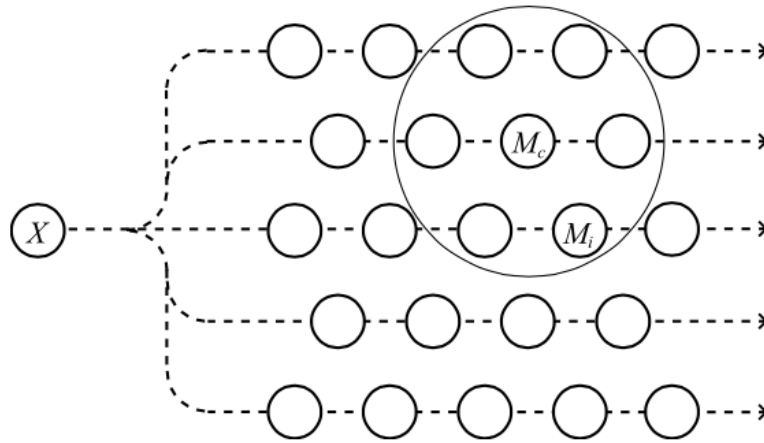
FIGURE 2.23 – CARTE AUTO-ORGANISATRICE — Illustration d'une carte auto-adaptatrice ( Self-Organizing Map ). Un vecteur d'entrée est envoyé à un ensemble de modèles (ou nœuds) M_i . Parmi tous ces modèles, M_c est celui qui représente le mieux la donnée d'entrée. Une étape d'apprentissage correspond à étendre cette similarité entre M_i et M_c à tous les modèles présents dans le voisinage direct de M_c (de [206]).
