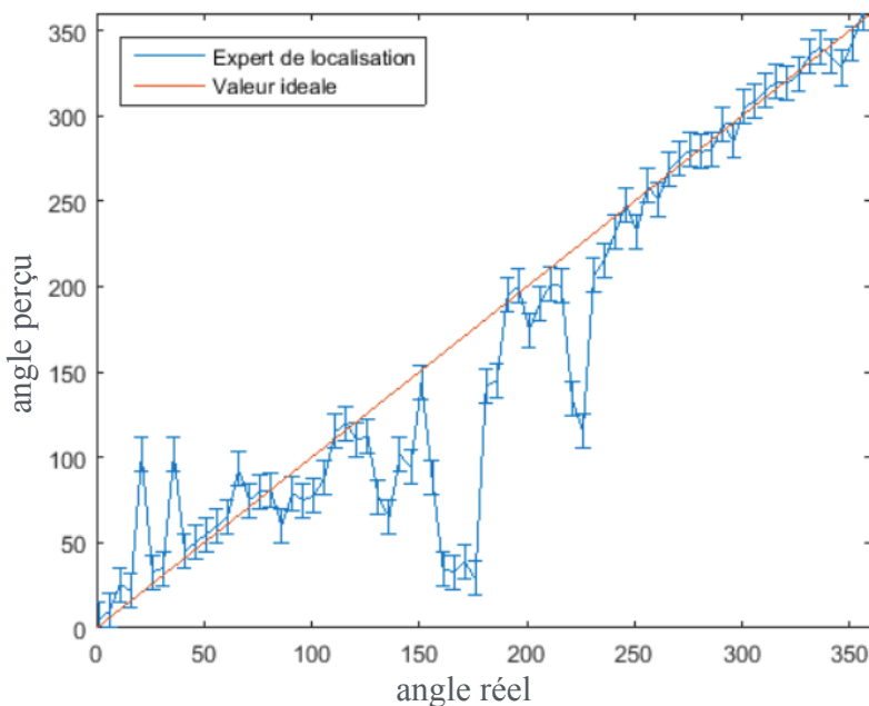
FIGURE 7.10 – TESTS DE L'EXPERT DE LOCALISATION — Effectué dans la salle de test de l'ISIR, ces résultats sont les moyennes de dix estimations successives de la position en azimuth d'une source sonore se déplaçant par pas de 5^\circ , effectuée par l'AUDIOLOCATIONKS utilisée en mai 2016. Une KS utilisant un apprentissage basé sur des réseaux de neurones profonds, la DnnLocationKS, est désormais utilisée. Ses performances sont légèrement meilleures.
