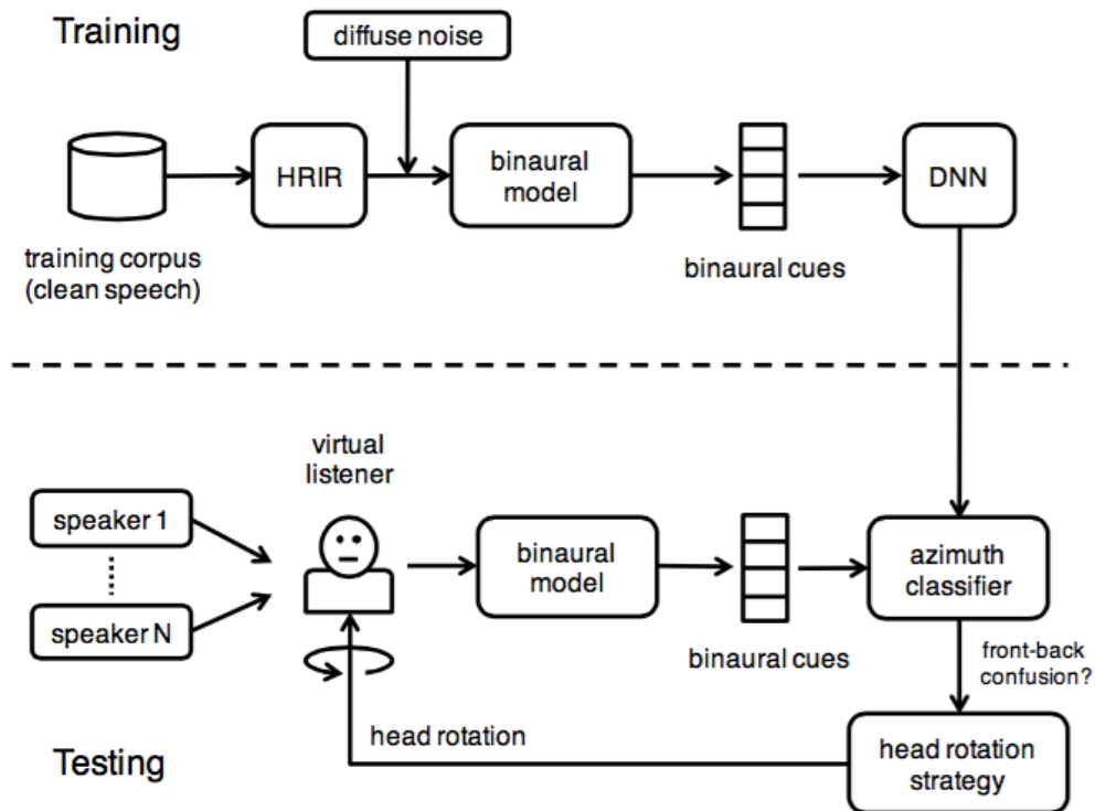
FIGURE 3.5 – SCHÉMA DU SYSTÈME DE LOCALISATION — ( haut ) Apprentissage, ( bas ) validation. Durant la phase de test, la scène sonore consistant en plusieurs locuteurs est simulée dans un environnement virtuel dans lequel un récepteur binaural est mû afin de simuler la rotation de la tête d'un auditeur humain.
