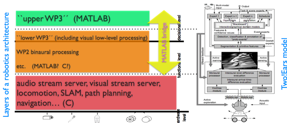
FIGURE 3.9 – De la modélisation computationnelle du projet TWO!EARS ( droite ) à une architecture logicielle robotique temps réel ( gauche )
