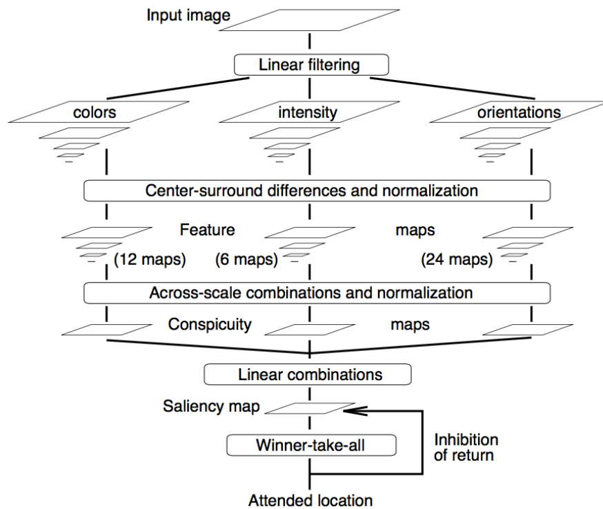
FIGURE 2.19 – CARTE DE SAILLANCE VISUELLE SELON ITTI et al. — (figure d'après [175]).
