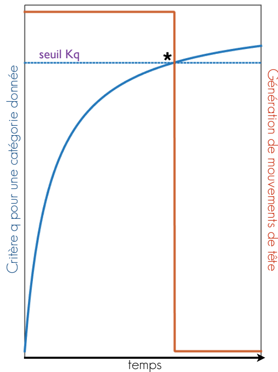
FIGURE 6.5 – CRITÈRE q — Illustration de l'impact du critère q sur la génération de mouvements de tête, pour une catégorie donnée : (bleu) critère q , (rouge) nombre de mouvements de tête, (*) point où q = K_q . C'est à partir de ce point que le module MFI juge qu'il peut faire confiance en ses connaissances sur cette catégorie audiovisuelle et ainsi ne plus requérir de mouvements de tête.
