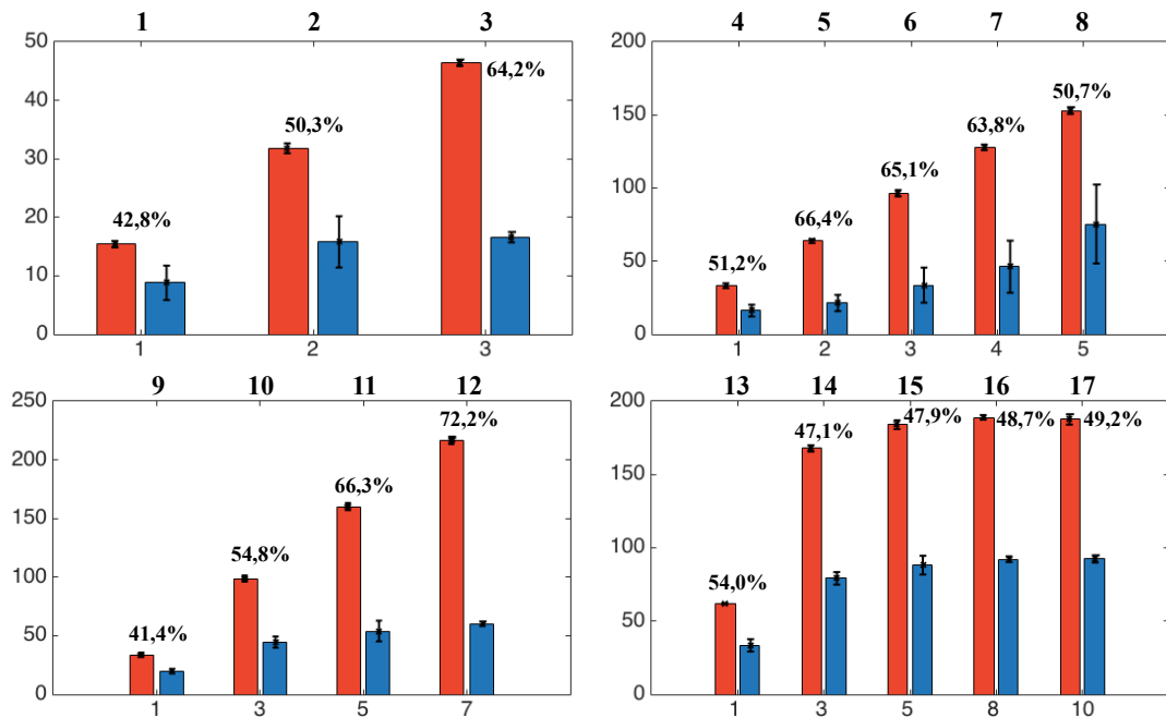
FIGURE 5.8 – NOMBRE DE MOUVEMENTS DE TÊTE GÉNÉRÉS PAR LE DW — Histogramme des mouvements de tête générés par ( rouge ) le robot naïf et ( bleu ) le module DW. 17 conditions différentes ont été créées (se référer au texte pour leur description) pour cette évaluation, chaque condition ayant été testée cinq fois. Chaque histogramme représente la moyenne sur ces cinq tests, les barres d'erreurs représentant l'écart-type. Les nombres représentent le rapport entre les deux nombres de mouvements générés, en pourcentage. Enfin, les numéros au-dessus des graphes correspondent au numéro de l'environnement simulé (cf. Tab. 5.2 ).
