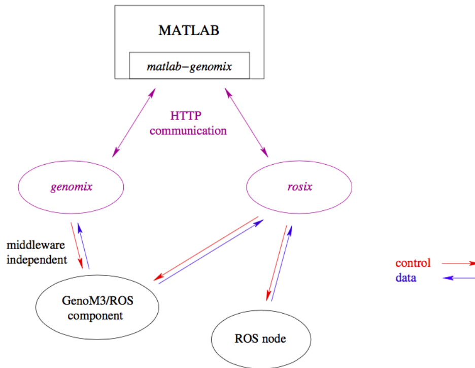
FIGURE 3.14 – MATLAB ROS BRIDGE — Utilisation de genomix et rosix afin de faire un pont entre ROS et MATLAB ® . genomix permet de contrôler les composants GenoM3 et de lire leurs flux de données, indépendamment du middleware employé. rosix peut contrôler et lire les données de n’importe quel nœud ROS de la couche fonctionnelle. matlab-genomix peut être un client de n’importe quel serveur genomix ou rosix .
