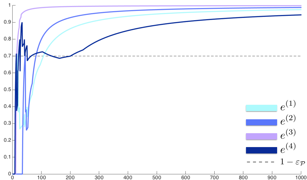
FIGURE 6.17 – TAUX DE CLASSIFICATION DANS DIFFÉRENTS ENVIRONNEMENTS — Chaque courbe représente le taux de classification \bar{\Gamma}_{\text{MFI}}^a dans chacun des quatre environnements simulés. (ligne pointillée) 1 - \varepsilon_{\mathcal{P}}
