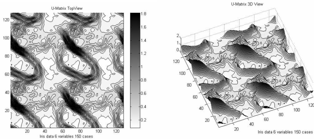
FIGURE 6.2 – U-MATRIX — Représentation en nuances de gris de la distance entre chaque neurone et ses neurones voisins selon la méthode de « U-Matrix » développée par ALFRED ULTSCH [264]. Plus la nuance de gris est claire, plus la distance est faible. Les données employées ici sont issues des données Iris de Fisher [266] (figure d'après [265]).
