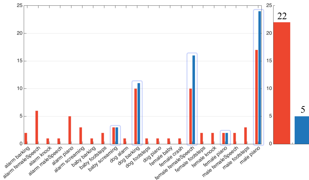
FIGURE 7.14 – CATÉGORIES AUDIOVISUELLES DÉTECTÉES — Illustration de la différence entre le système de fusion « naïf » et le module MFI du point de vue du nombre de catégories audiovisuelles différentes détectées par ( rouge ) le système naïf, ( bleu ) le module MFI. ( gauche ) La hauteur des histogrammes représente le nombre de trames pour lesquelles la catégorie audiovisuelle considérée a été le résultat de la fusion des experts. Les rectangles bleu clair mettent en avant les catégories audiovisuelles communes entre les deux systèmes. ( droite ) nombre total de catégories audiovisuelles différentes détectées.
