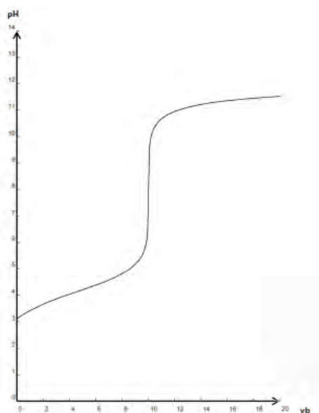
Figure 2 : évolution du pH au cours de titrage de 10 mL d'acide éthanique 10^{-2} mol.L -1 par une solution de soude 10^{-2} M
